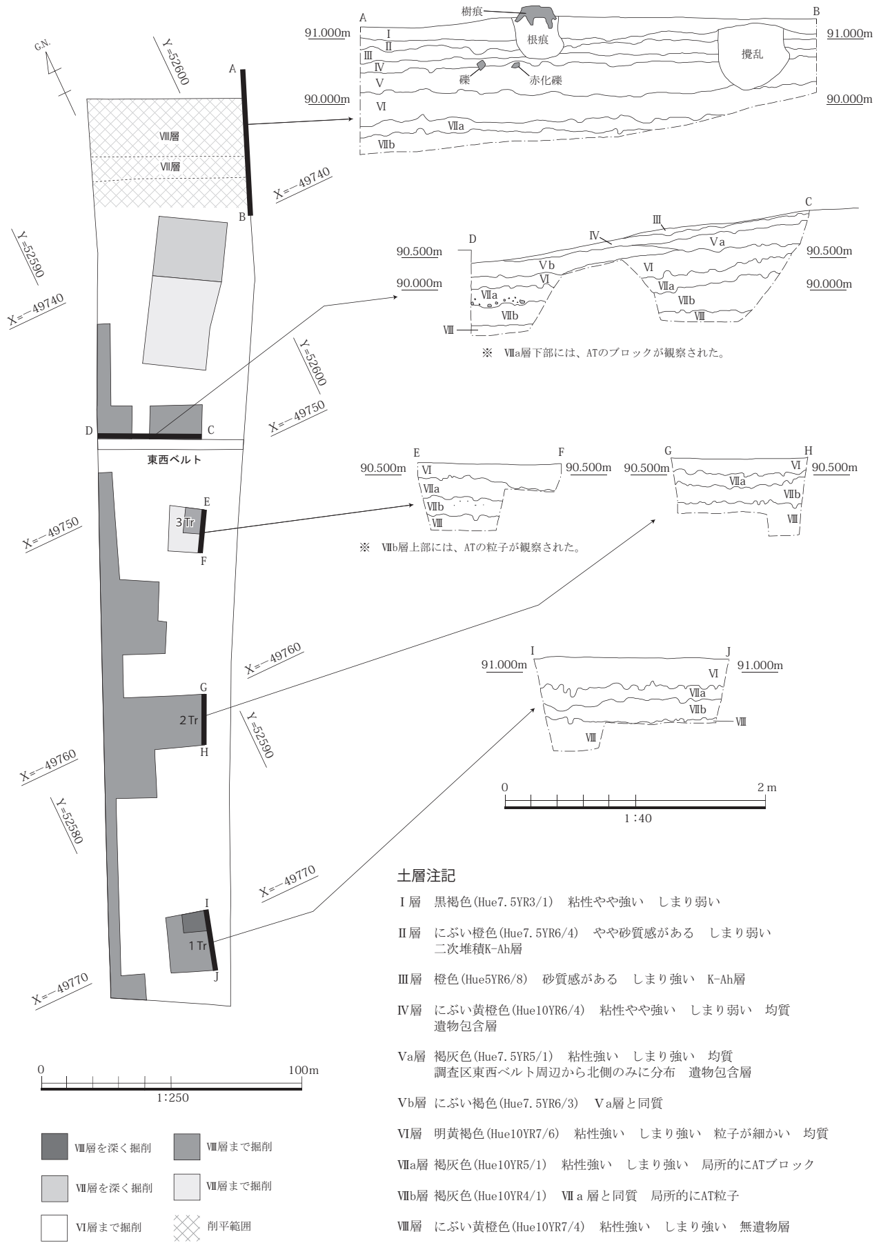
第3図 Tr配置図及び土層断面図
