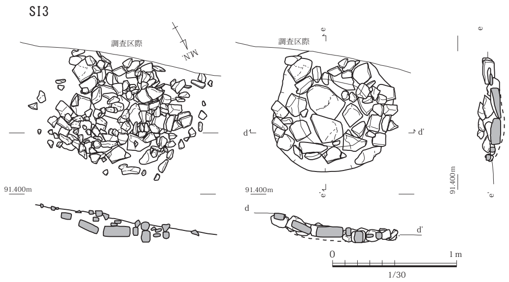
第5図 集石遺構実測図1 (S=1/30)
