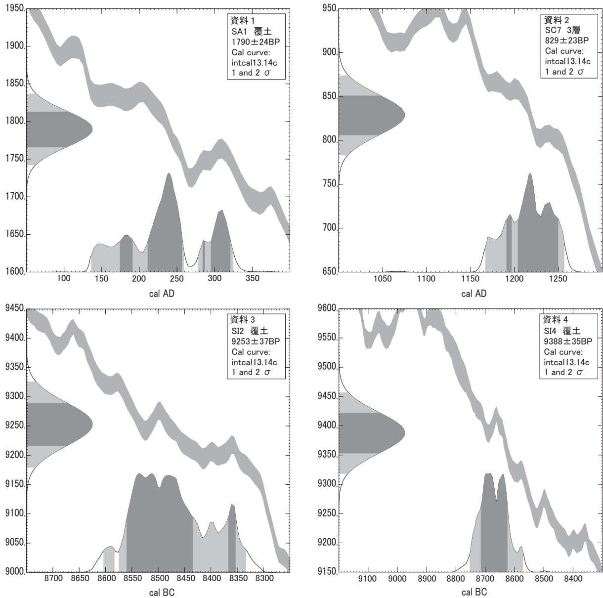
第18図 暦年較正曲線図
