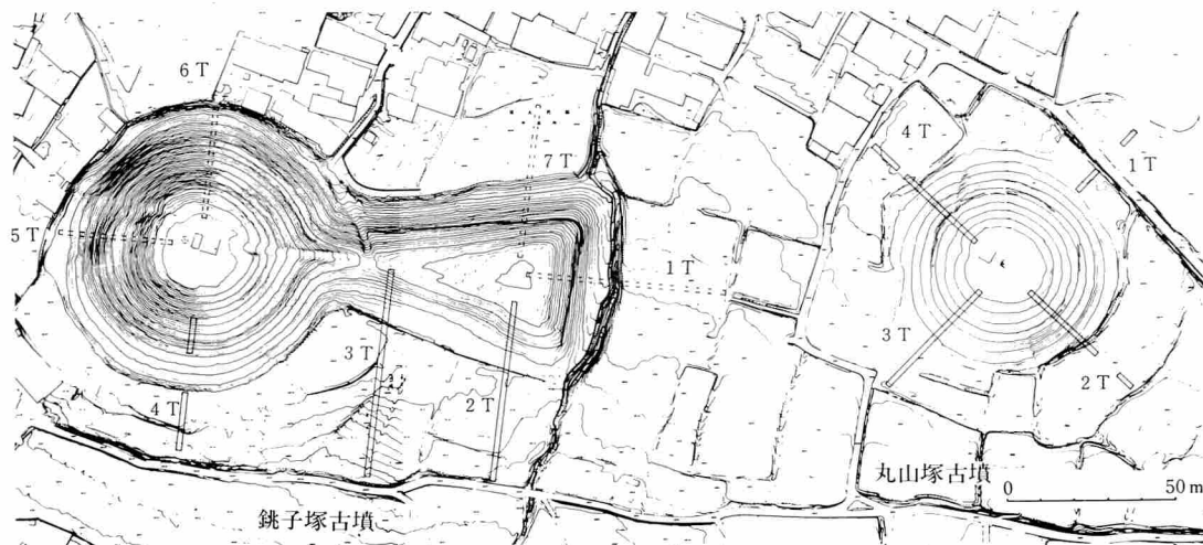
第2図 トレンチ配置図
