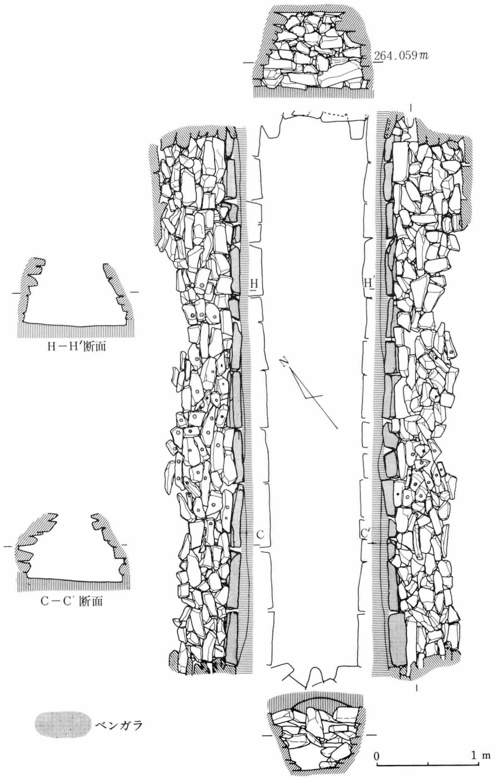
第9図 丸山塚古墳石室展開図
