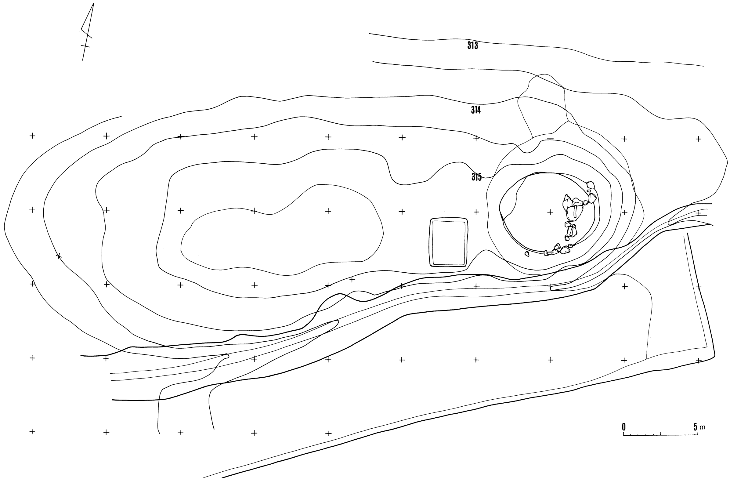
第3図 鍋弦塚地形図
