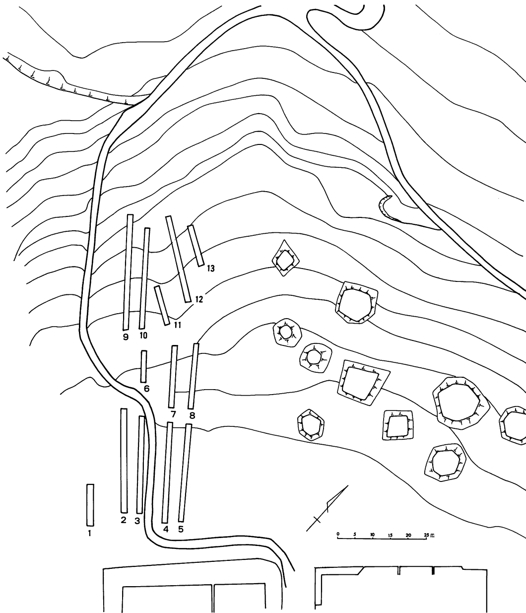
第12図 東山南遺跡調査区全体図
