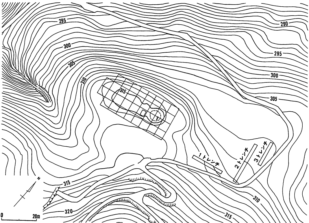
第2図 調査地区全体図
