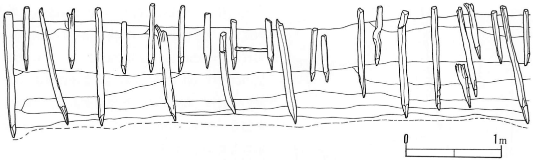
第一面 3号杭列側面図（部分）（1/40）
