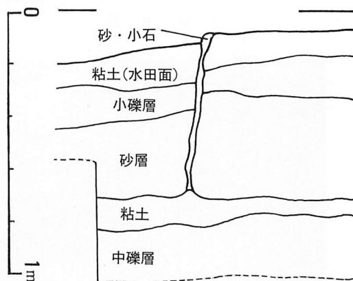
地割れ断面(噴砂)図(1/20)
