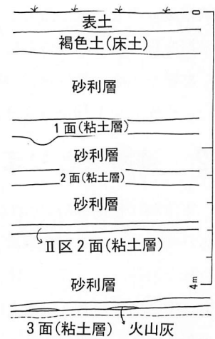
土層断面模式図 (1/80)
