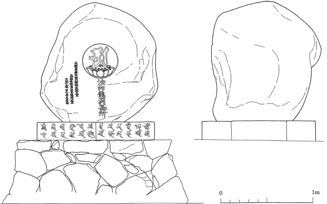
图1 閻魔堂境内阿字觀碑・龍淵墓 実測図
