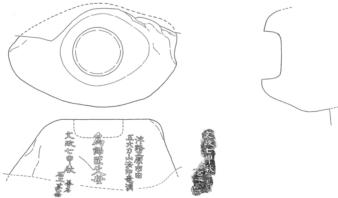
図6 閻魔堂参道入口の手水鉢 実測図
