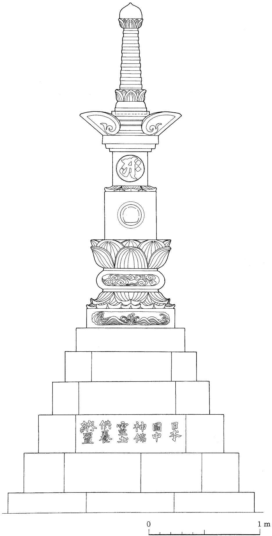
大岩山日石寺宝篋印塔 実測図
