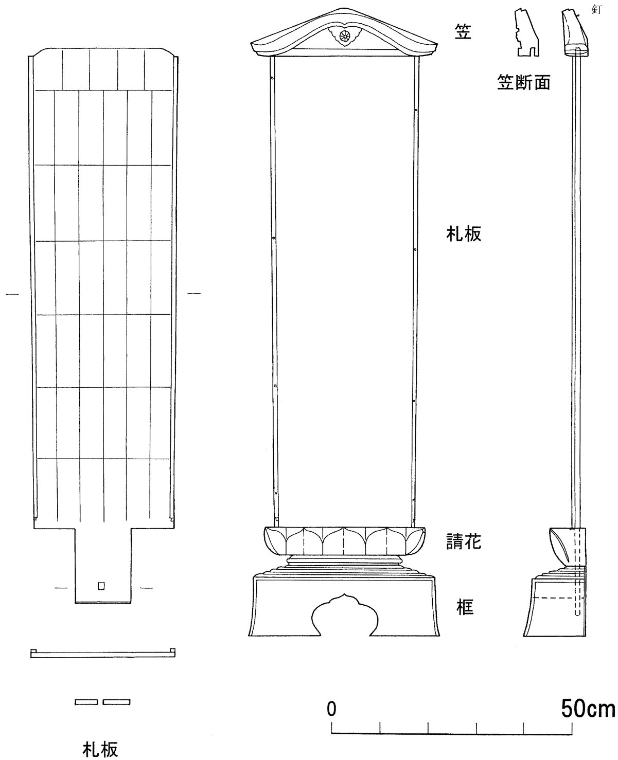
图1 佐伯家位牌 実測図
