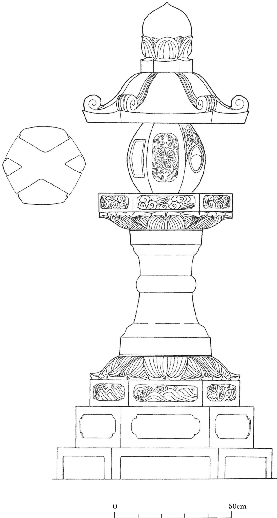
西光寺燈籠 実測図
