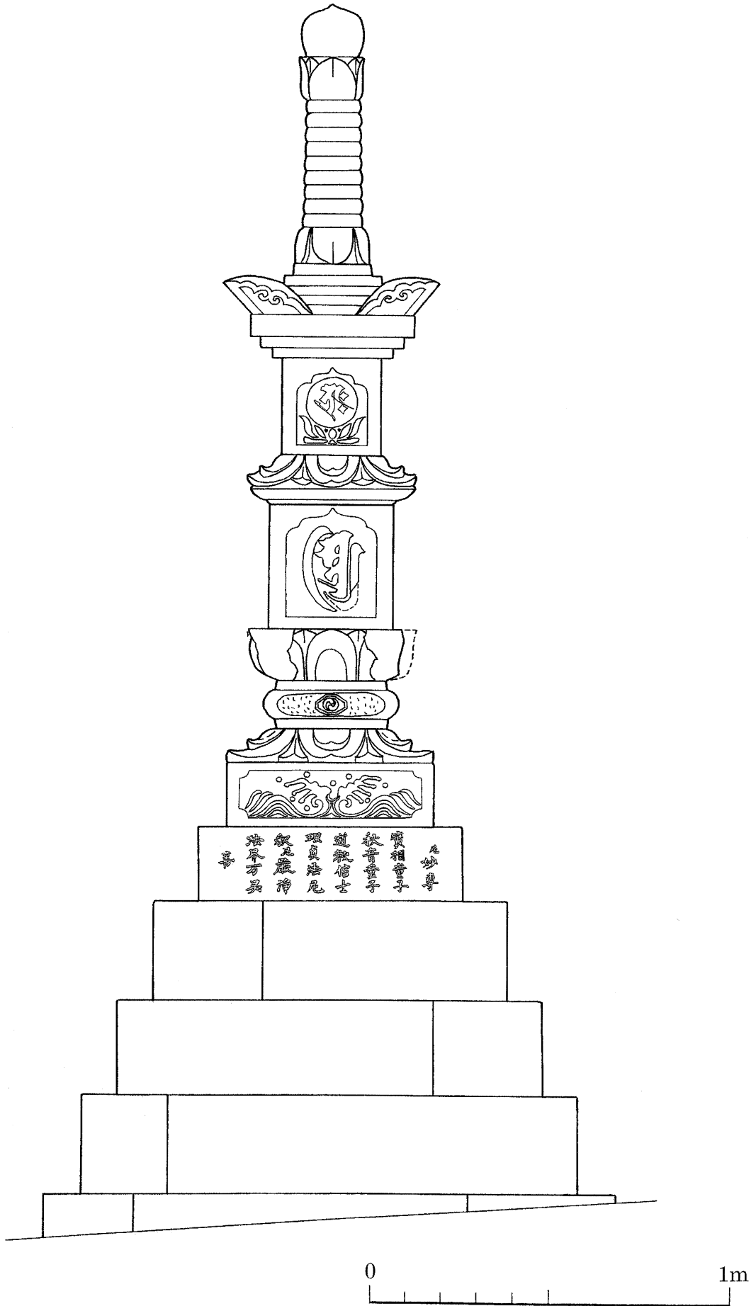
图8 富山寺宝篋印塔实测图
