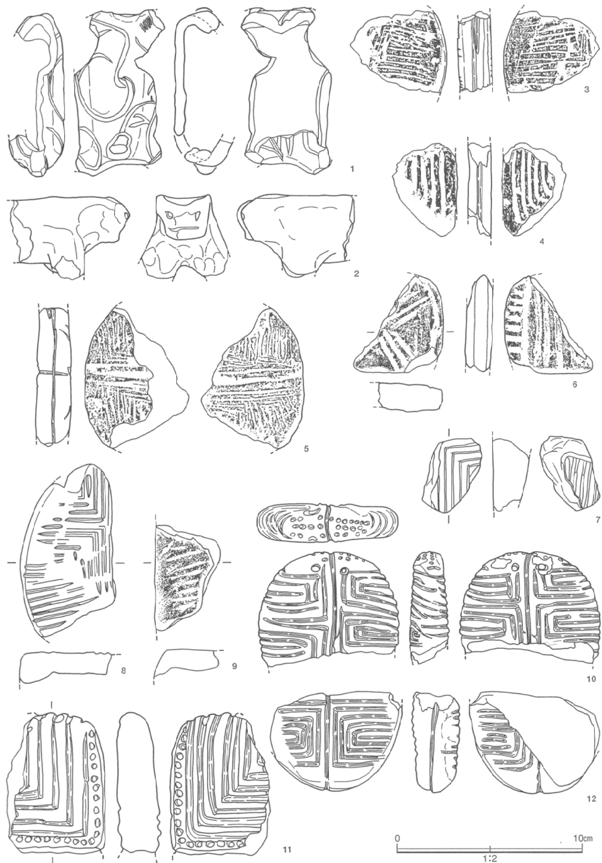
第97図 土製品 (1)
