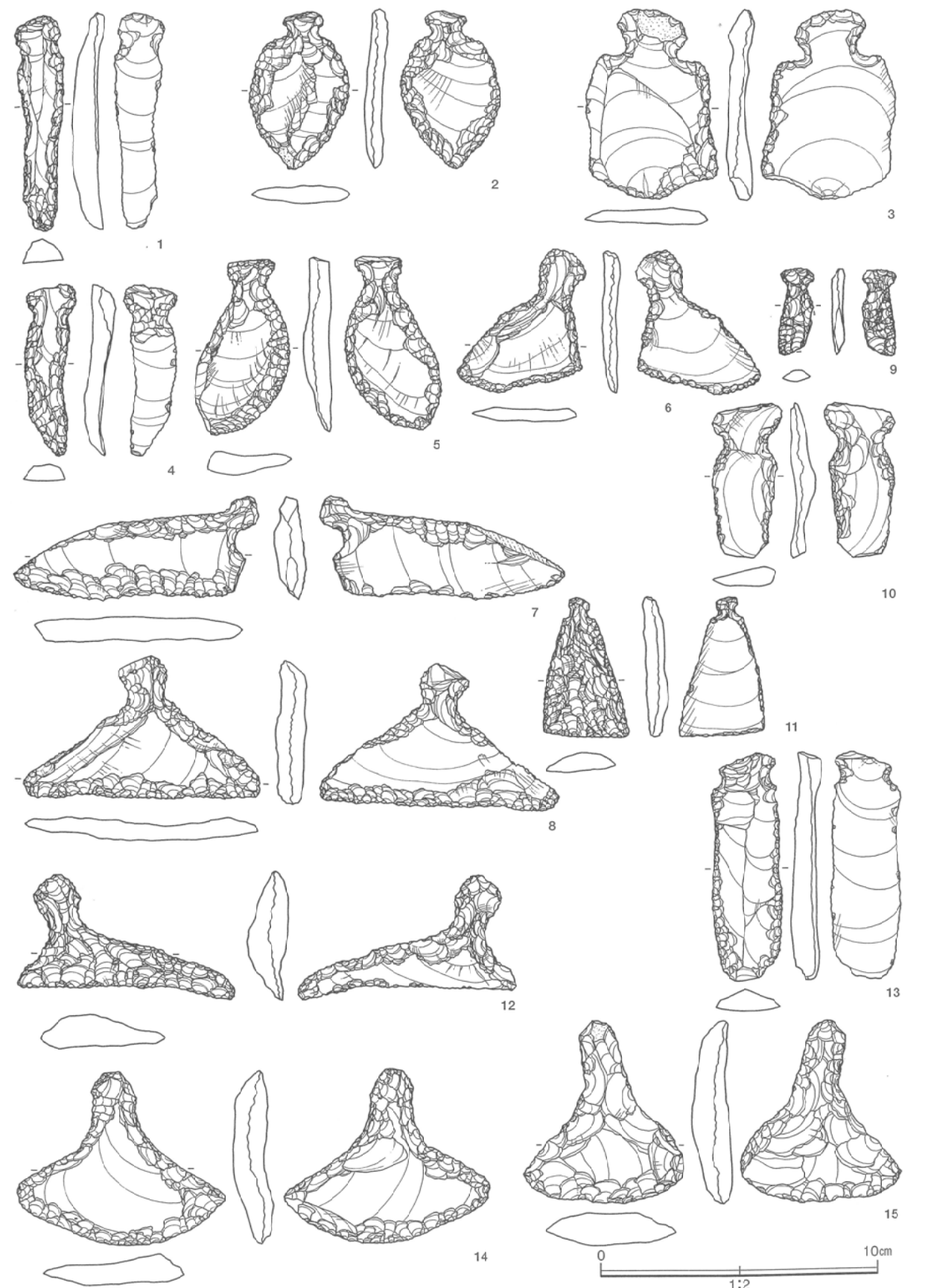
第104図 石器 (3)
