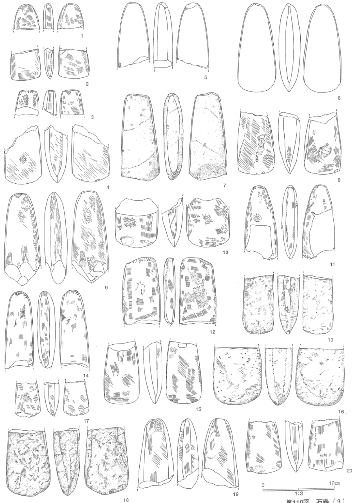
第110図 石器 (9)
