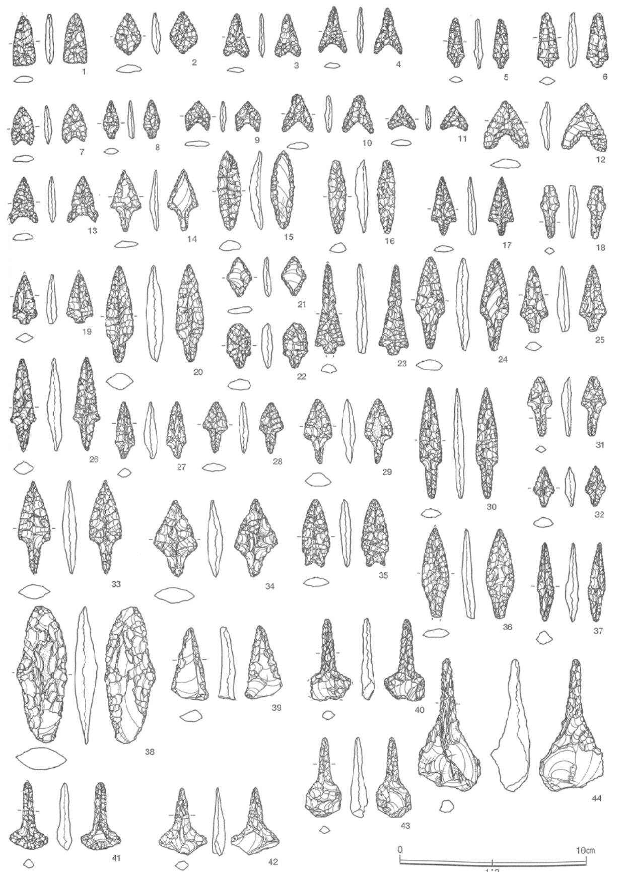
第102図 石器 (1)
