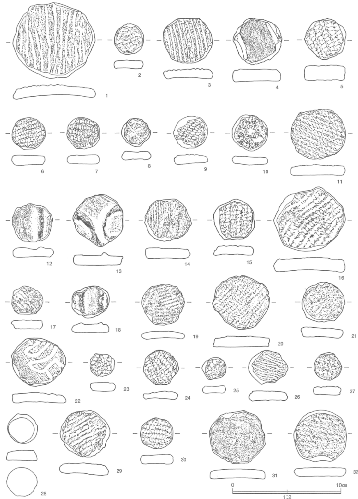
第99図 土製品 (3)
