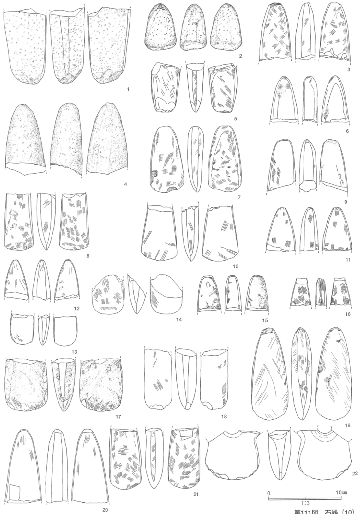
第111図 石器 (10)
