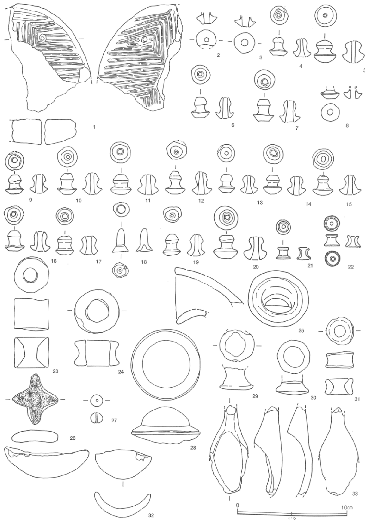
第98図 土製品 (2)
