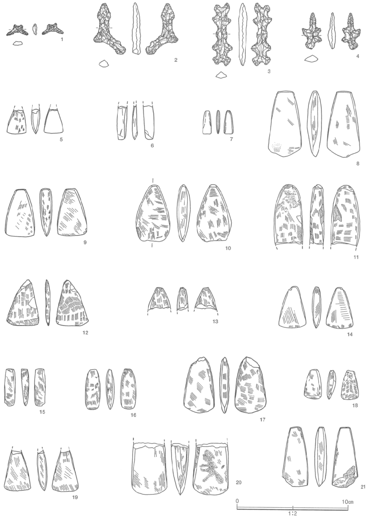
第109図 石器 (8)
