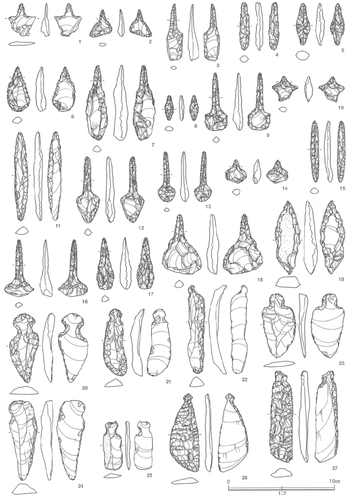
第103図 石器 (2)
