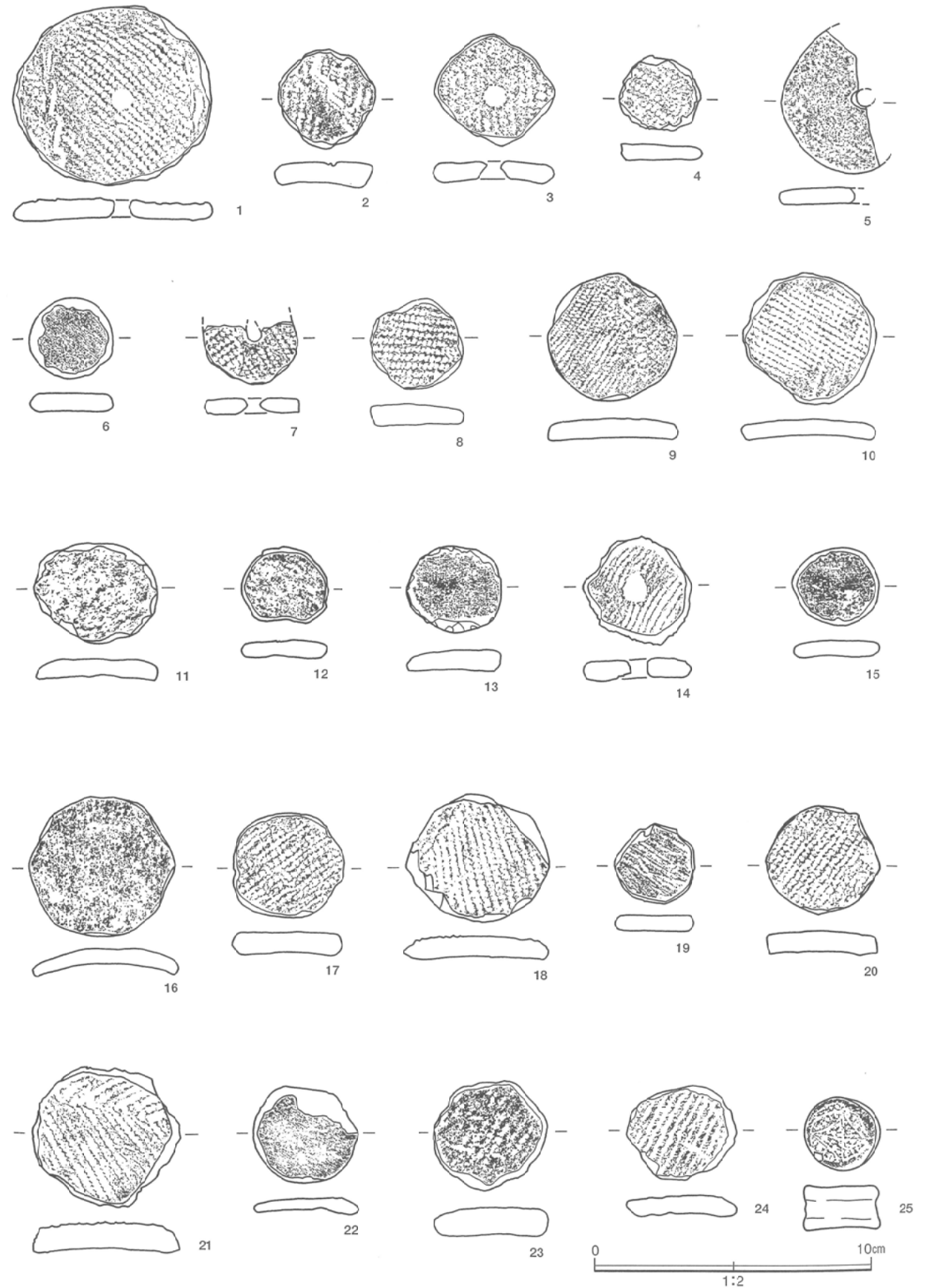
第100図 土製品 (4)
