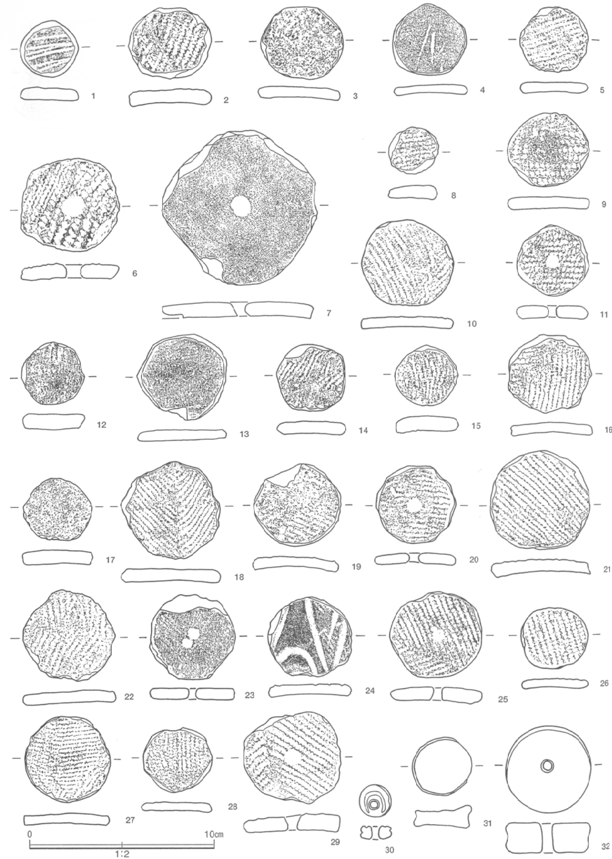
第101図 土製品 (5)
