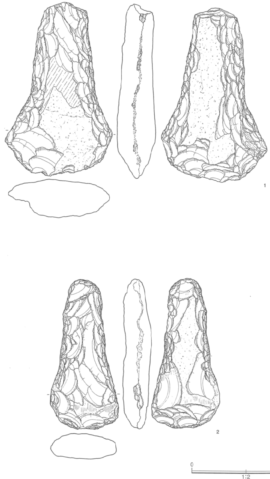
第108図 石器 (7)
