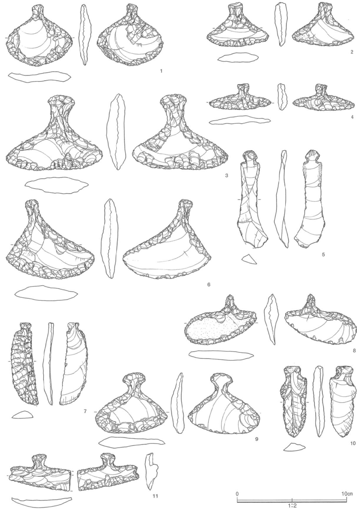
第105図 石器 (4)
