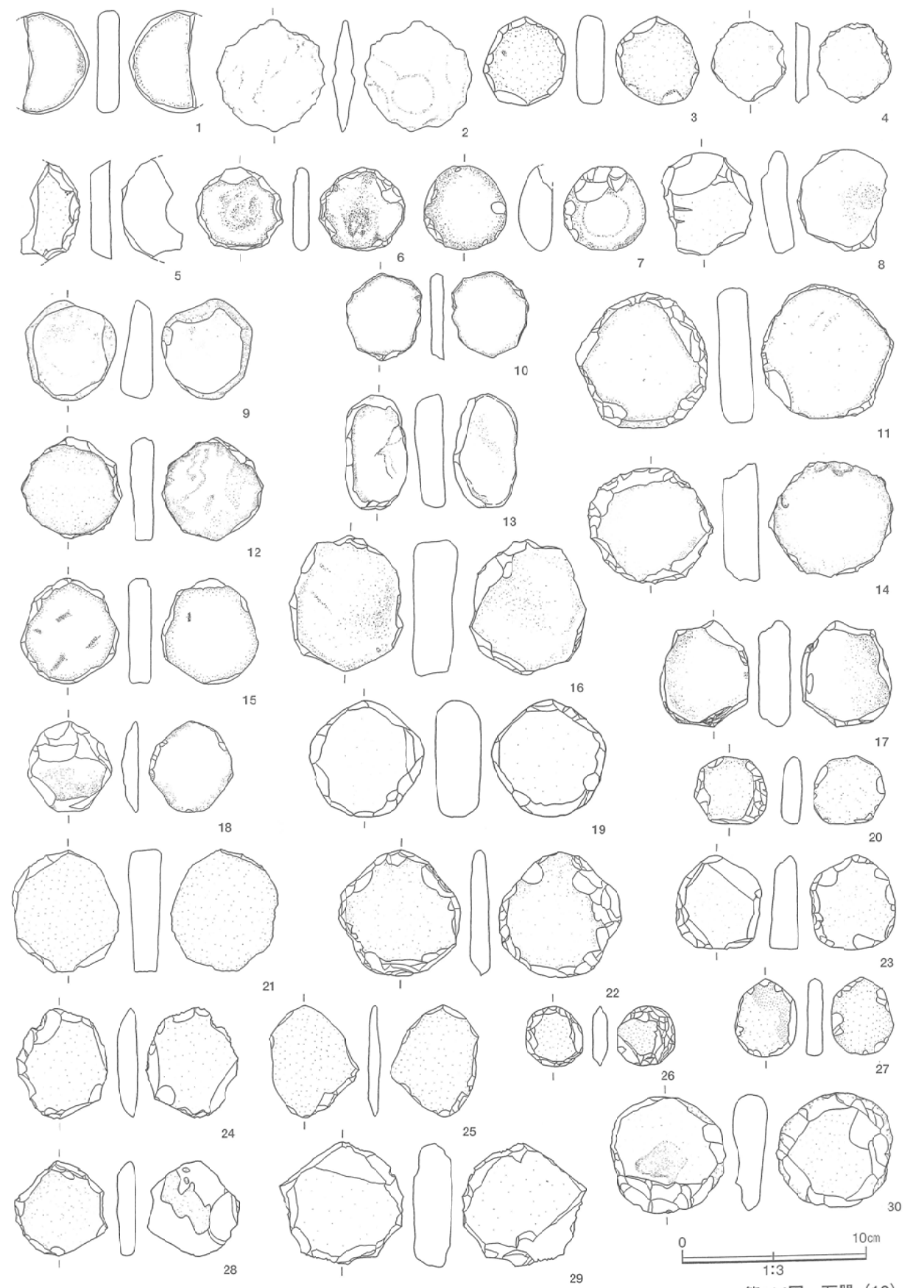
第114図 石器 (13)
