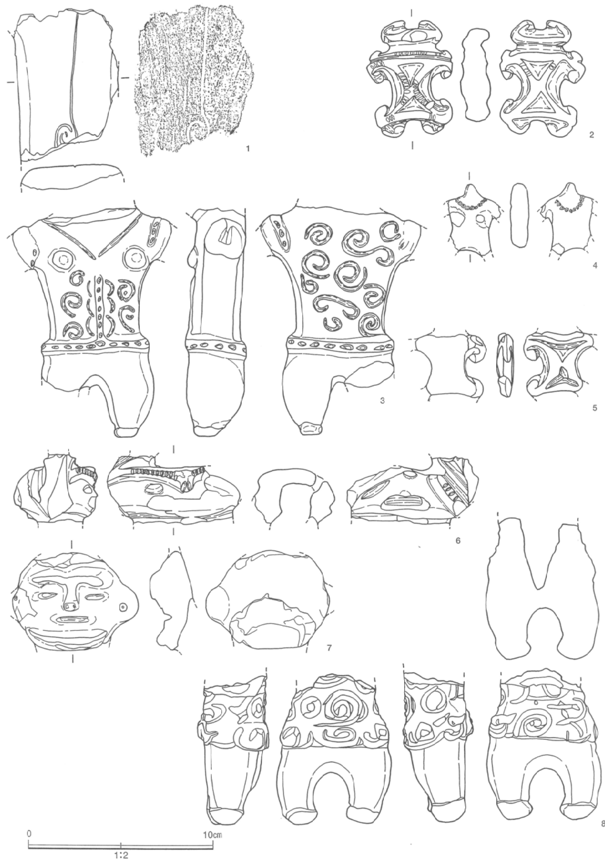
第95図 土偶(1)
