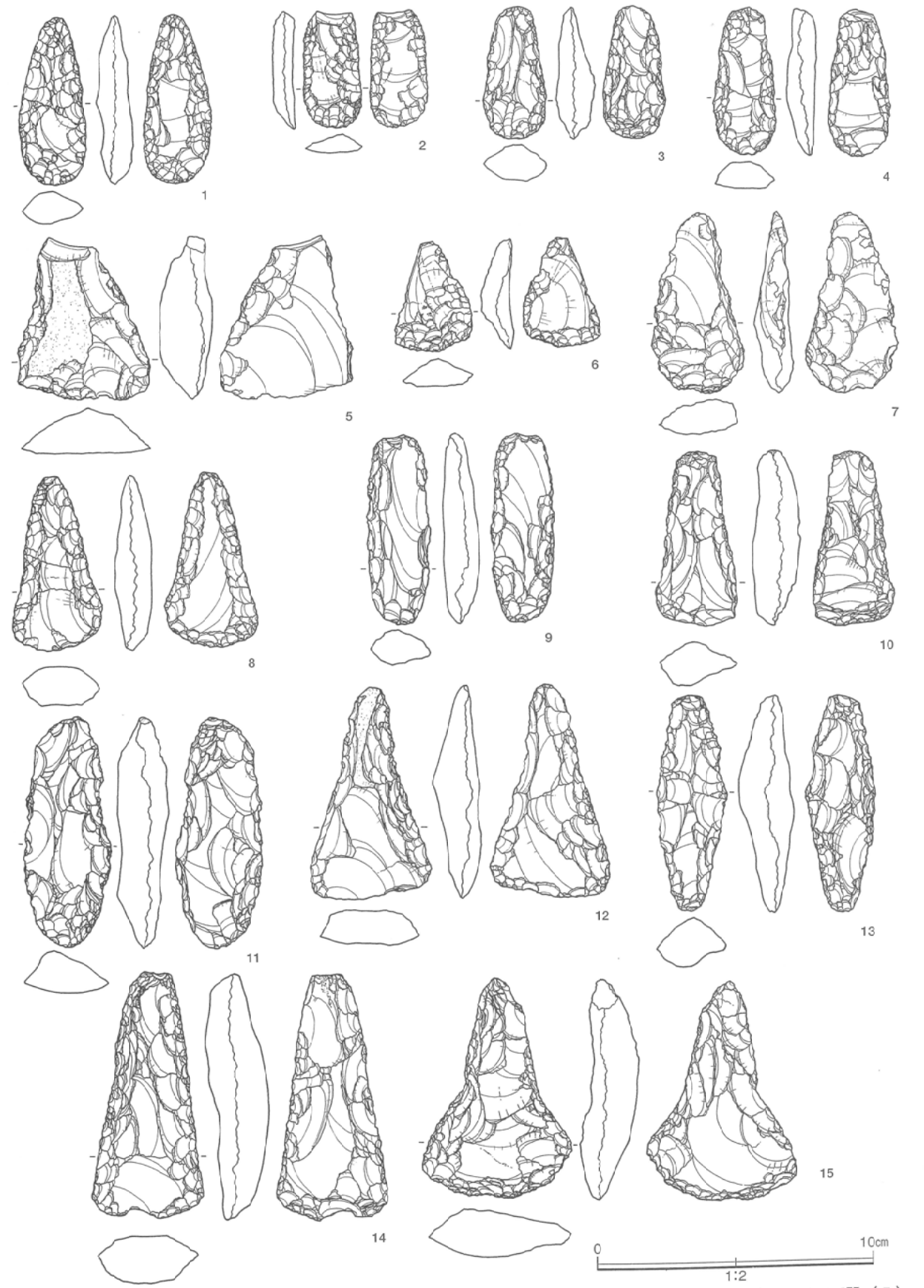
第106図 石器 (5)
