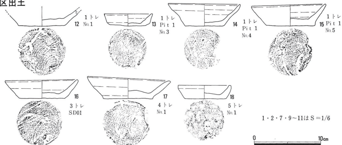
図41 B・C区出土遺物実測図
