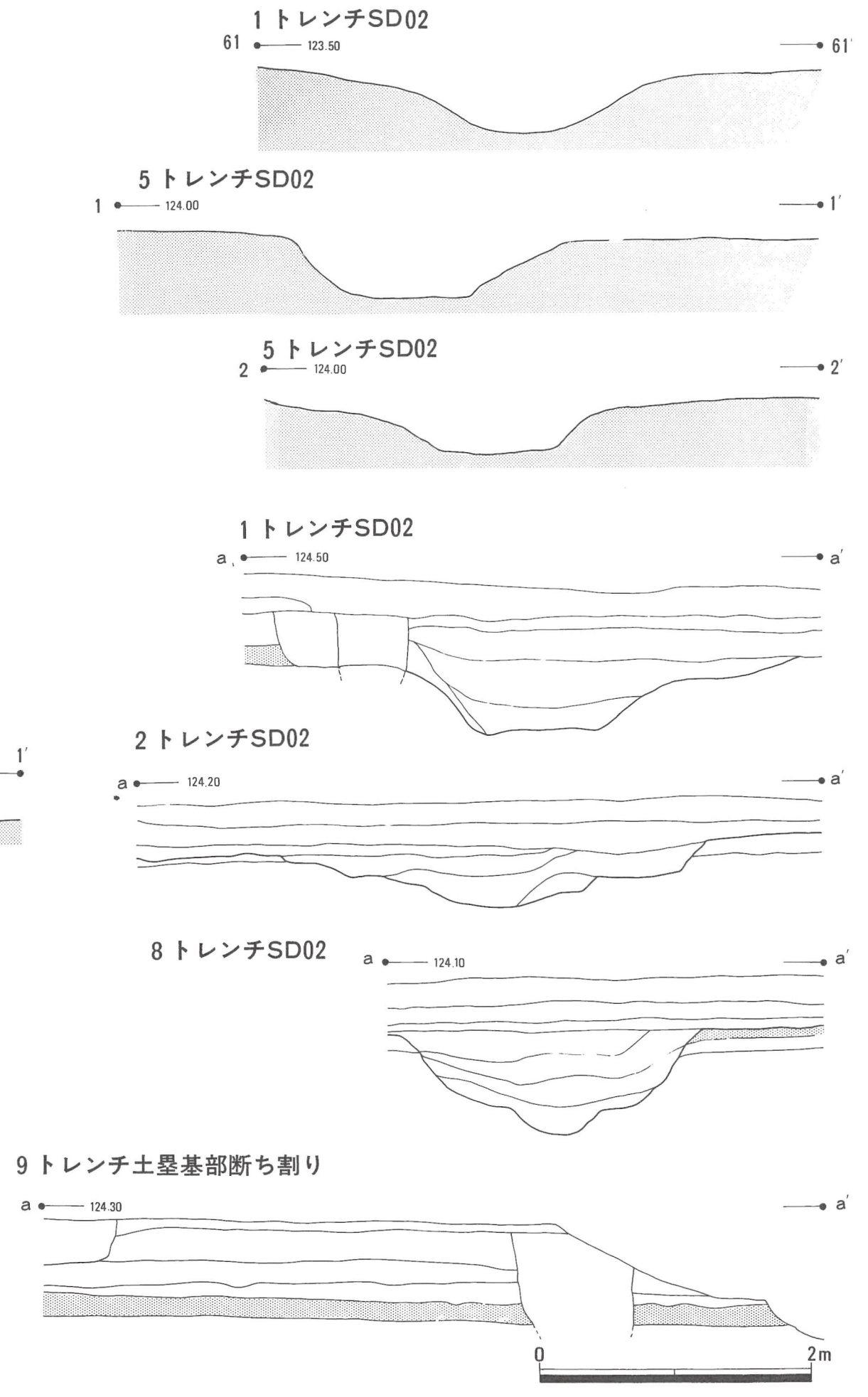
図34 B区柵列・堀エレベーション及び土層断面図
