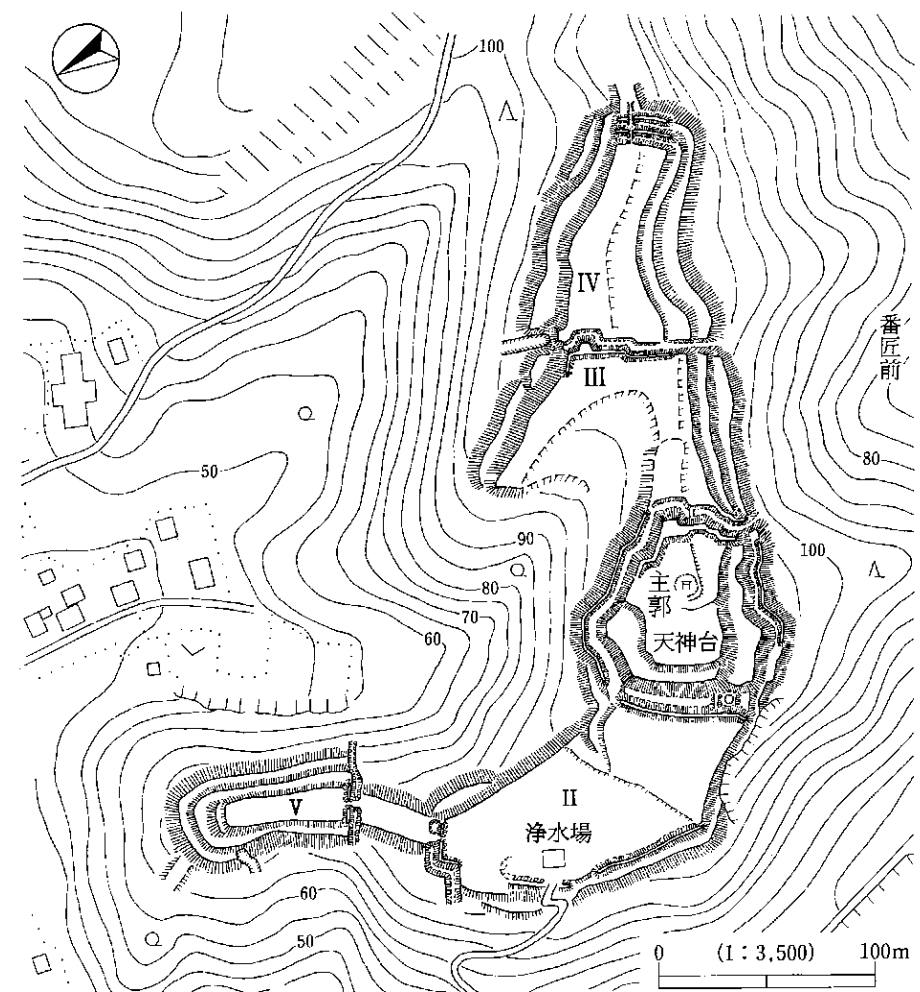
天神台城跡概念図
