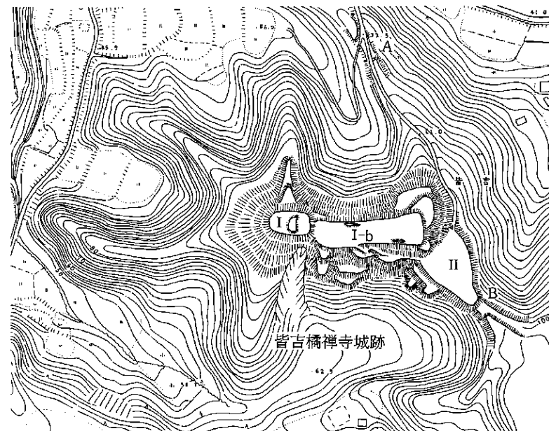
〔参考〕皆吉橋禪寺城跡縄張り図
