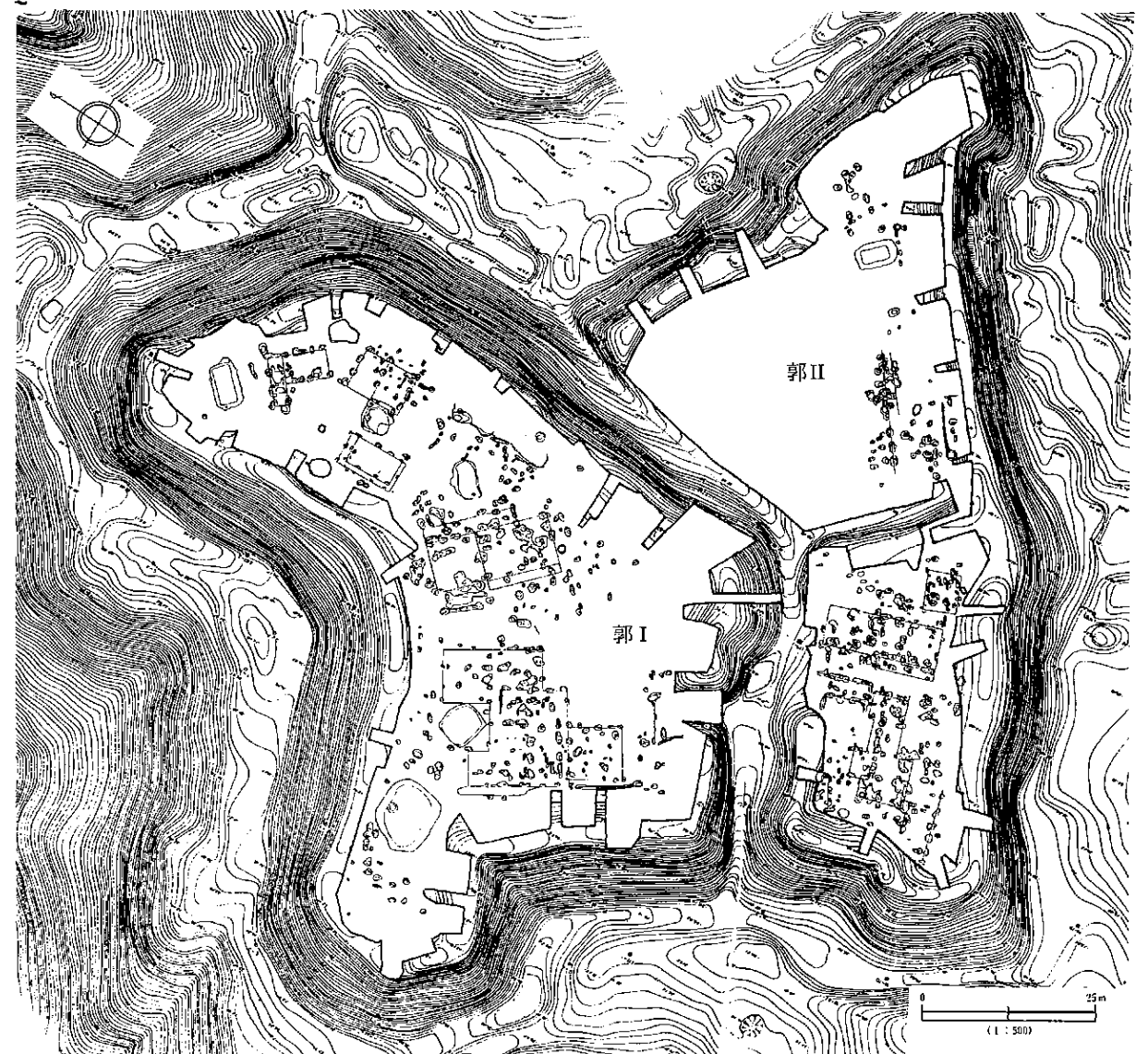
田向城主郭遺構配置図（山武郡市文化財センター『田向城』に一部加筆）
