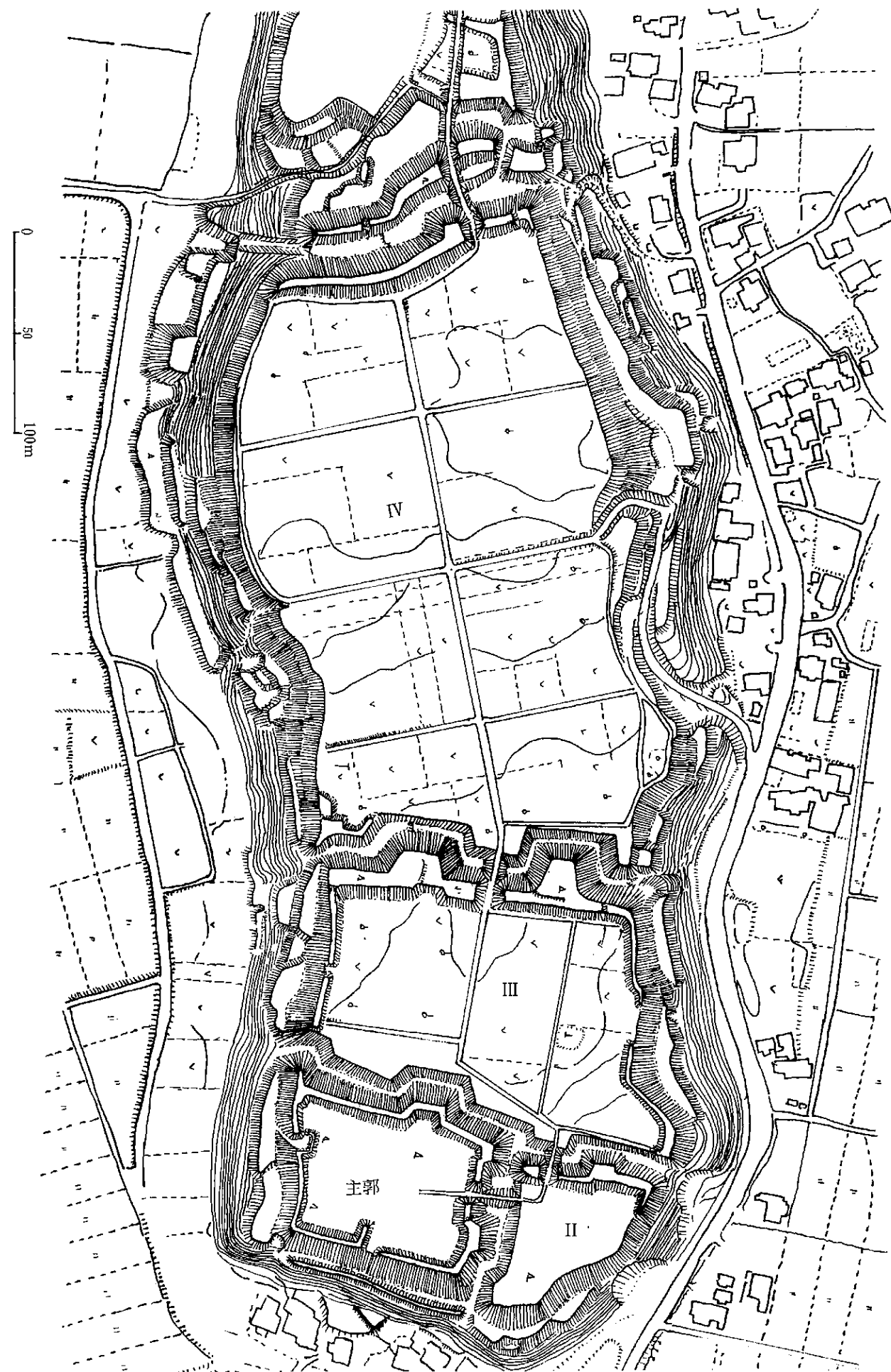
坂田城跡概念図
