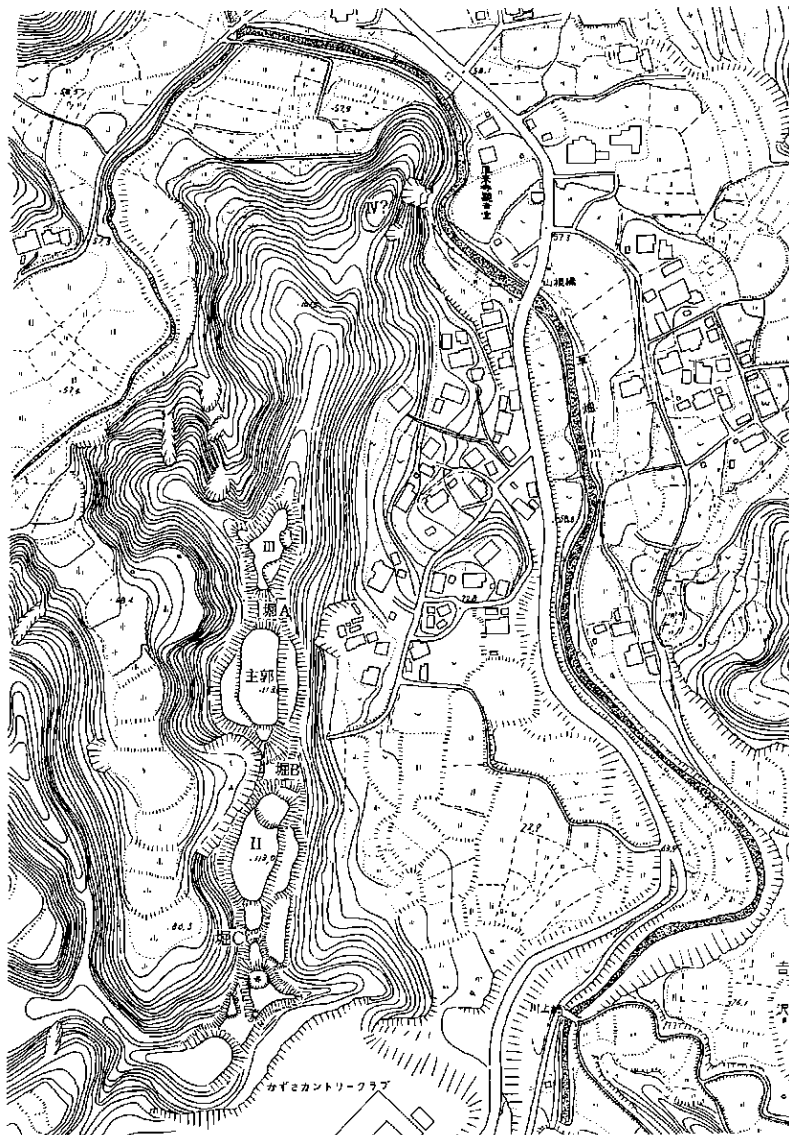
吉沢城跡遺構配置図 (S=1/5,000)
