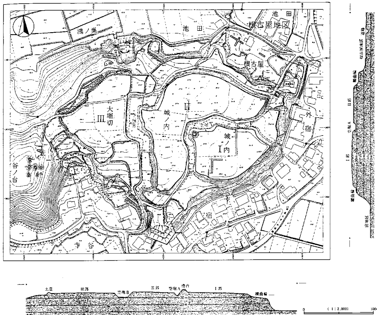
飯櫃城跡測量図（『千葉県中近世城跡研究調査報告書第7集』より）
