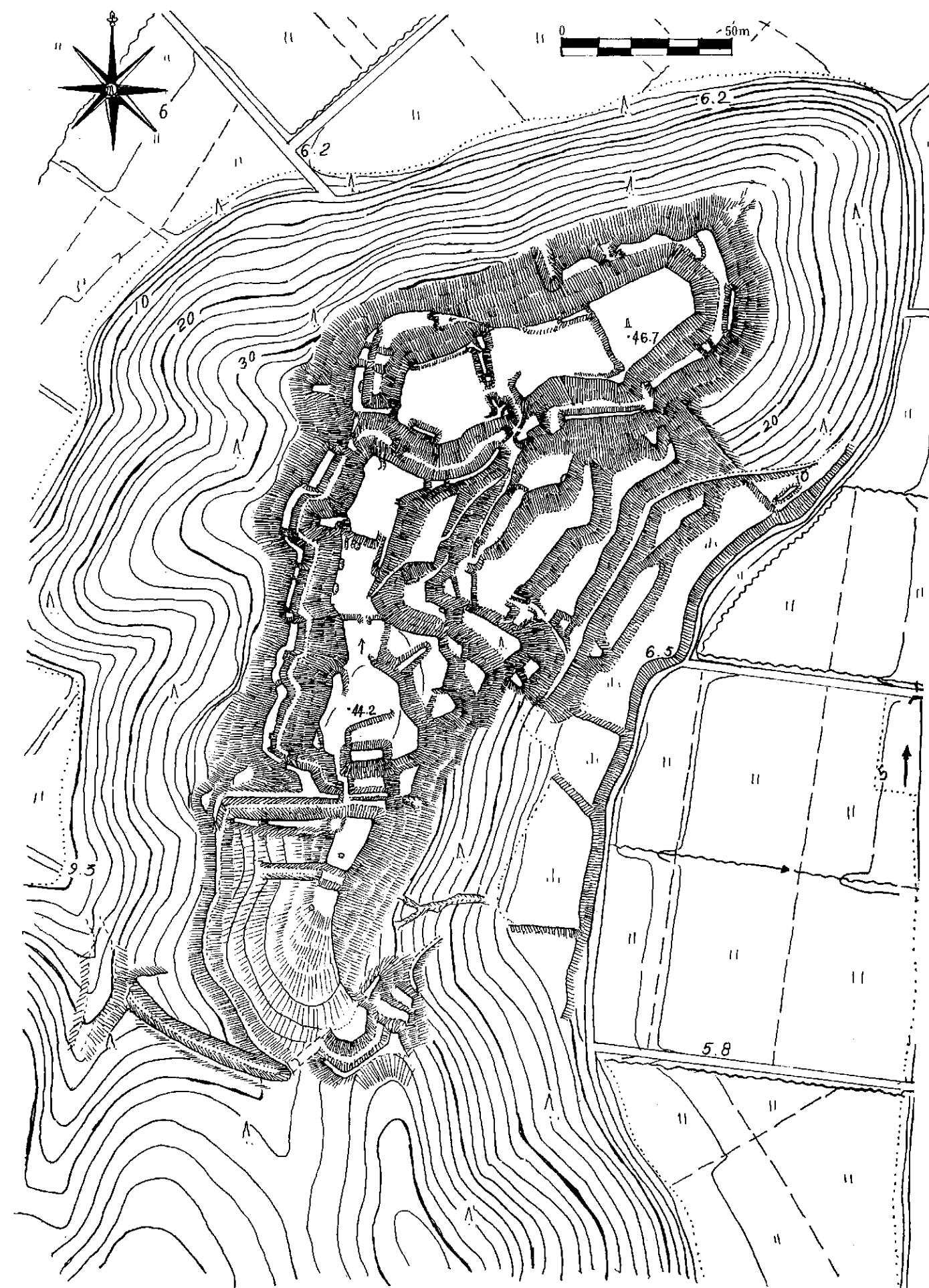
小野城跡概念図
