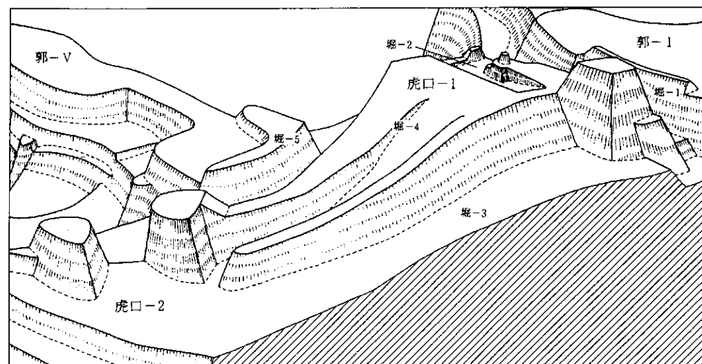
鶴ヶ城跡虎口俯瞰図（『千葉県中近世城跡研究調査報告書第13集より』）
