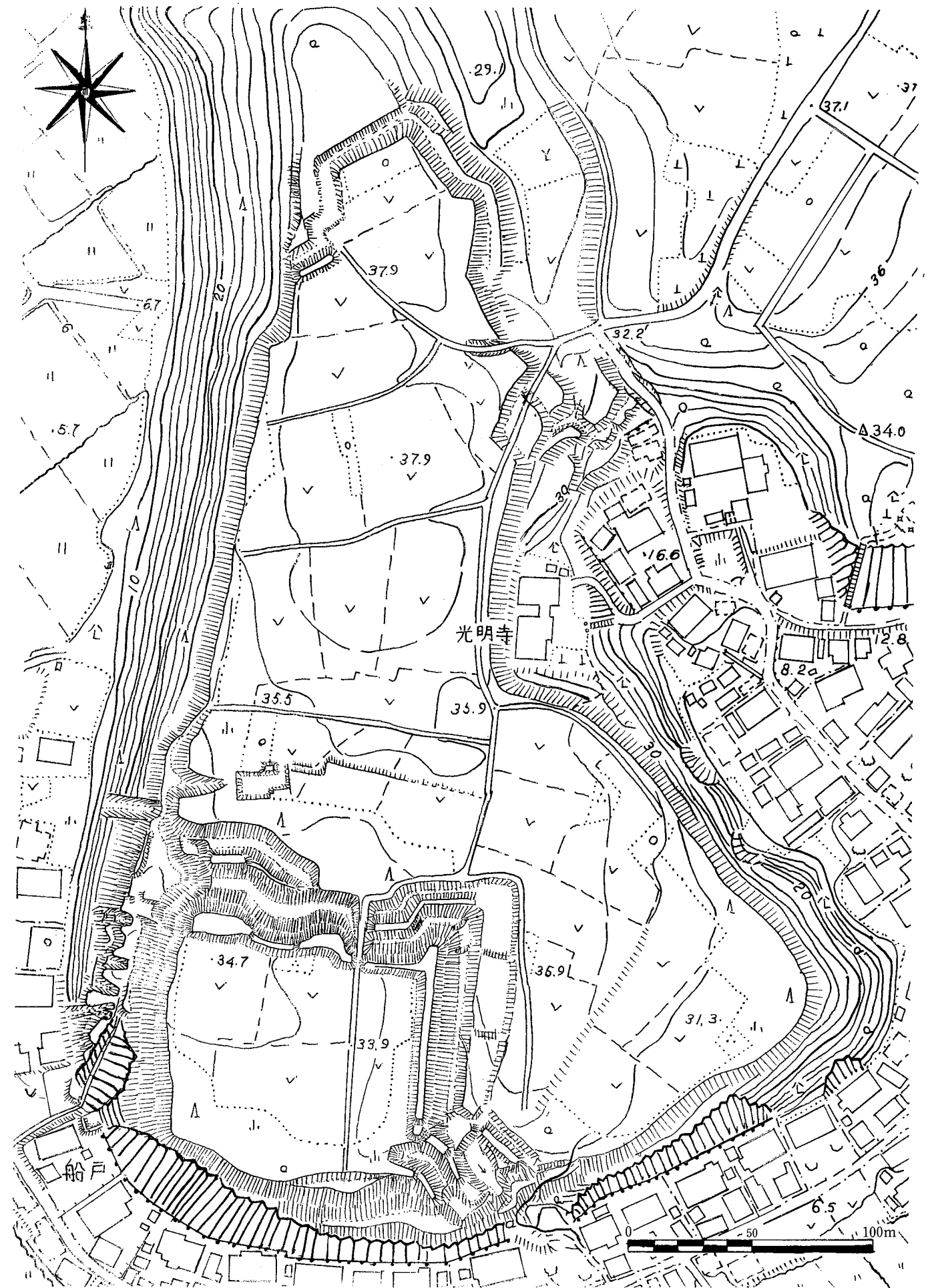
南並木城跡概念図
