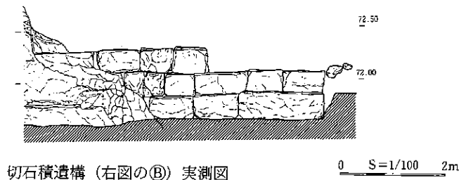
切石積遺構（右図の②）実測図
