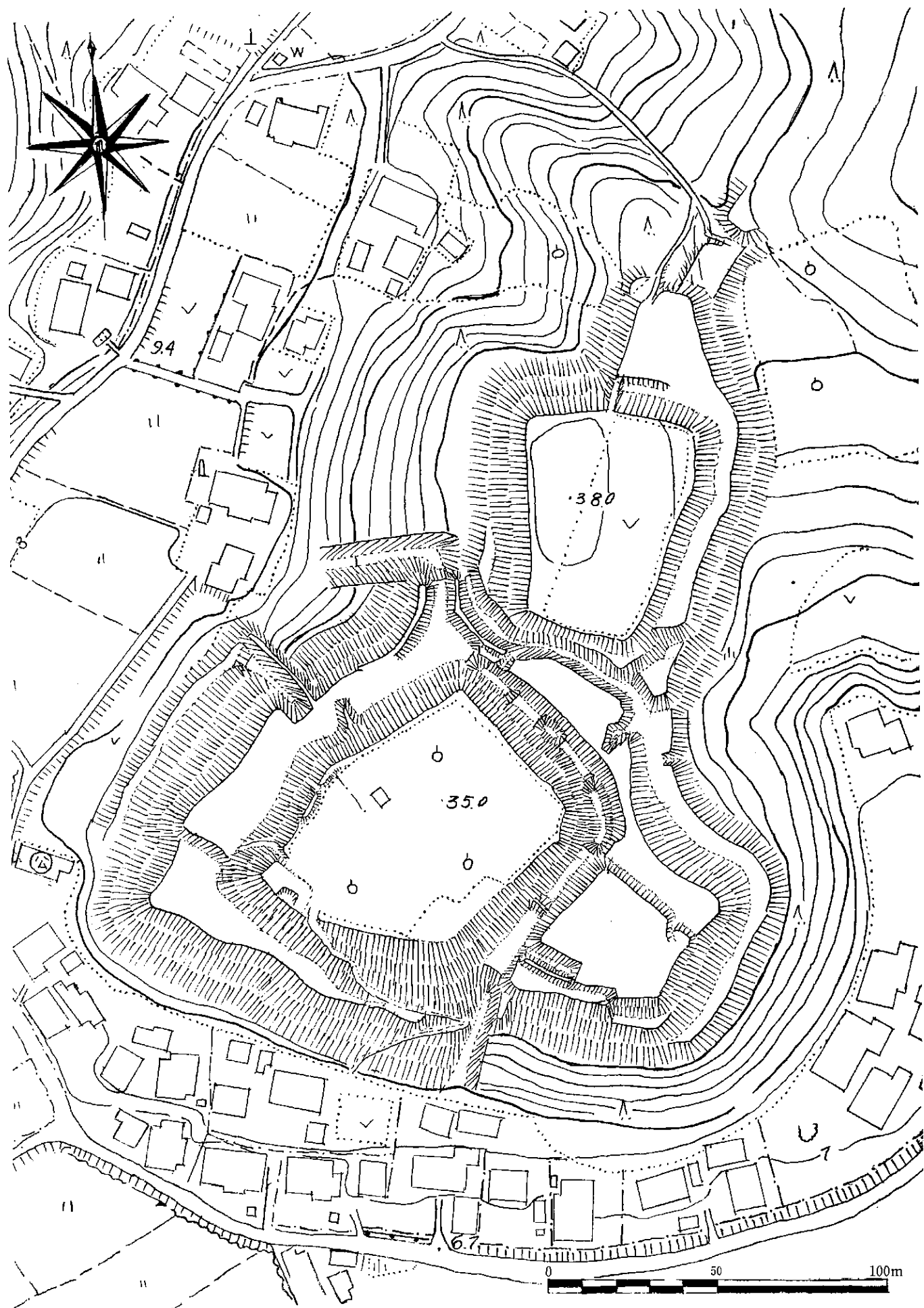
大倉城跡概念図
