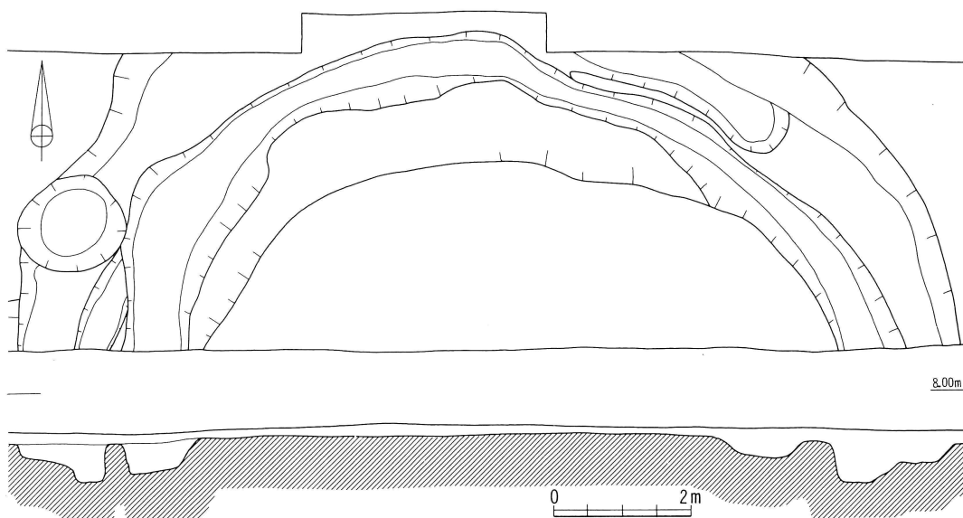
第65図 S D - 012実測図
