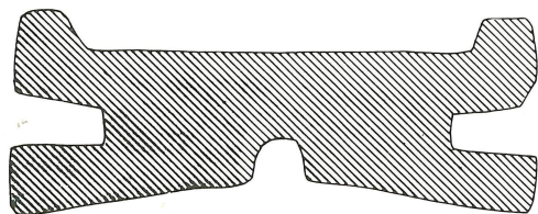
第40図 下筋生田畑田遺跡出土石臼実測図1 (1・2)
