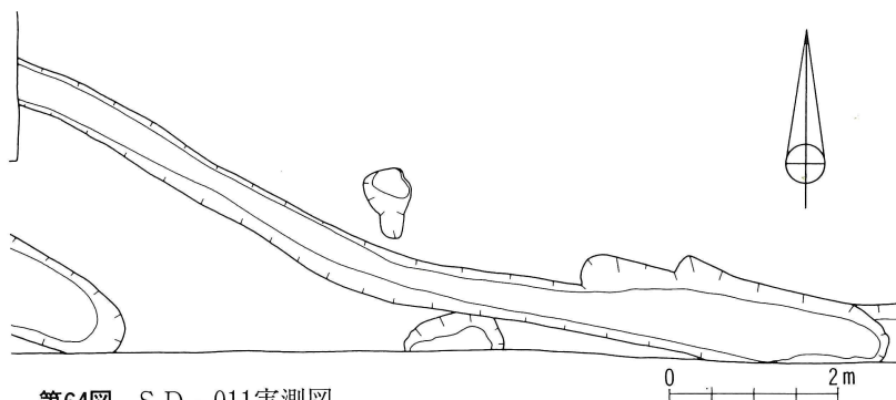
第64図 S D - 011実測図
