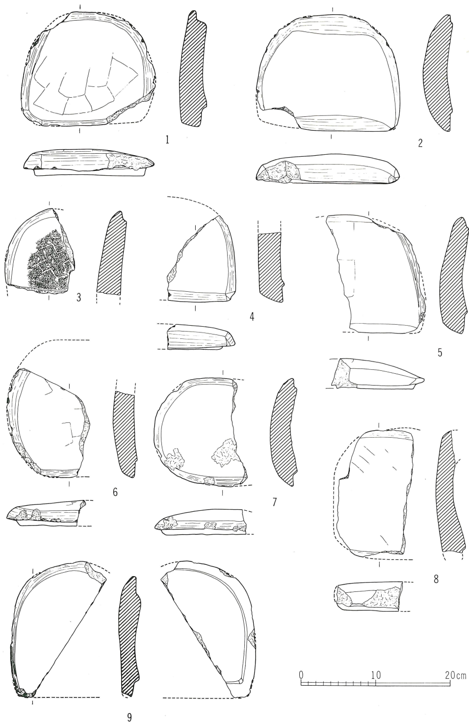
第45図 下筋生田畑田遺跡出土火炉蓋実測図(1～9)
