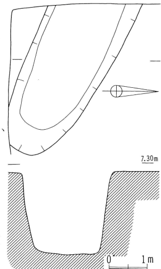
第63図 SK-010実測図
