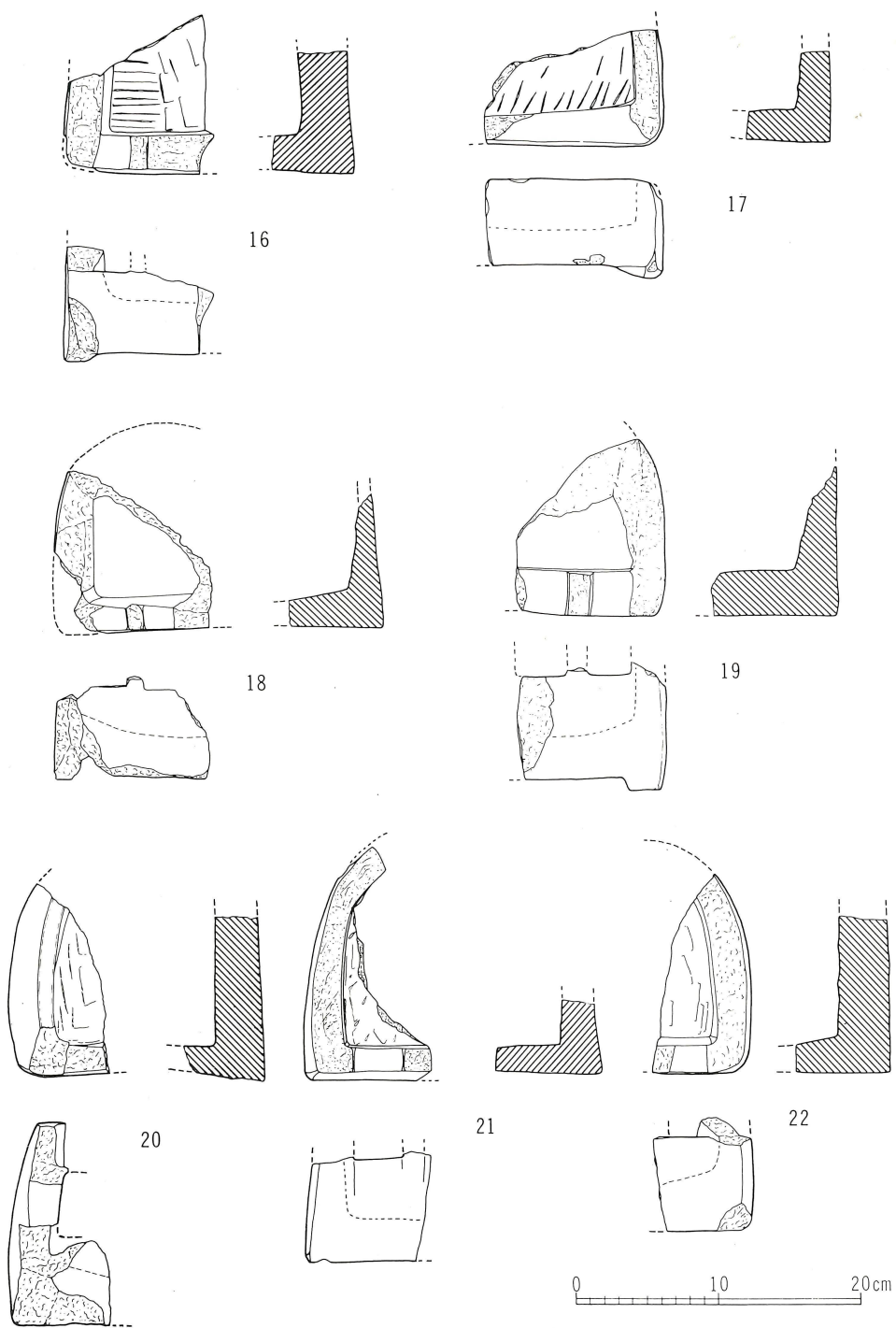
第47図 下叻生田畑田遺跡出土火炉身実測図 2 (16~22)
