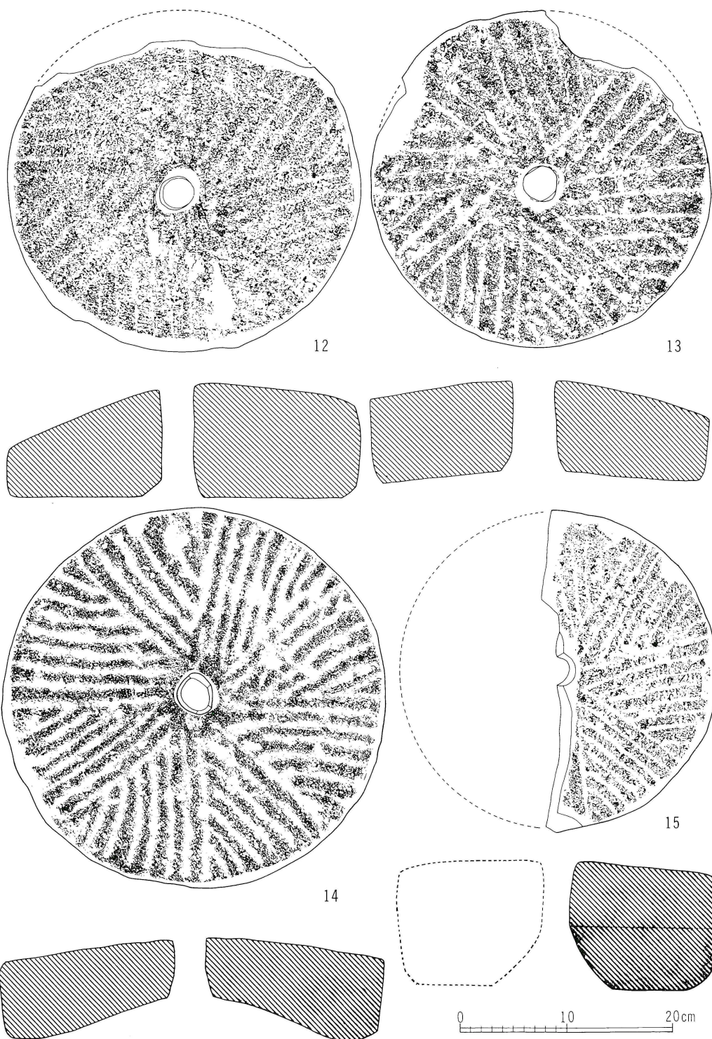
第44図 下筋生田畑田遺跡出土石臼実測図 5 (12~15)
