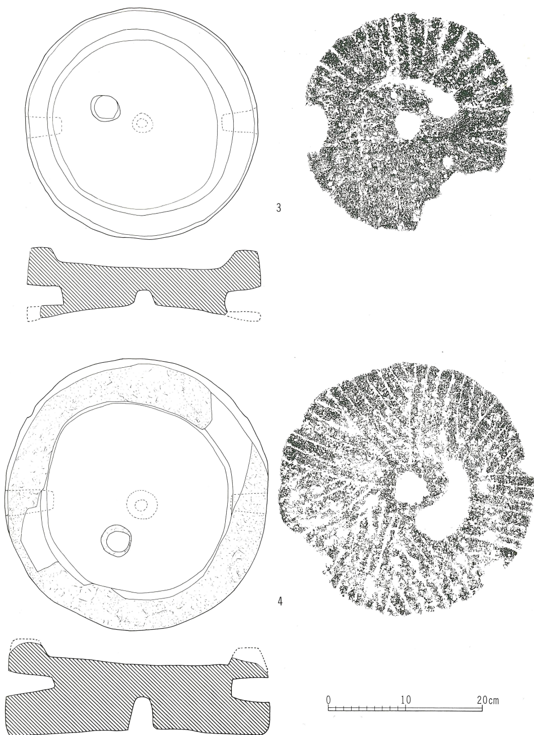
第41図 下筋生田畑田遺跡出土石臼実測図2(3・4)
