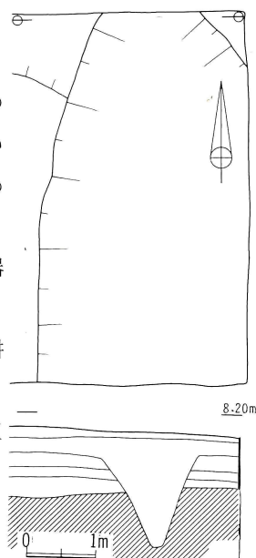
第58図 SD-004実測図
