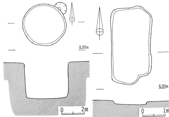
第56図 SE-002実測図
