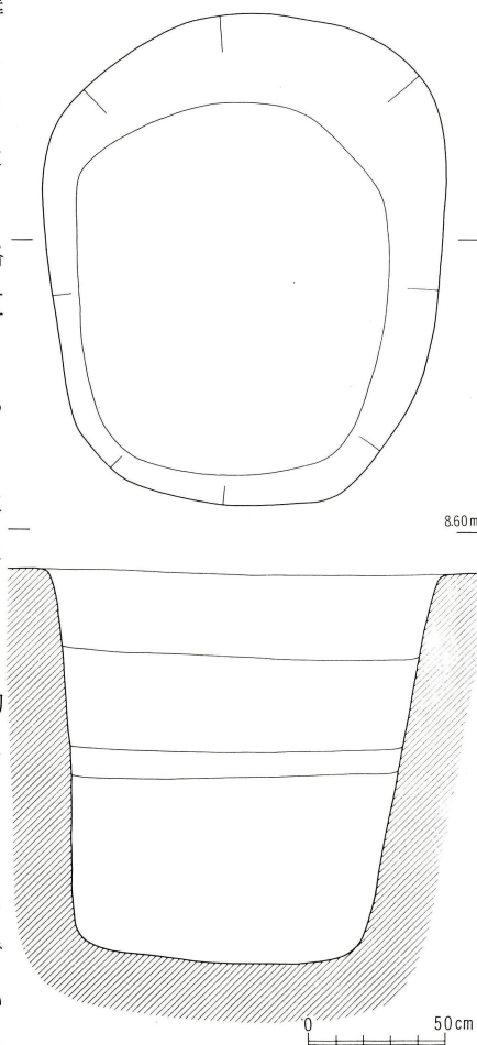
第32図 3号土壙実測図
