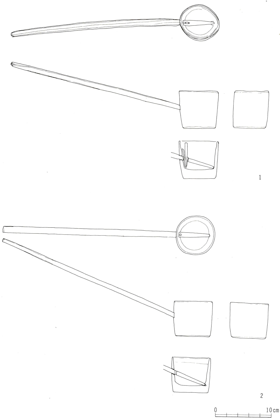
第51図 下筋生田畑田遺跡出土木製柄杓実測図（1・2）
