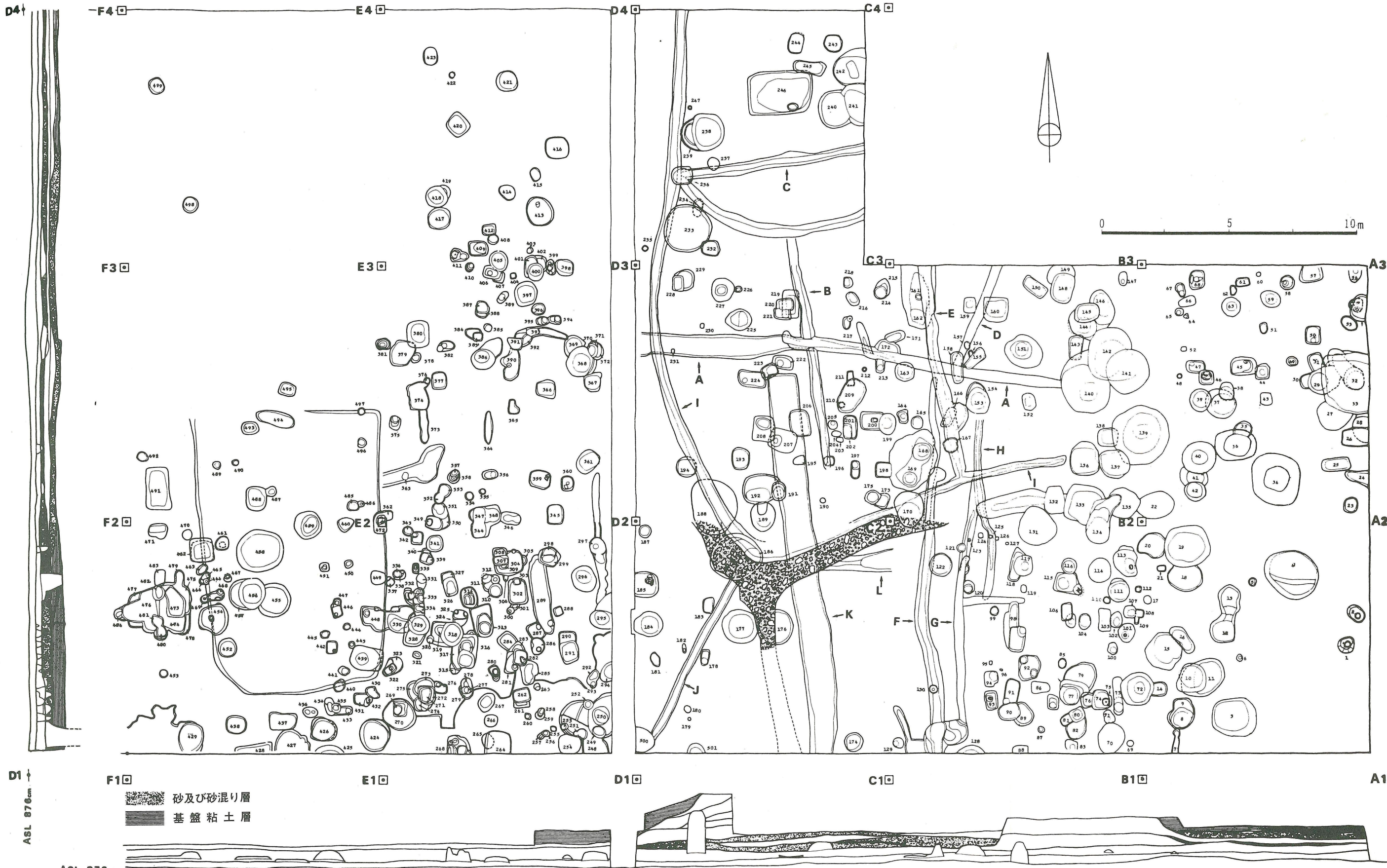
第33図 下筋生田畑田遺跡遺構全体図
