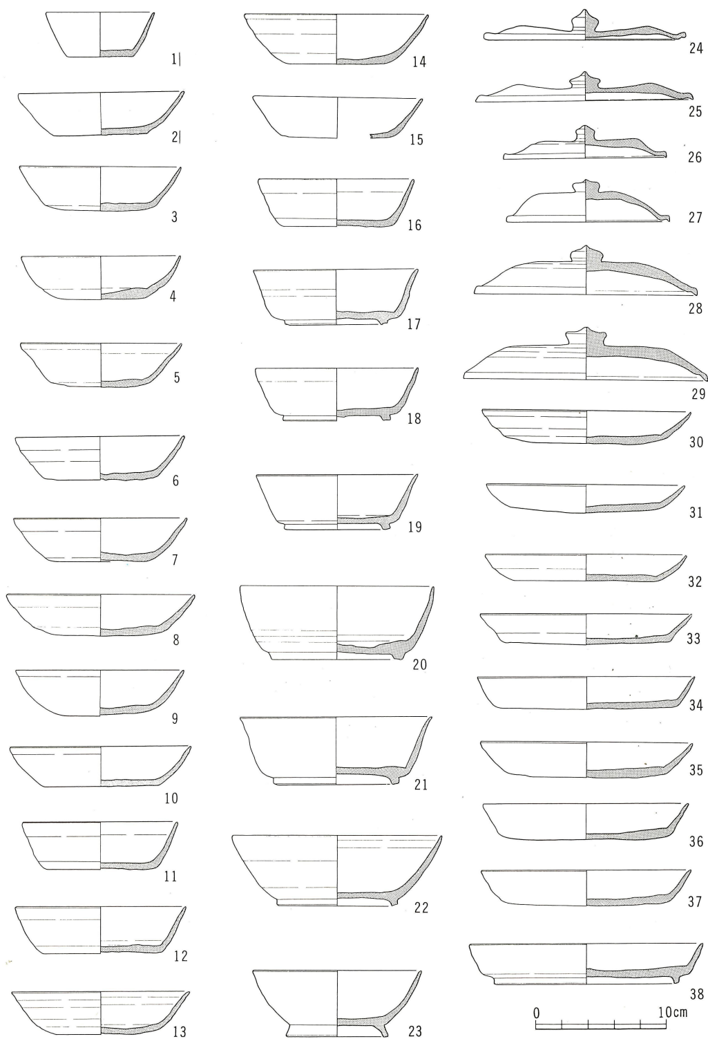
第36図 下筋生田畑田遺跡出土須恵器実測図（1～38）
