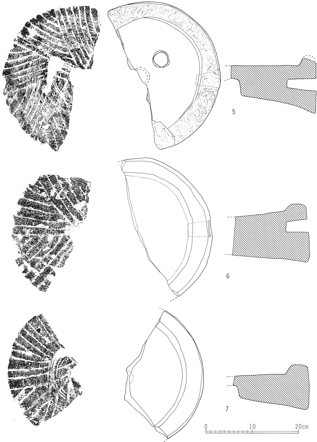
第42図 下筋生田畑田遺跡出土石臼実測図3 (5~7)
