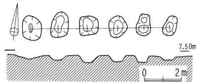
第62図 SA-009実測図
