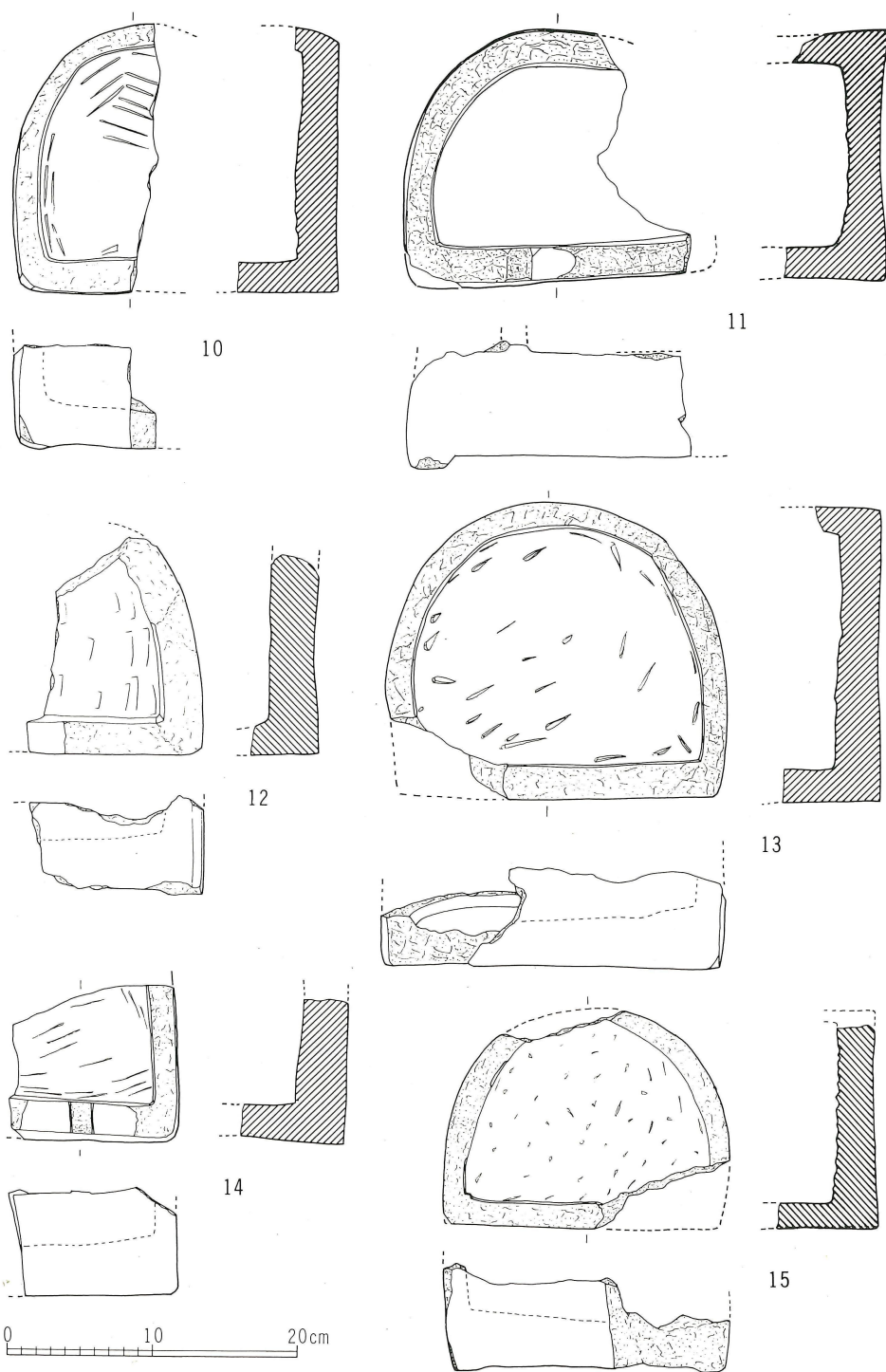
第46図 下筋生田畑田遺跡出土火炉身実測図1 (10~15)
