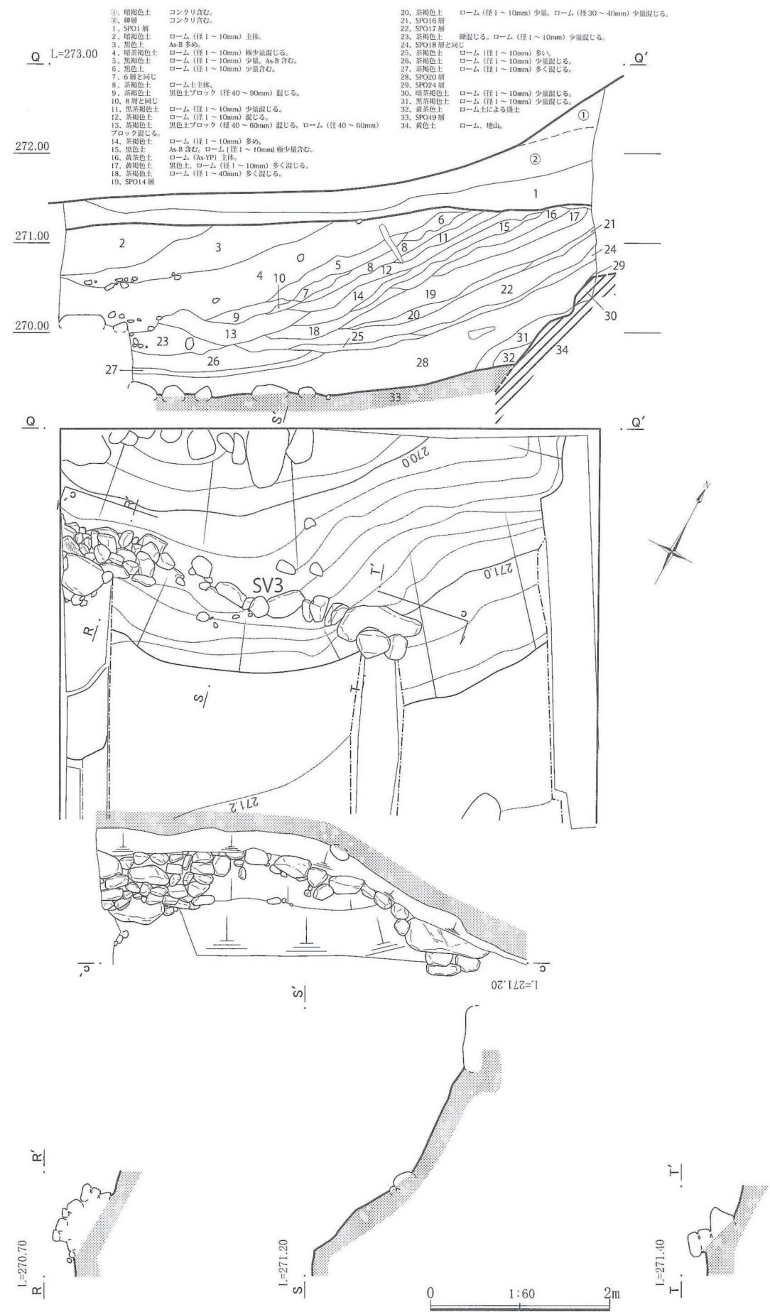
第 253 図 御前曲輪・通仲曲輪間地区 SV3 付近（平面図・セクション図・立面図・エレベーション図）
