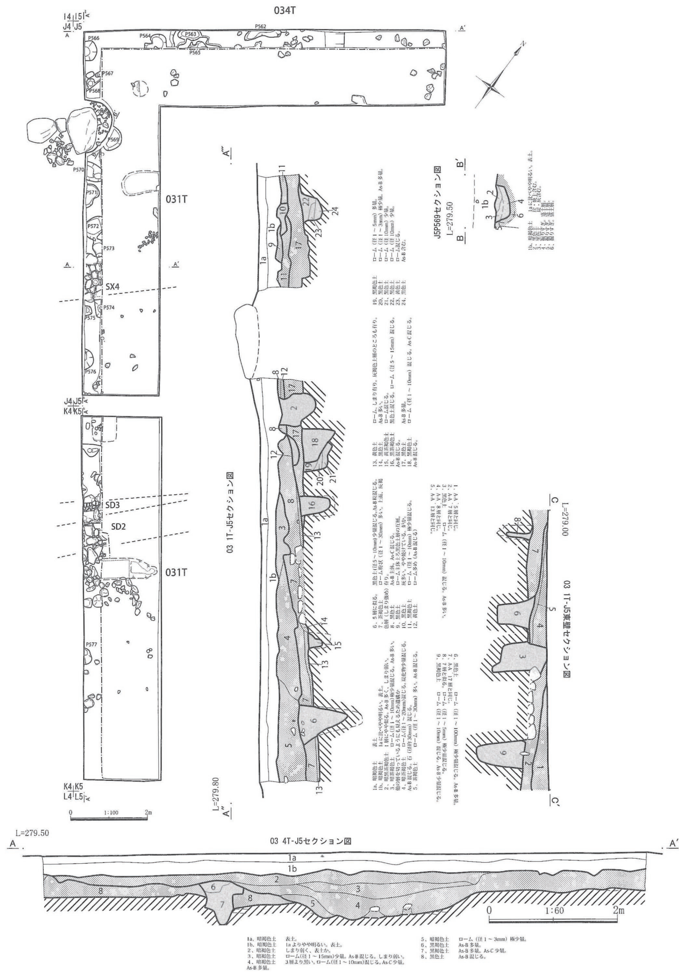
第190図 本丸地区 J5・K5 グリット 031T・034T (平面図・セクション図①)
