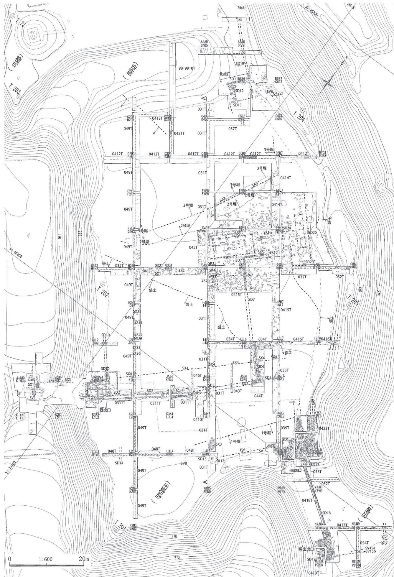
第 144 図 本丸地区全体図
