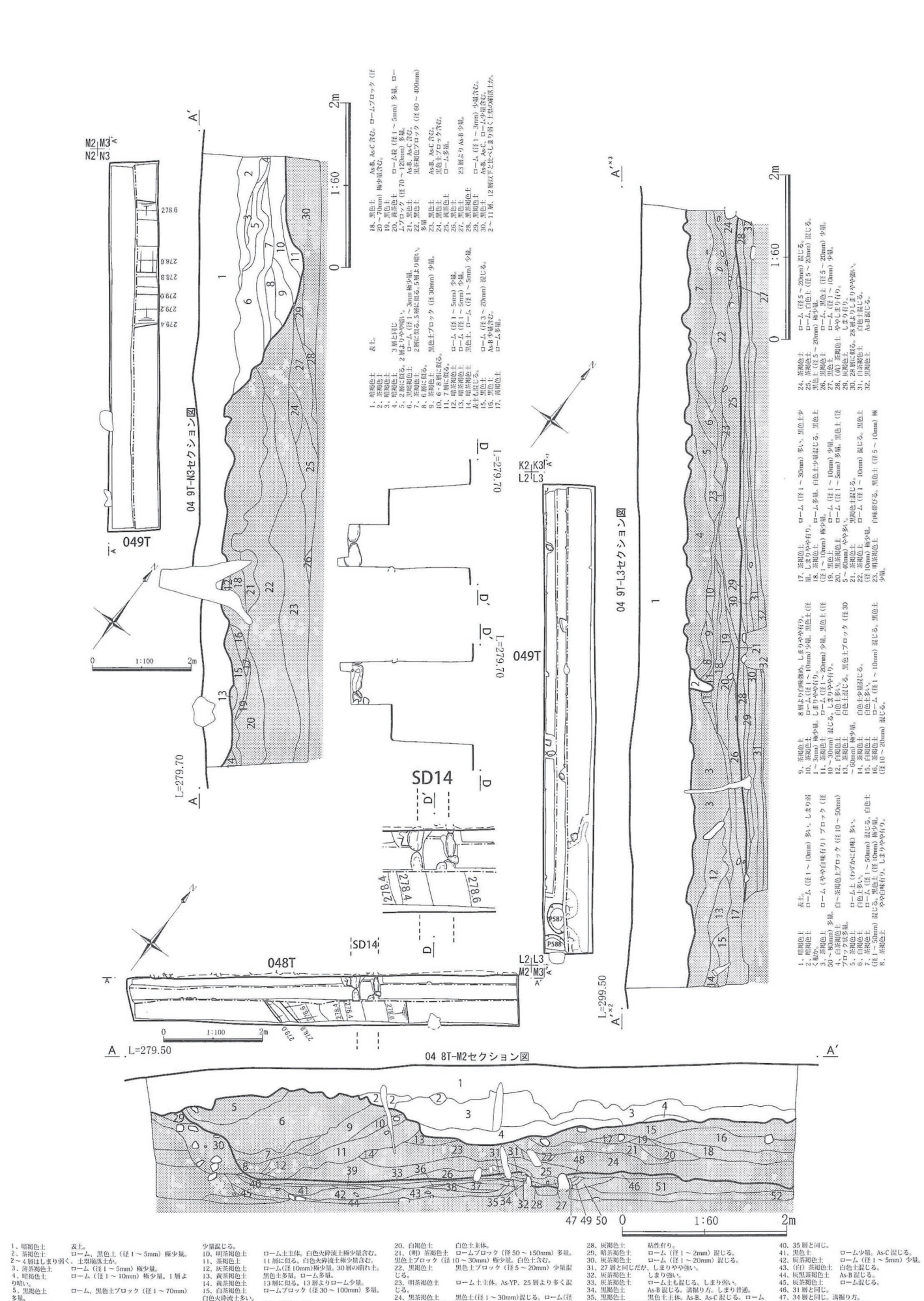
第195図 本丸地区 L3・M2・N3 グリット 048T・049T (平面図・セクション図)、SD14 (平面図・立面図)
