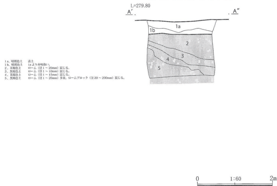
03 7T-D6セクション図
