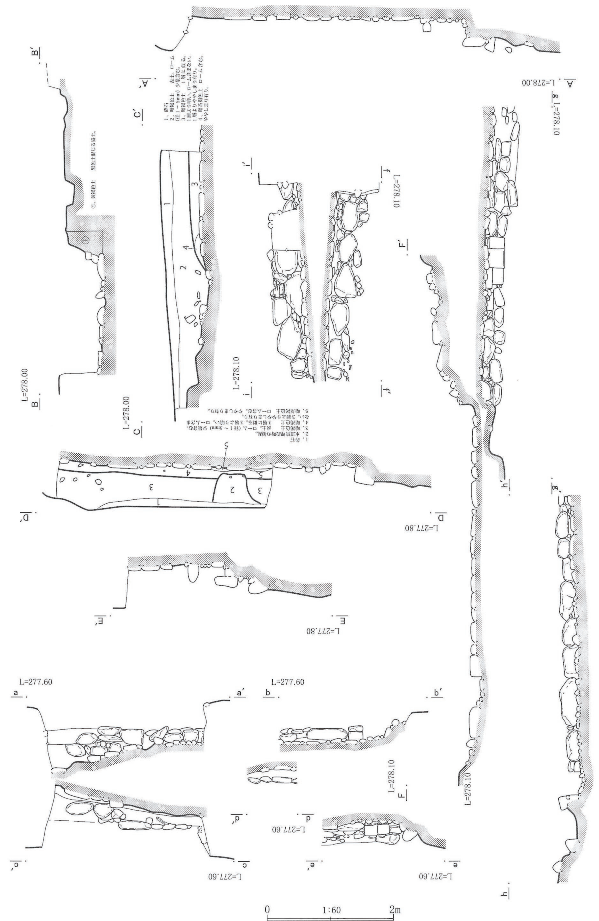
第 187 図 本丸地区 07・08・P8 グリット馬出虎口 (セクション図・立面図・エレベーション図)
