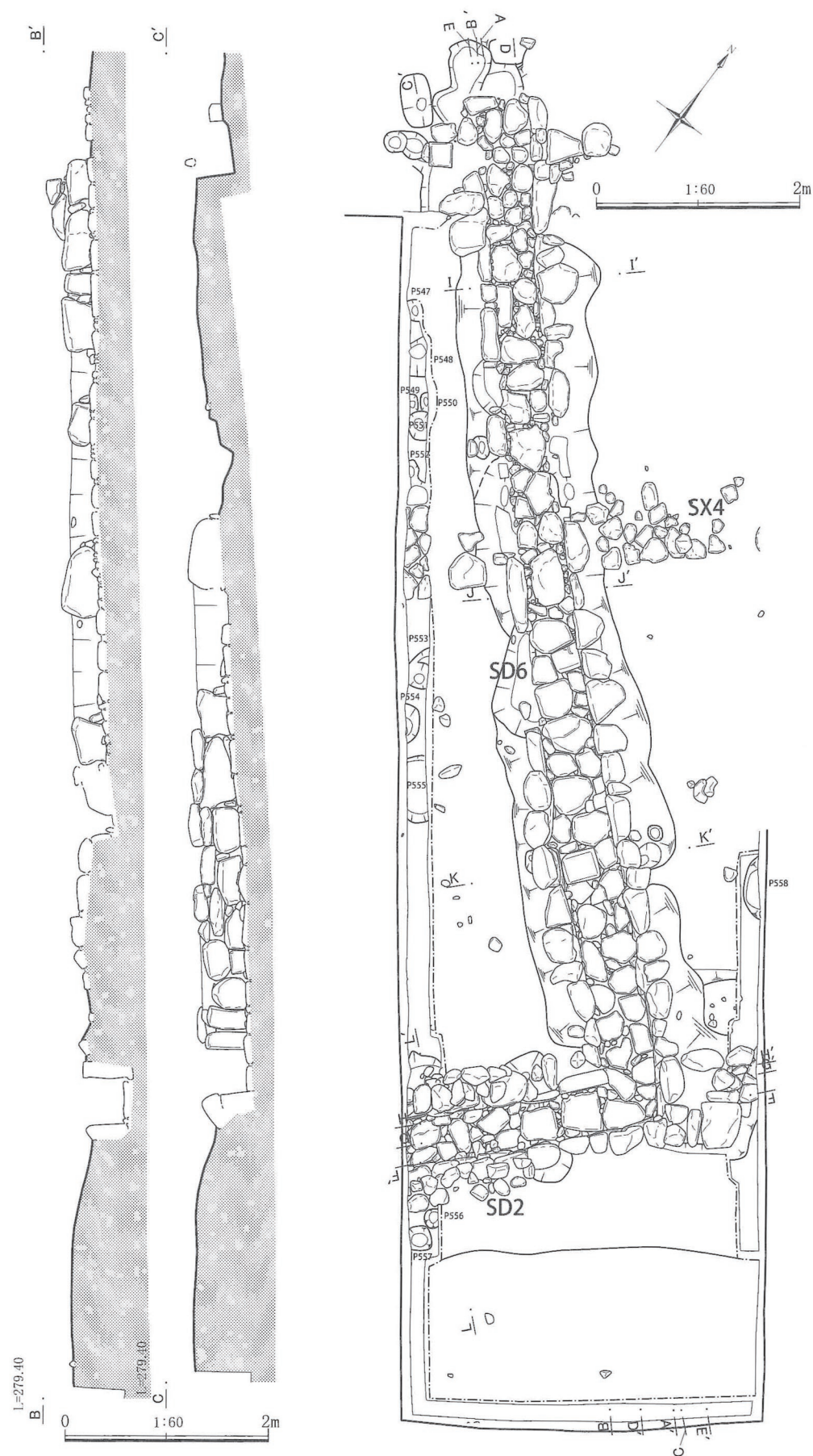
第 178 図 本丸地区 J6・K6 グリット 044TSD2・SD6 (平面図・立面図①)
