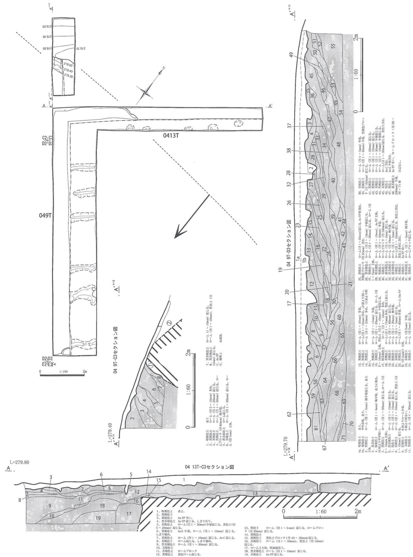
第 153 図 本丸地区 C3・D3 グリット 049T・0413T (平面図・セクション図)
