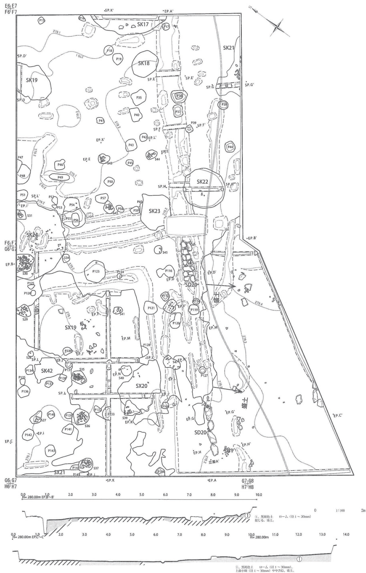
第162図 本丸地区F7・G7グリット（平面図・エレベーション図①）
