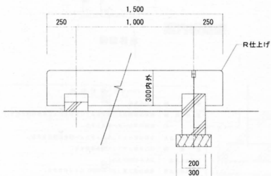
正面断面詳細図
