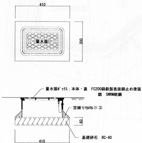
量水器
