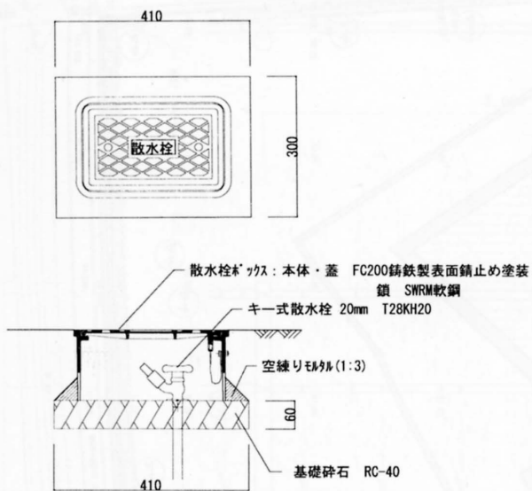
散水栓
