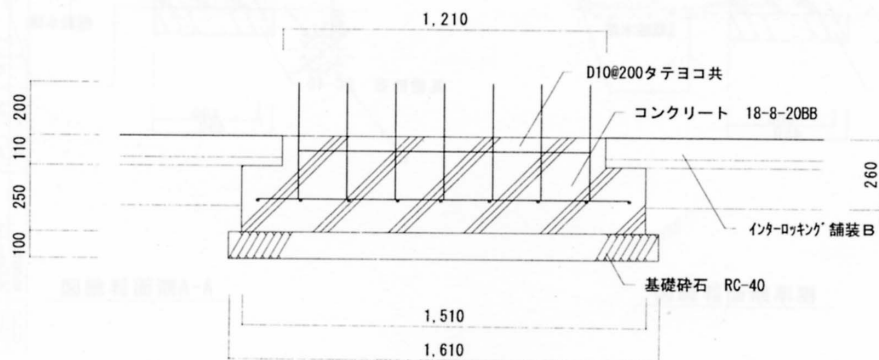
第13図 切石縁石・同B断面詳細図、地先境界ブロック断面詳細図、案内板基礎正面断面詳細図、車止め平面図・断面詳細図
