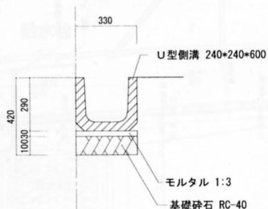
断面詳細図
