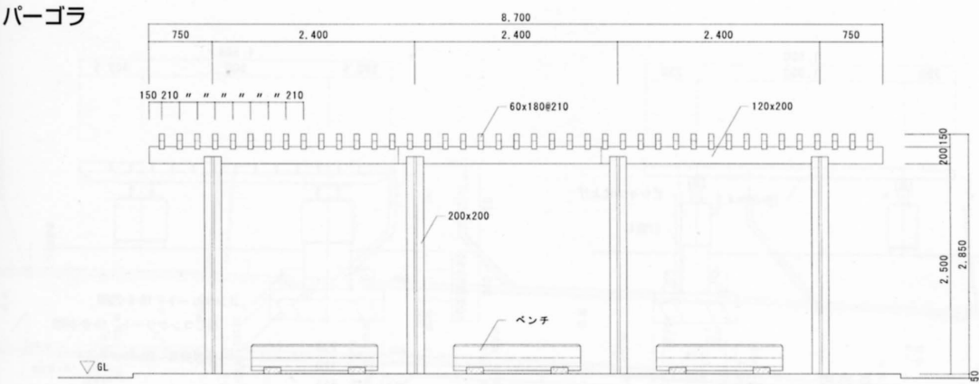
立断面図
