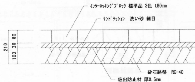
断面詳細図
