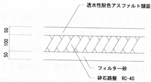
透水脱色アスファルト舗装詳細図
