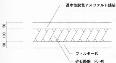
断面詳細図
