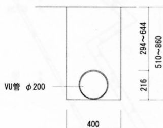
断面詳細図
