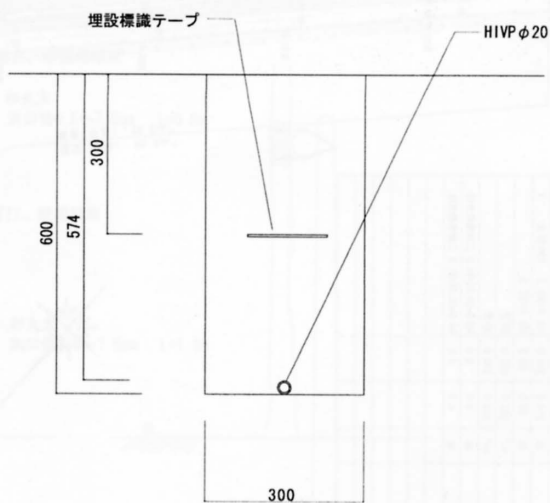
HIVPφ20
