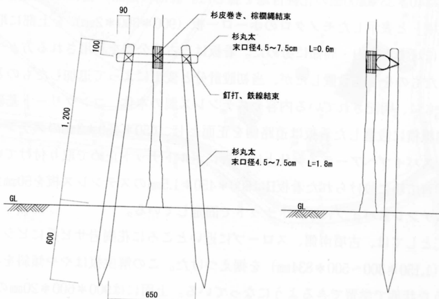
第24図 生垣支柱、二脚鳥居支柱
