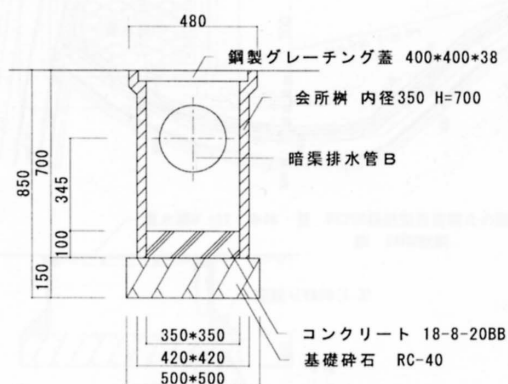
断面詳細図
