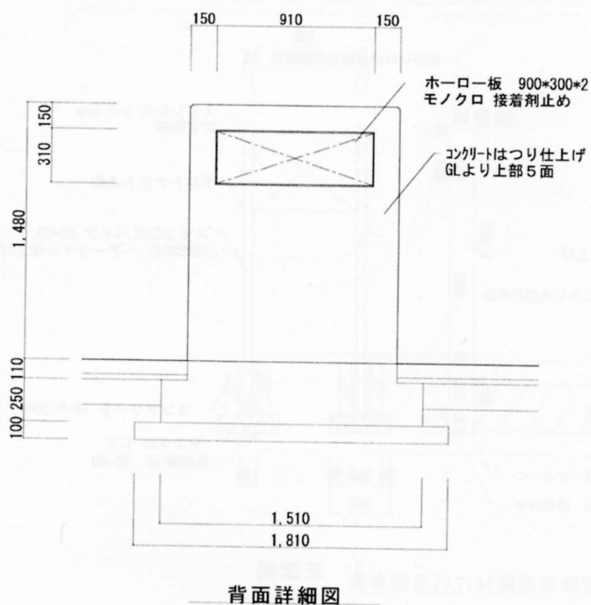
第27図 案内板平面図・正面詳細図・背面詳細図・側面断面詳細図
