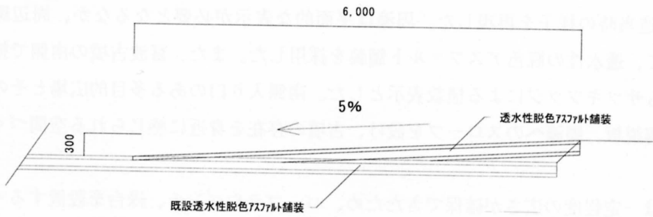
断面図
