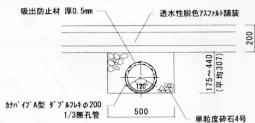
断面詳細図
