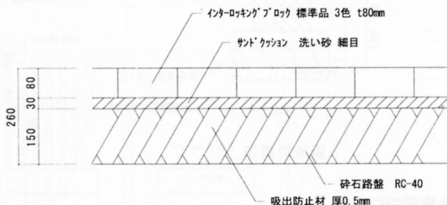
断面詳細図
