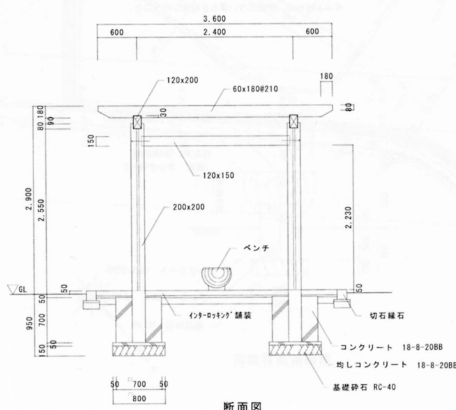
第14図 パーゴラ立断面図・平面図・断面図・柱詳細図
