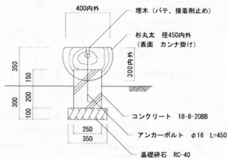
側面断面詳細図
