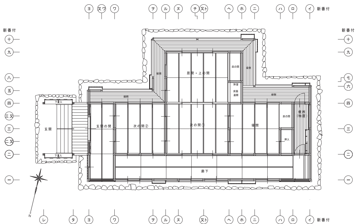
竣工平面図
