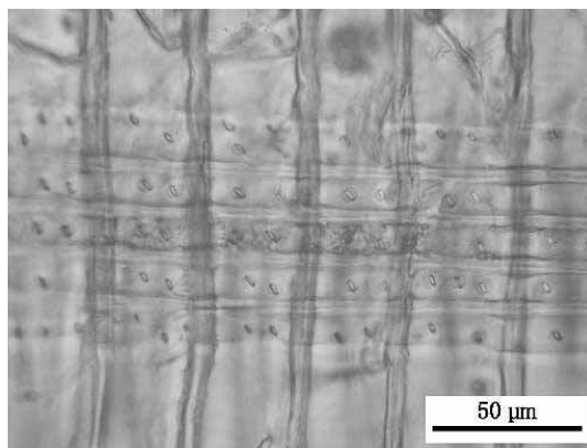
柱ホー十 (No. 3) から採取した木片の柁目面 (400α×)
