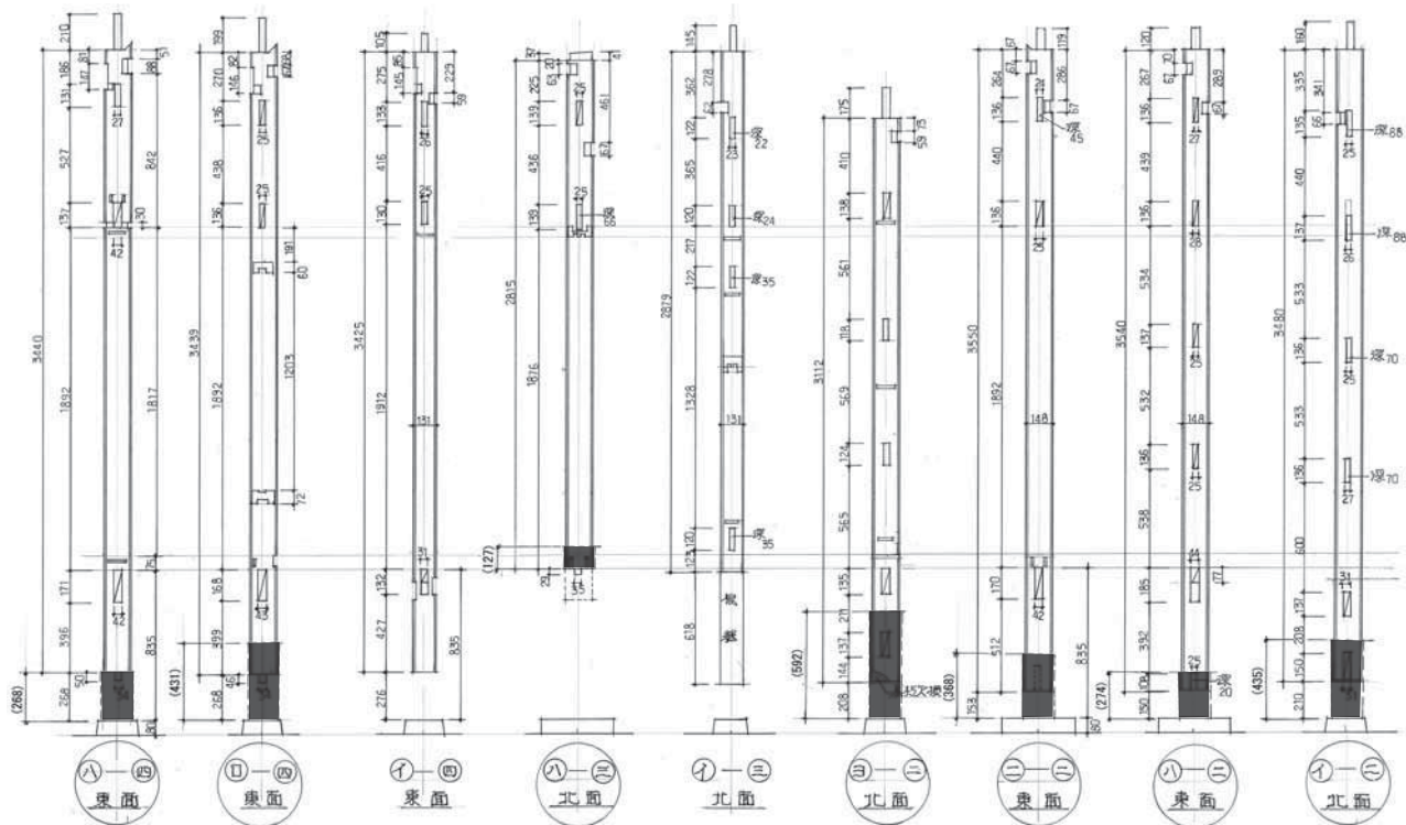
根継ぎ位置図 No. 2
