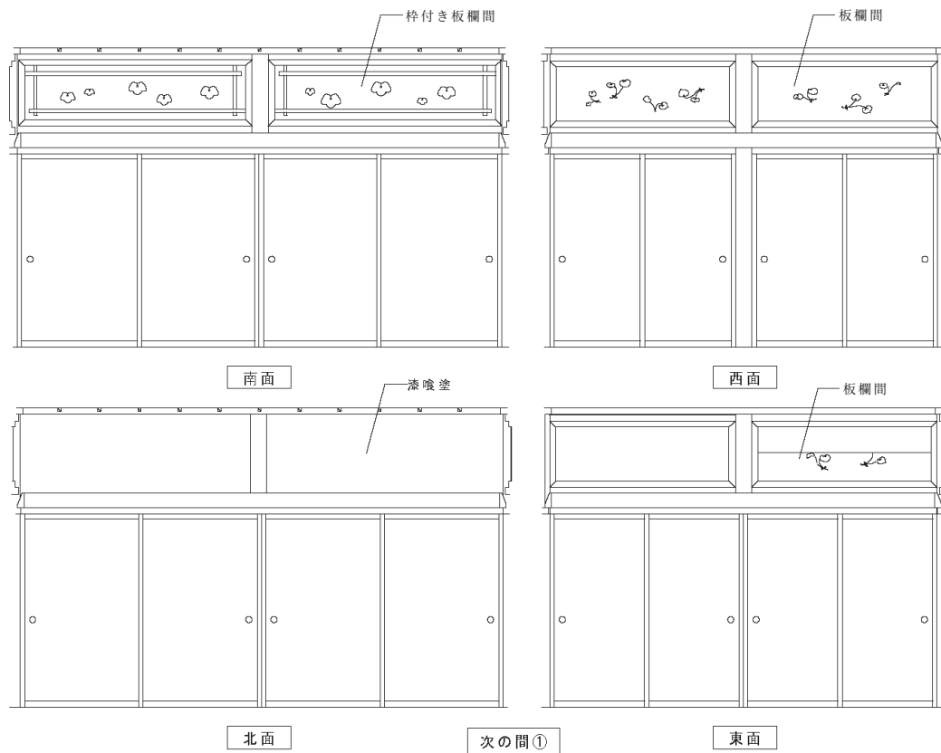
次の間①展開図
