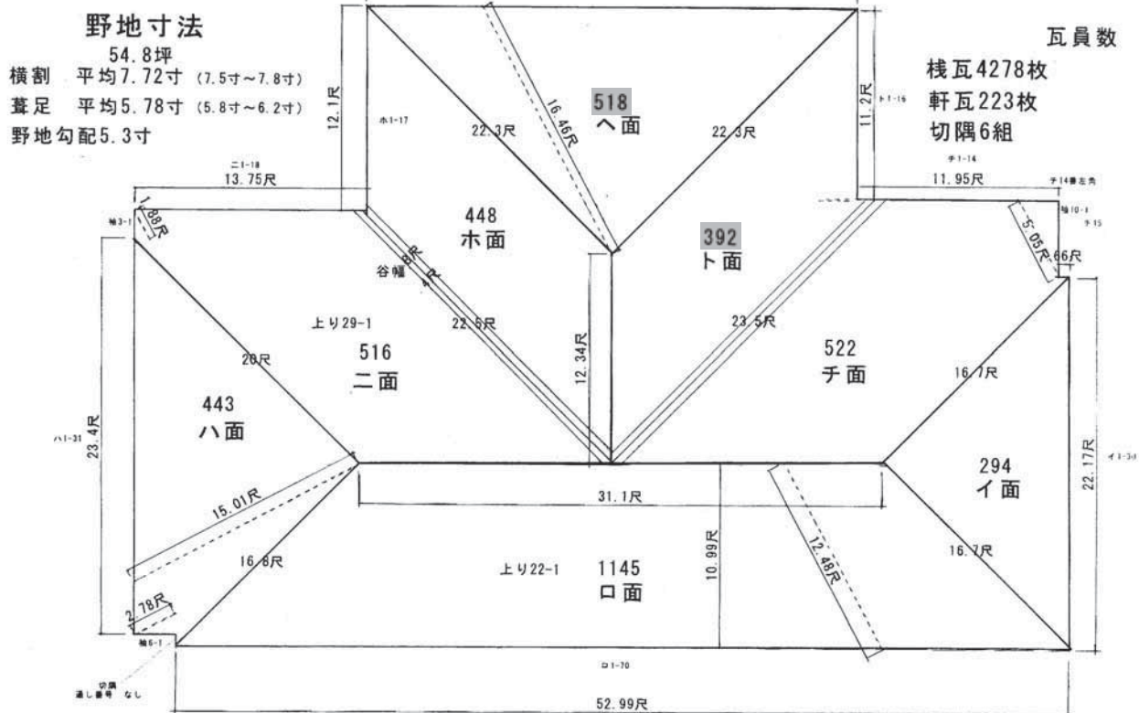
移築前屋根瓦図
