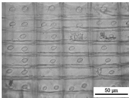
桁ルー四～九 (No. 4) から採取した木片の柁目面 (400α×)
