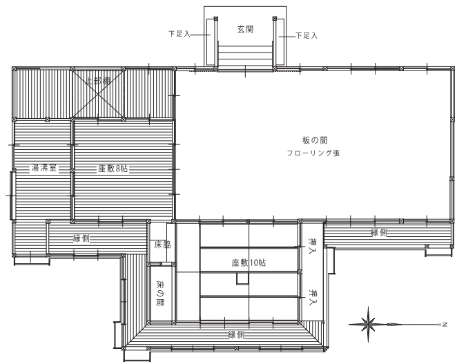
小島公会堂（解体前）平面図
