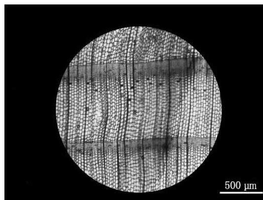
桁ルー四～九 (No. 4) から採取した木片の木口面 (100×)
