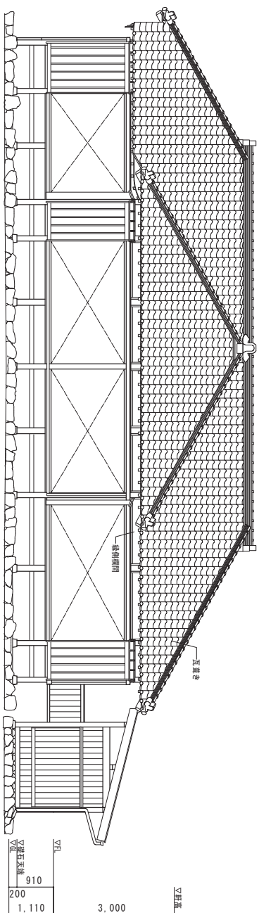
南側立面図
