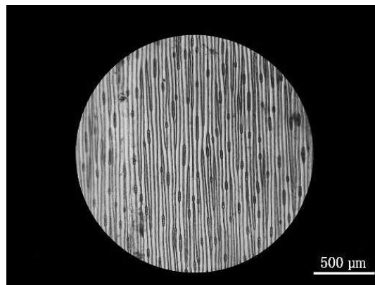
野隅木トー六〜ヲー10 (No. 8) から採取した木片の板目面 (100×)
