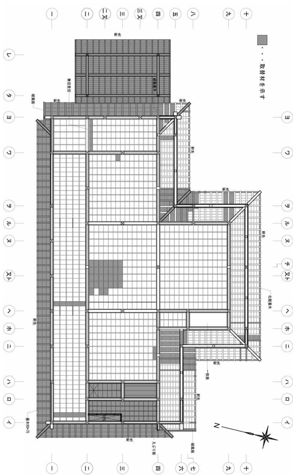
天井伏図
