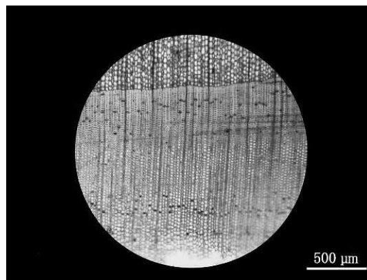
垂木帯鋸仕上げ (No. 7) から採取した木片の木口面 (100×)
