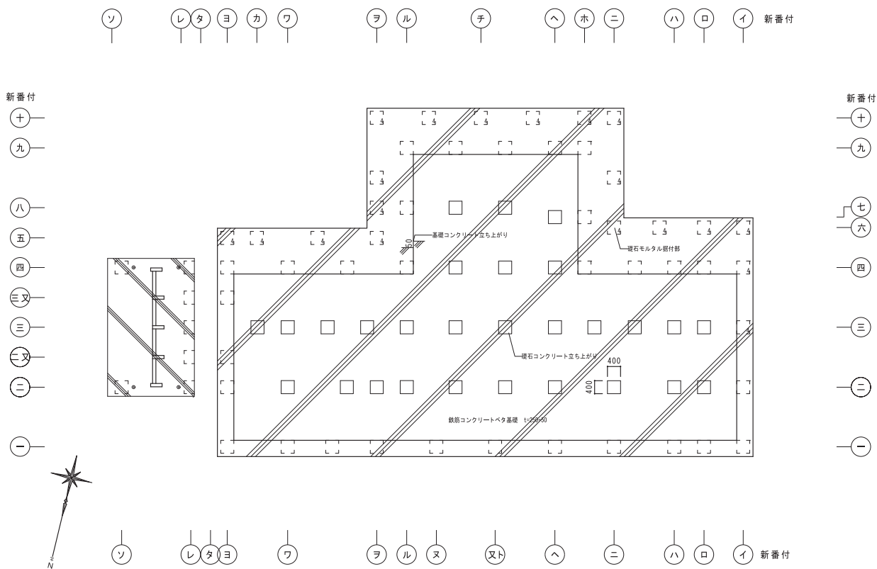
竣工基礎伏図
