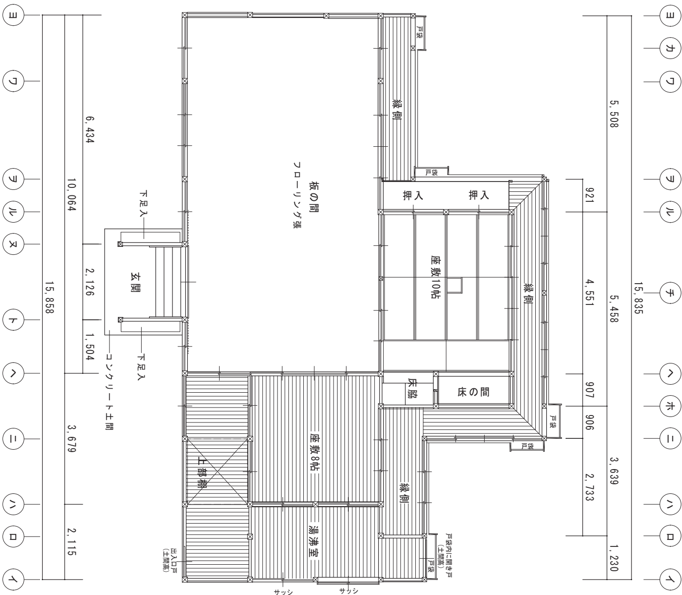
移築前平面図 1/100
