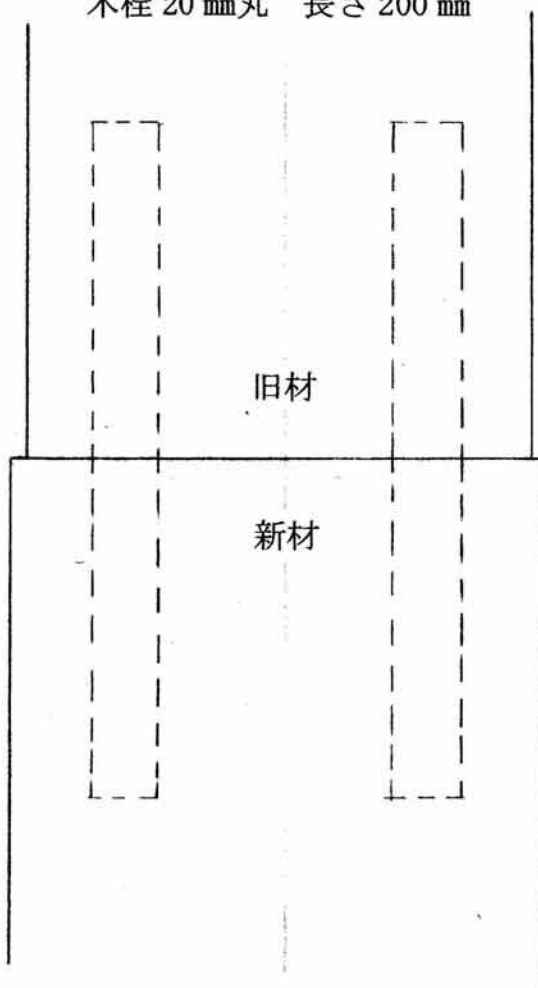
柱根継ぎ図 S = 1 / 2
