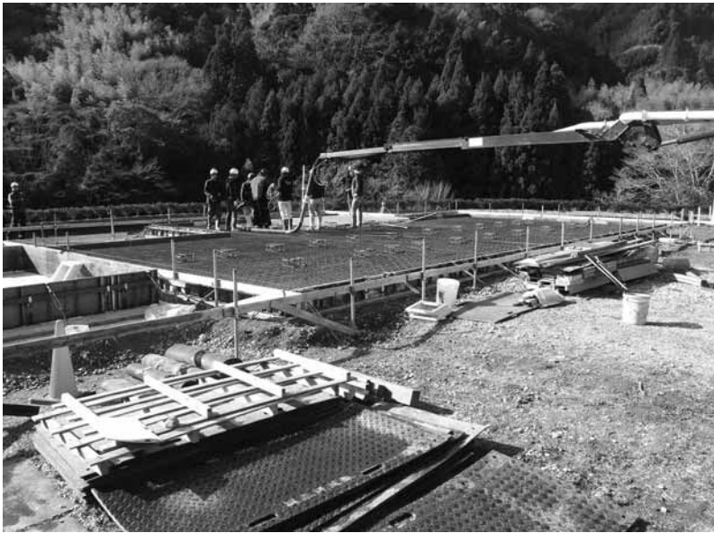
40. ベースコンクリート打ち
