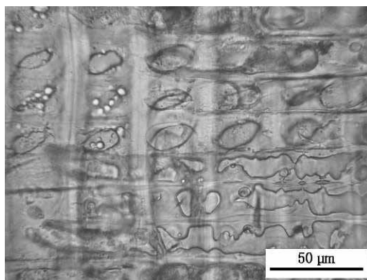
垂木ヨキ仕上げ (No. 6) から採取した木片の柁目面 (400α×)
