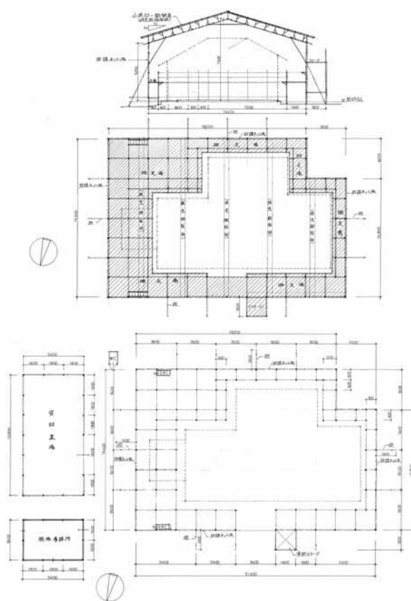
仮設図
