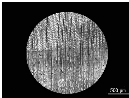
柱ヘー九 (No. 2) から採取した木片の木口面 (100×)
