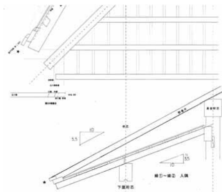
毛抜き合わせ納まり図（図一）
