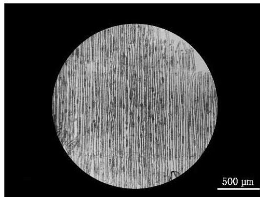
柱ヘー九 (No. 2) から採取した木片の板目面 (100×)
