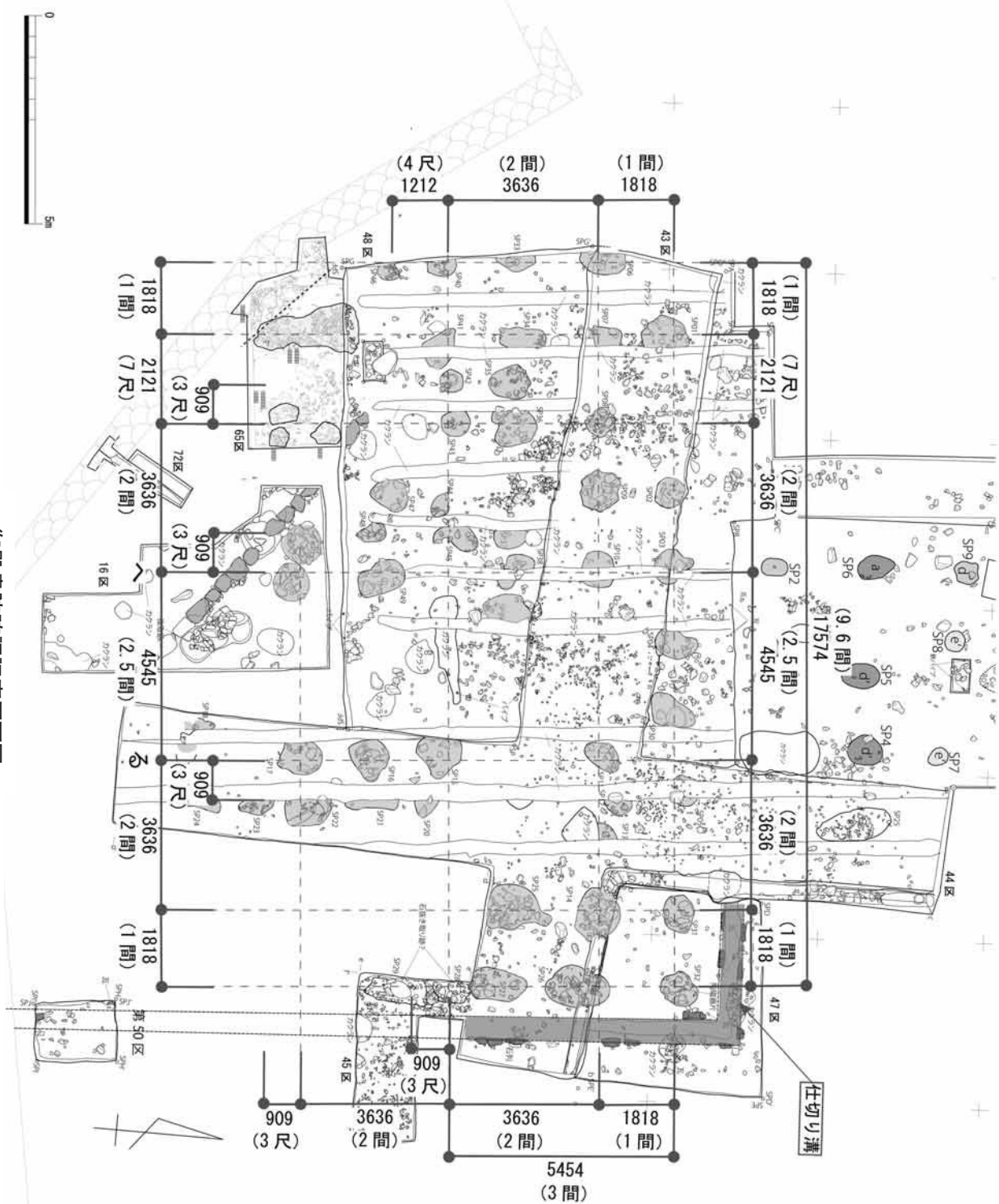
御殿書院確認調査平面図
