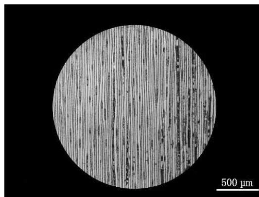
桁ルー四～九 (No. 4) から採取した木片の板目面 (100×)
