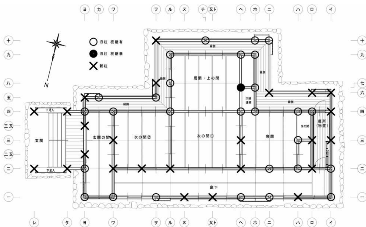
柱根継位置図
