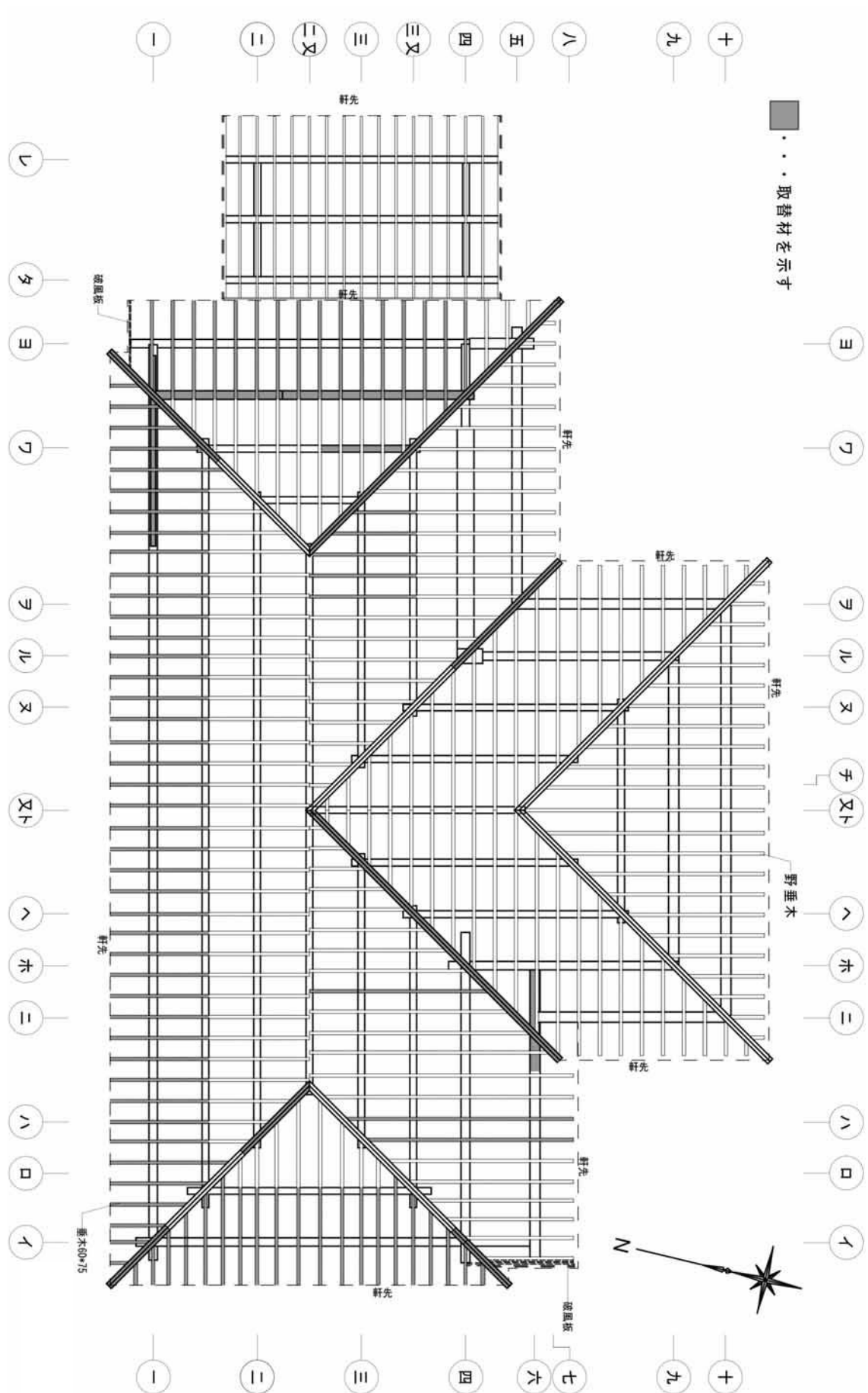
垂木伏図
