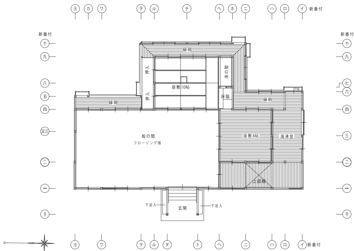
修理番付図
