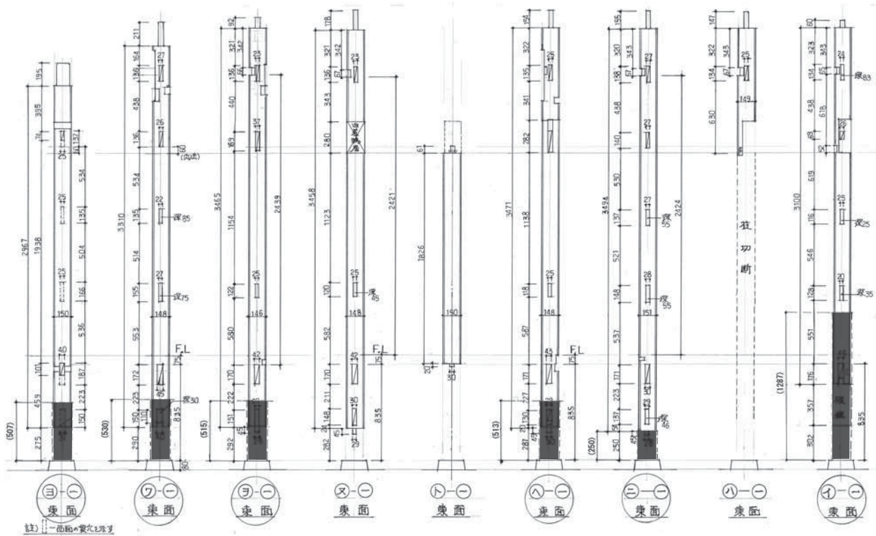
根継ぎ位置図 No. 1
