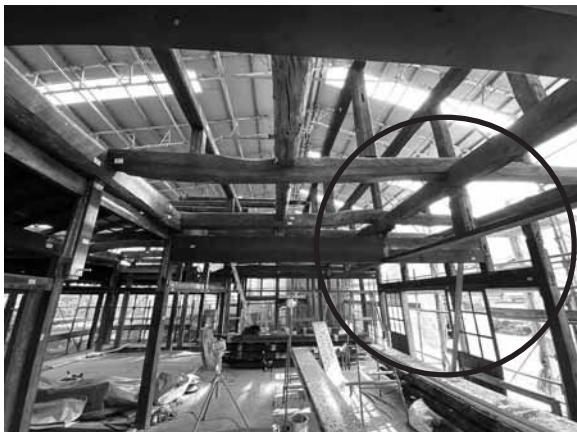
ルー一 大梁受け写真
