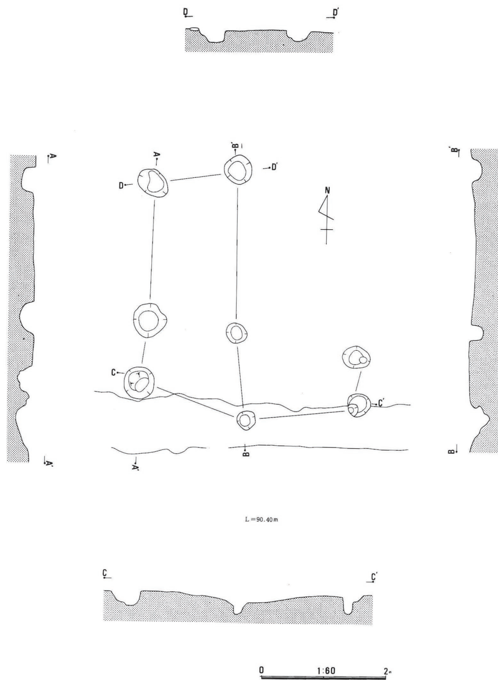
第28図 S B 6 遺構図
