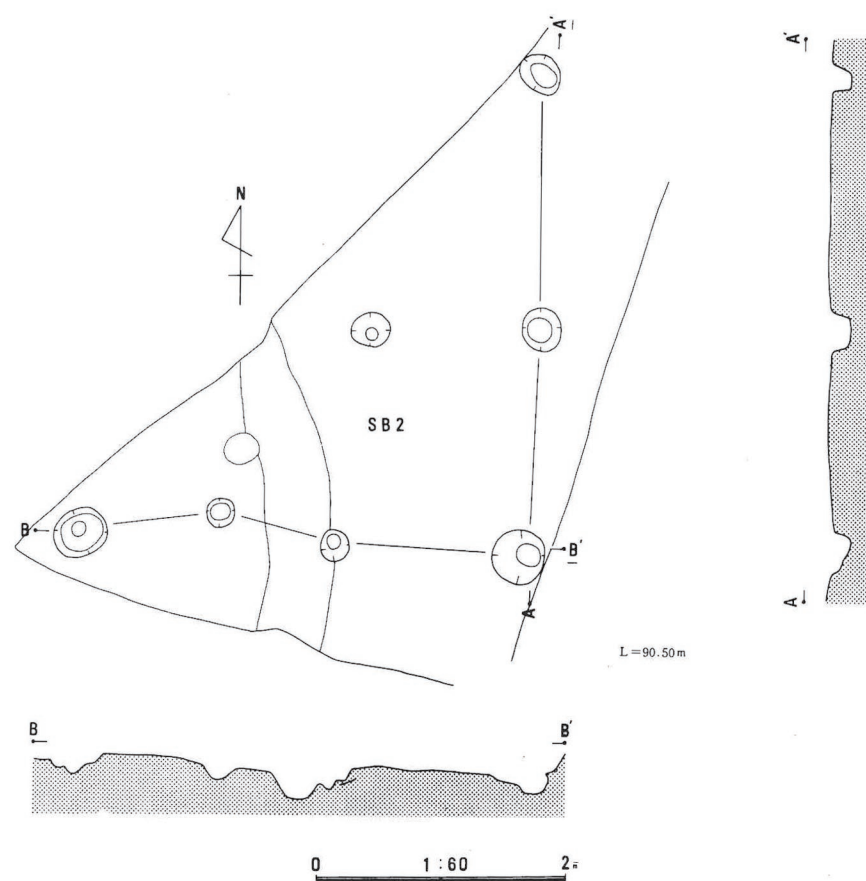
第26図 SB 5 遺構図
