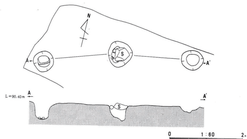
第25図 SB 3 遺構図
