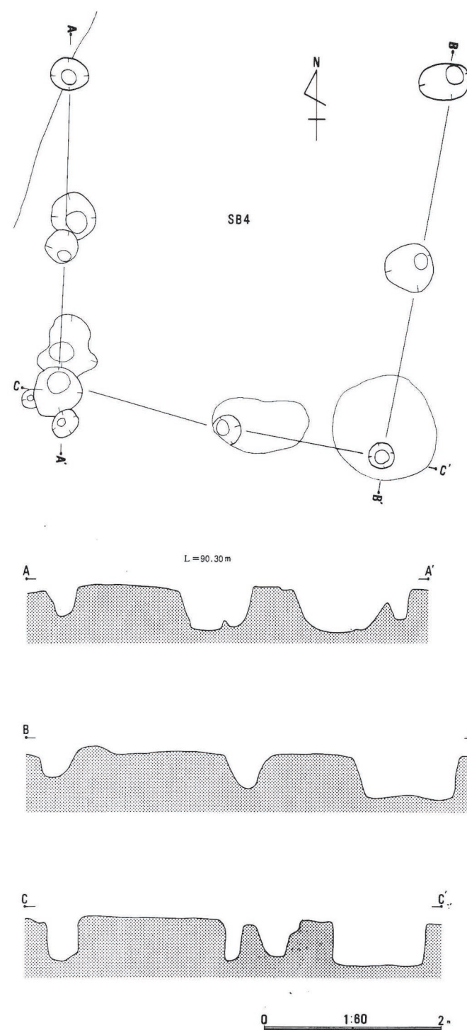
第27図 SB 4 遺構図
