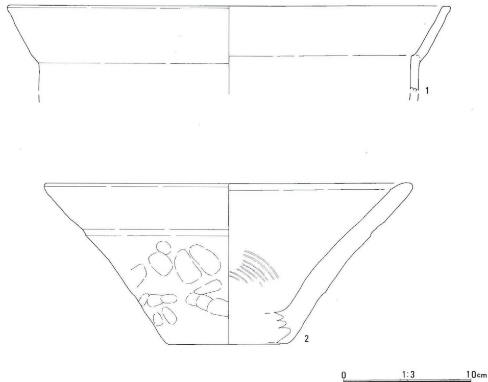
第10図 SD2出土遺物
