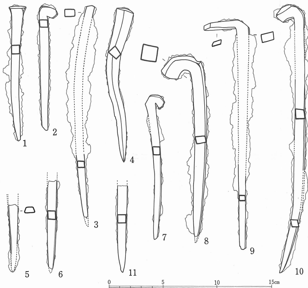
第24図 法鏡寺跡出土瓦釘実測図
