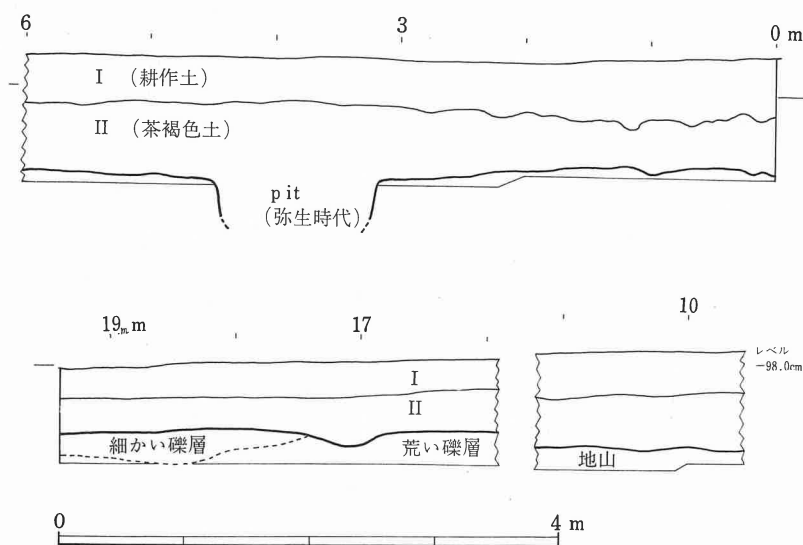
第11図 法鏡寺跡Ⅻトレンチ（金堂西側）土層実測図
