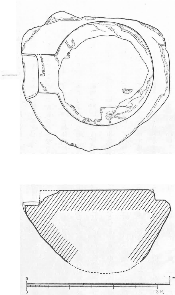
第52図 虚空蔵寺跡金堂礎石実測図
