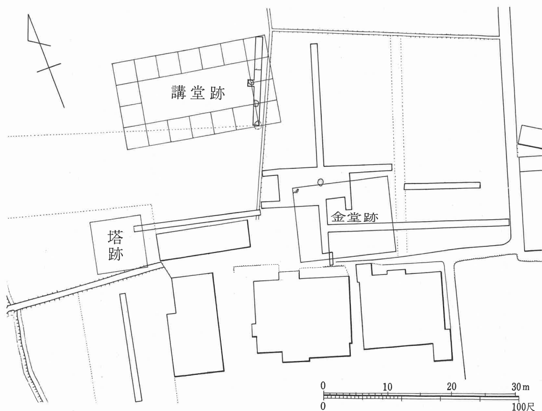
第29図 法鏡寺伽藍復原想定図 (一)
