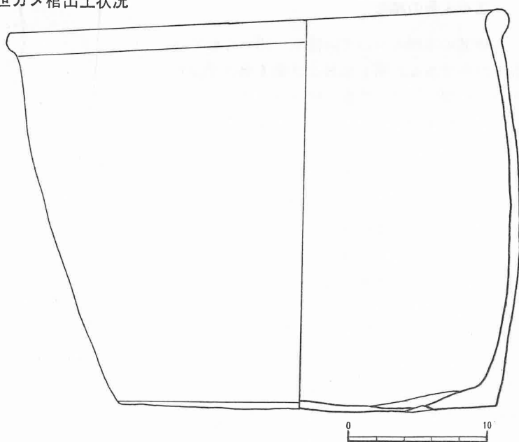
第17図 カメ棺実測図
