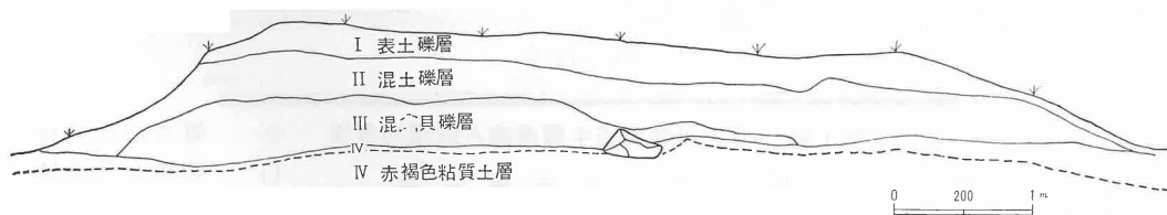
第3図 貝塚西側土層断面図
