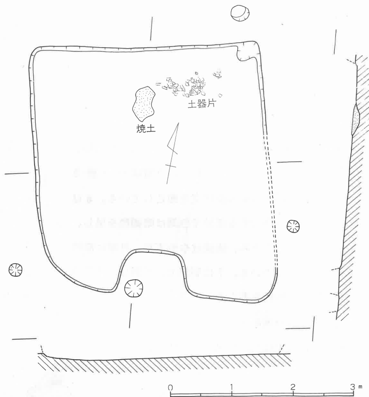
第9図 2号住居跡実測図
