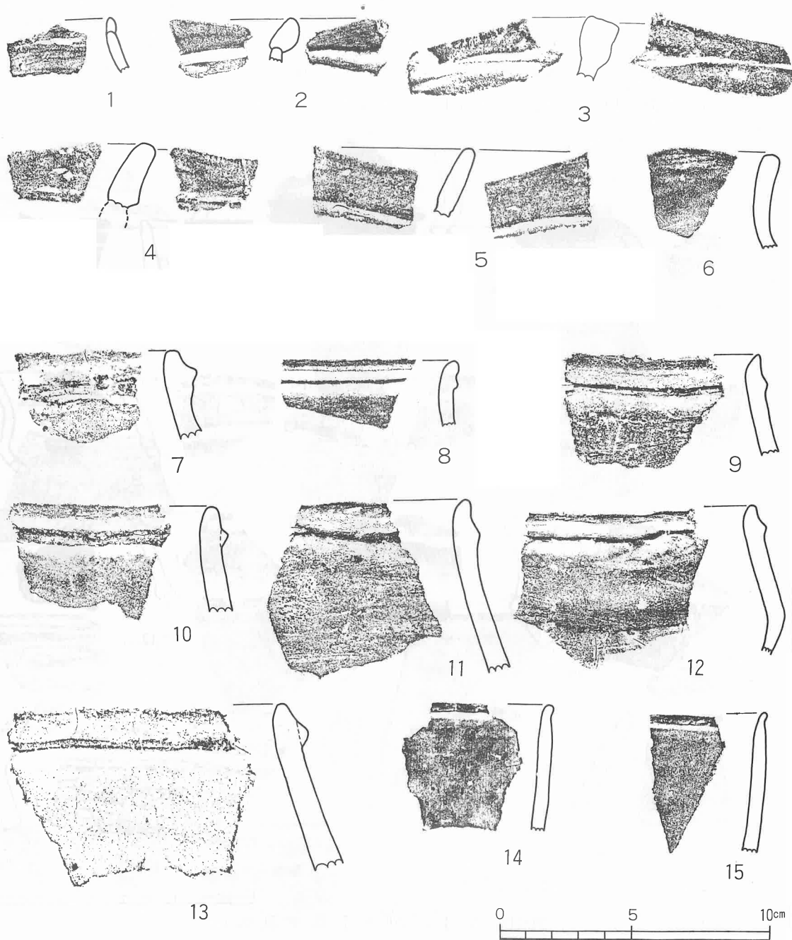
第32図 第I区出土土器実測図(4)
