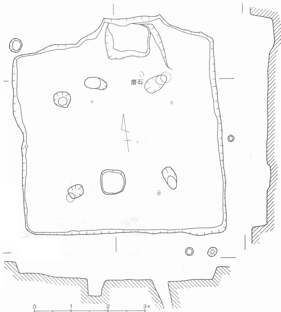
第17図 5号住居跡実測図
