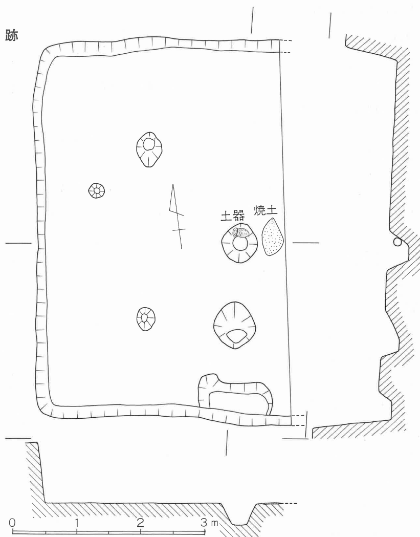
第11図 3号住居跡実測図
