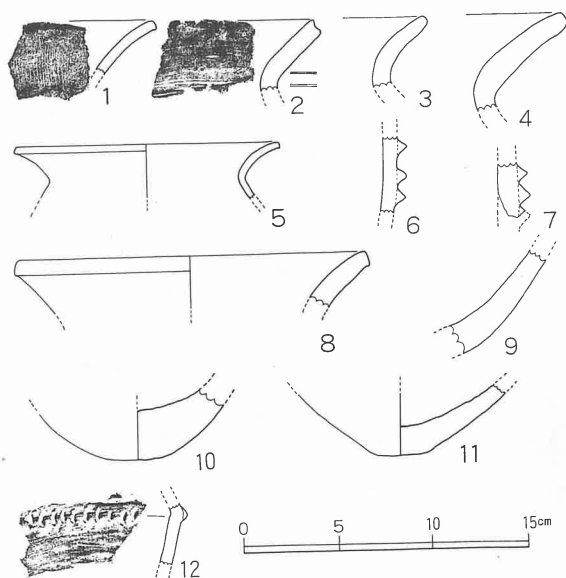
第13図 3号住居跡出土土器実測図(2)
