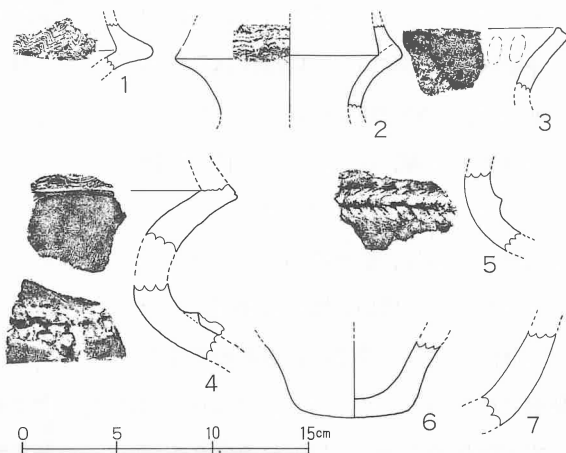
第10図 2号住居跡出土器実測図
