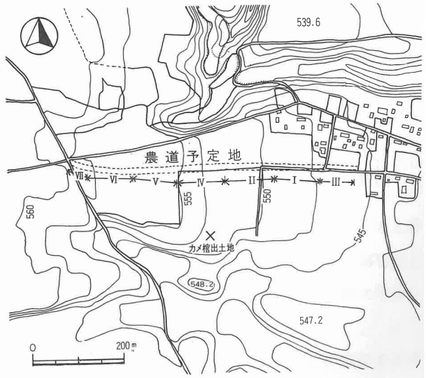
第3図 遺跡周辺の地形図（調査区と縄文晩期カメ棺出土地点×）
