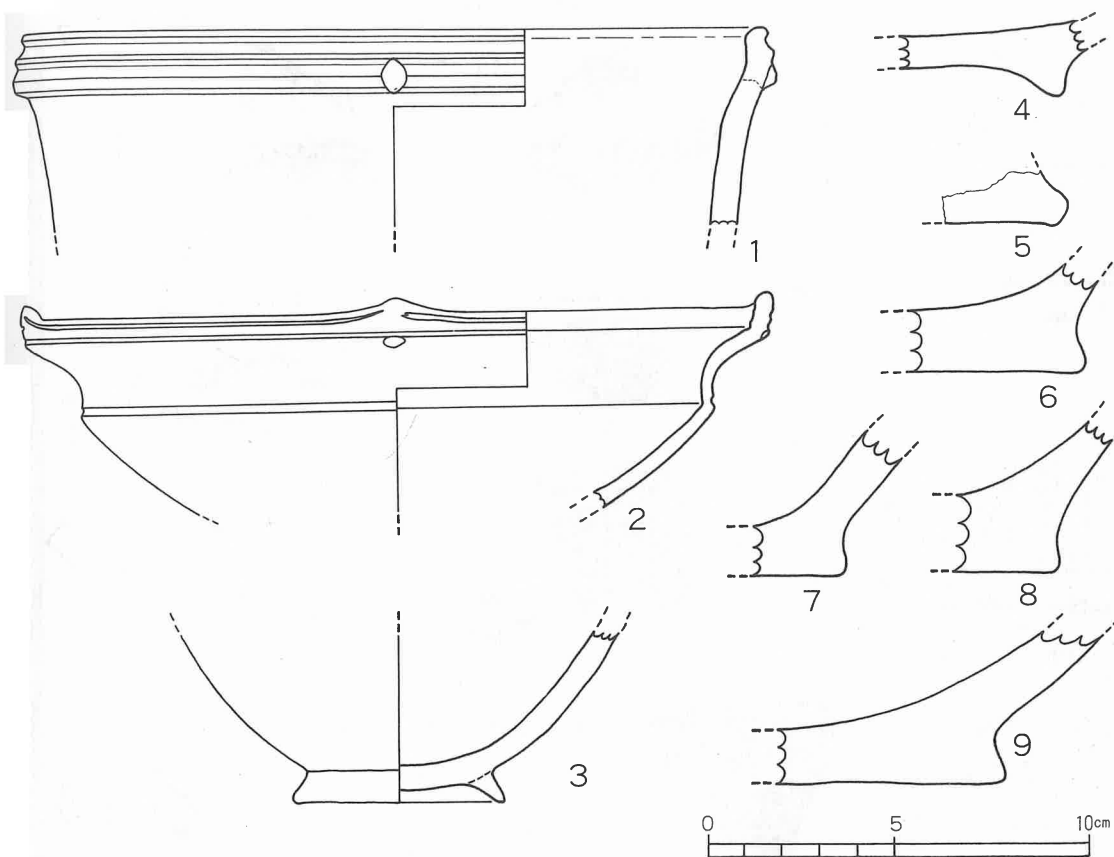
第29図 第I区出土土器実測図(1)
