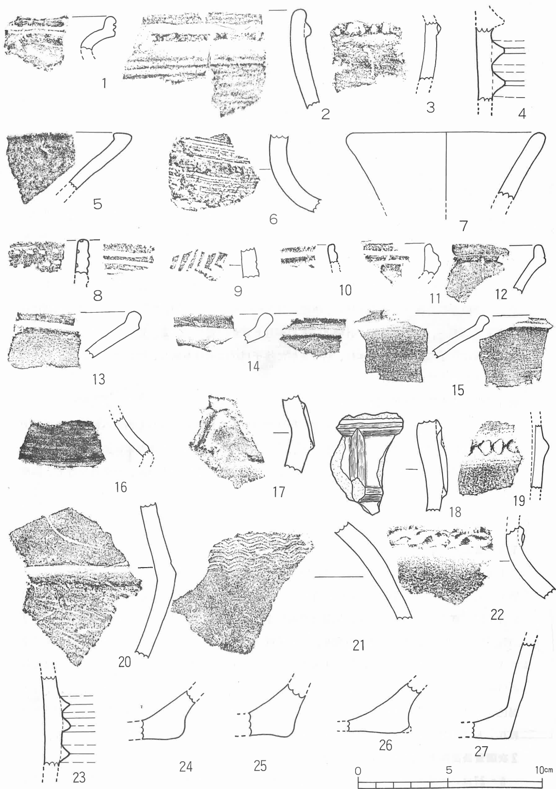
第36图 表面采集土器实测图
