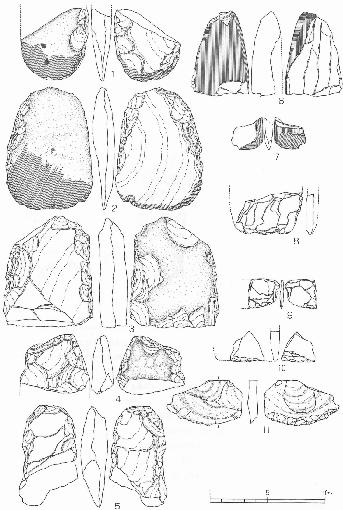
第40图 表面采集石器实测图(2)
