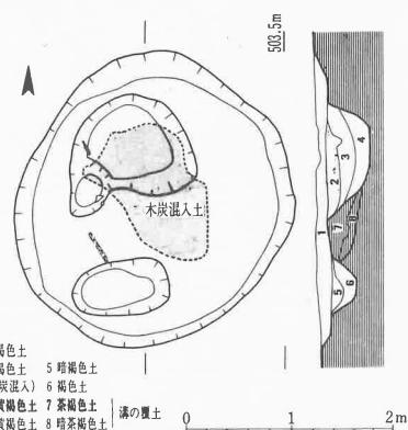
第48図 第16号竪穴実測図
