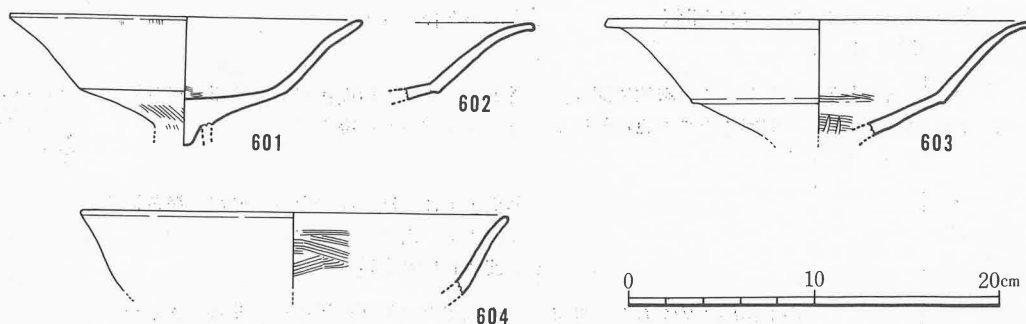
第18図 第6号竪穴出土土器実測図
