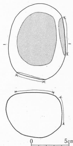
第32図 第11号竪穴出土石器実測図
