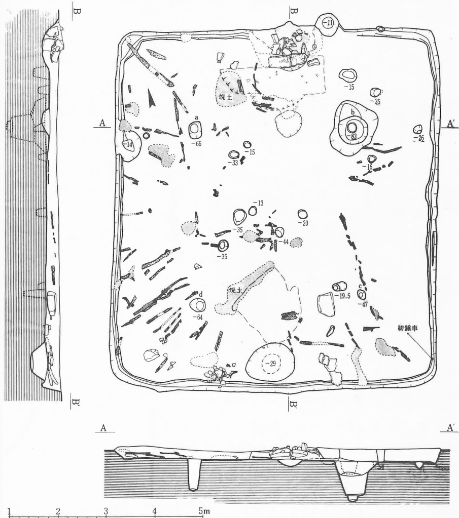
第49図 第17号竪穴実測図
