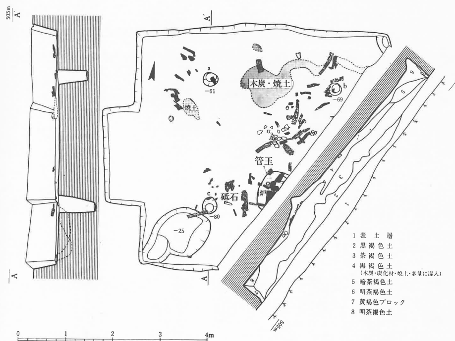
第34図 第 12 号 竖 穴 実 測 図
