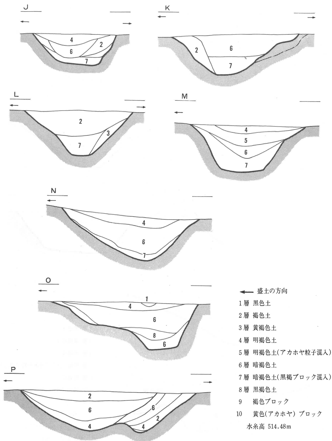
第56図： 方形周溝墓周溝土層図(2)
