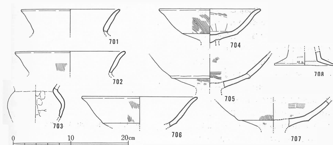
第20図 第7号竪穴出土土器実測図
