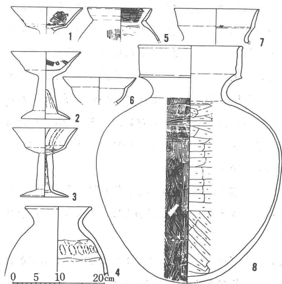
第66図 小園遺跡第110号住居跡出土土器（1/8）
