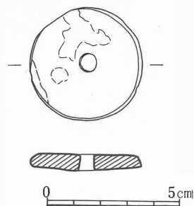
第52図 第17号竪穴出土紡錘車実測図
