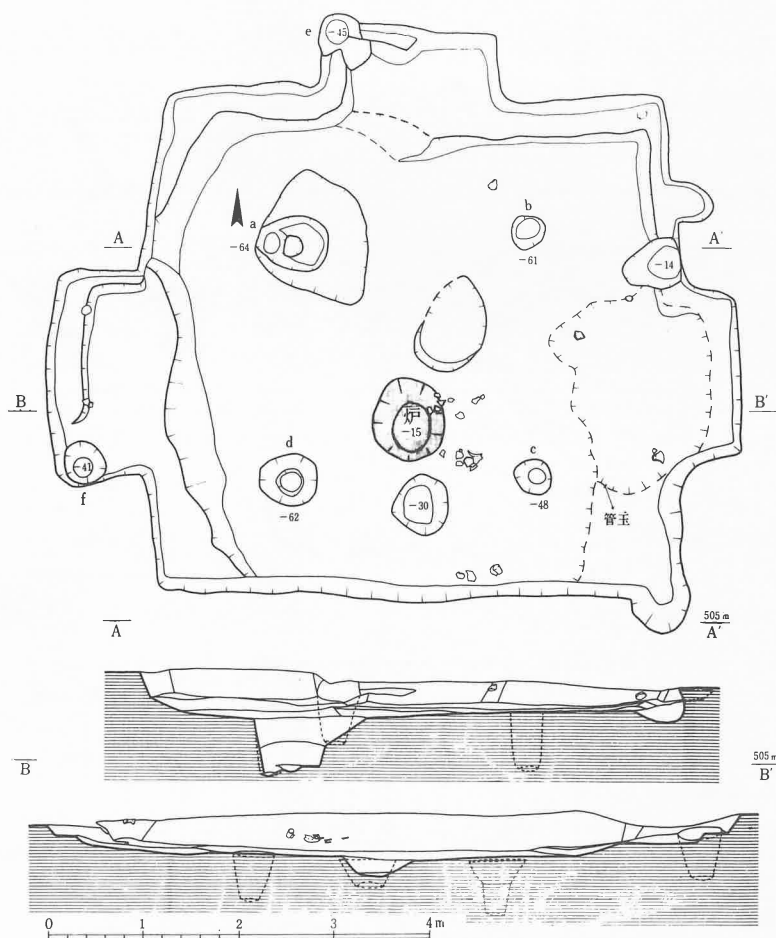
第40図 第 14 号 竪 穴 実 測 図
