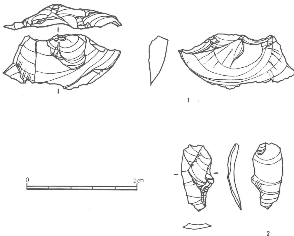
第83図 楠野遺跡K J I 地区の石器 (1/1)
