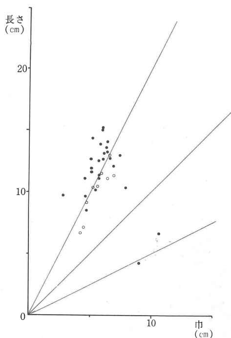
第97図 後期後半の打製石斧の相関図 (白ヌキは欠損品の現在長)
