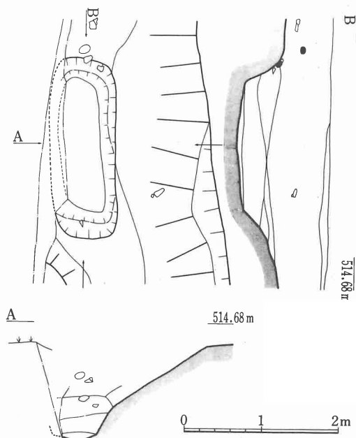
第53図 第2号方形周溝墓周溝内土壇墓実測図
