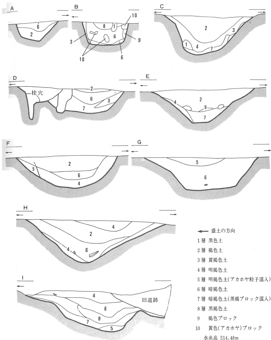
第55図 方形周溝墓周溝土層図(1)
