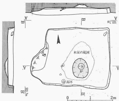
第19図 第7号竪穴実測図
