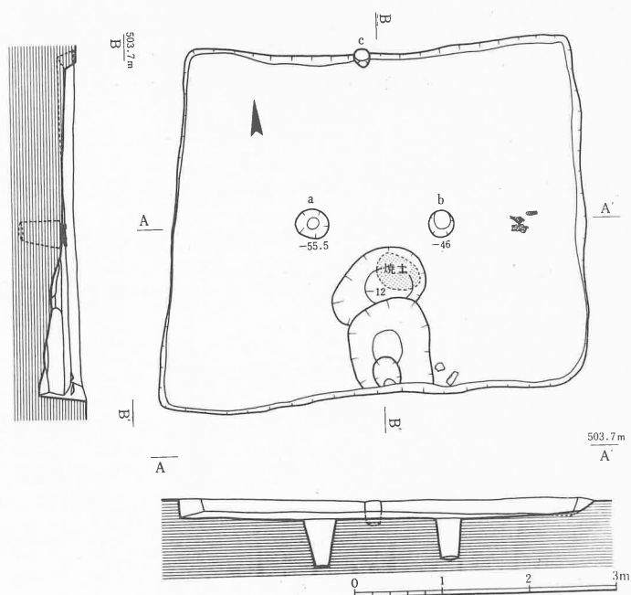
第17図 第6号竖穴実測図
