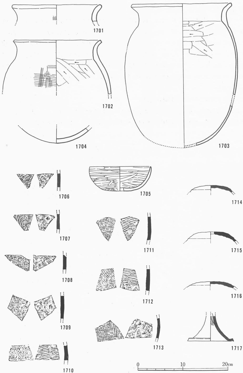
第50图 第17号竖穴出土土器实测图
