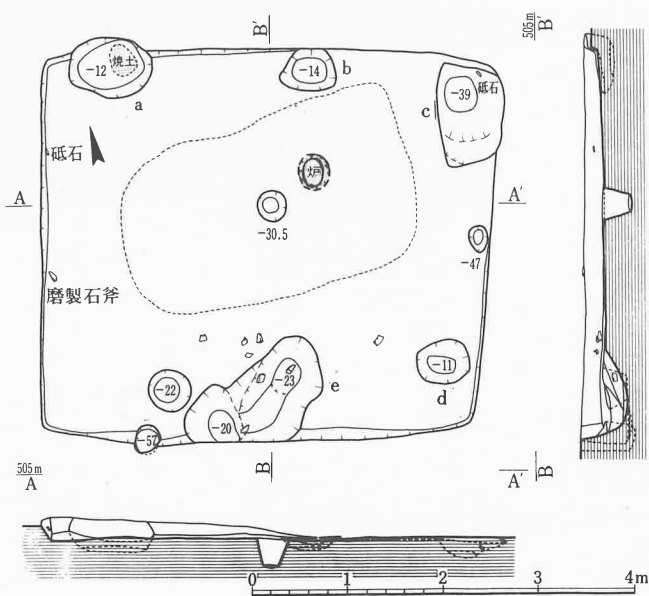
第37図 第13号堅穴実測図
