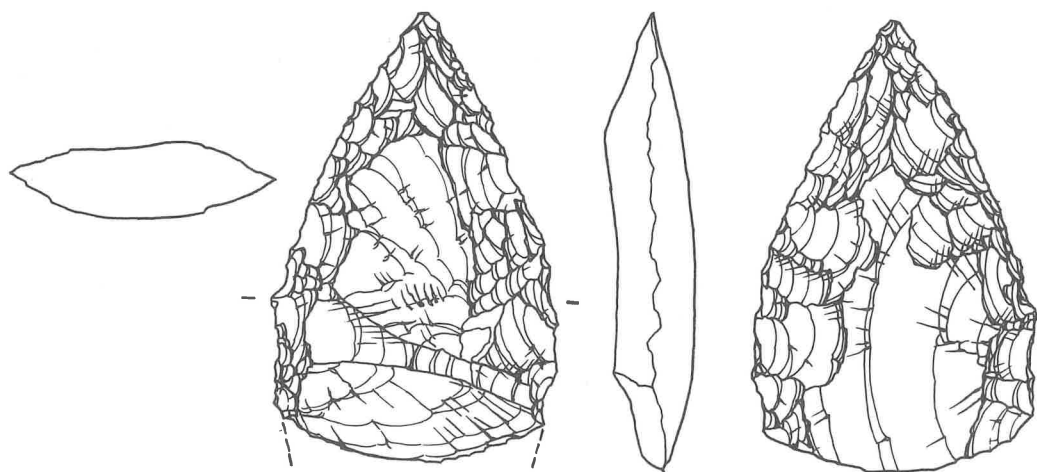
第91図 楠野遺跡出土石器実測図 (7) (1/1)
