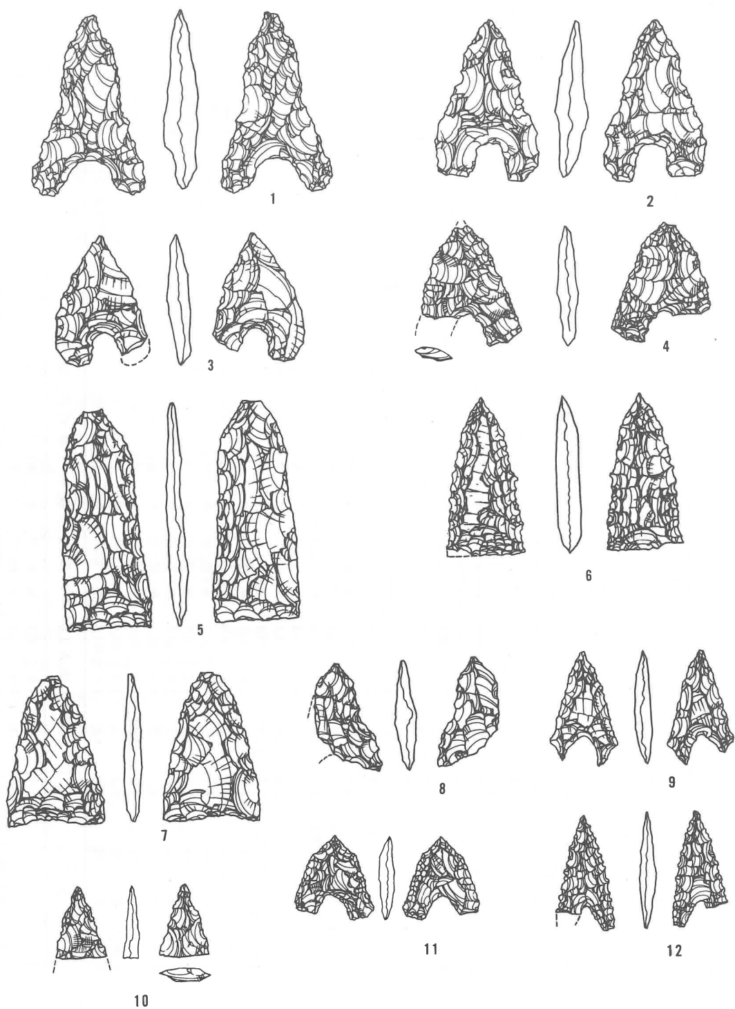
第88図 楠野遺跡出土石器実測図 (4) (1/1)
