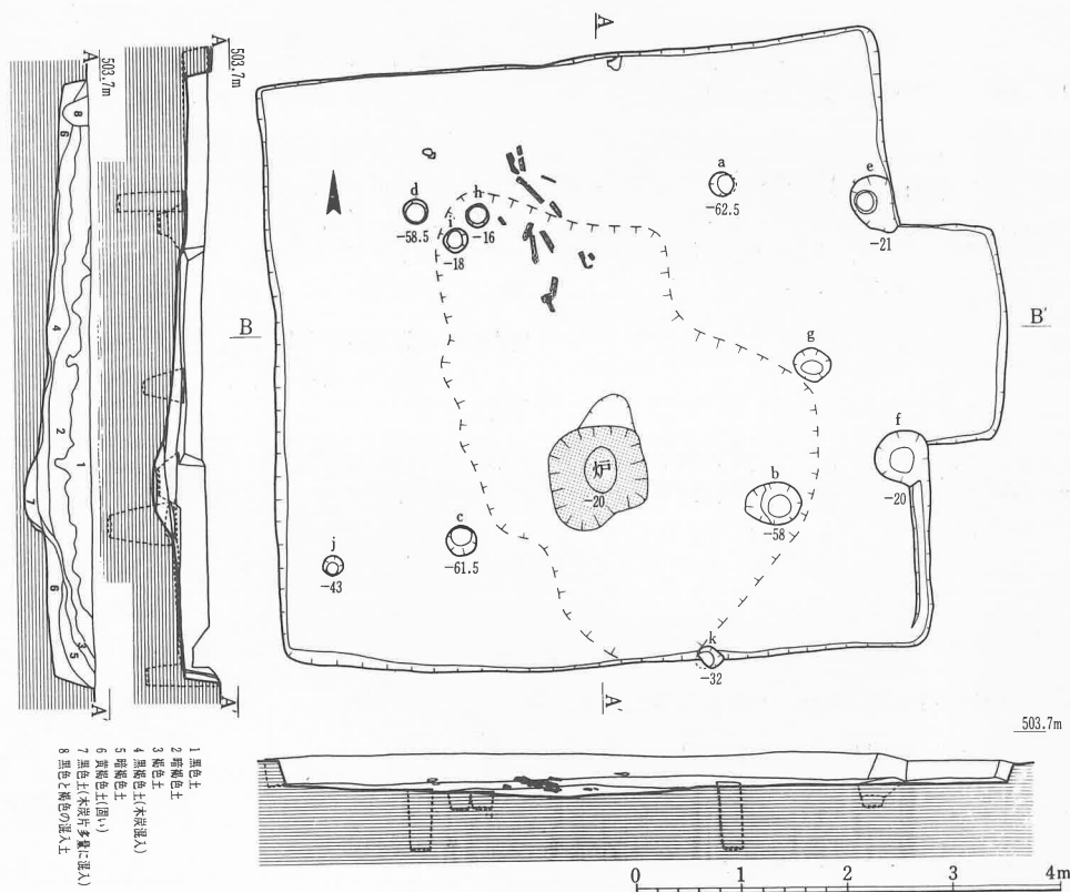
第4図 第1号堅穴実測図
