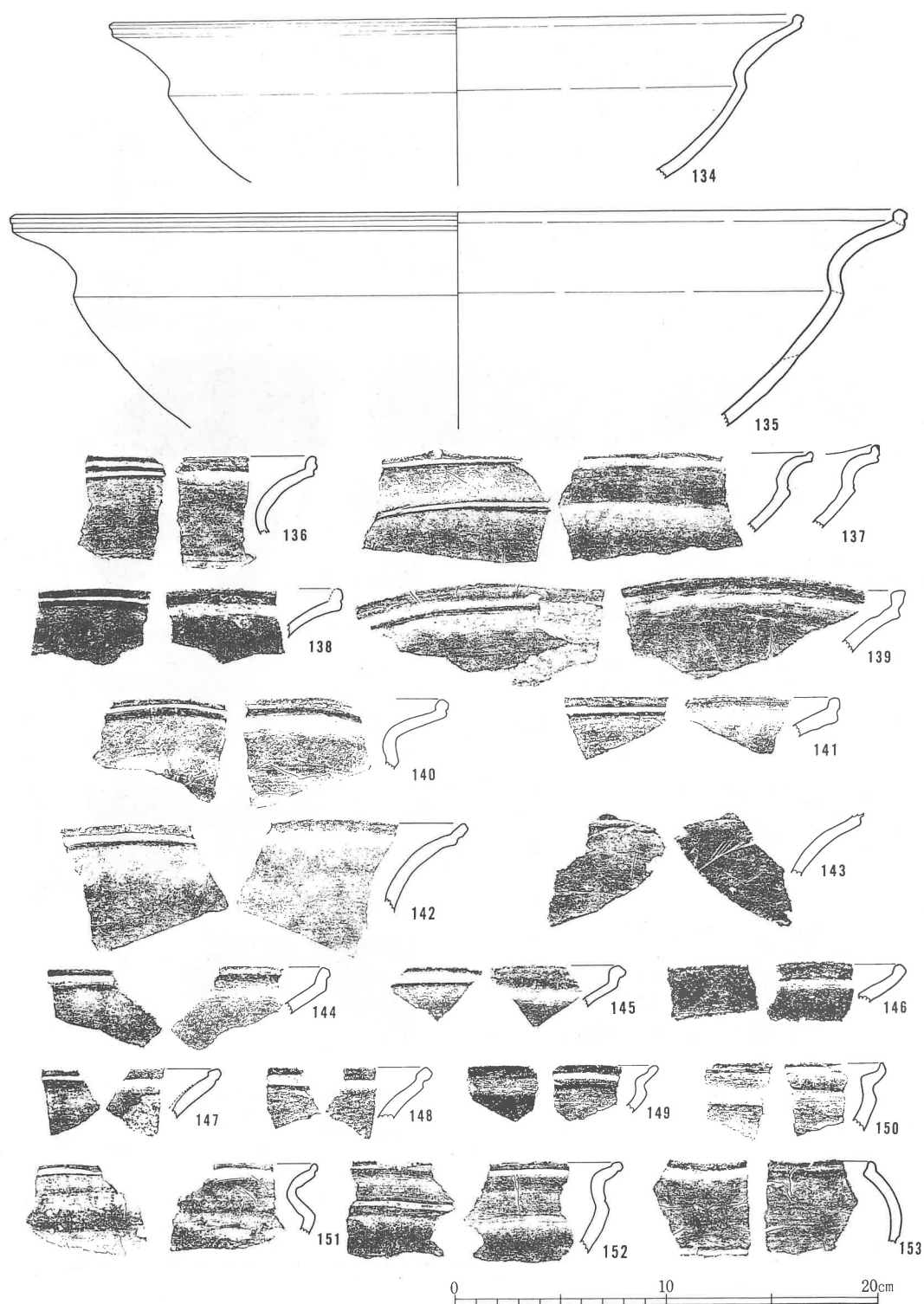
第80图 楠野遺跡K JⅡ—b地区出土土器实测图 (3)
