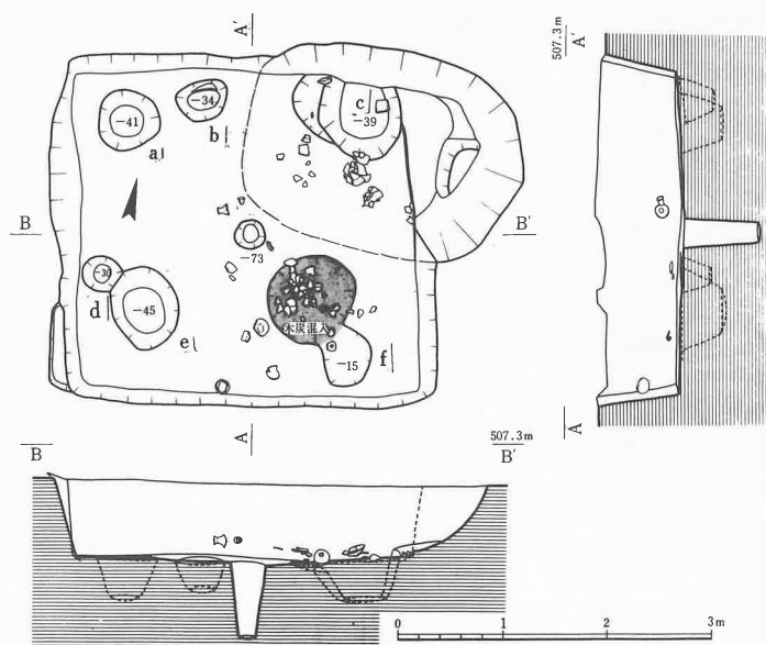
第7図 第2号竪穴実測図
