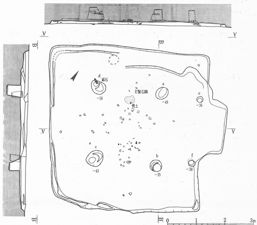
第46图 第15号竖穴实测图
