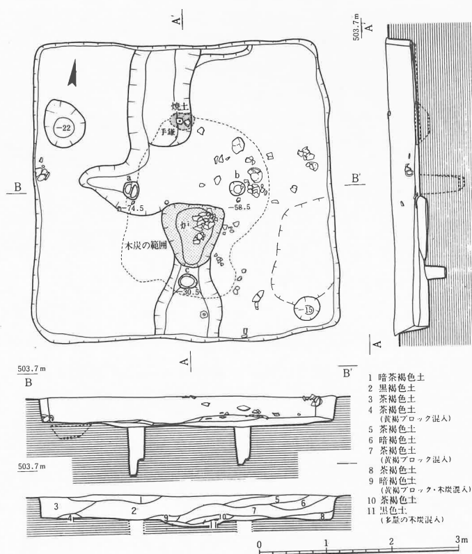
第10図 第3号竪穴実測図
