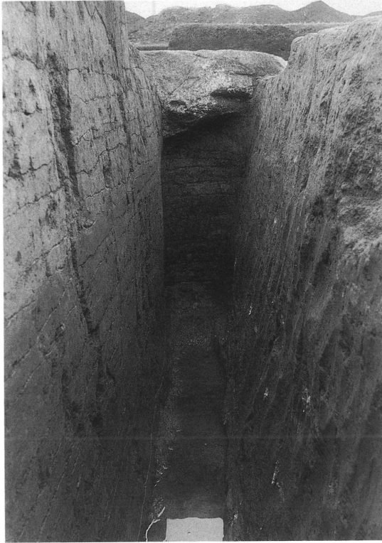
塔跡・掘り込み地業断面
