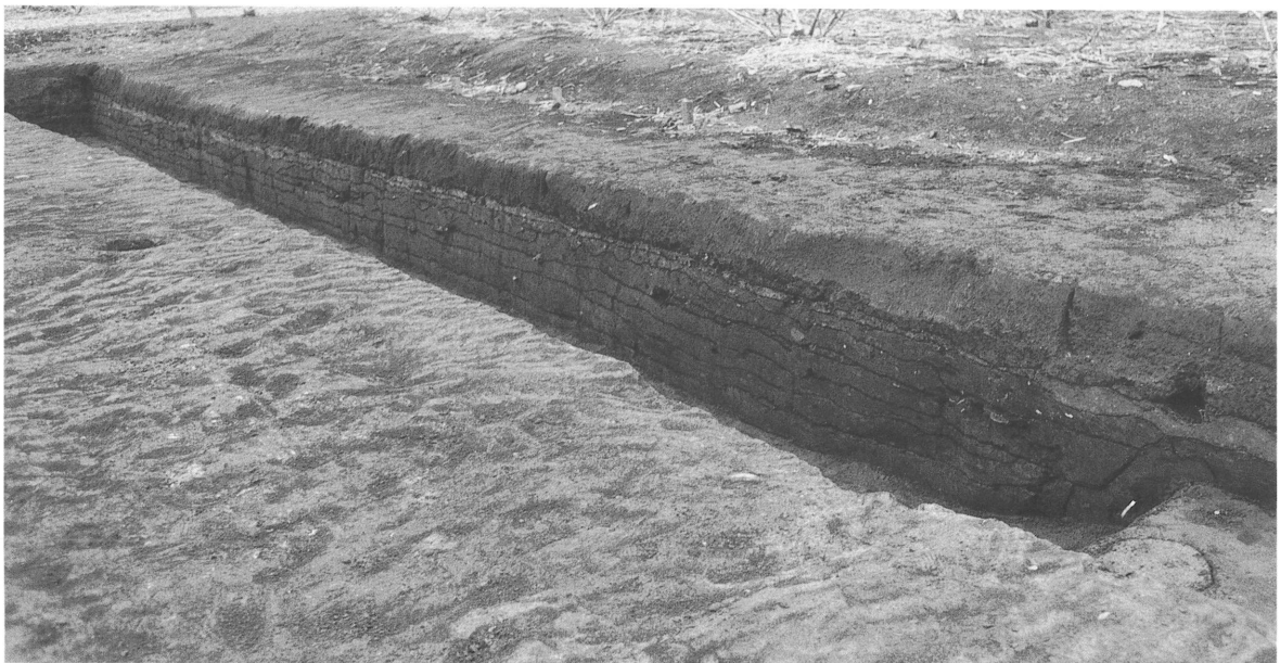
講堂跡・掘り込み地業（A－A'）
