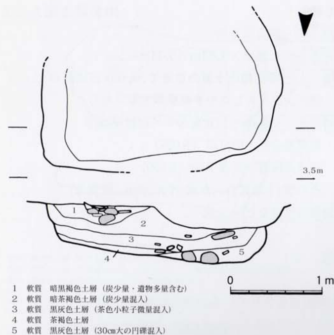
第13図 S026平面図 南面断面図 (1/40)
