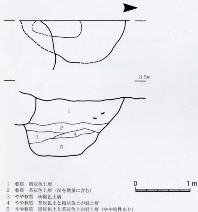
第14図 S036平面図 西面断面図 (1/40)
