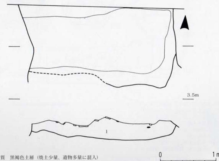
第20図 S087平面図 北面断面図 (1/40)
