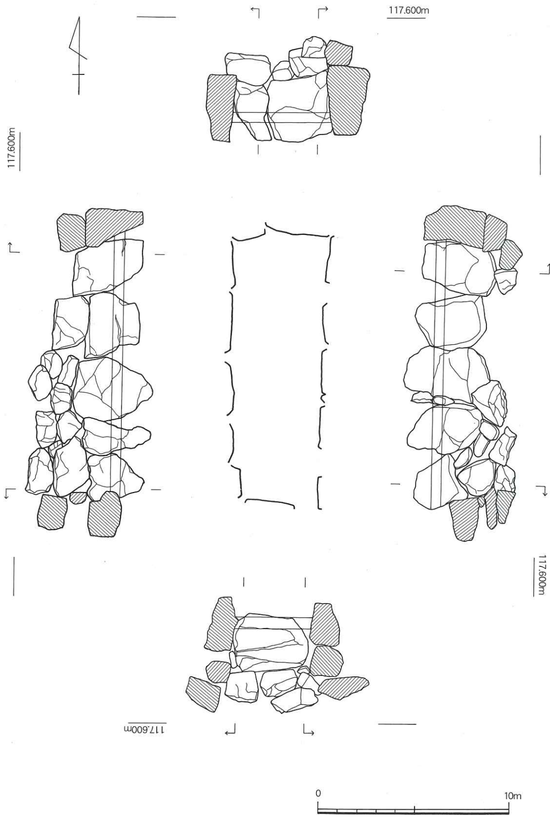
4号填石室立面实测图
