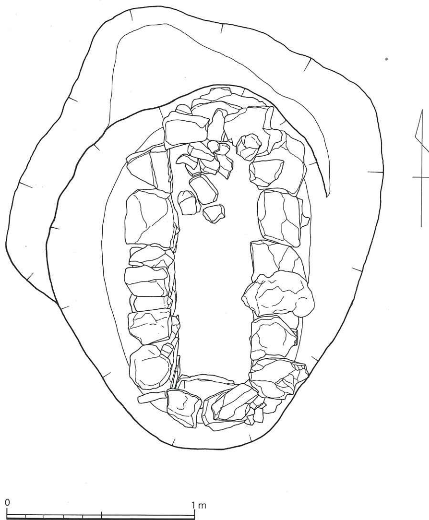
4号墳石室上面実測図
