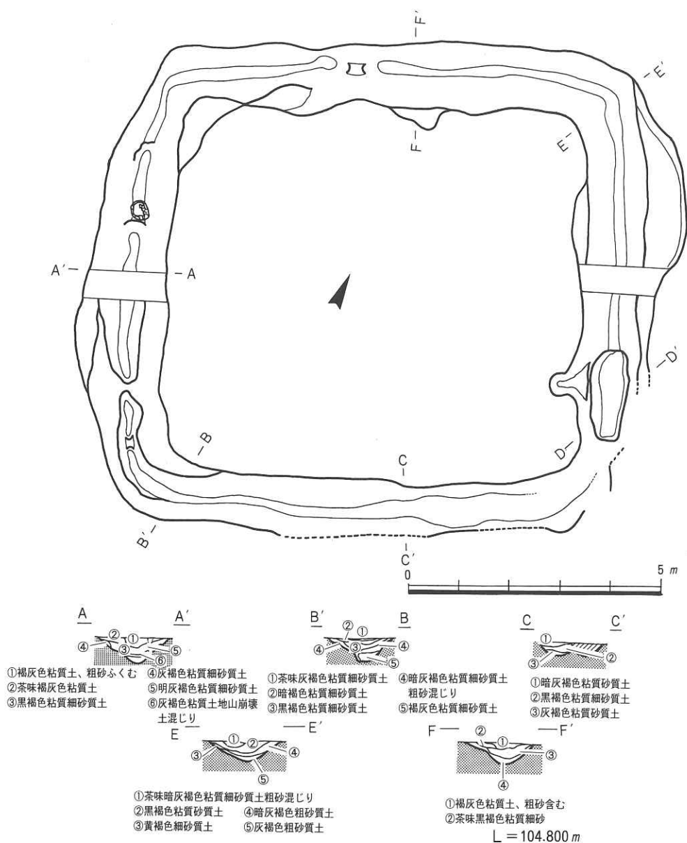
図10 SX101 遺構図
