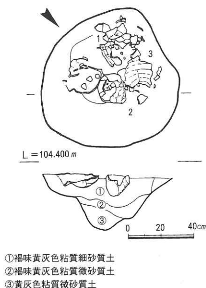
図6 SK105遺構図
