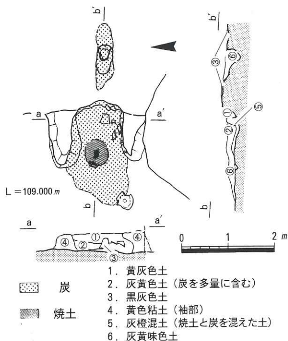
図5 SH-1、2 遺物出土状況及断面図
