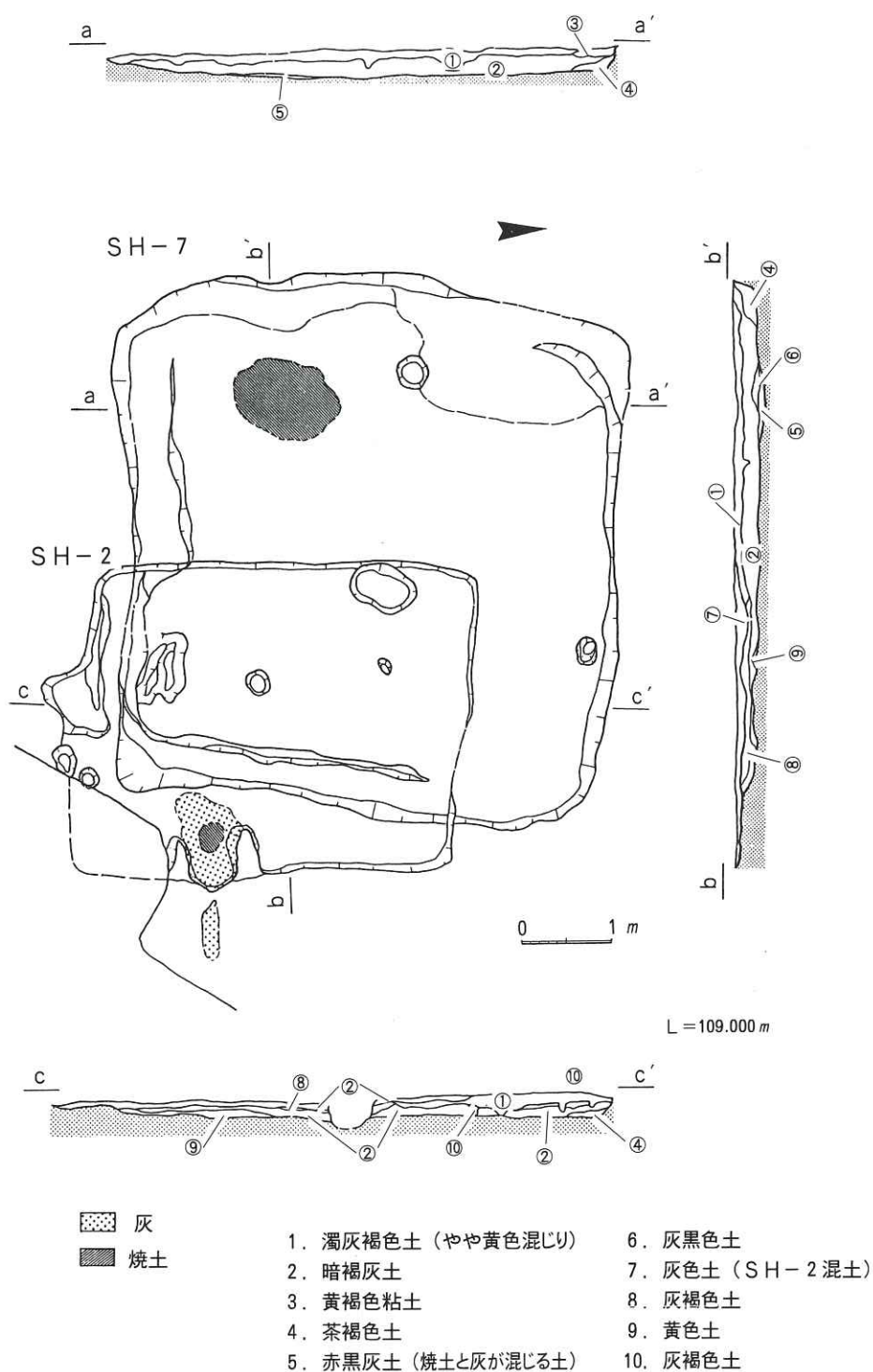
図14 SH-2,7 遺構図
