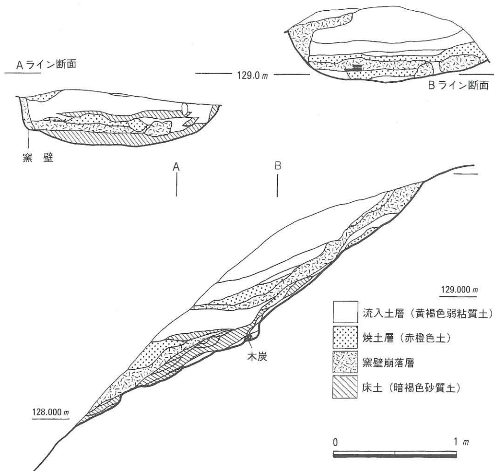
第5図 窯 断面図
