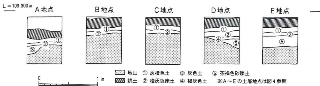
図3 調査区 北壁断面図
