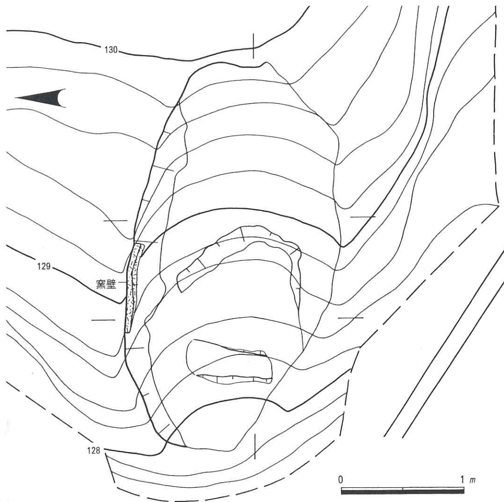
第4図 窯 平面図
