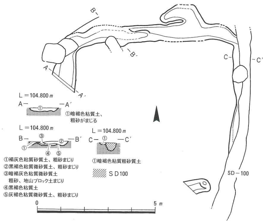
図22 SX105 遺構図
