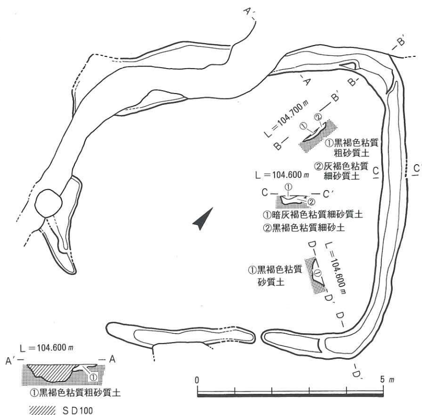
図20 SX103 遺構図
