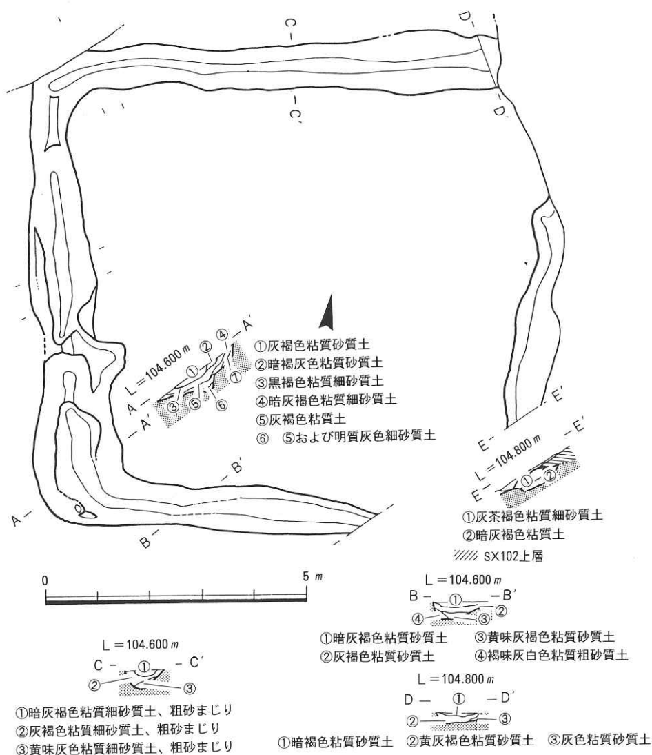
図9 SX100 遺構図
