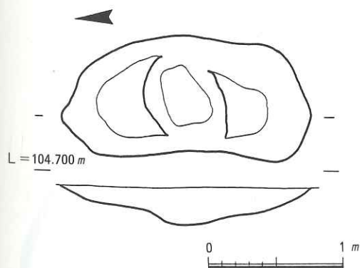
図5 SK103 遺構図
