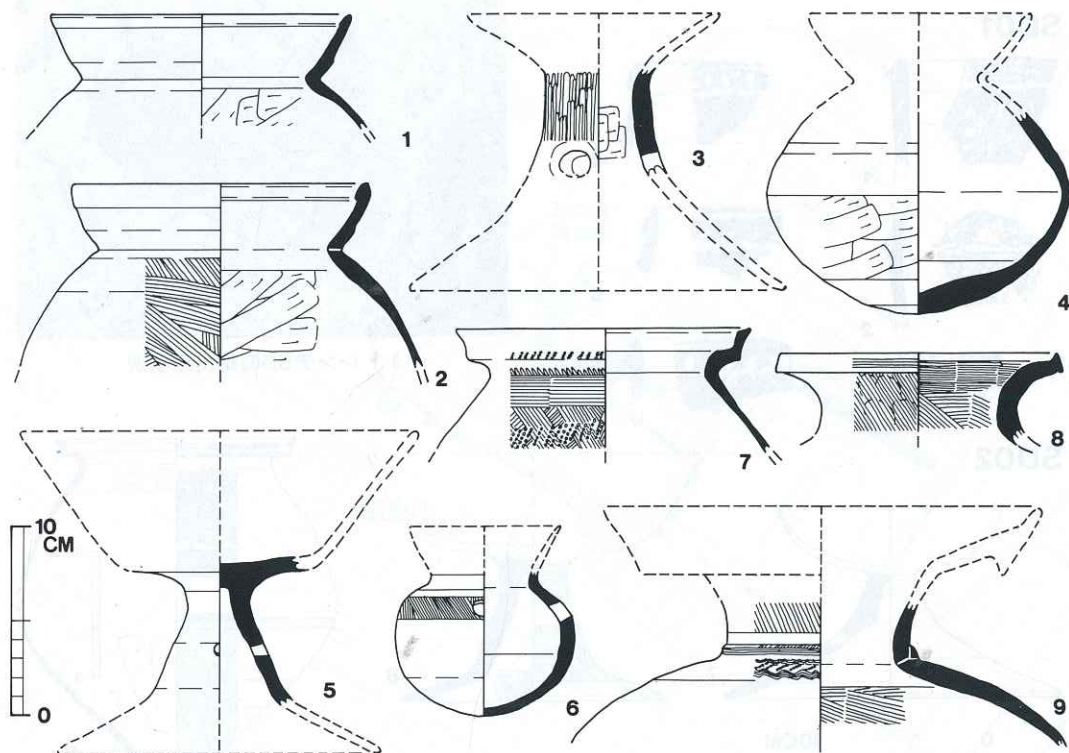
9 トレンチ SD03土器実測図
