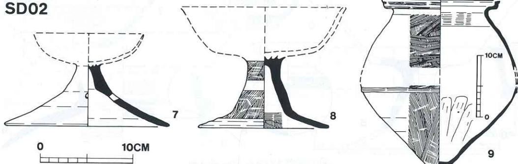
9 トレンチ SD01・SD02土器実測図
