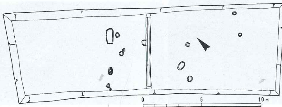
第1遺構面遺構図
