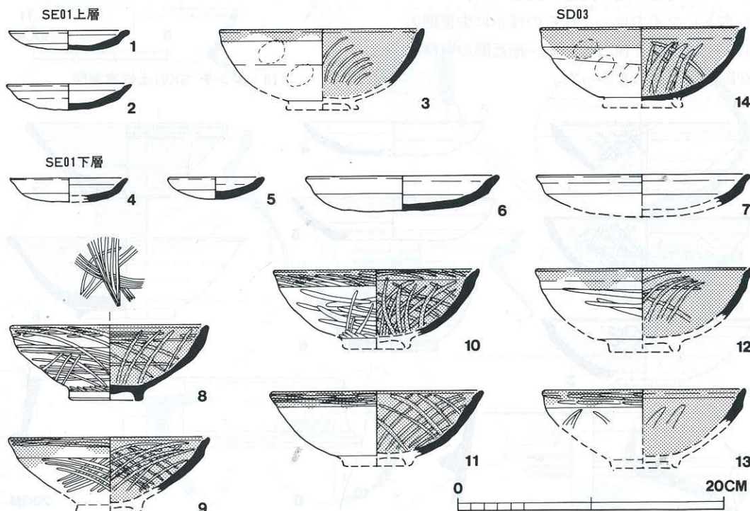
24-Sトレンチ 土器実測図
