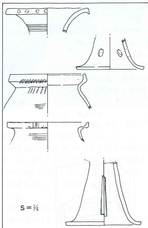
出土土器実測図
