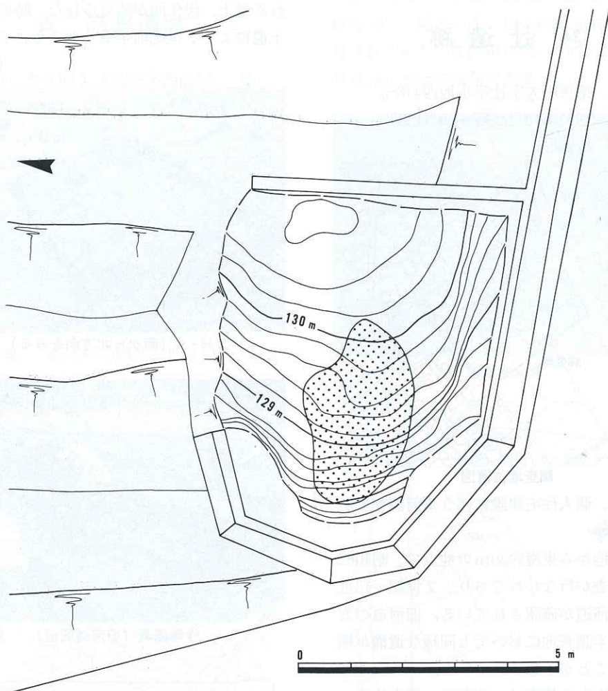
山田窯平面実測図
