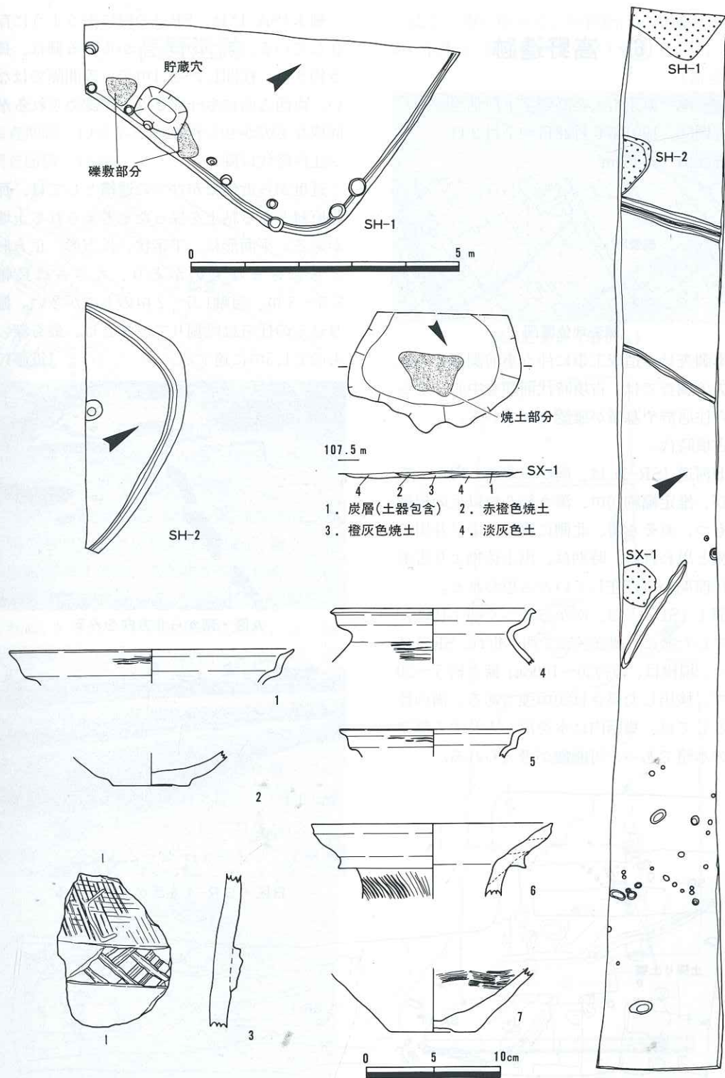
調査地遺構図 (S=1/400)
