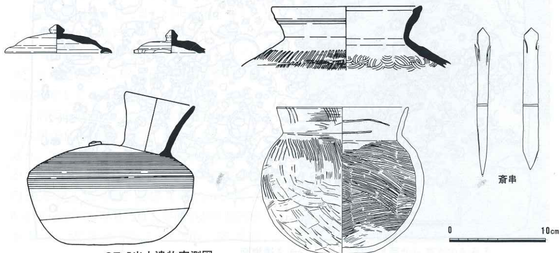
SE-7出土遺物実測図
