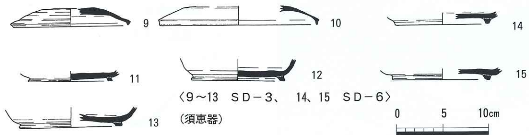
出土遺物実測図
