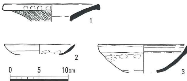
出土遺物実測図
