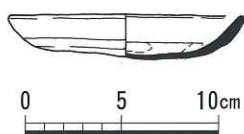
出土土師器実測図
