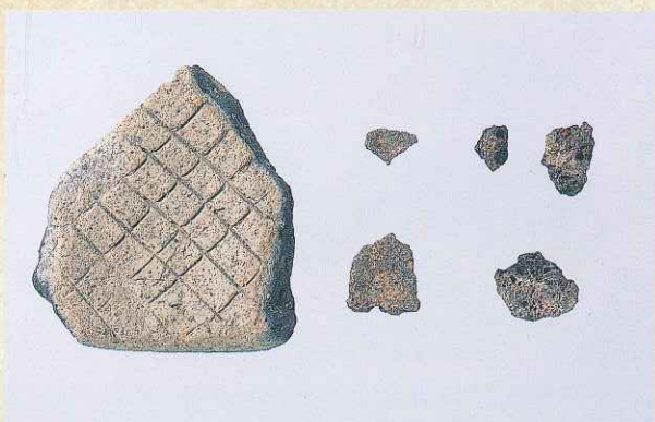
▲土製鑄型・残滓
