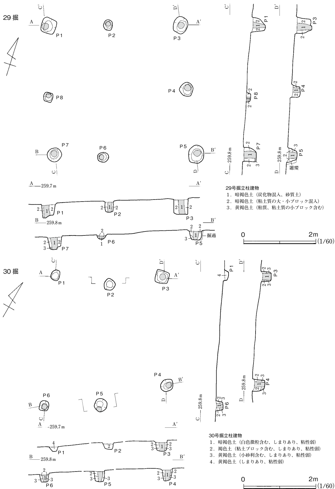
第23図 29・30号掘立柱建物
