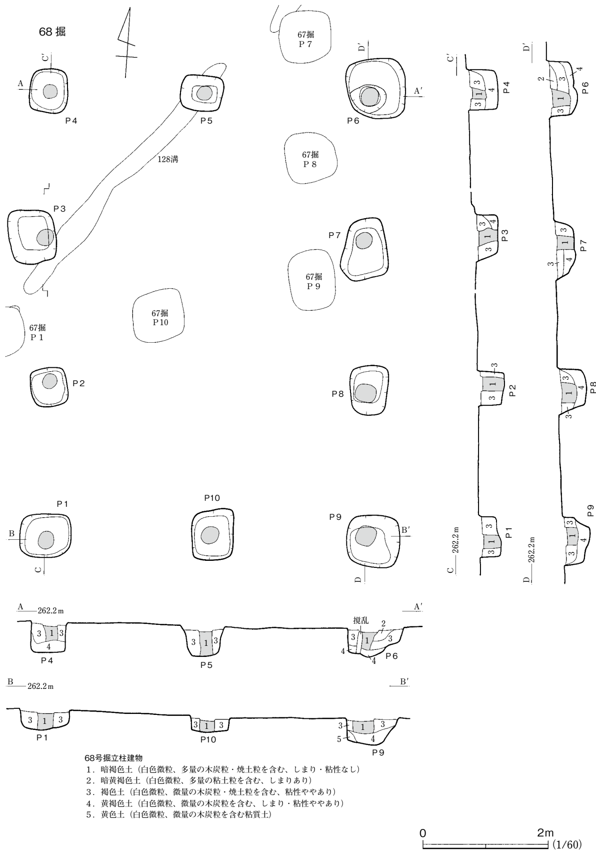
第59図 68号掘立柱建物
