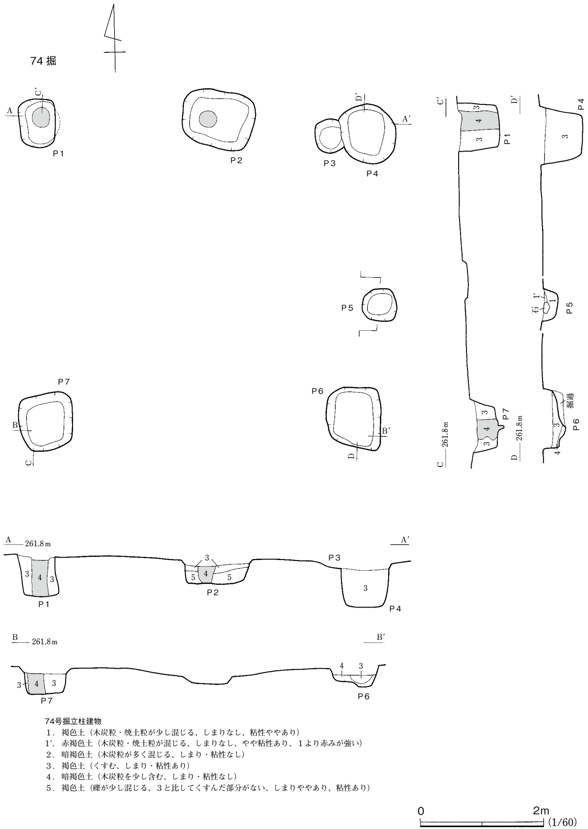
第65図 74号掘立柱建物
