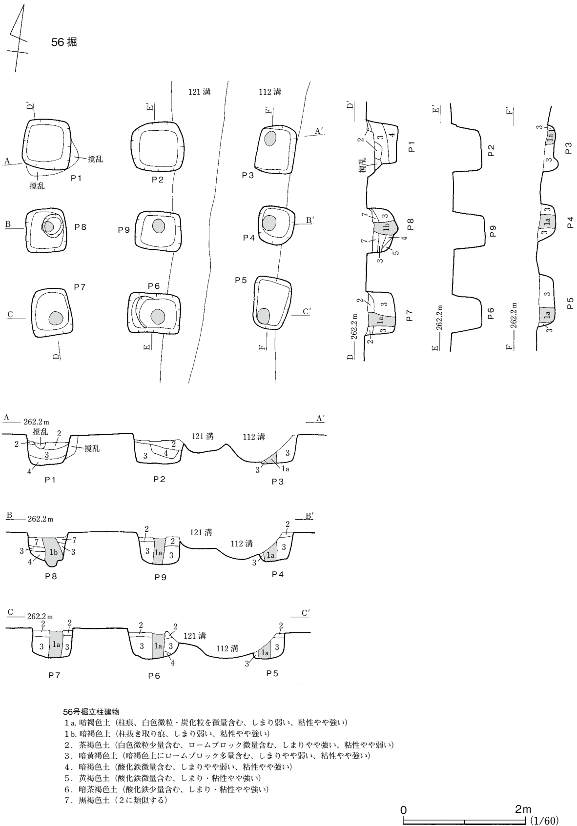
第47図 56号掘立柱建物
