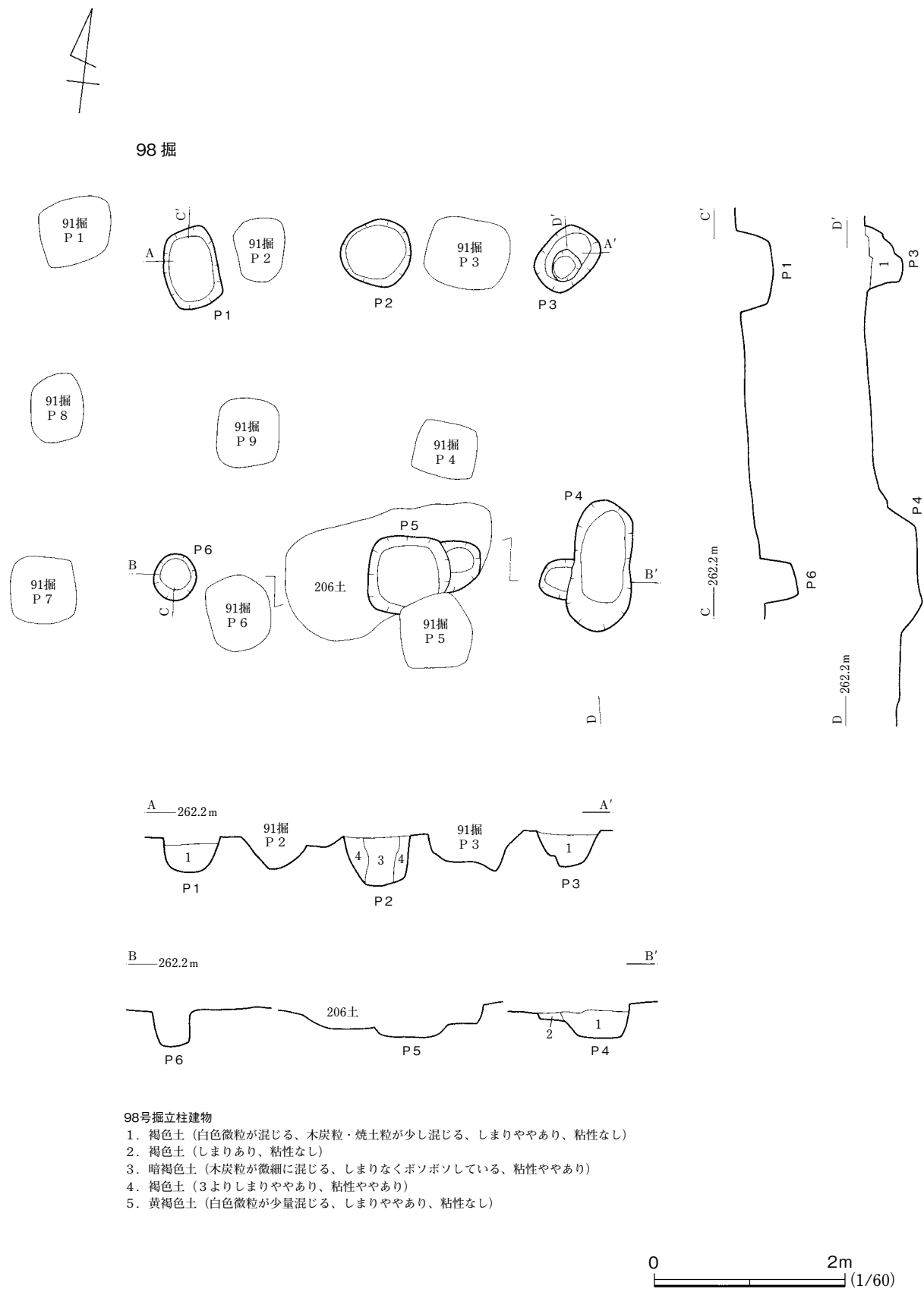
第91図 98号掘立柱建物
