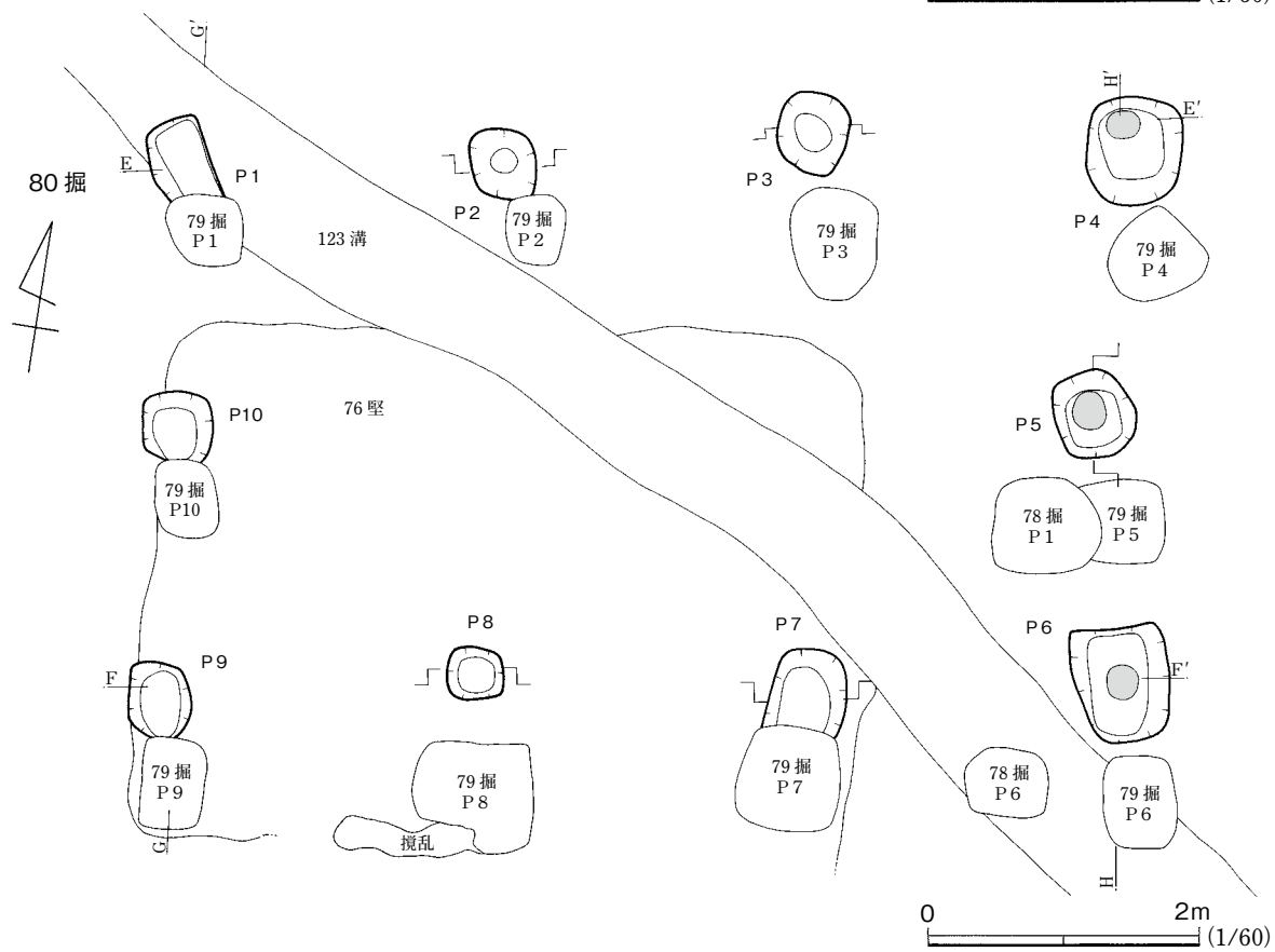
第70図 79・80号掘立柱建物 (1)
