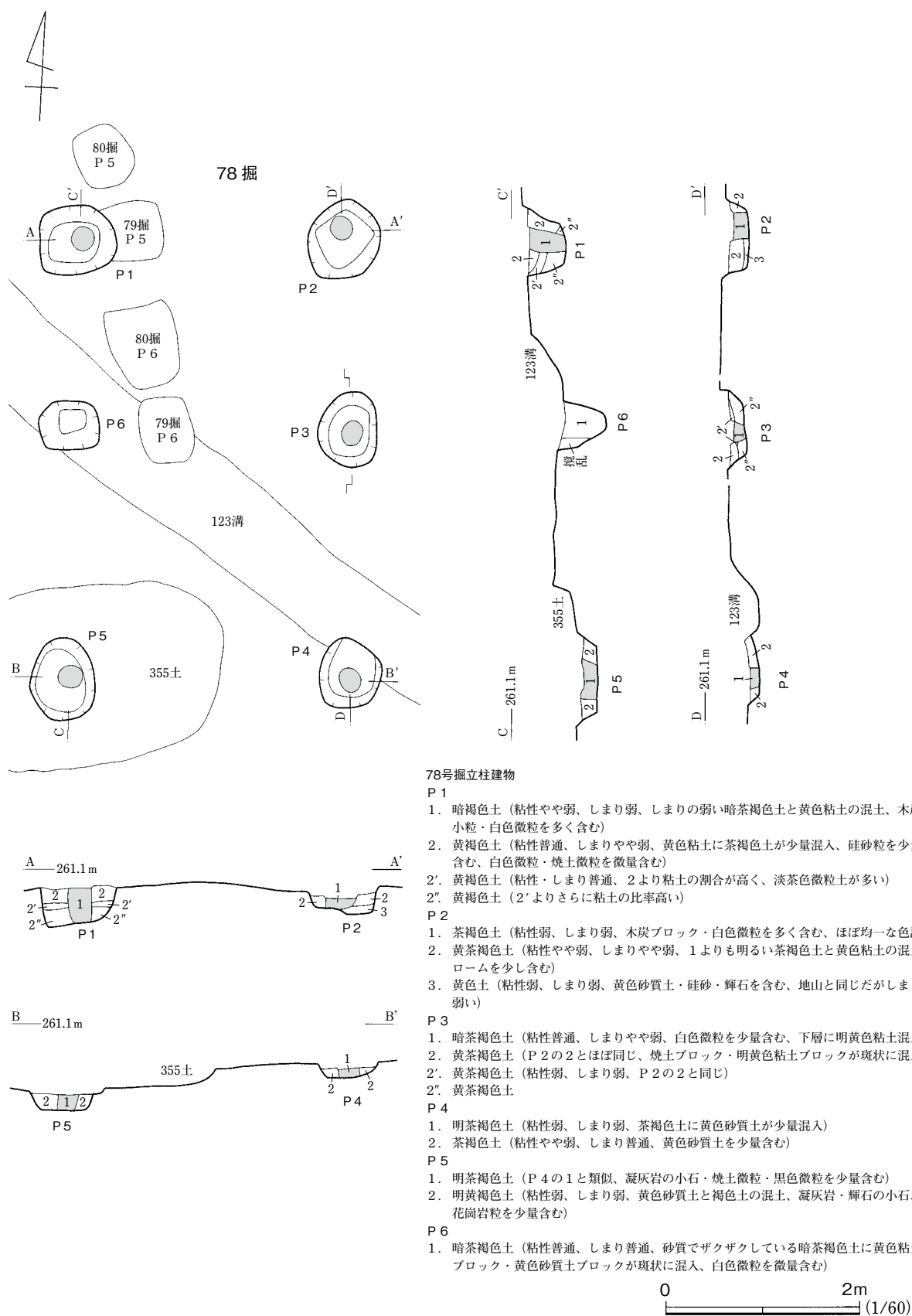
第69図 78号掘立柱建物
