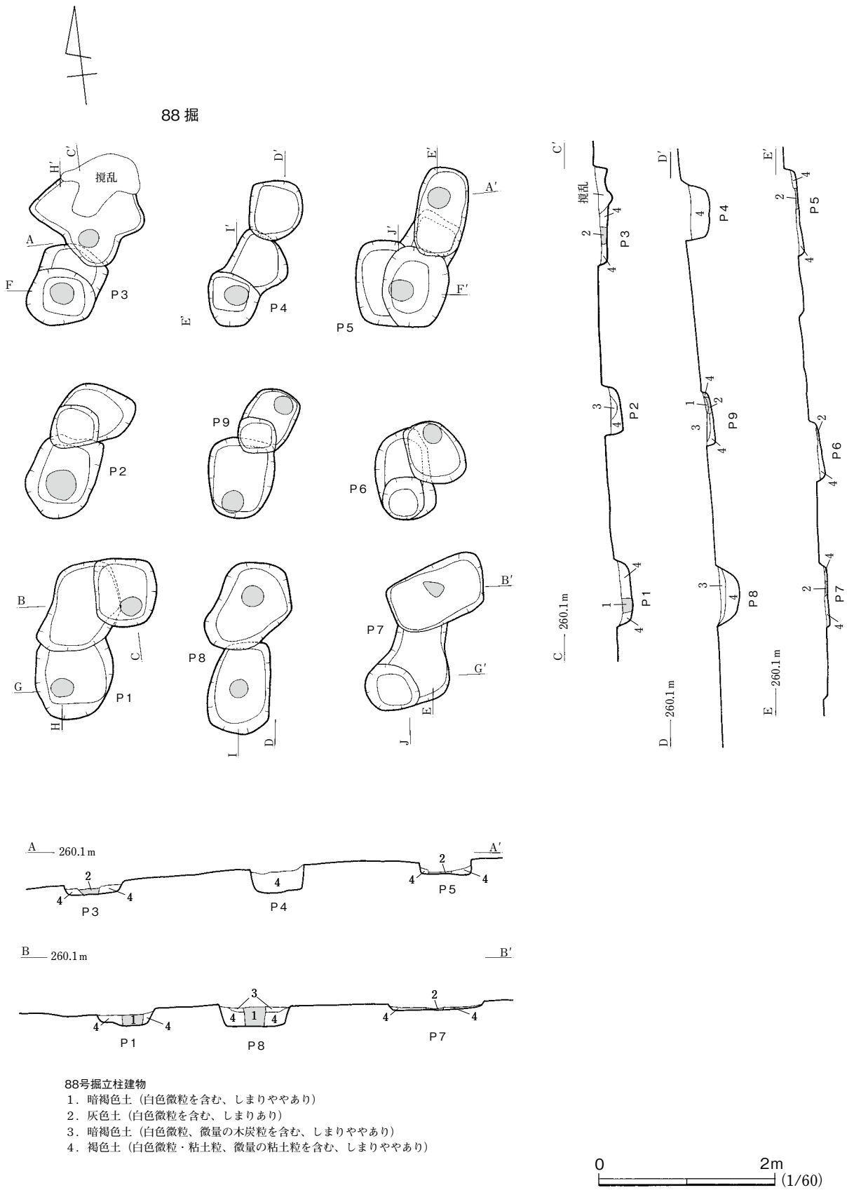
第79図 88号掘立柱建物 (1)
