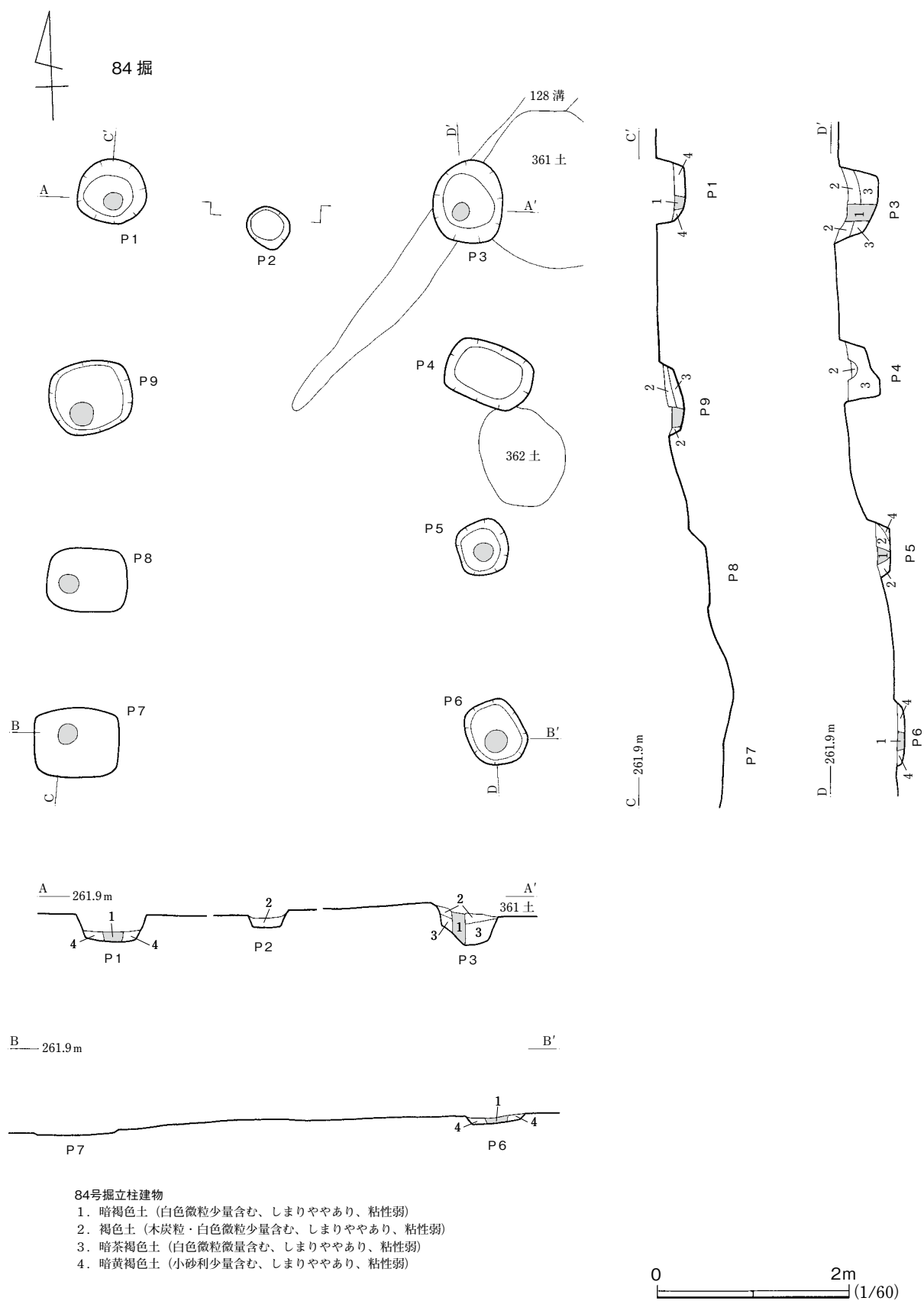
第76図 84号掘立柱建物
