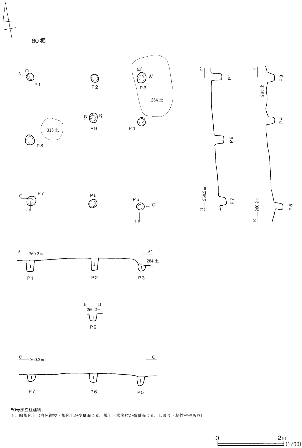
第51図 60号掘立柱建物
