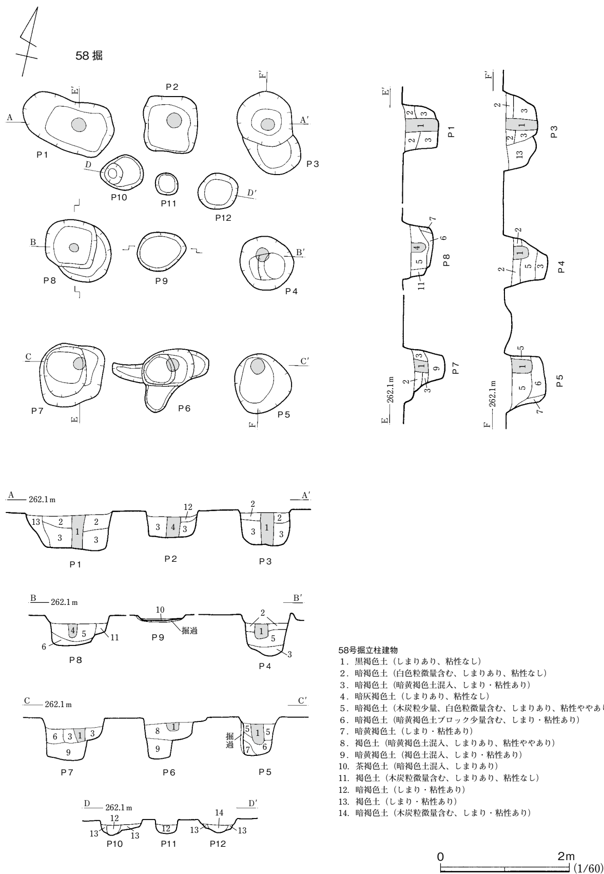
第49図 58号掘立柱建物
