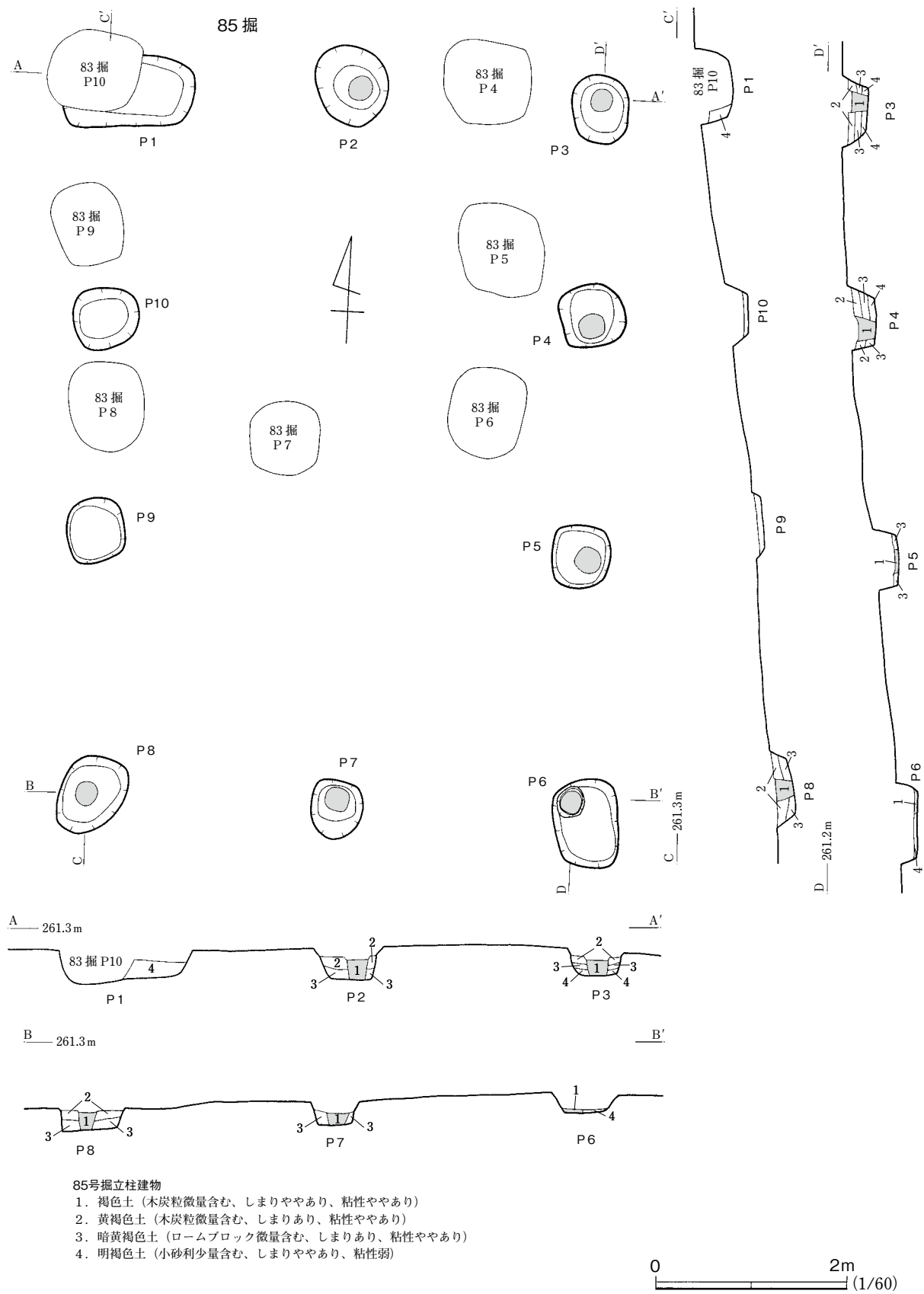
第77図 85号掘立柱建物
