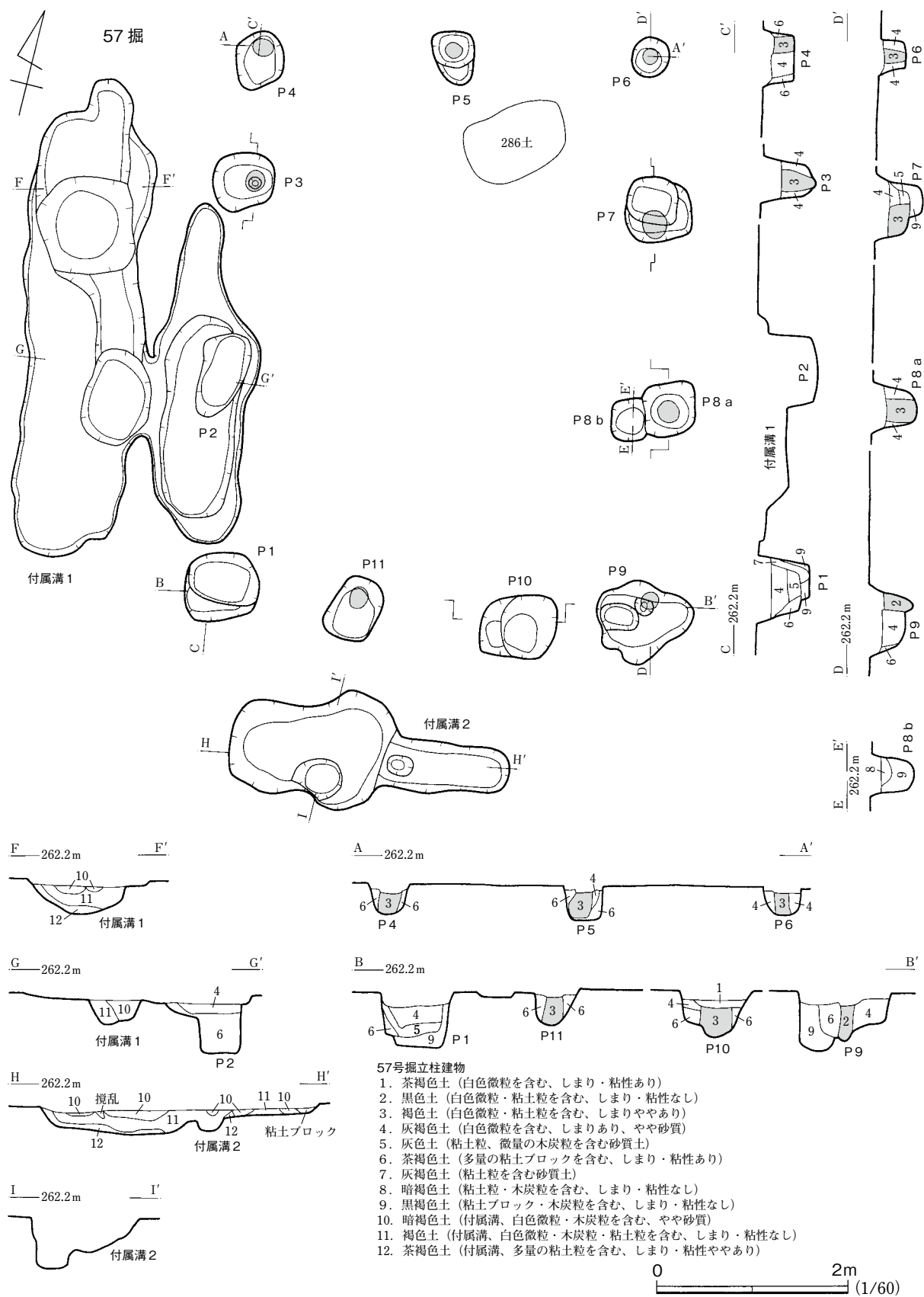
第48図 57号掘立柱建物
