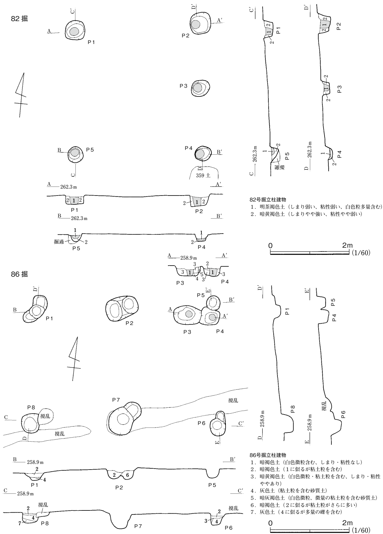
第74図 82・86号掘立柱建物
