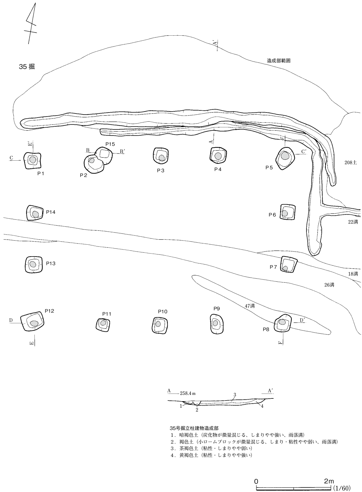
第27図 35号掘立柱建物 (1)
