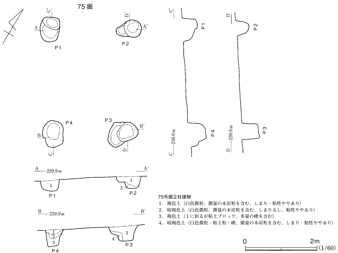
第64図 73・75号掘立柱建物
