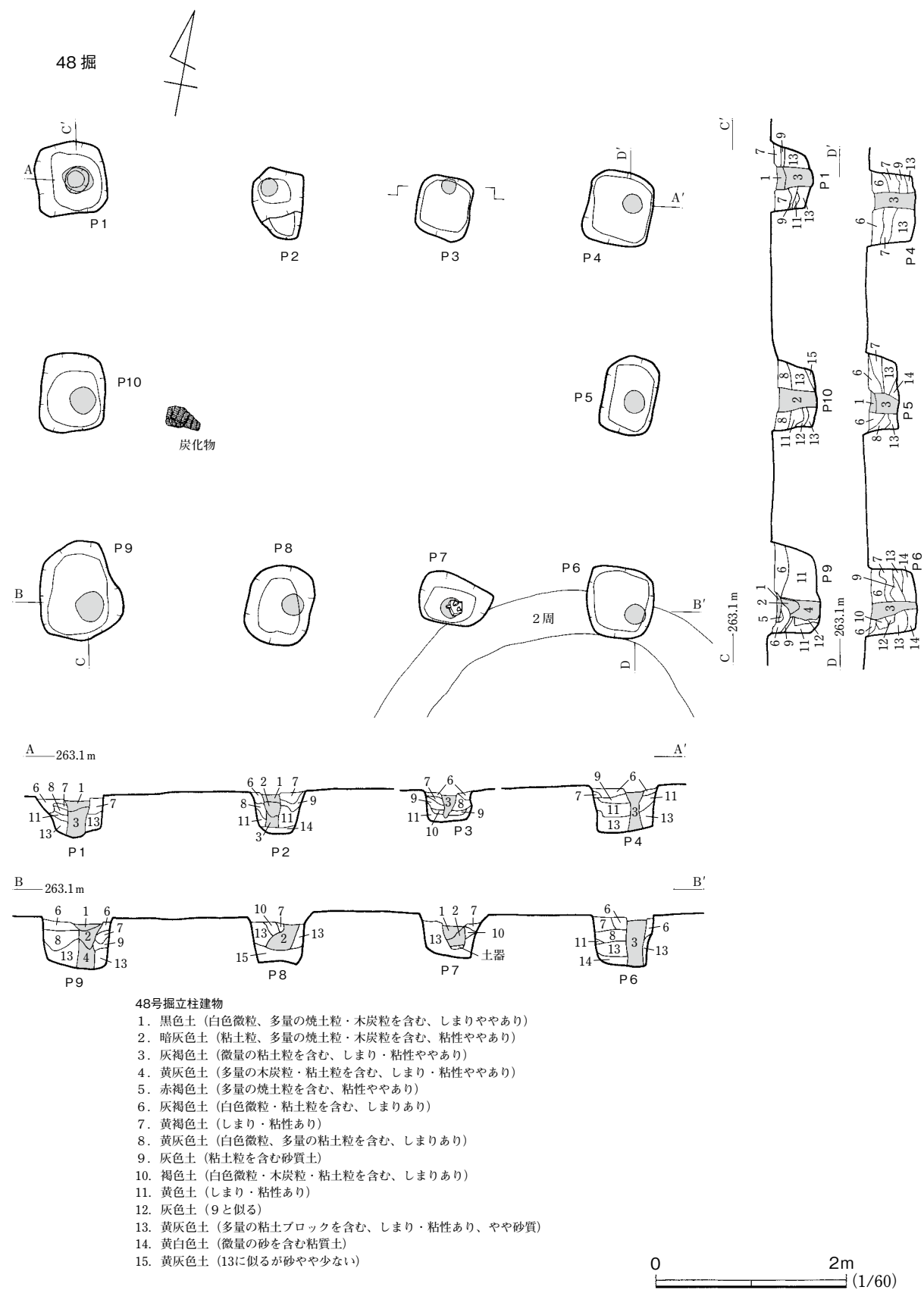
第40図 48号掘立柱建物
