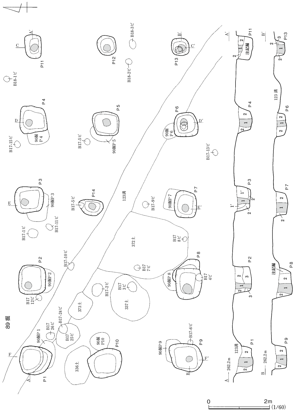
第81図 89号掘立柱建物 (1)
