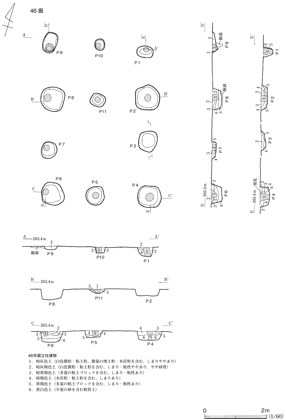
第37図 46号掘立柱建物
