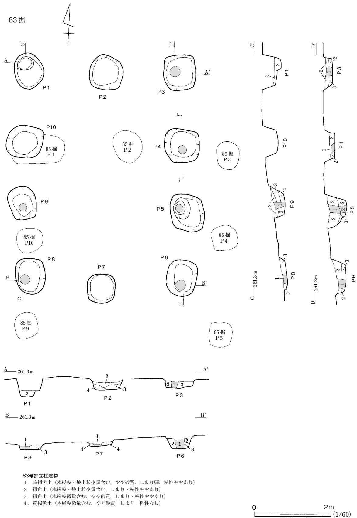
第75図 83号掘立柱建物
