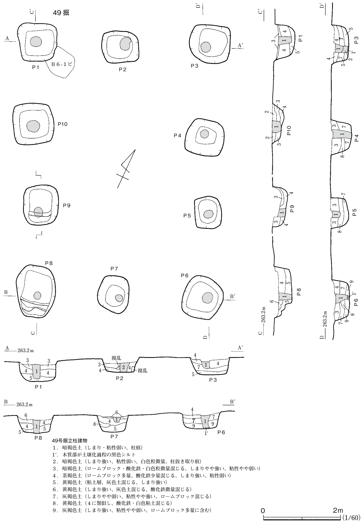
第41図 49号掘立柱建物
