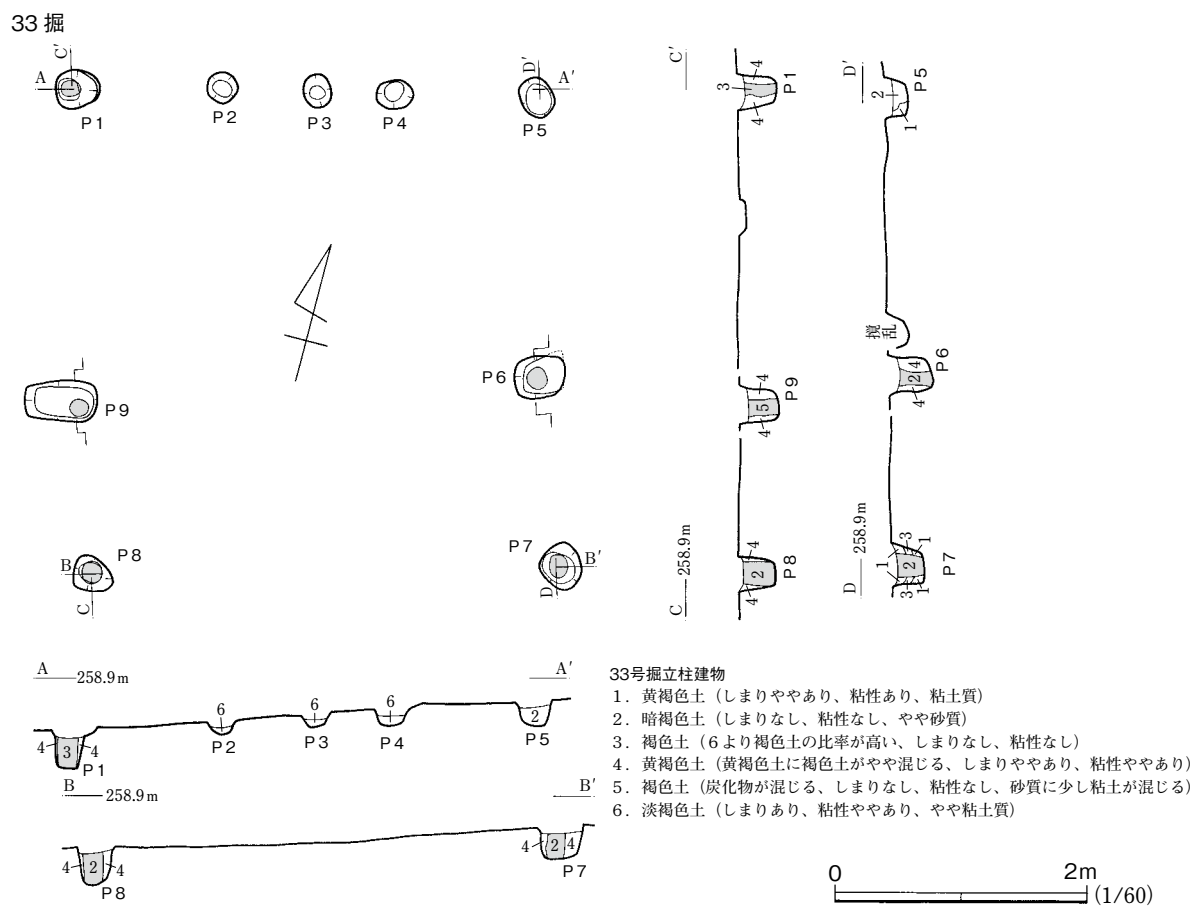
第24図 31・33号掘立柱建物
