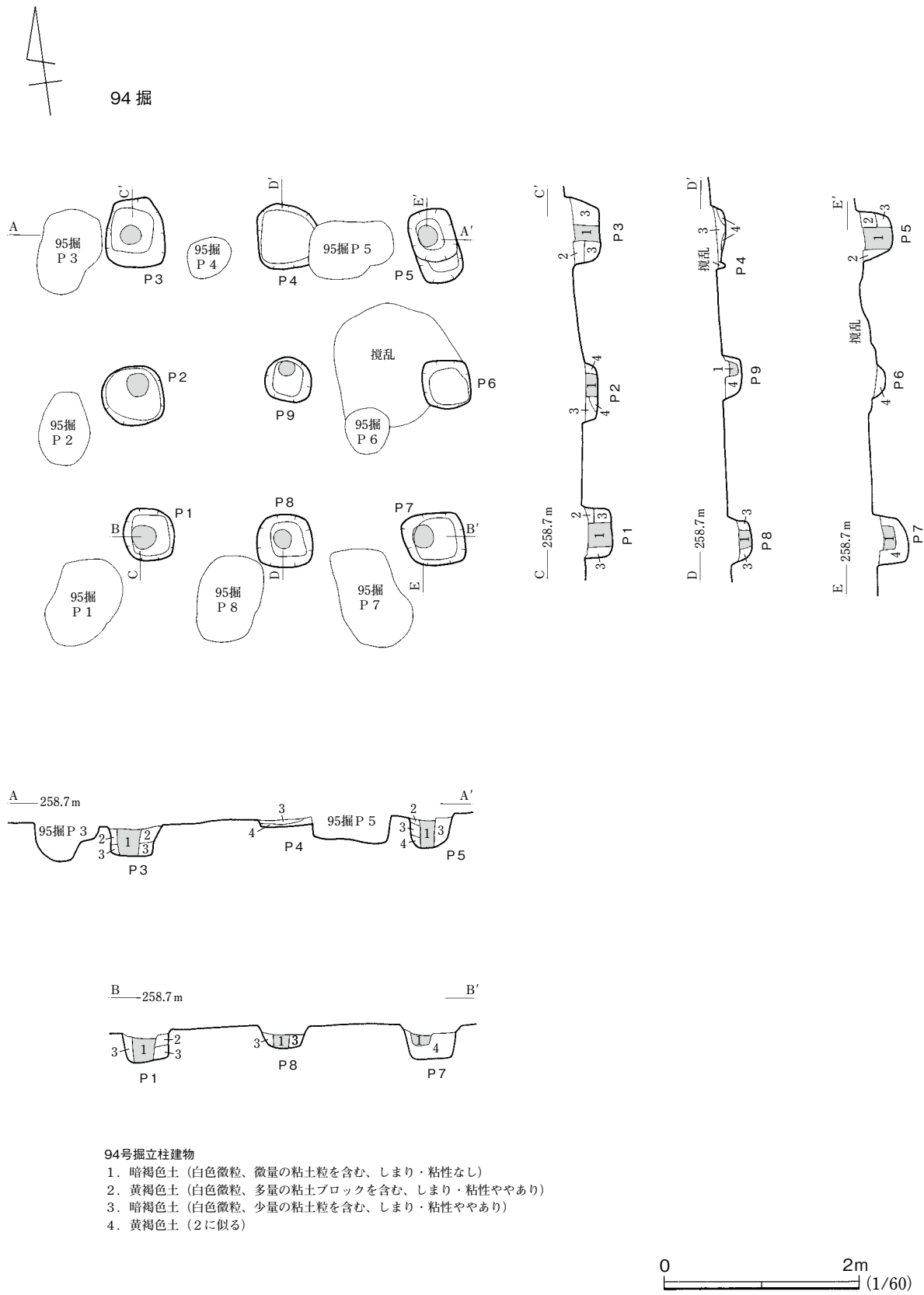
第87図 94号掘立柱建物
