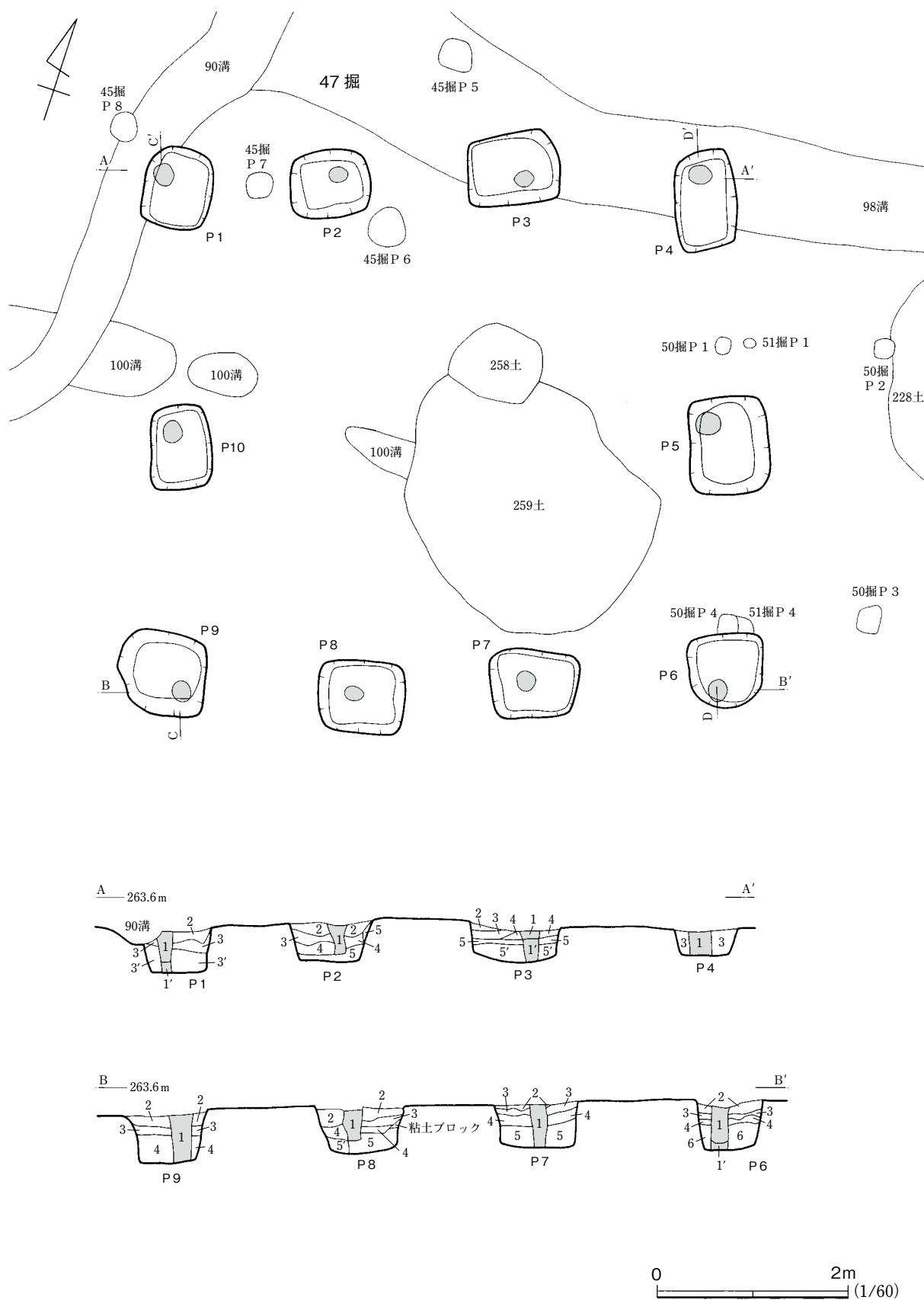
第38図 47号掘立柱建物 (1)
