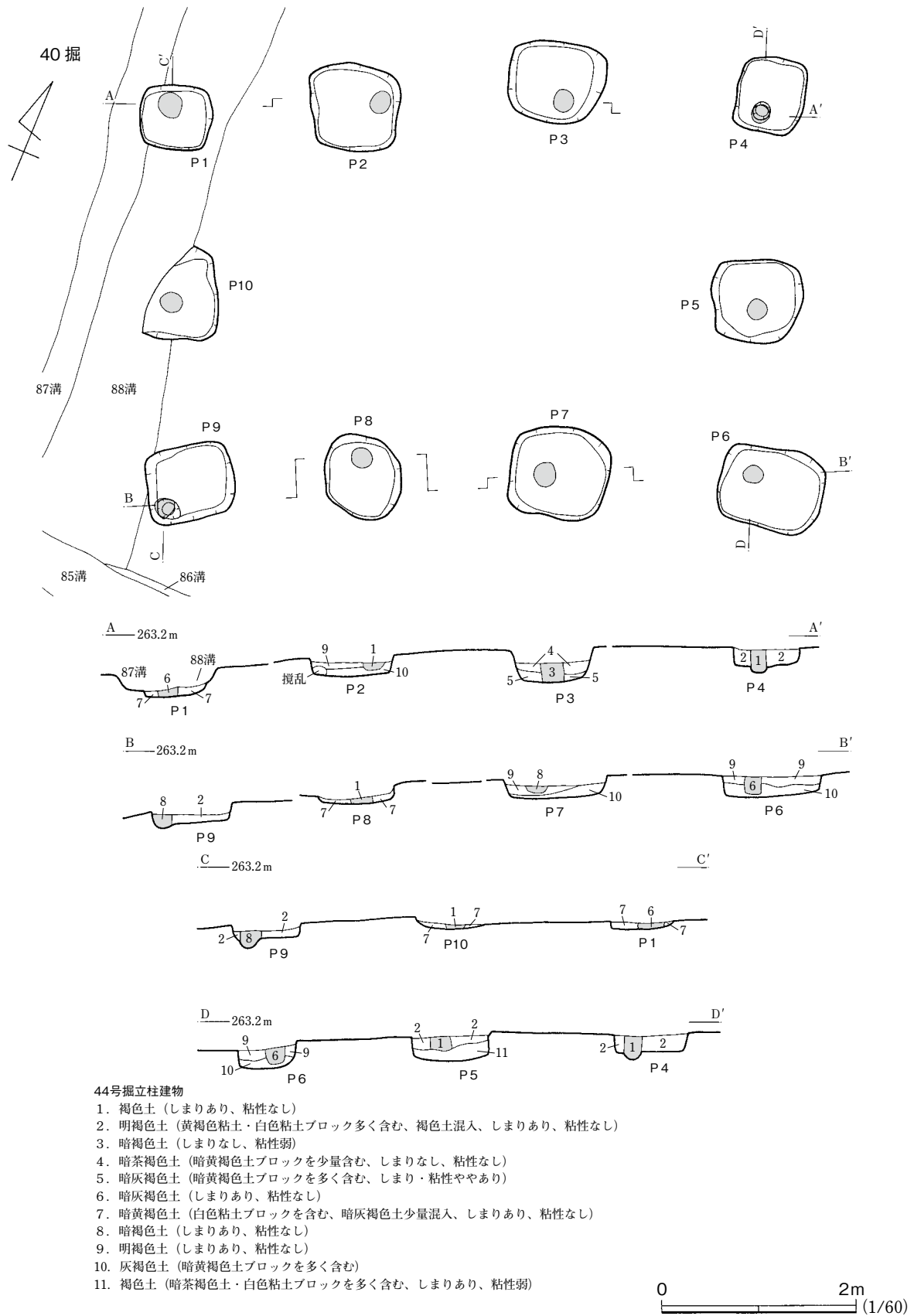
第35図 44号掘立柱建物
