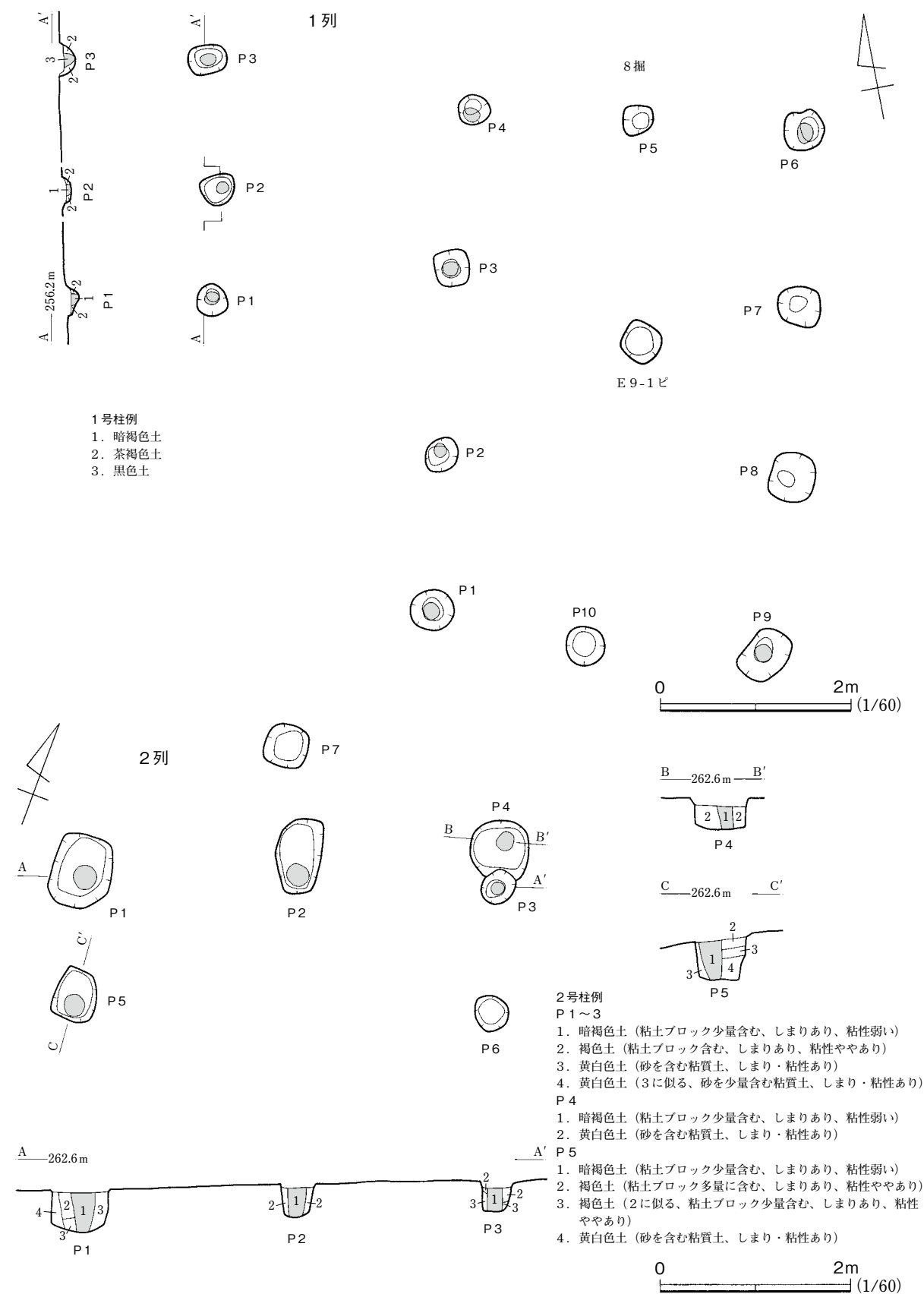
第96図 1・2号柱列
