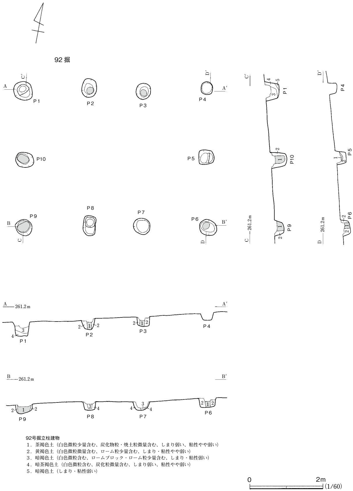
第85図 92号掘立柱建物
