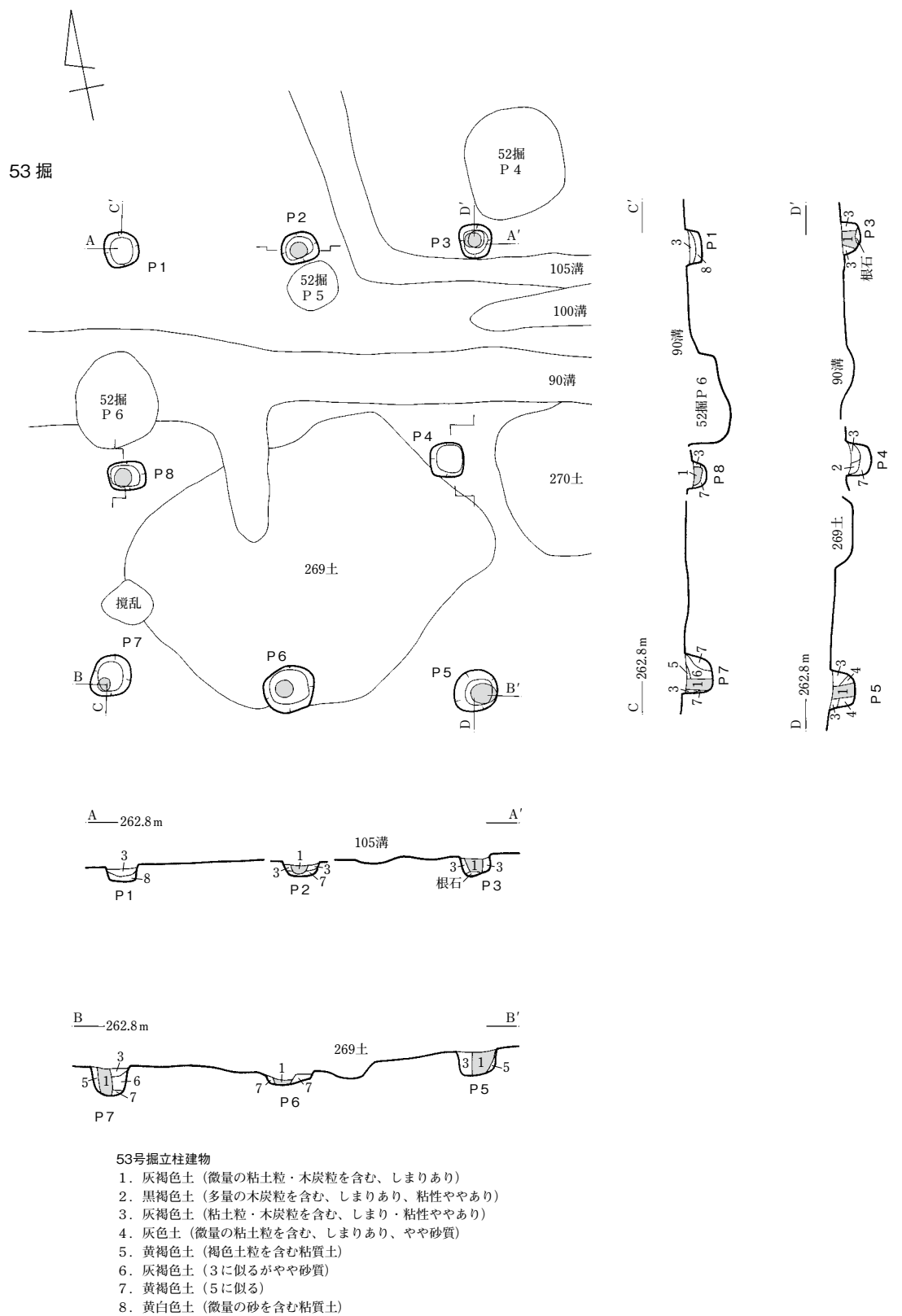
第44図 53号掘立柱建物
