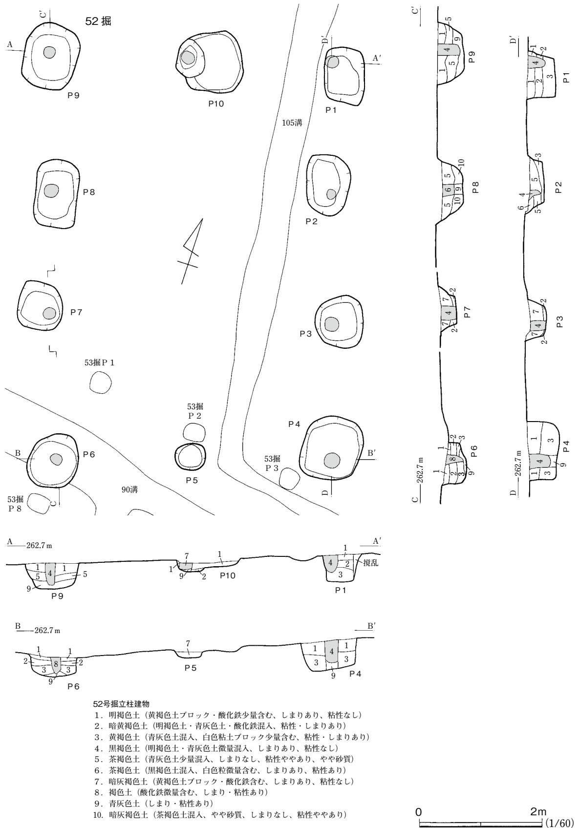
第43図 52号掘立柱建物
