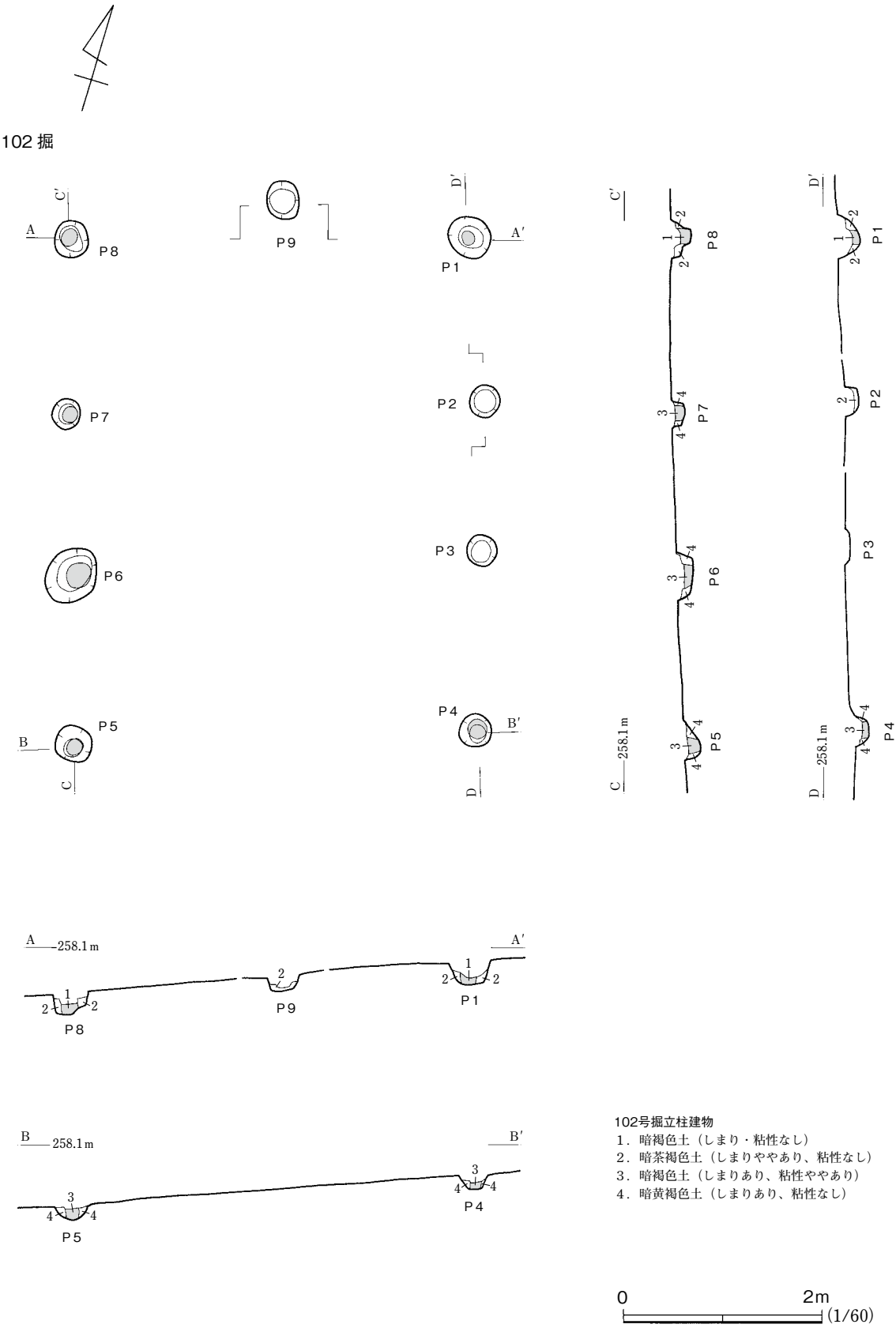
第95図 102号掘立柱建物
