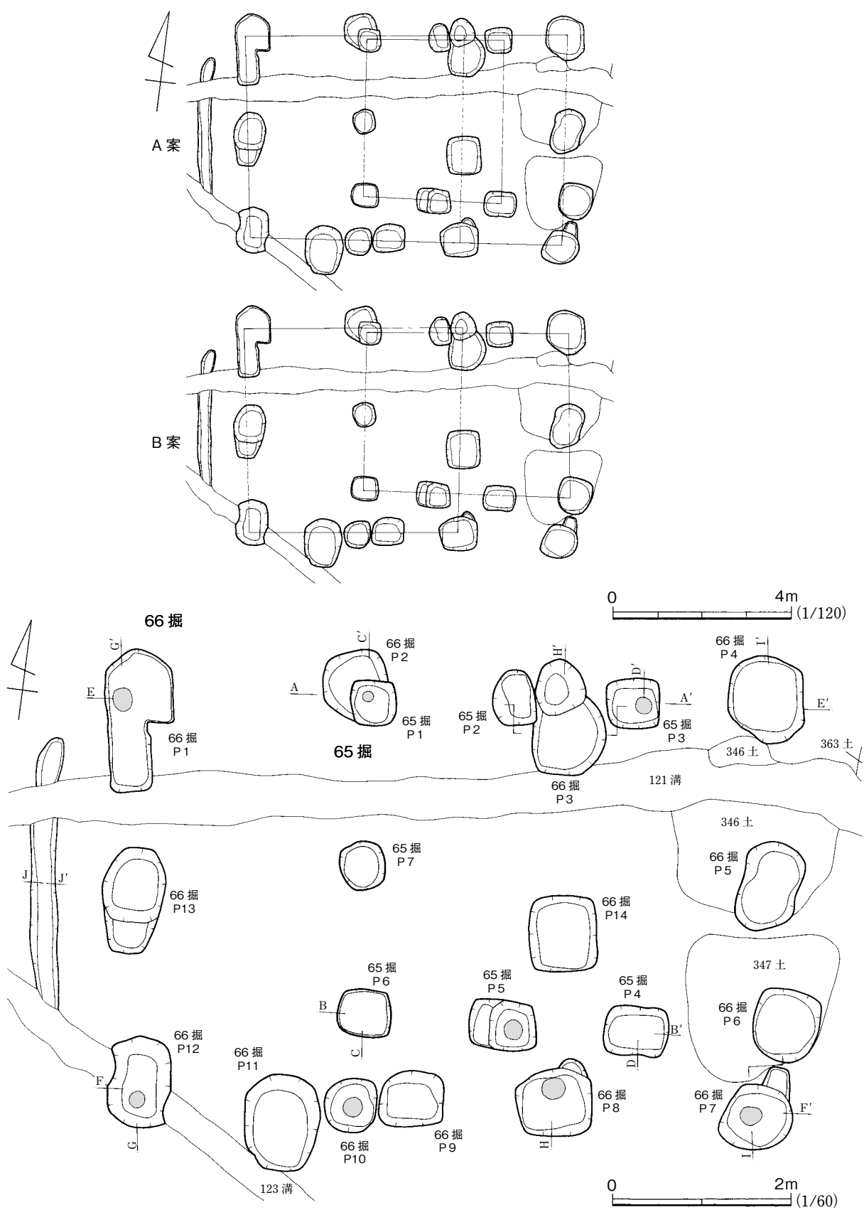
第56図 65・66号掘立柱建物 (1)
