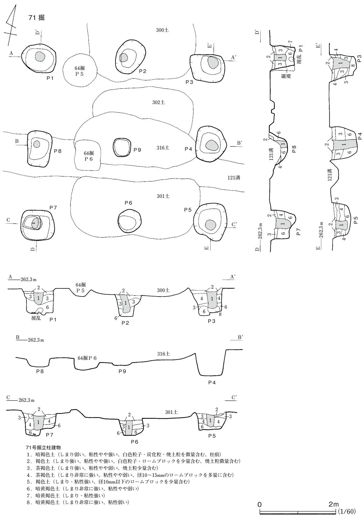
第62図 71号掘立柱建物
