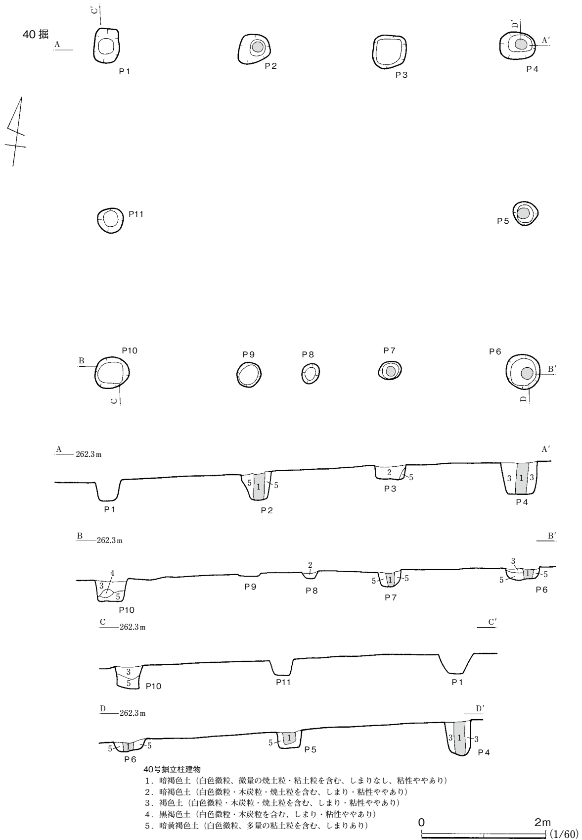
第31図 40号掘立柱建物
