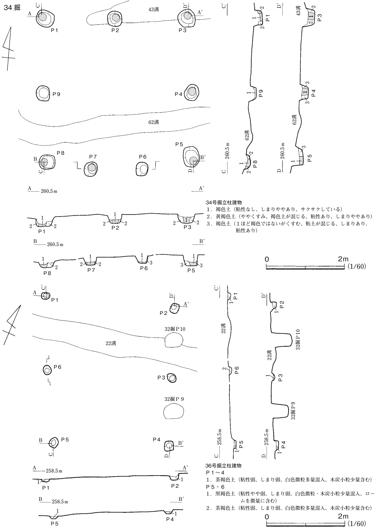
第26図 34・36号掘立柱建物
