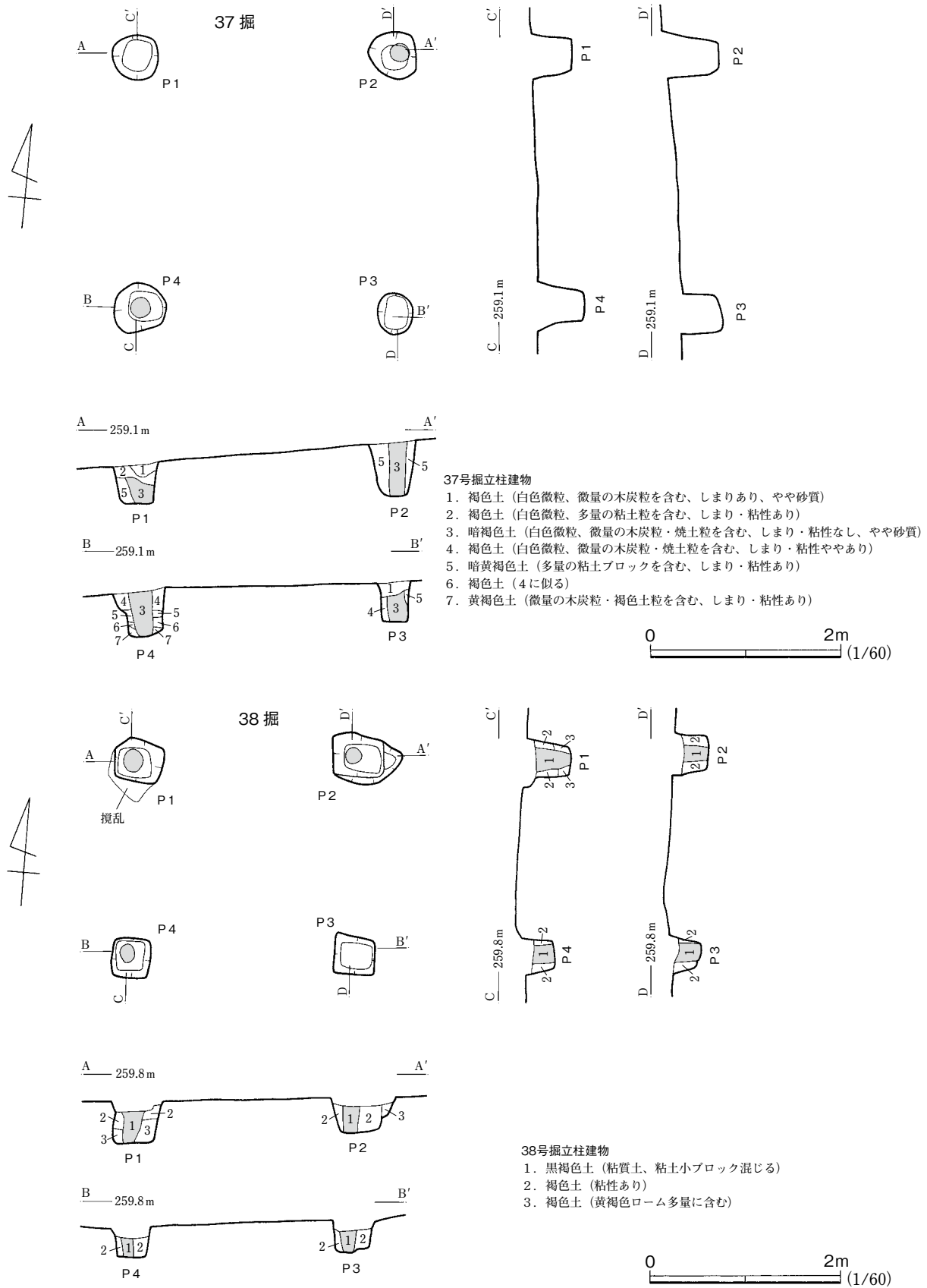
第29図 37・38号掘立柱建物
