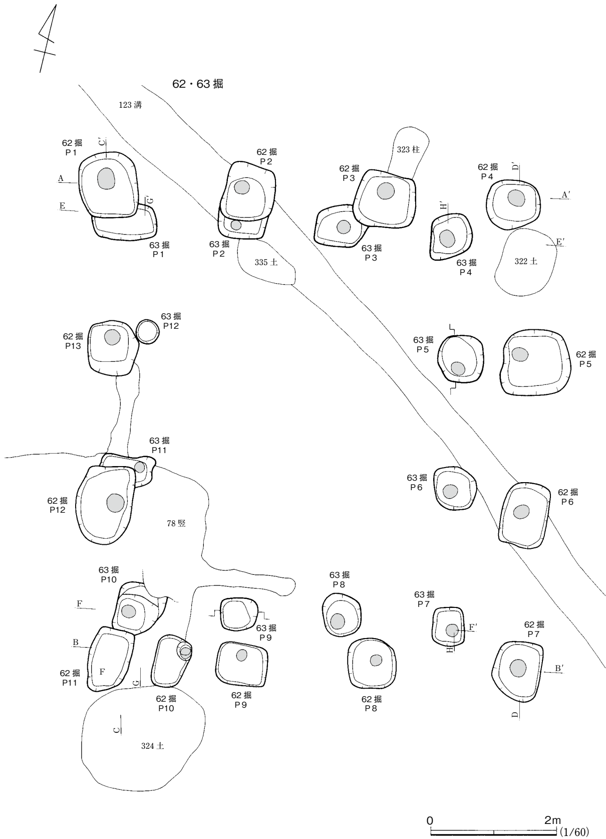
第53図 62・63号掘立柱建物 (1)
