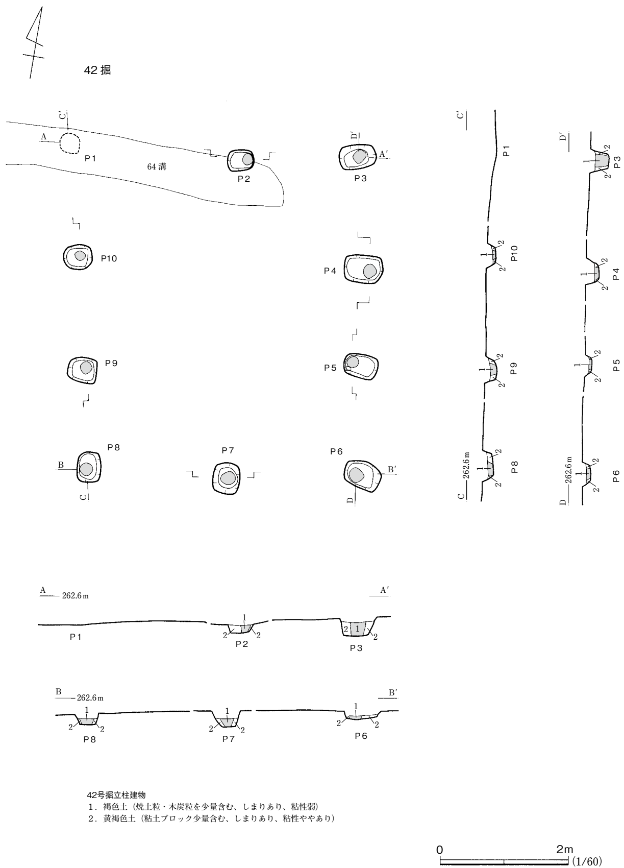
第33図 42号掘立柱建物
