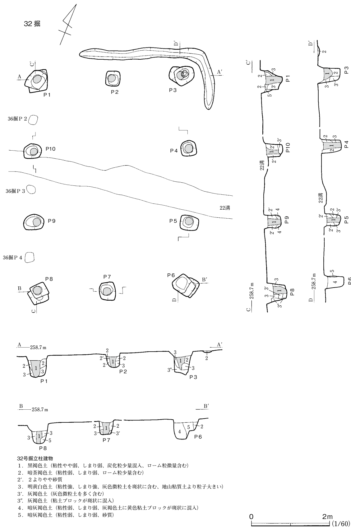
第25図 32号掘立柱建物
