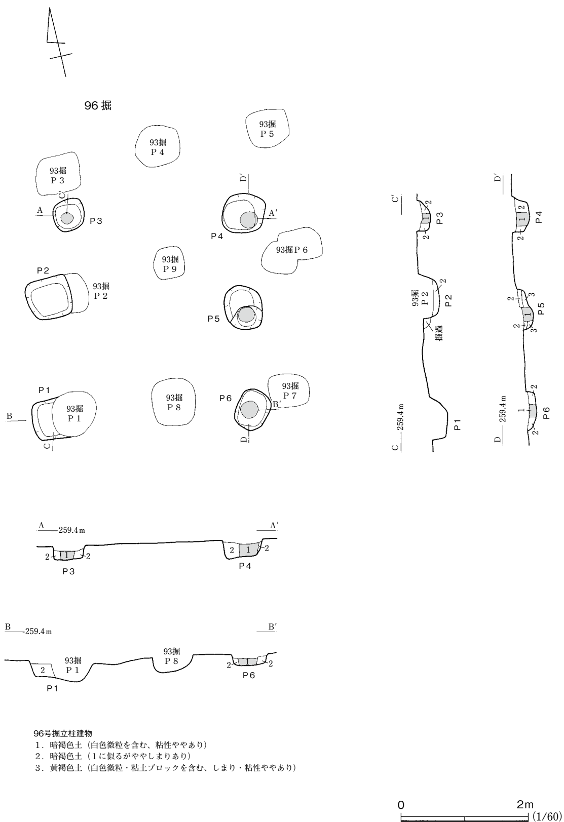
第89図 96号掘立柱建物
