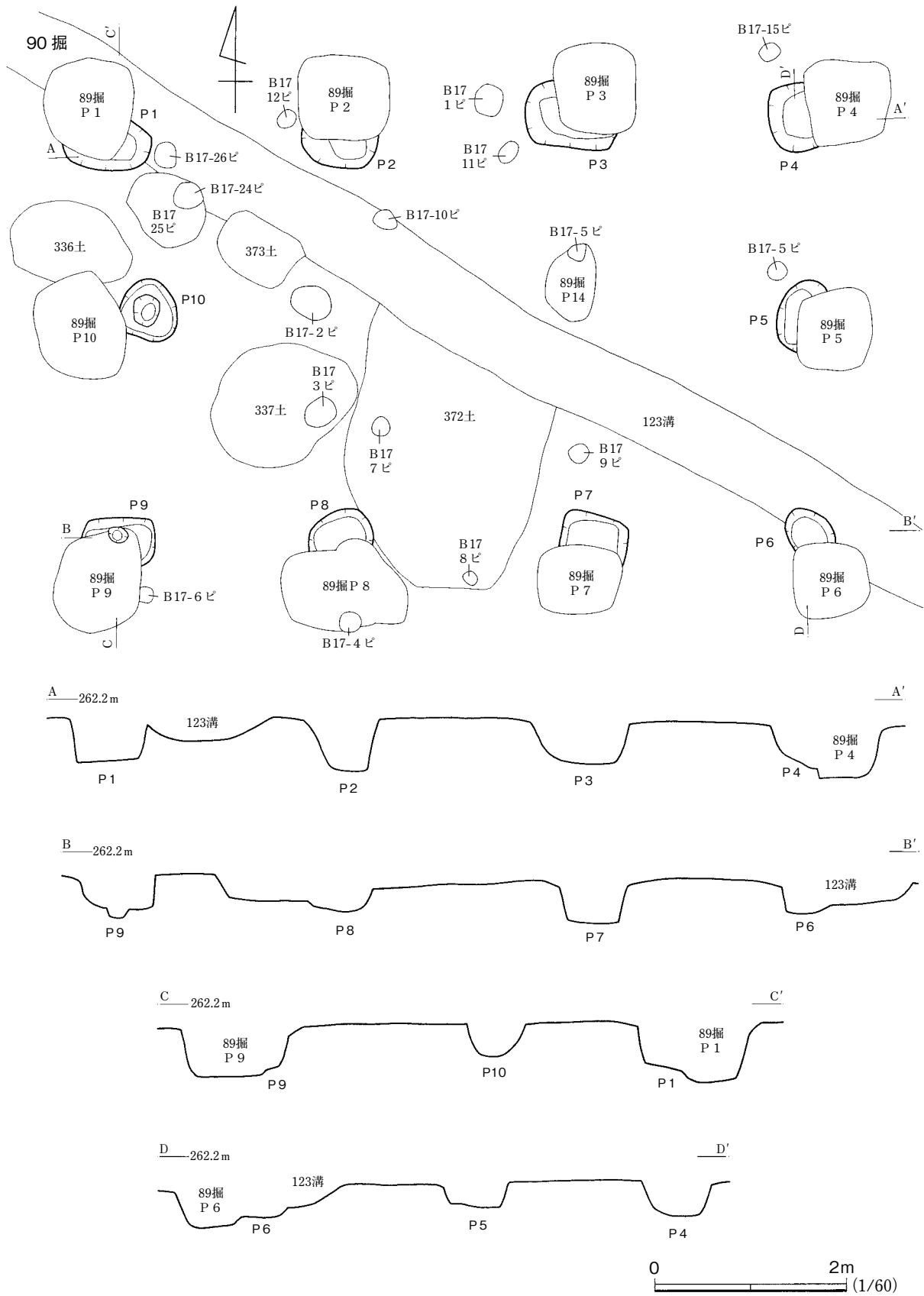
第83図 90号掘立柱建物
