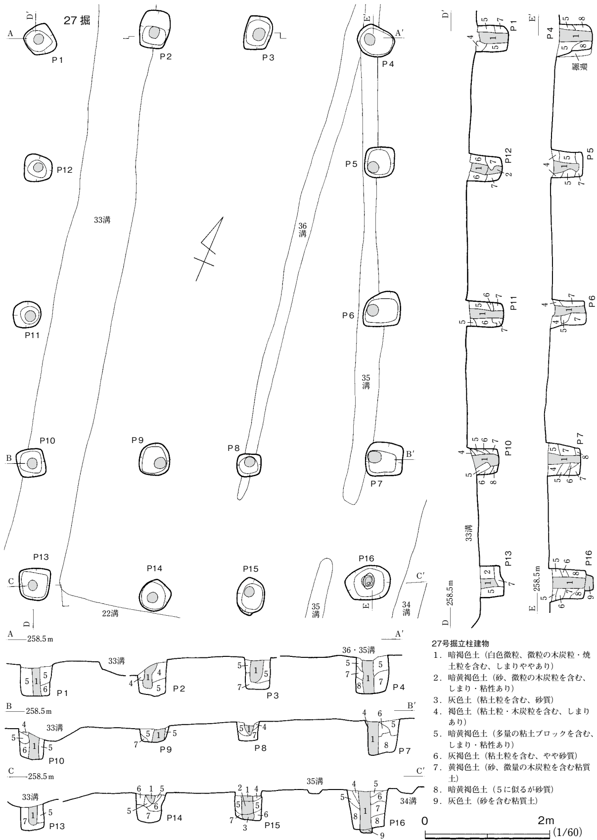
第21図 27号掘立柱建物
