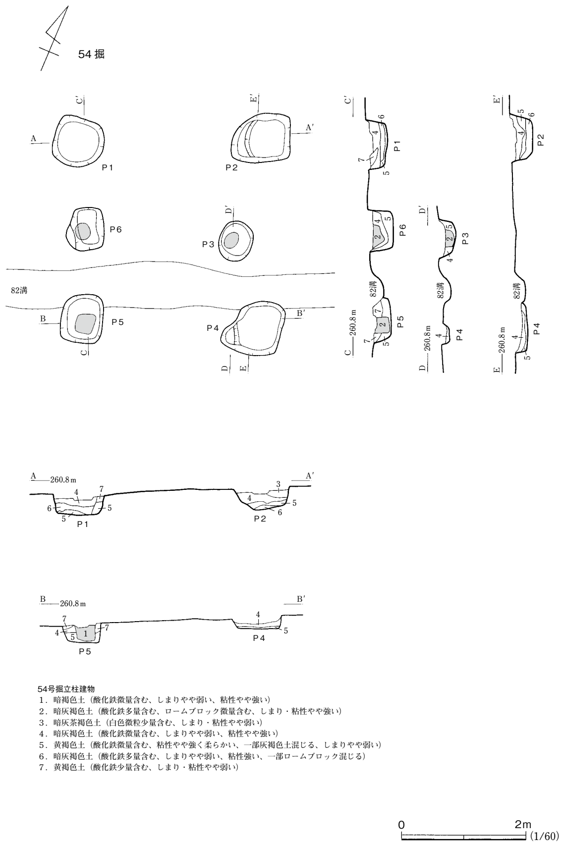
第45図 54号掘立柱建物
