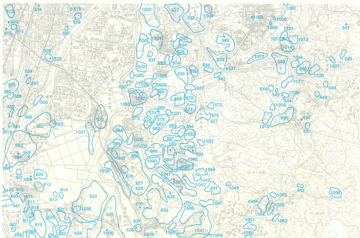
第1図 周辺地形図
