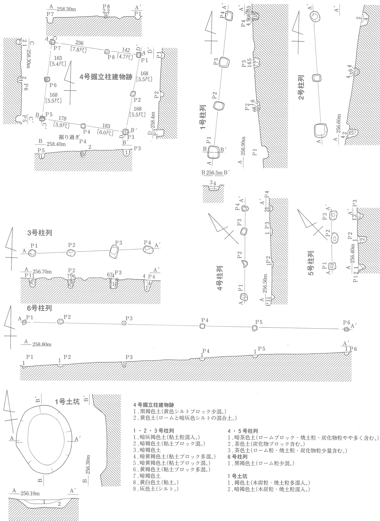
第6図 4号掘立柱建物跡・1～6号柱列・1号土坑
