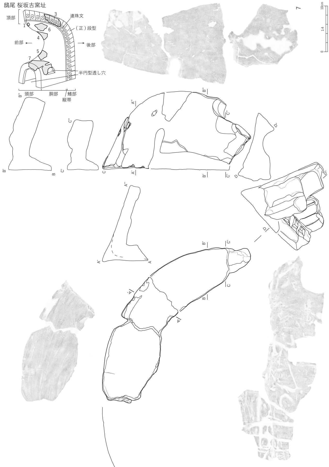
第210図 鷗尾 桜坂古窯址
