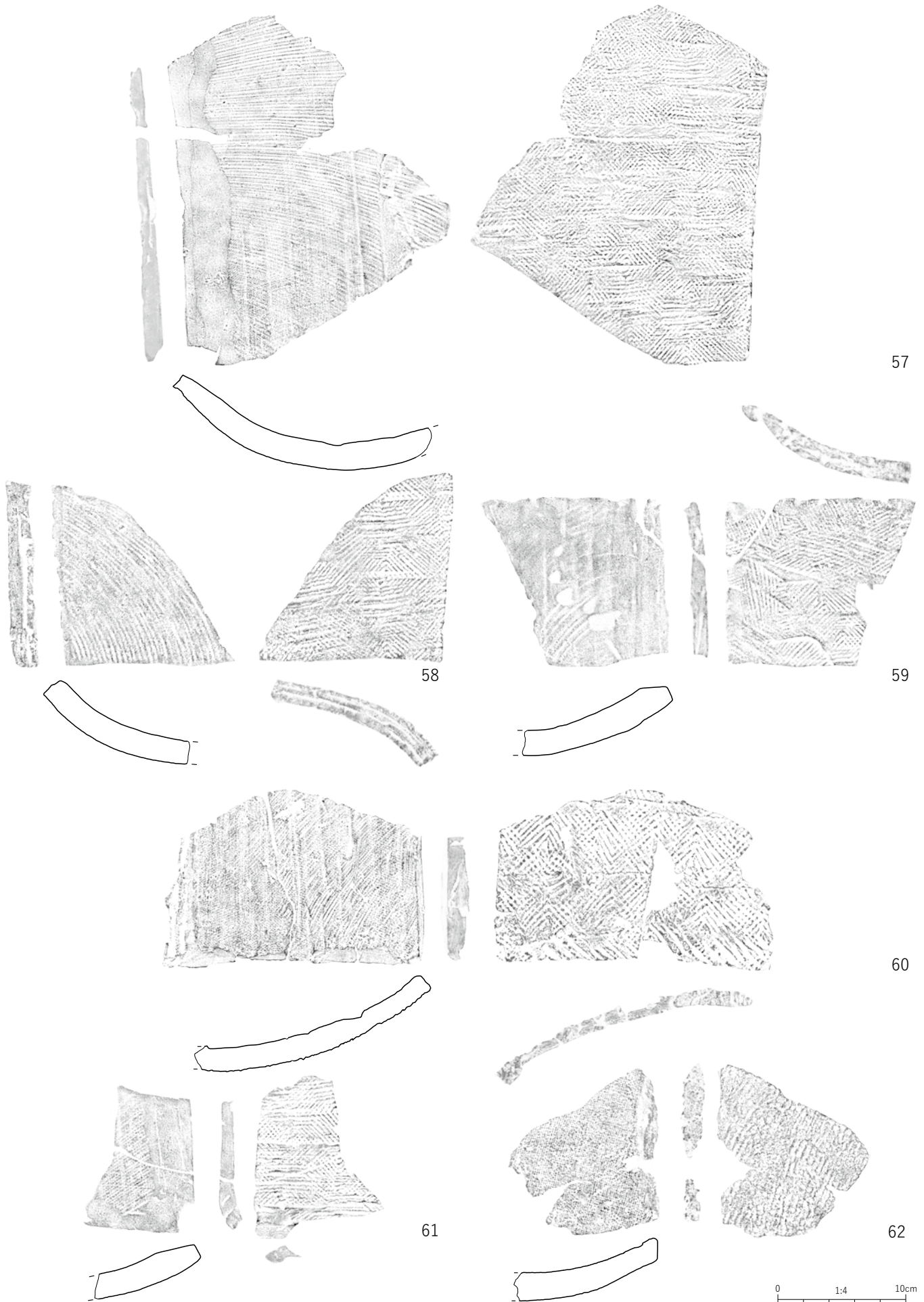
第180図 平瓦 粘土板桶巻づくりⅡ②類
