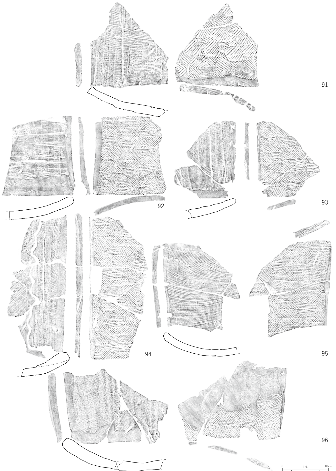
第189図 平瓦 粘土板桶巻づくりⅡ③類
