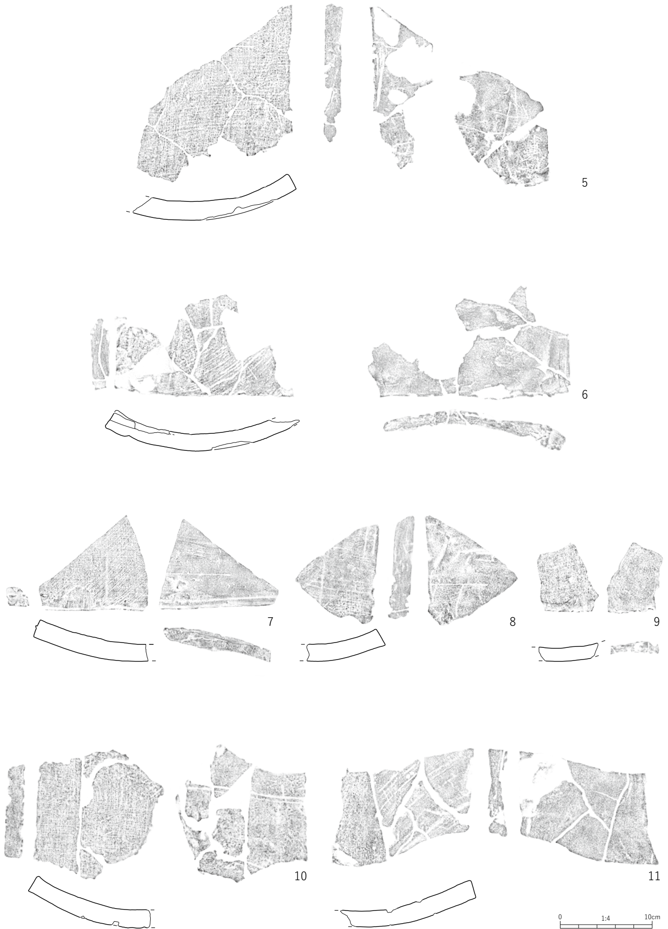
第168図 平瓦 SX01
