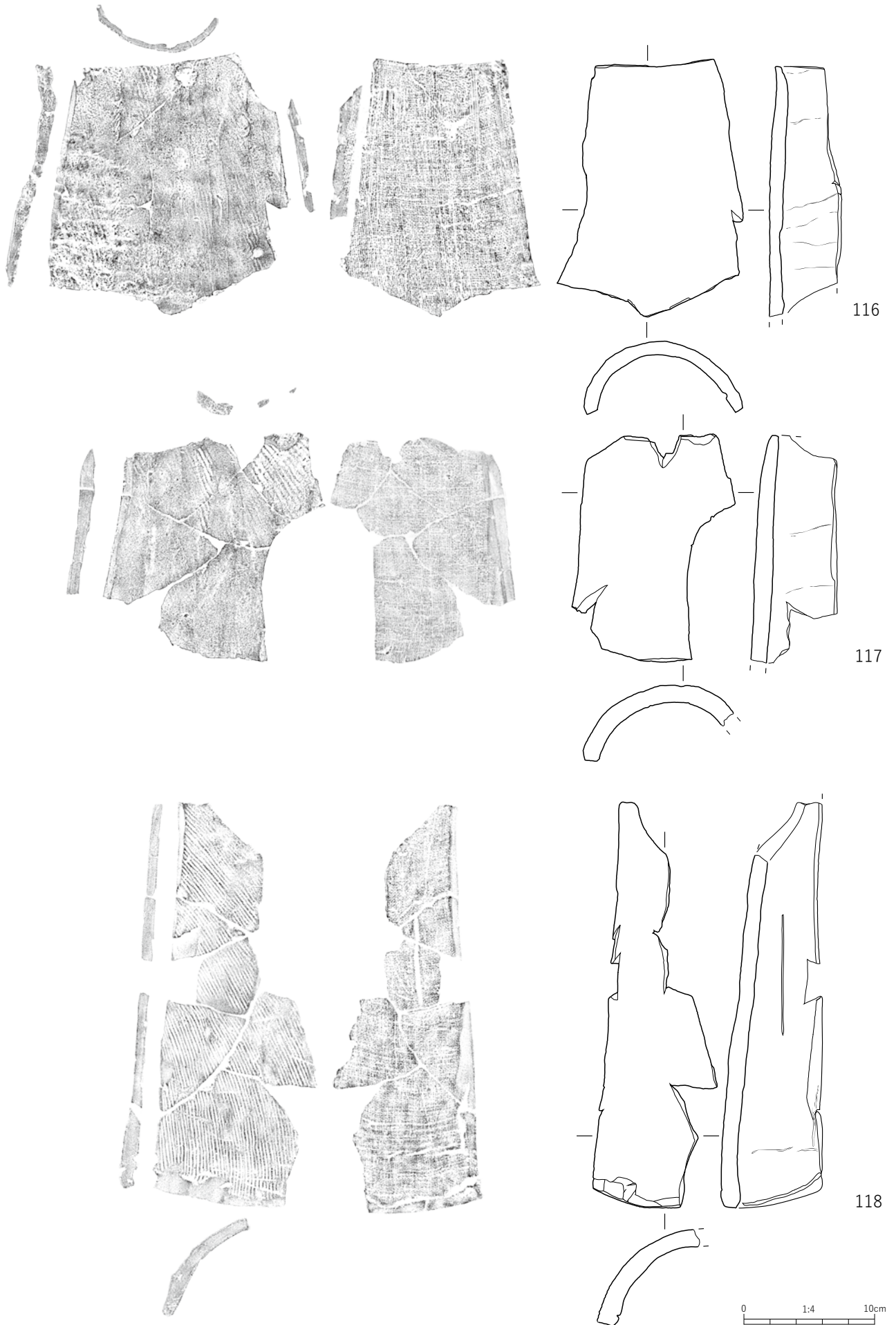
第153図 丸瓦 無段式 粘土帯桶巻づくりⅡ③類
