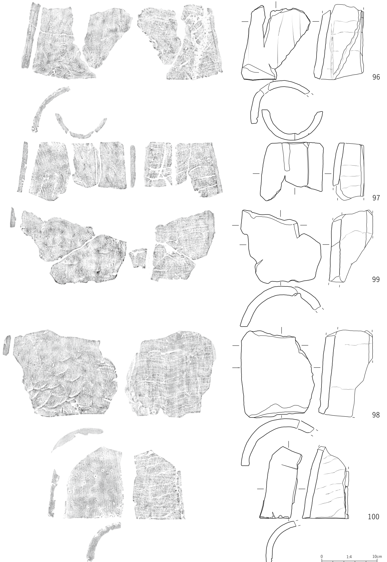
第147図 丸瓦 無段式 粘土帯桶巻づくりⅡ①類
