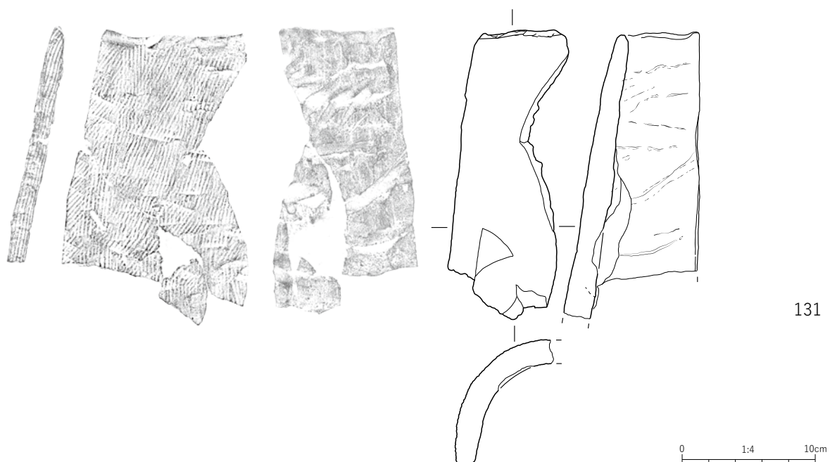
第157図 丸瓦 無段式 粘土紐マキアゲⅠ類
