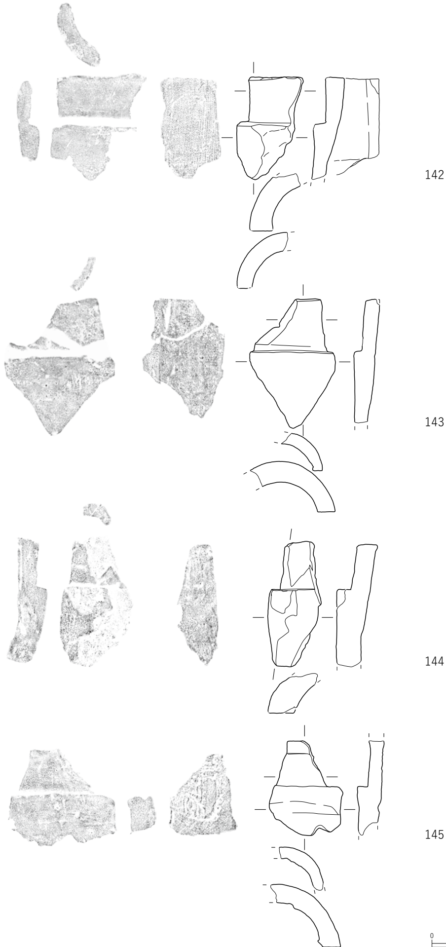
第162図 丸瓦 有段式 粘土板桶巻づくり I 類
