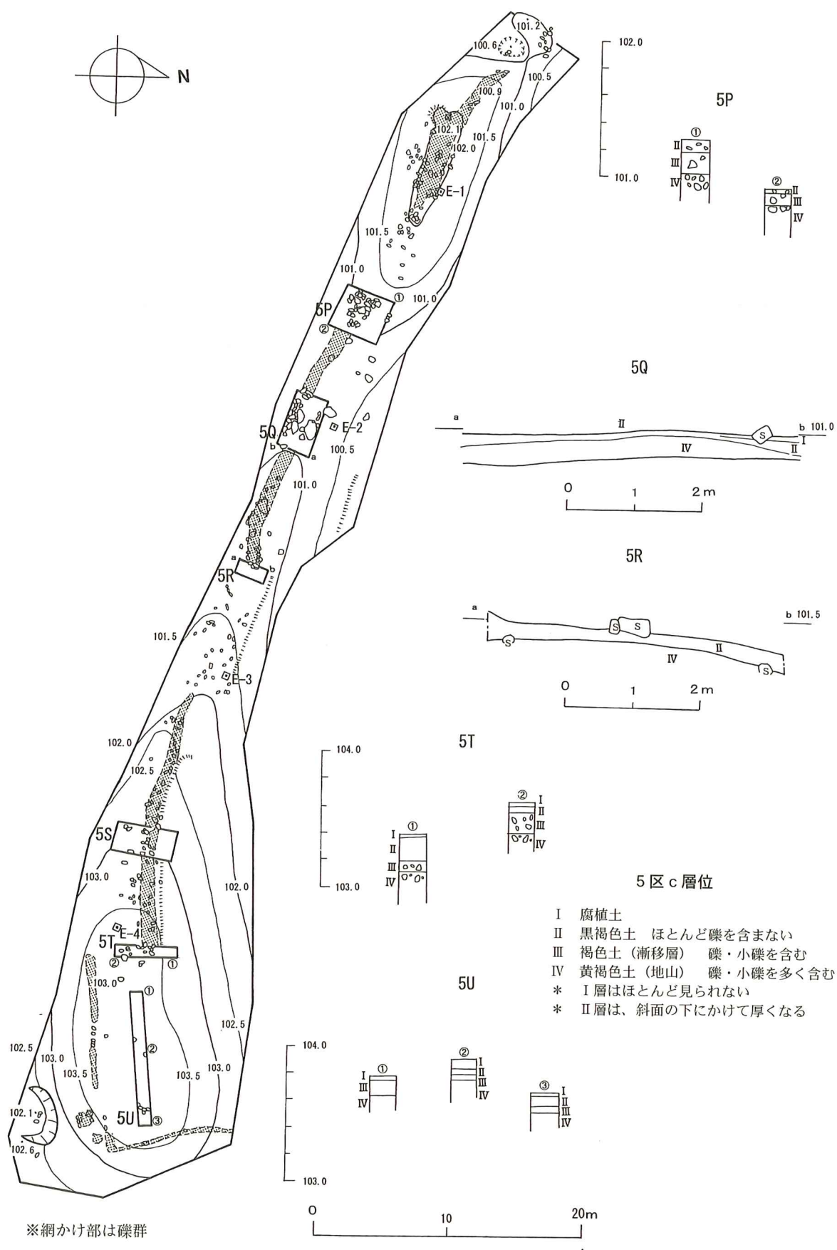
図VII-3 5区cの地形とトレンチ
