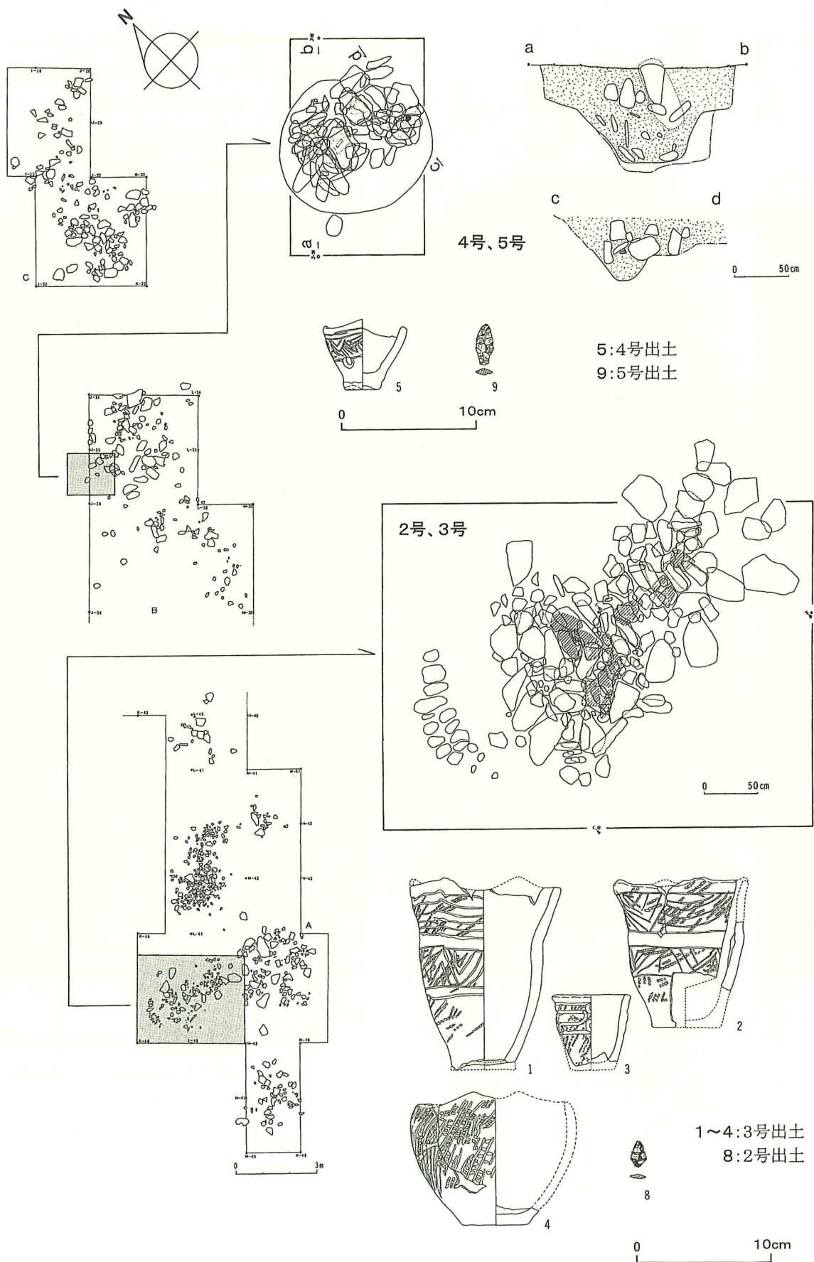
図VI-2 北海道大学調査実測図 (大場・重松 1977に加筆)
