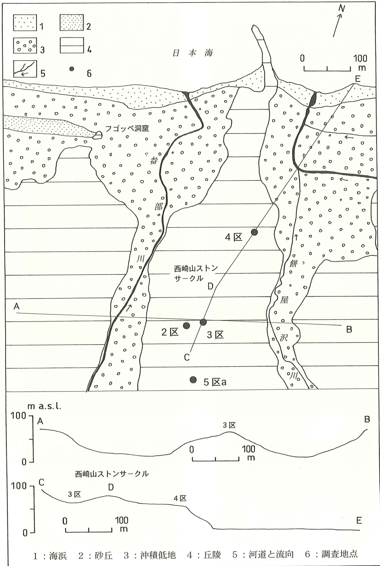
図Ⅱ-3 遺跡周辺の地形分類図
