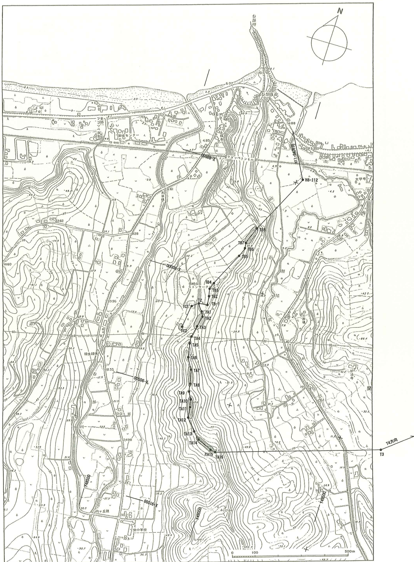
図Ⅲ—1 測量基準点網図
