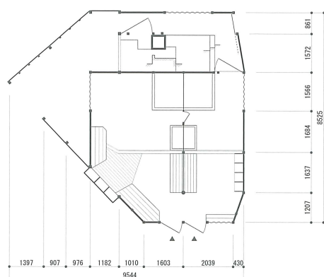
↑ 犬子淵共同浴場現況平面図 (1:200)
