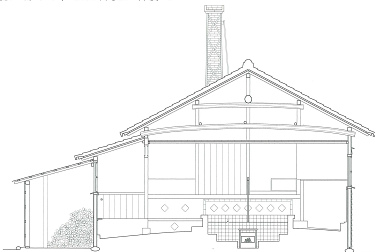
↑ 犬子淵共同浴場現状断面図 (1:100)
