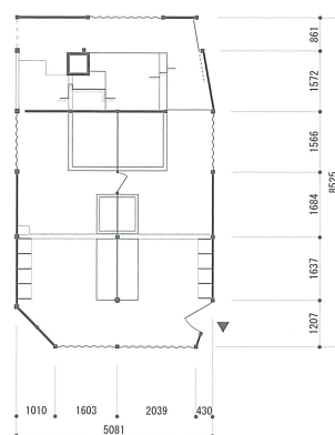
↑ 犬子淵共同浴場復原平面図 (1:200)
