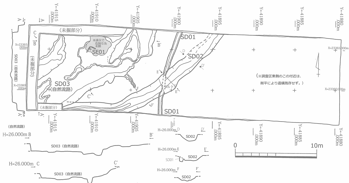
第4図 稲富・道免遺跡2区全体図 (S = 1 / 200)
