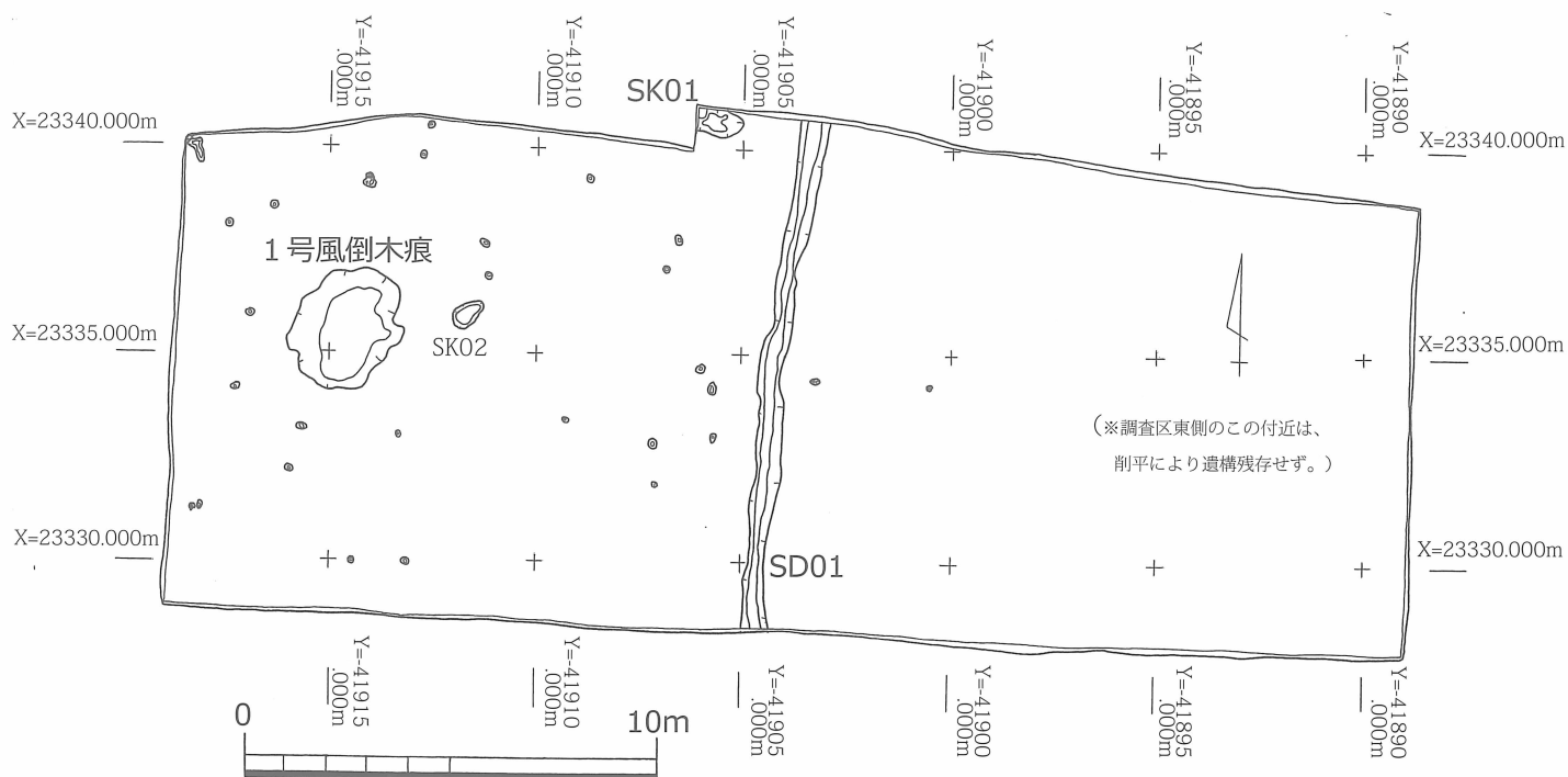
第5図 稲富・道免遺跡1区全体図 (S = 1 / 200)
