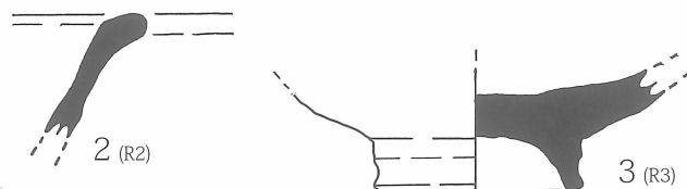
第8図 稲富・道免遺跡出土遺物実測図 (S = 1 / 2)
