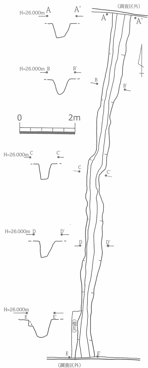
第6図 稲富・道免遺跡 SD01 溝状遺構実測図 (S = 1 / 80)
