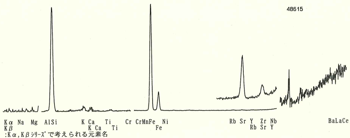
図Ⅷ-10-2 7-管玉 (48615) の蛍光X線スペクトル
