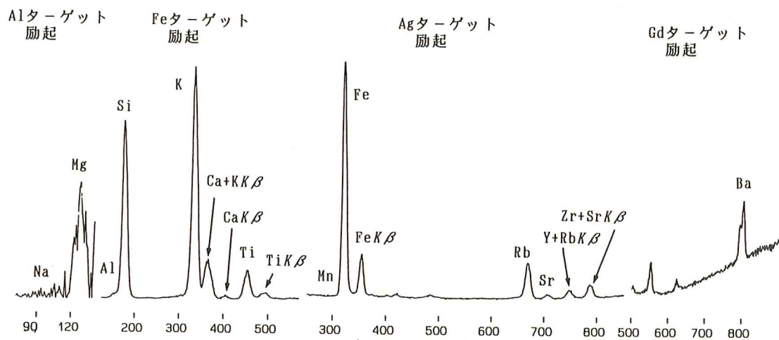
図Ⅷ-7-2 花仙山産碧玉原石の蛍光X線スペクトル
