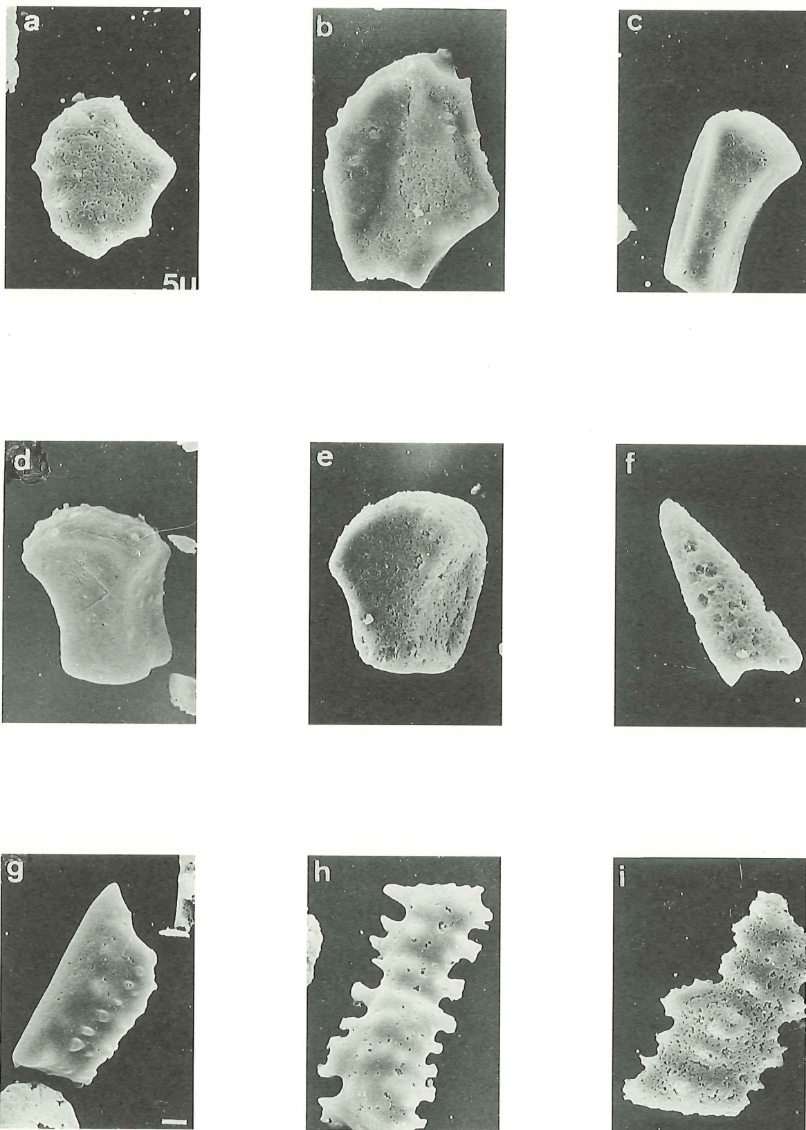
図Ⅷ-32 イネ科植物起源珪酸体の走査型電子顕微鏡写真（ファン型：a～d，ポイント型：f, g, 棒状型：h, i） M-2:g, i M-4:c M-7:f MF-3:d, e MX-:a, i MX-2:b
