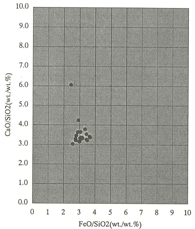
図Ⅷ－36 試料 1 (K o-d) の火山ガラスの化学成分分布
