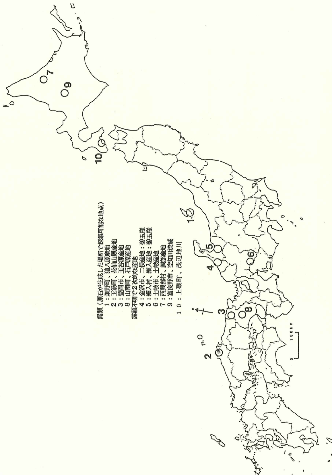
図Ⅷ-6 碧玉および碧玉様緑色石の原産地
