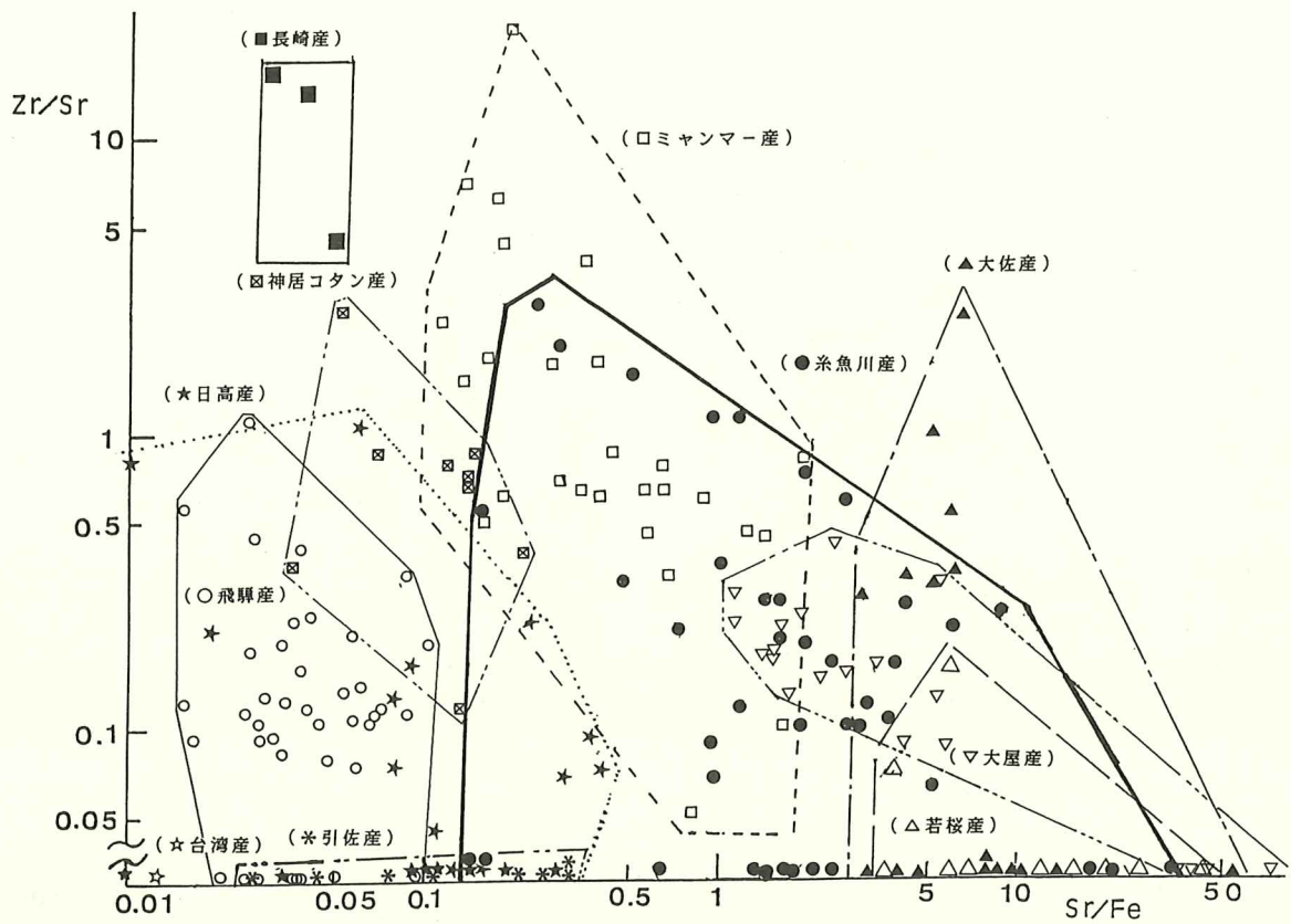
図Ⅷ-3-1 ヒスイ原石の元素比值Zr/Sr対Sr/Feの分布および分布範囲
