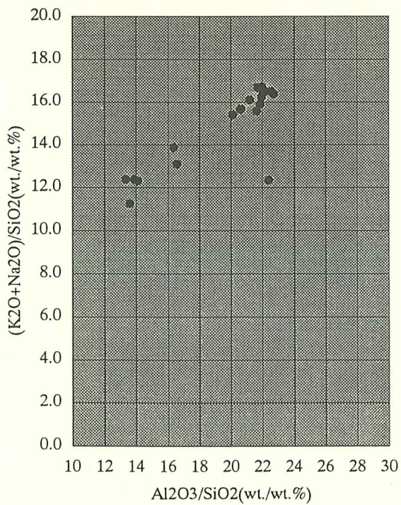
図Ⅷ-37 試料 2 (B-Tm) の火山ガラスの化学成分分布
