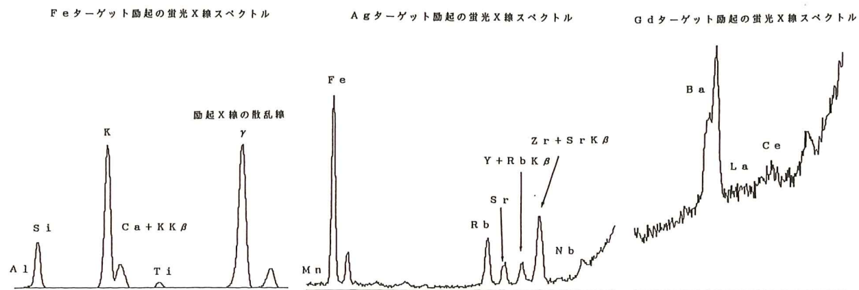
図Ⅷ-7-1 猿八産碧玉原石の蛍光X線スペクトル
