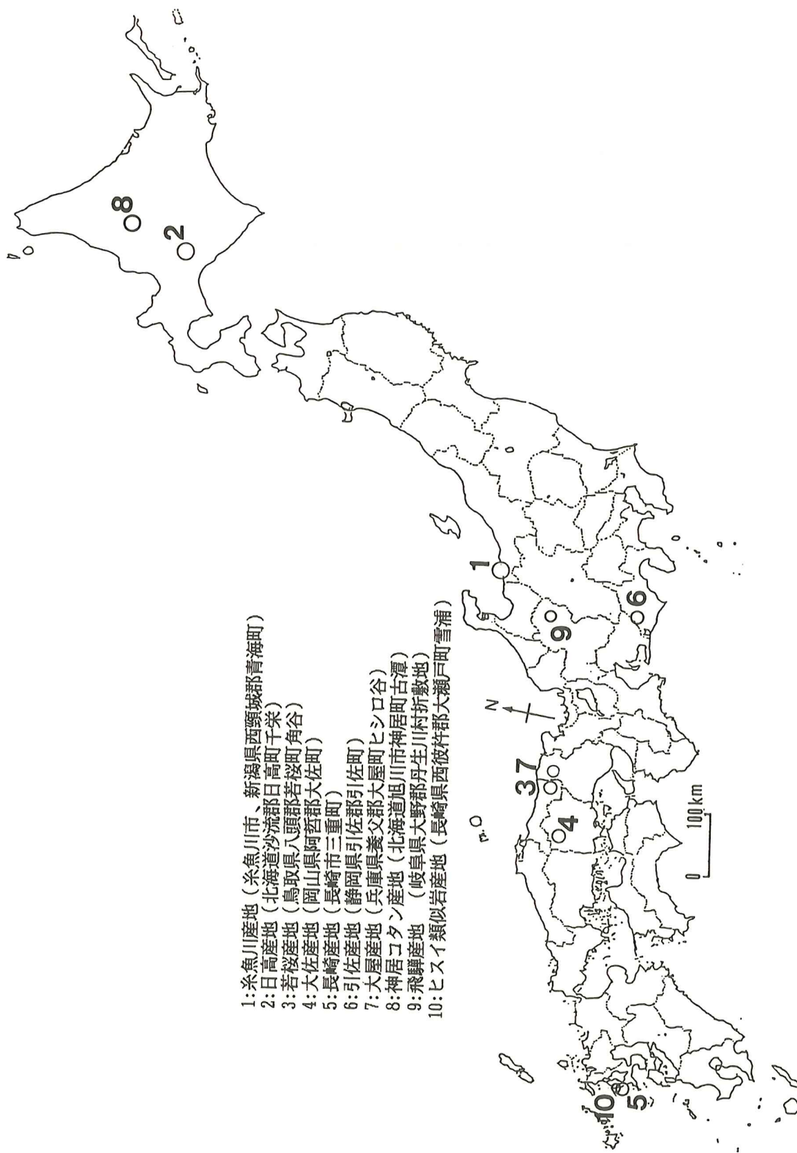
図Ⅷ-2 ヒスイとヒスイ類似岩の原産地
