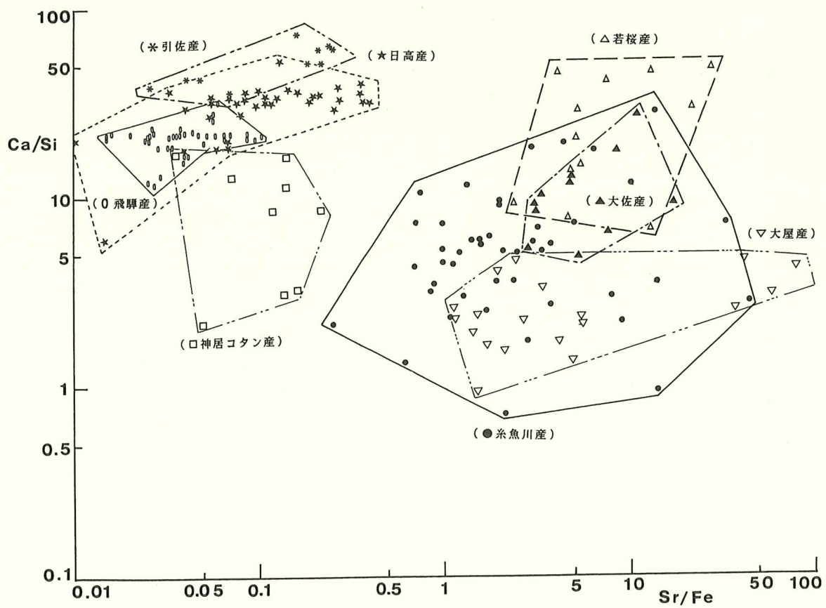
図Ⅷ-3-2 ヒスイ原石の元素比值Ca/Si対Sr/Feの分布および分布範囲
