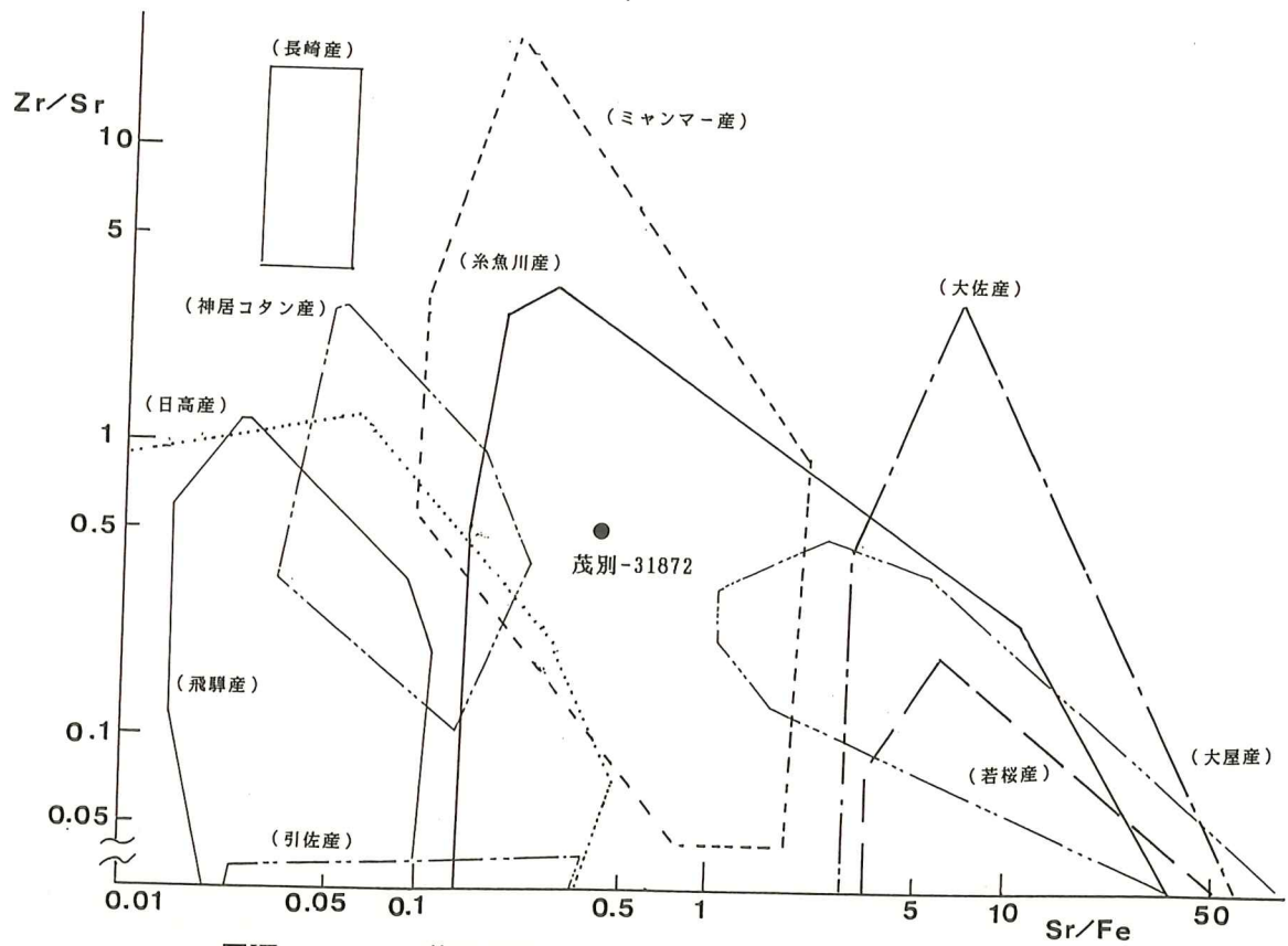
図Ⅷ-4-2 茂別遺跡出土のヒスイ製玉のZr/Sr対Sr/Feの分布
