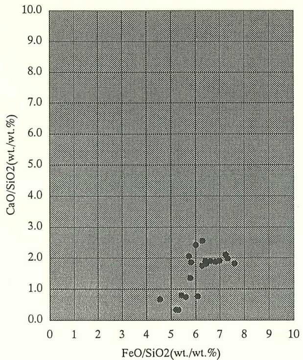
図Ⅷ-37 試料 2 (B-Tm) の火山ガラスの化学成分分布
