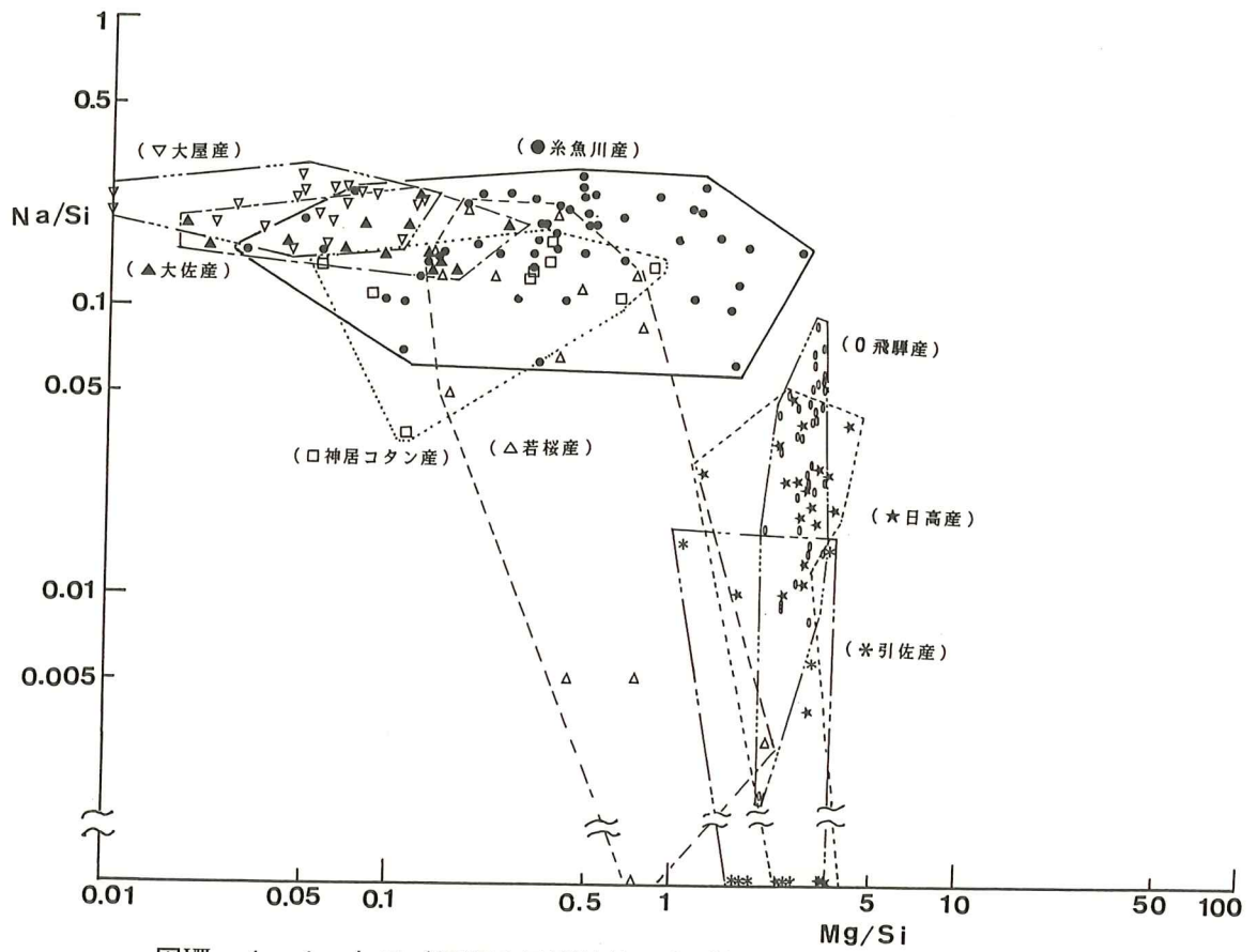
図Ⅷ-4-1 ヒスイ原石の元素比值Na/Si対Mg/Siの分布および分布範囲
