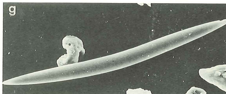
図Ⅷ-34 イネ科植物起源珪酸体、珪藻および海綿骨針の走査型電子顕微鏡写真（根由来の薄板状珪酸体：a, b, c 珪藻：f 海綿骨針：d, e, f） M-2：f M-4：a, b M-5：c M-7：d FM-3：g MX-2：e
