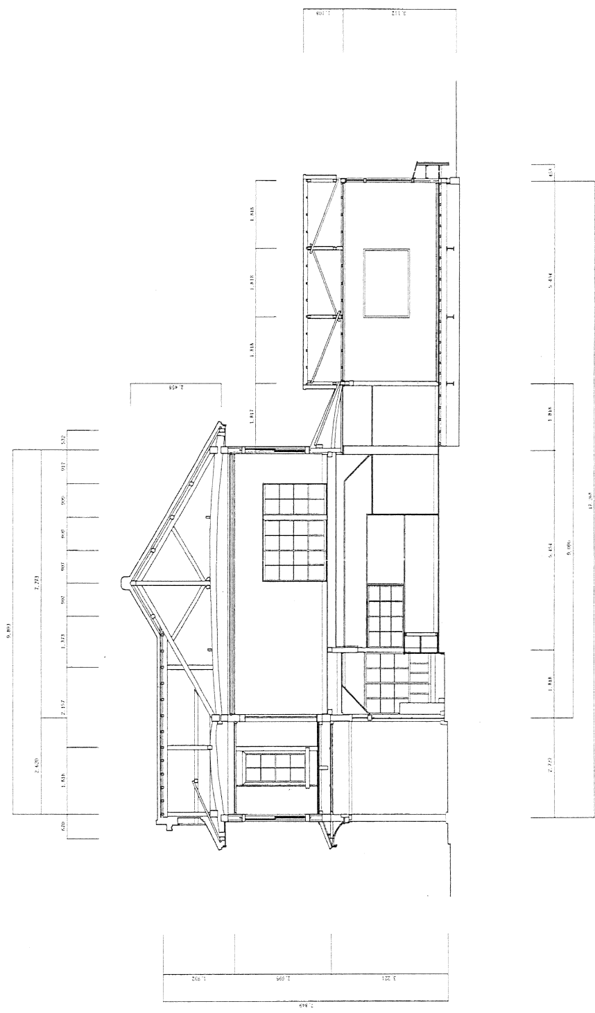
0-1-B' 断面图
