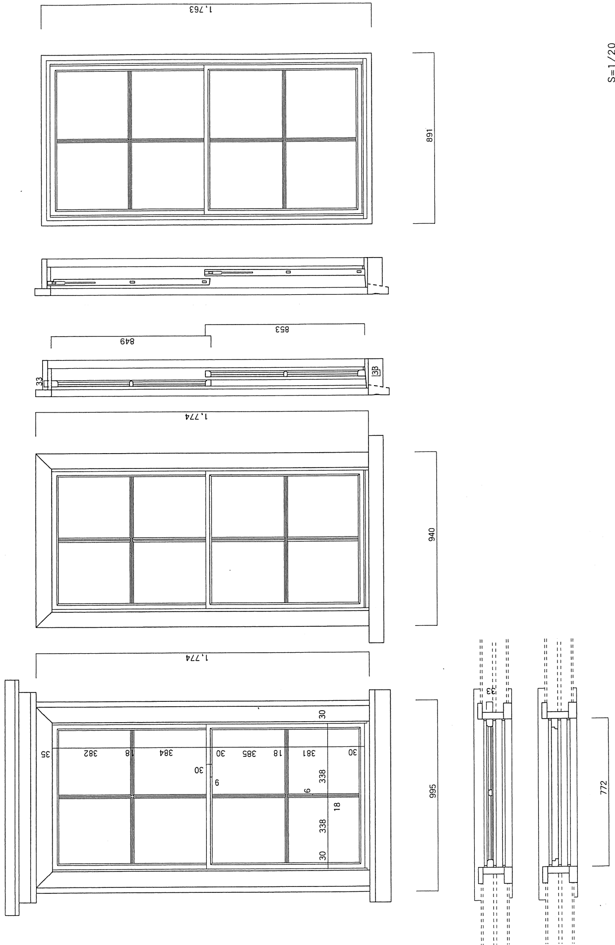
上げ下げ窓実測図
