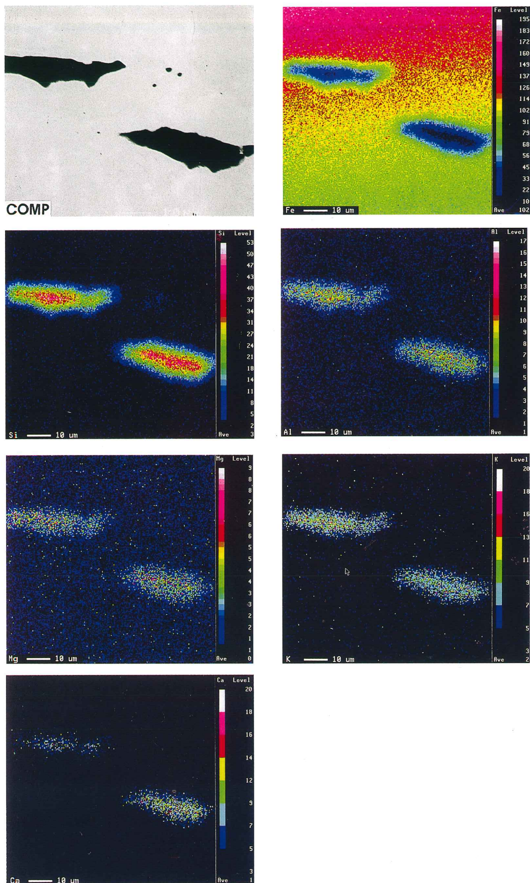
Fig. 108 蛇行剣(73)に見いだされた非金属介在物の EPMA による組成像 (COMP) と含有される元素濃度分布のカラーマップ 色が青→黄→赤→白の順に含有量レベルが高い。
