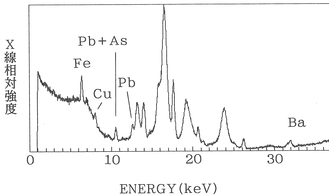
Fig. 112 蛍光X線スペクトル(試料名称190)
