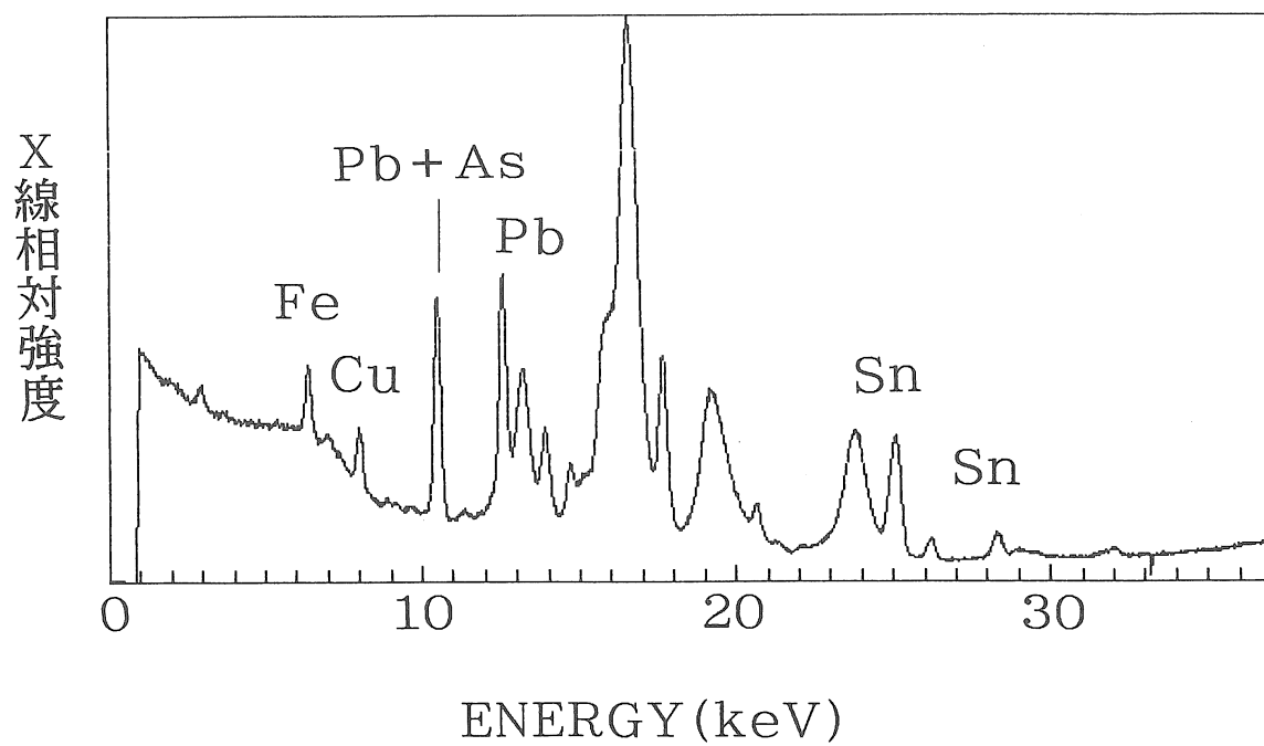
Fig. 110 蛍光X線スペクトル(試料名称254)
