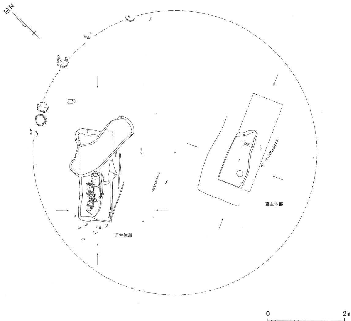
Fig. 115 墳頂部 円筒埴輪列・主体部配置復元図〔1:60〕
