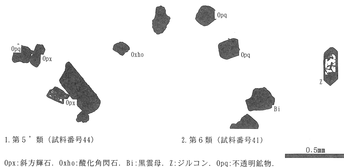
Fig. 100 胎土中の重鉱物 2
