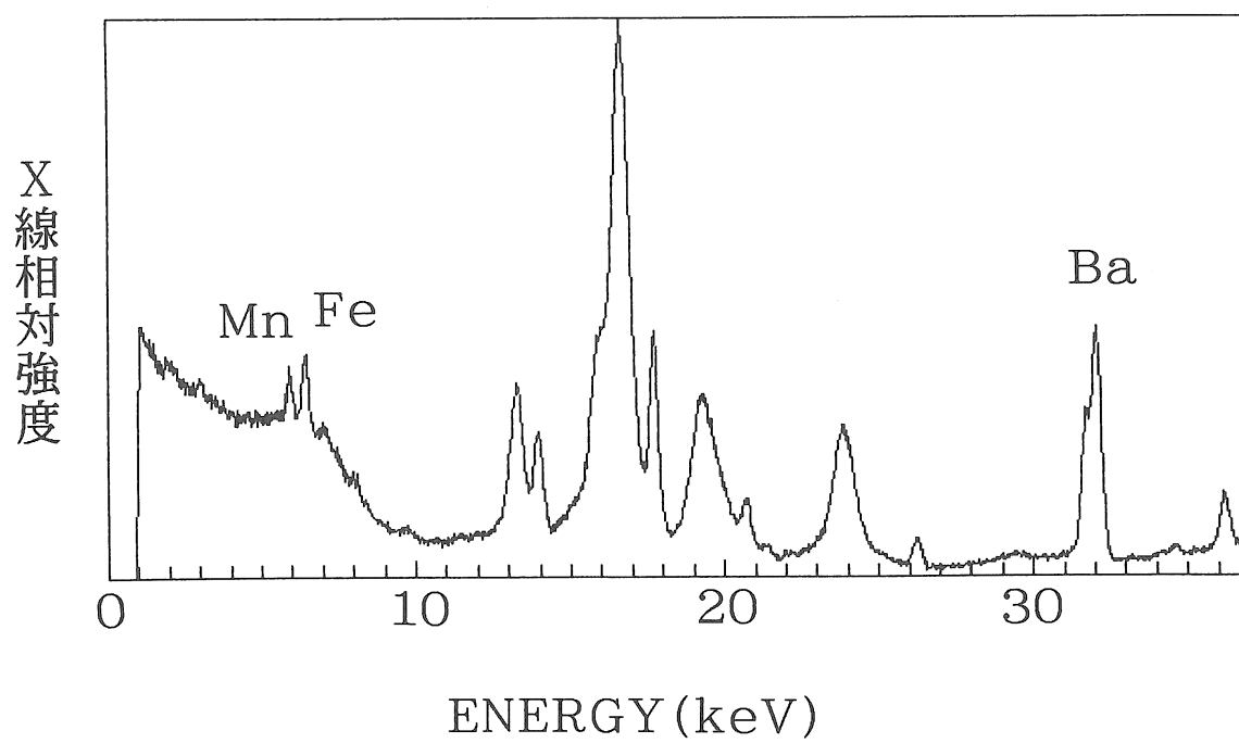
Fig. 111 蛍光X線スペクトル(試料名称210)
