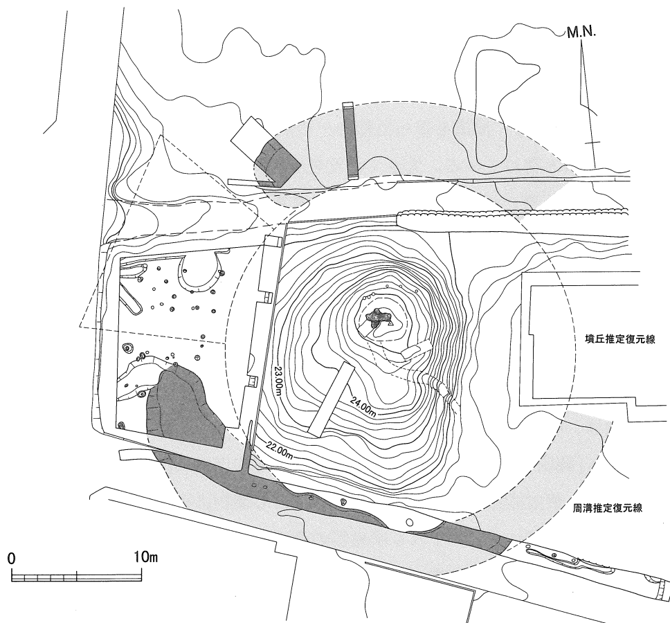
Fig. 114 墳丘・周溝形態復元図〔1:400〕
