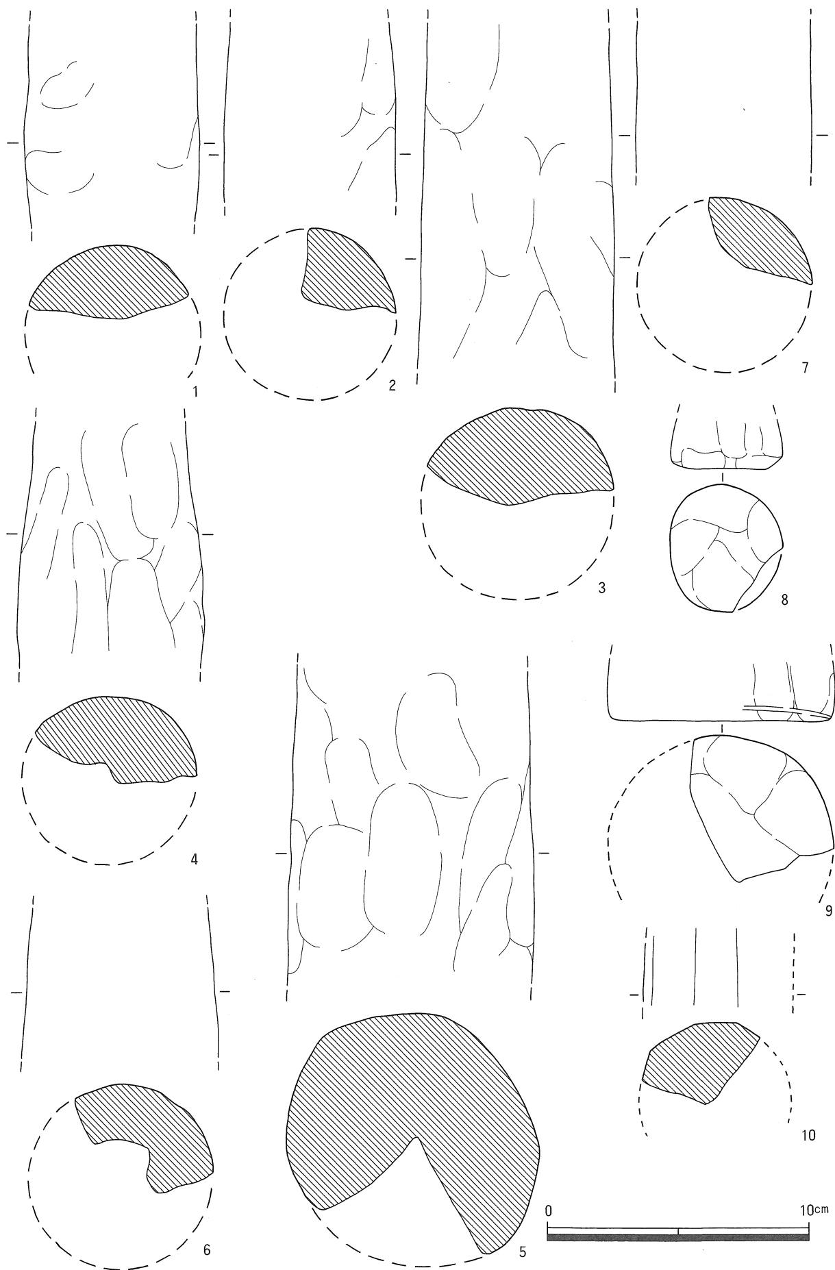
第137図 土製支脚実測図
