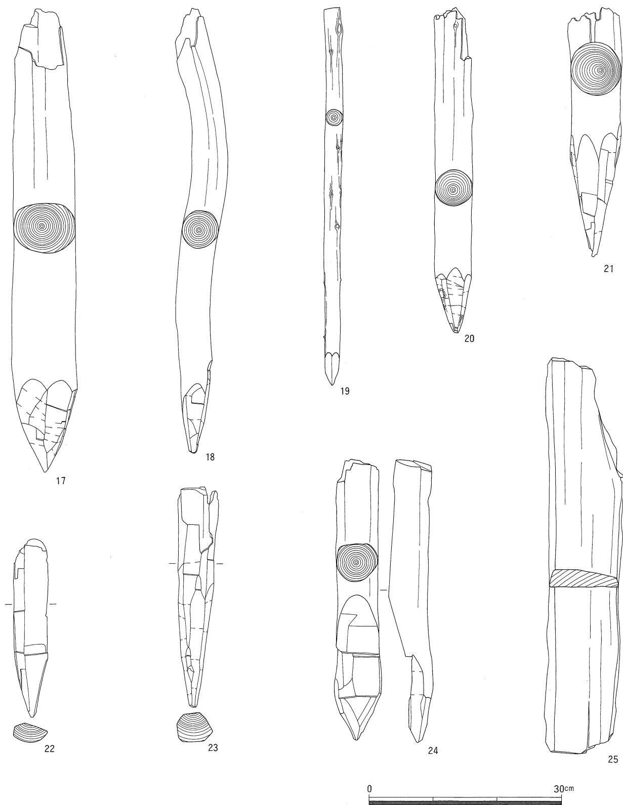
第142図 杭実測図（2）
