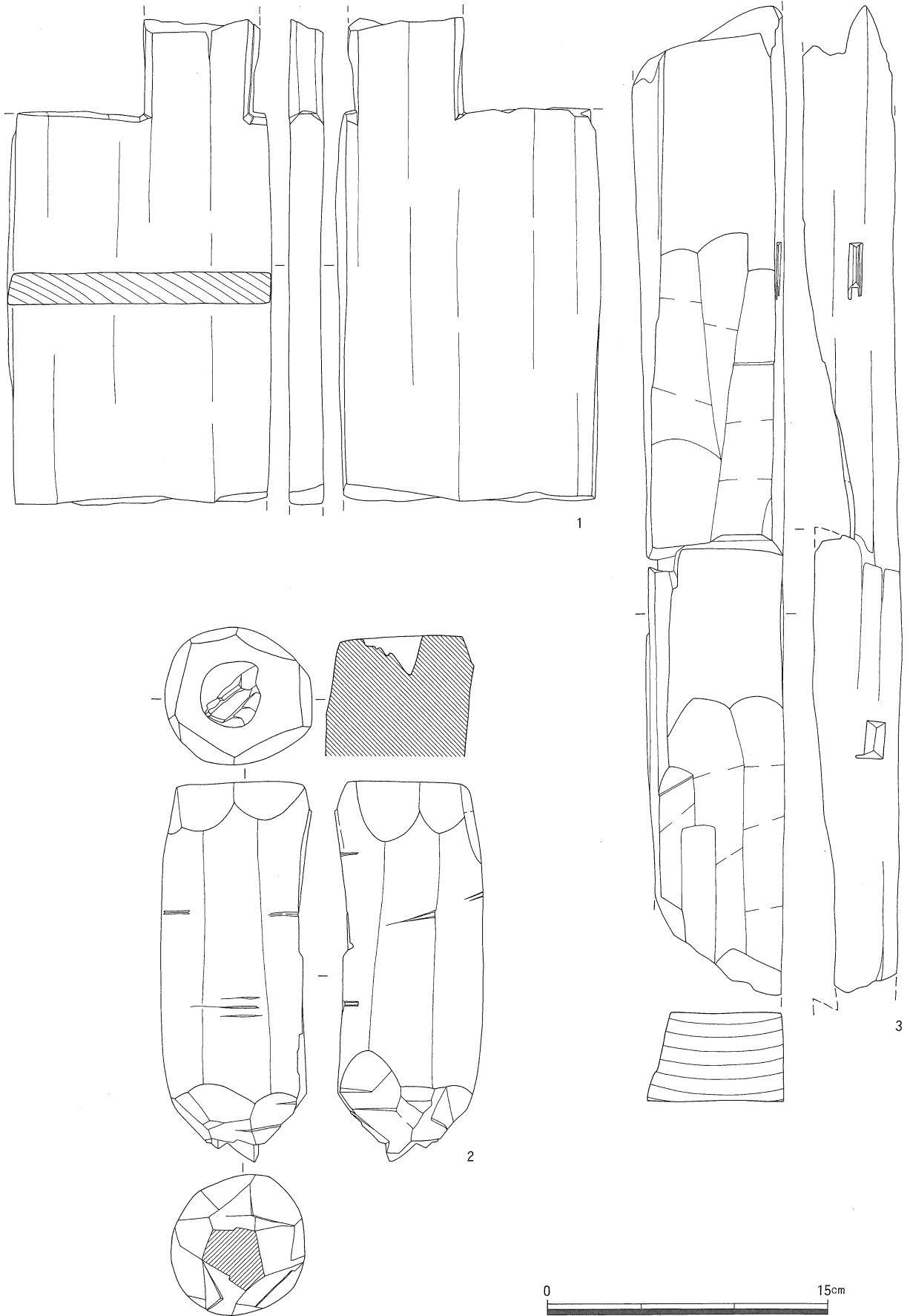
第143図 部材実測図
