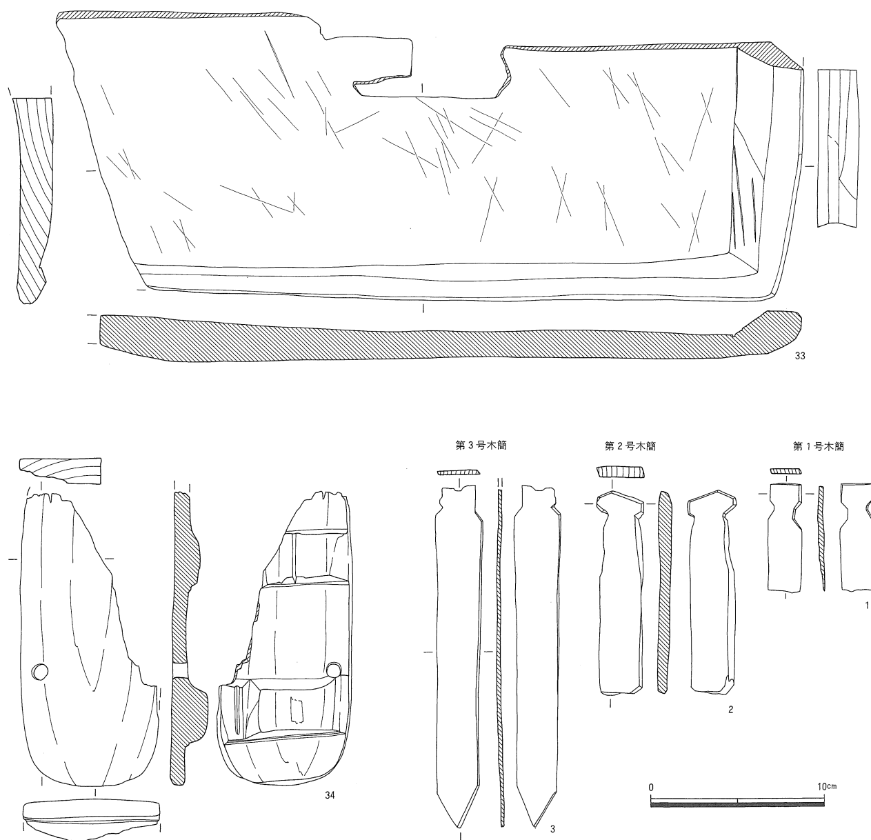
第149図 木製品実測図（5） 木簡実測図
