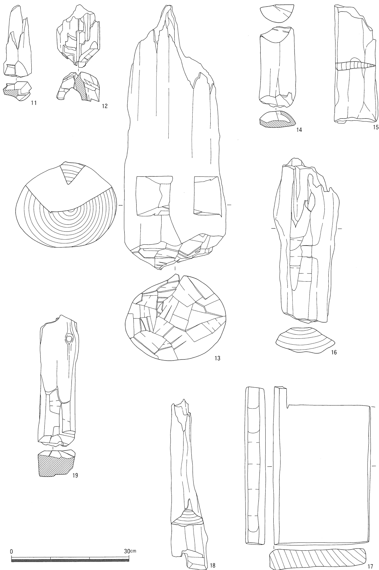
第140図 柱根実測図（2） 礎板実測図
