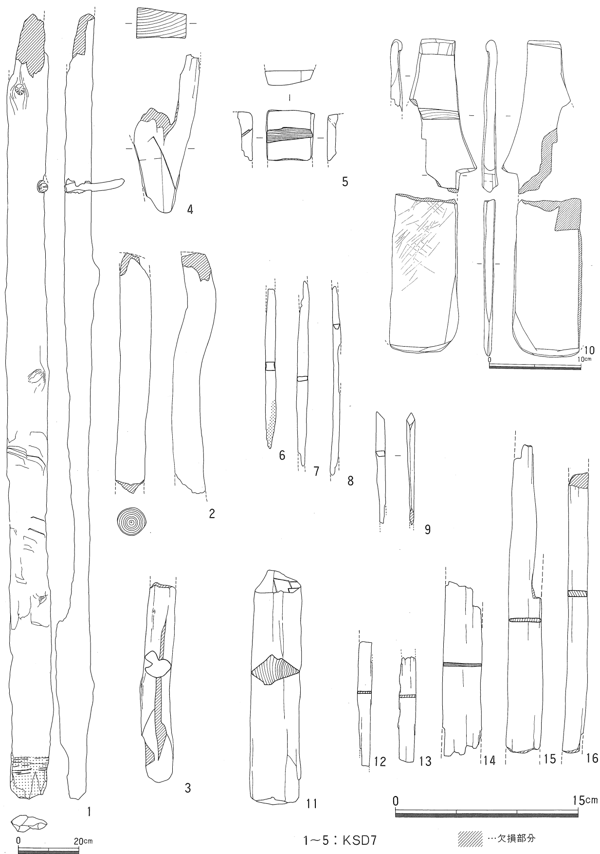
第122図 木製品実測図（1）
