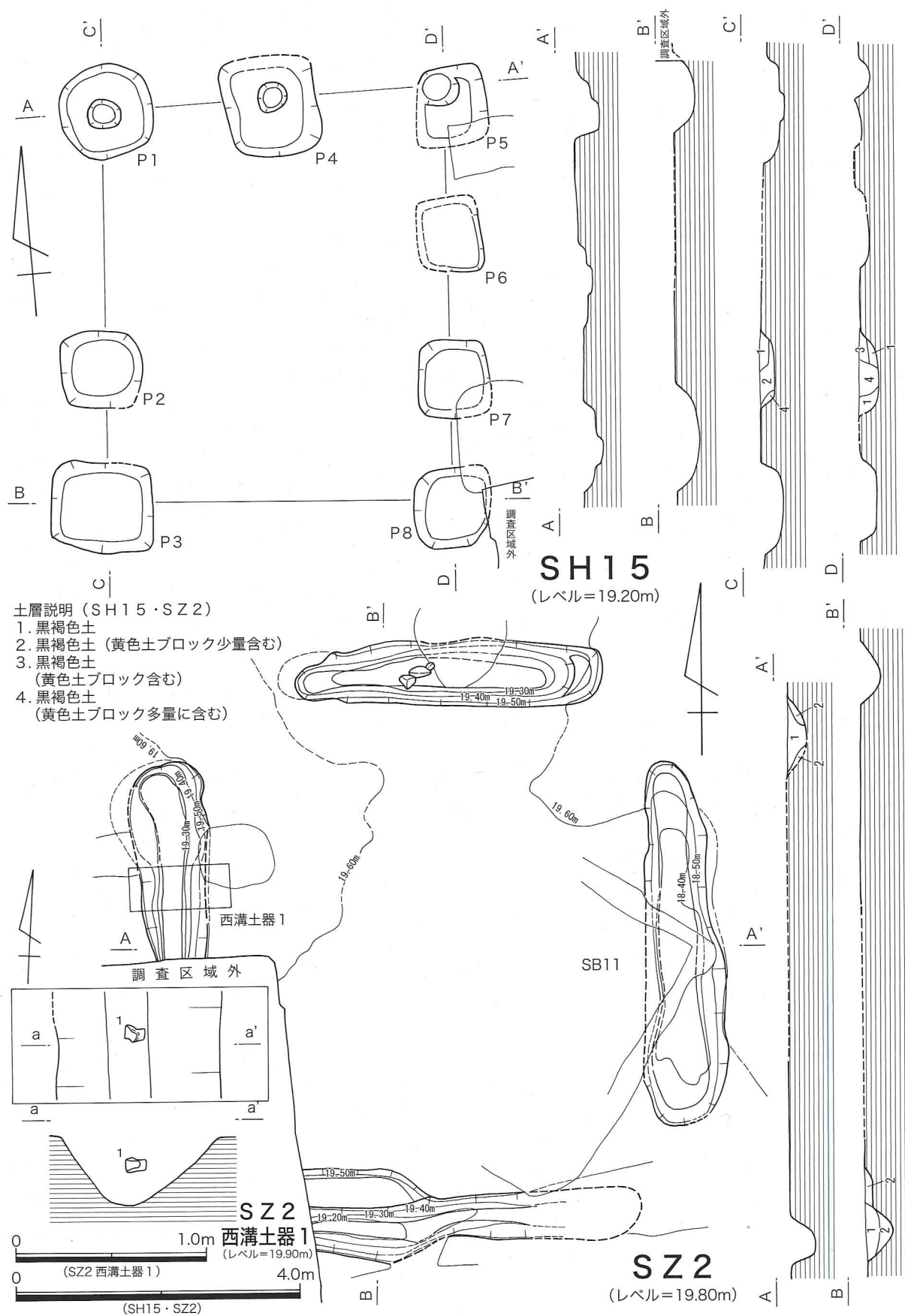
第6図 第38～40・48次 SH15・SZ2 実測図
