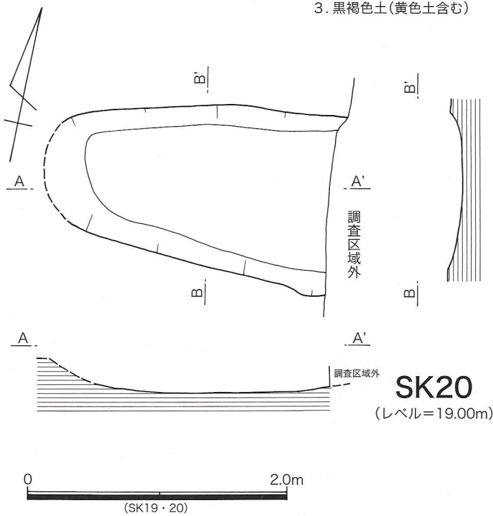
第25図 第41～43次 SK18～20、P5 実測図
