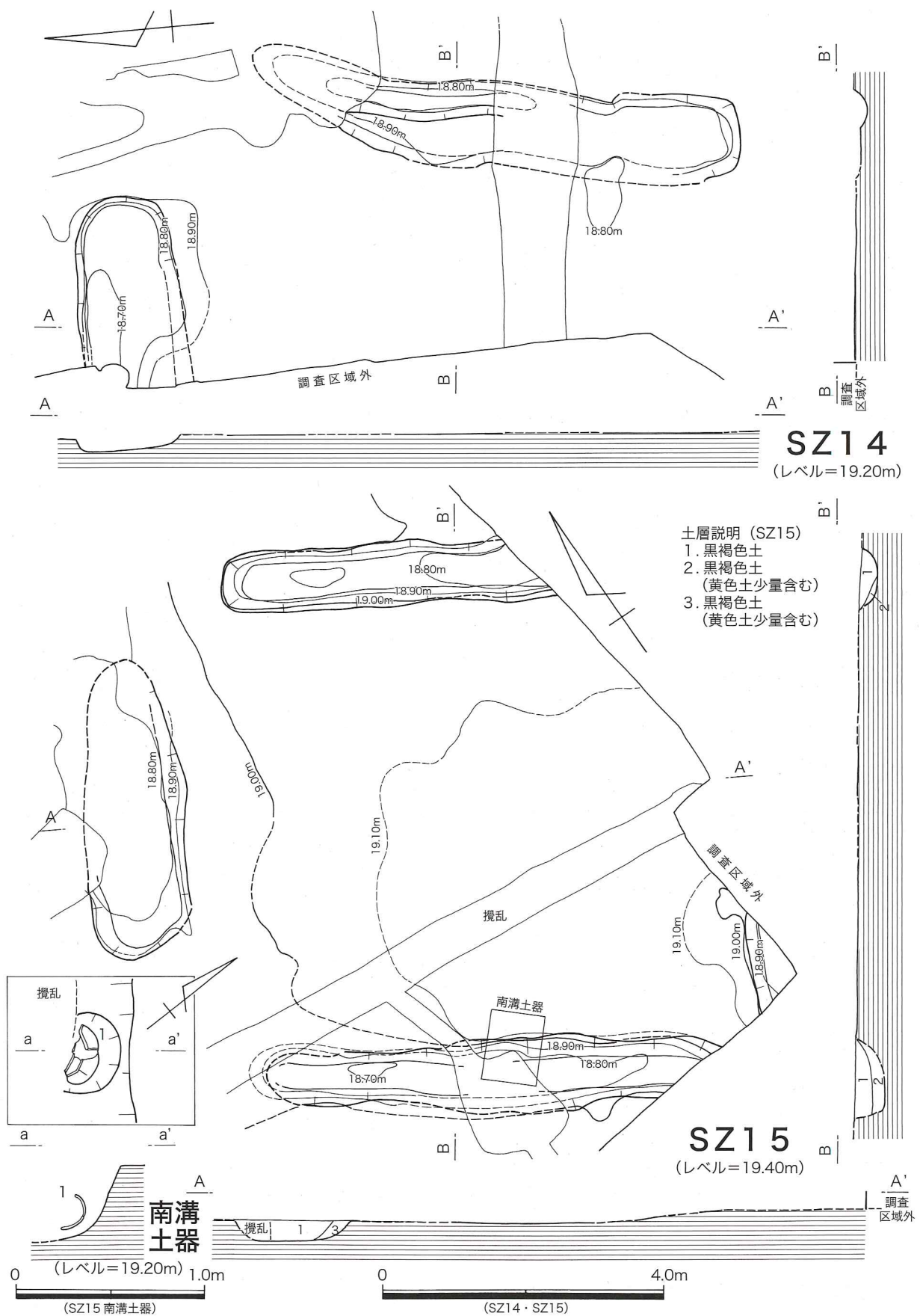
第9図 第38～40・48次 SZ14・15 実測図
