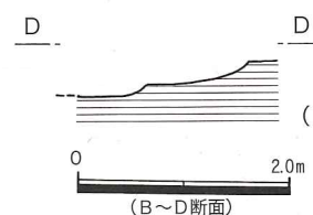
第147図 第49次 P96・111実測図、SD30～32土層図
