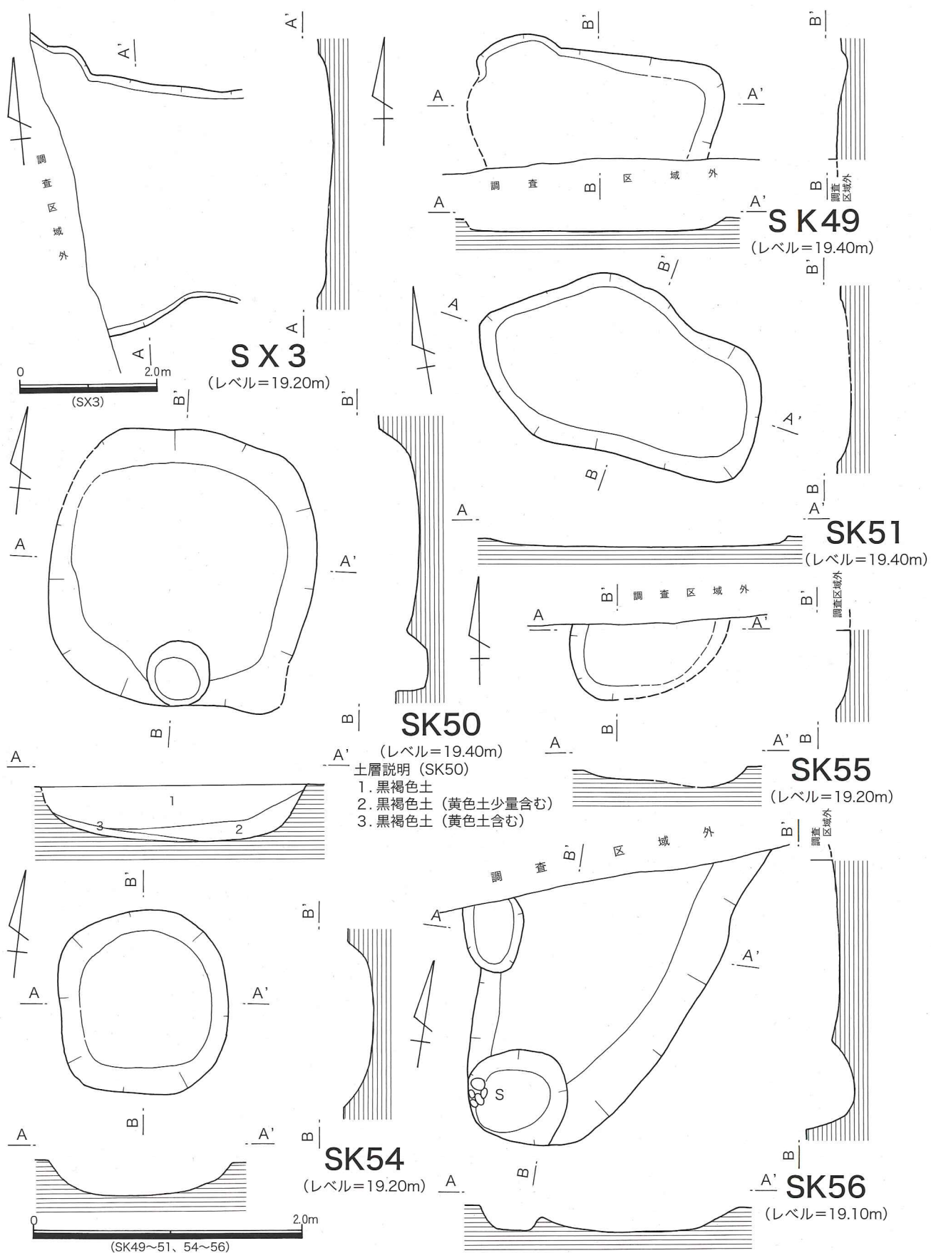
第174図 第52次 SX3、SK49~51・54~56実測図
