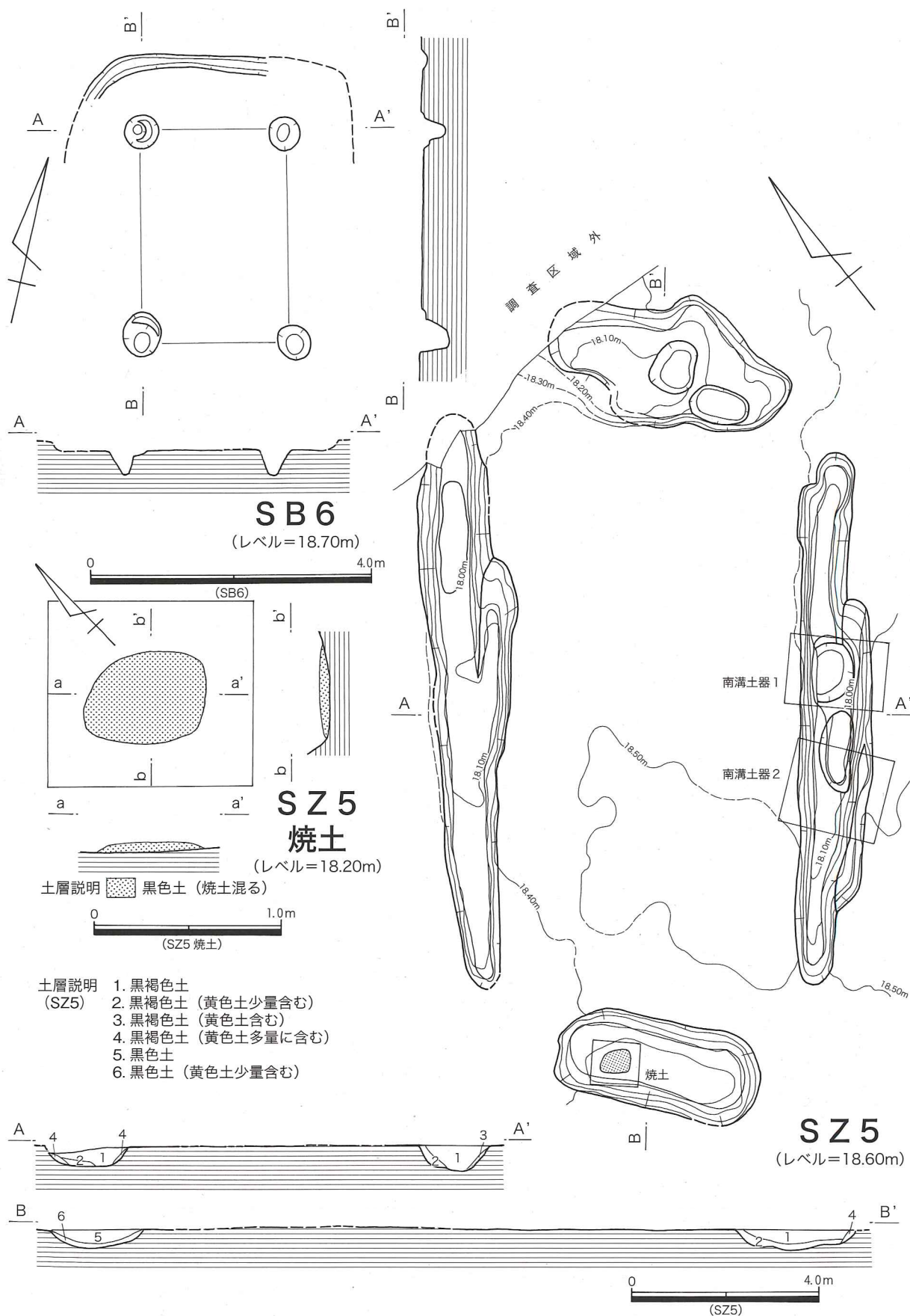
第206図 第55次 SB6、SZ5実測図
