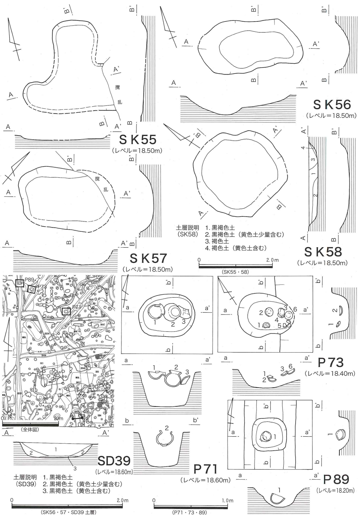
第213図 第55次 SK55～58、P71・73・89実測図、SD39土層図
