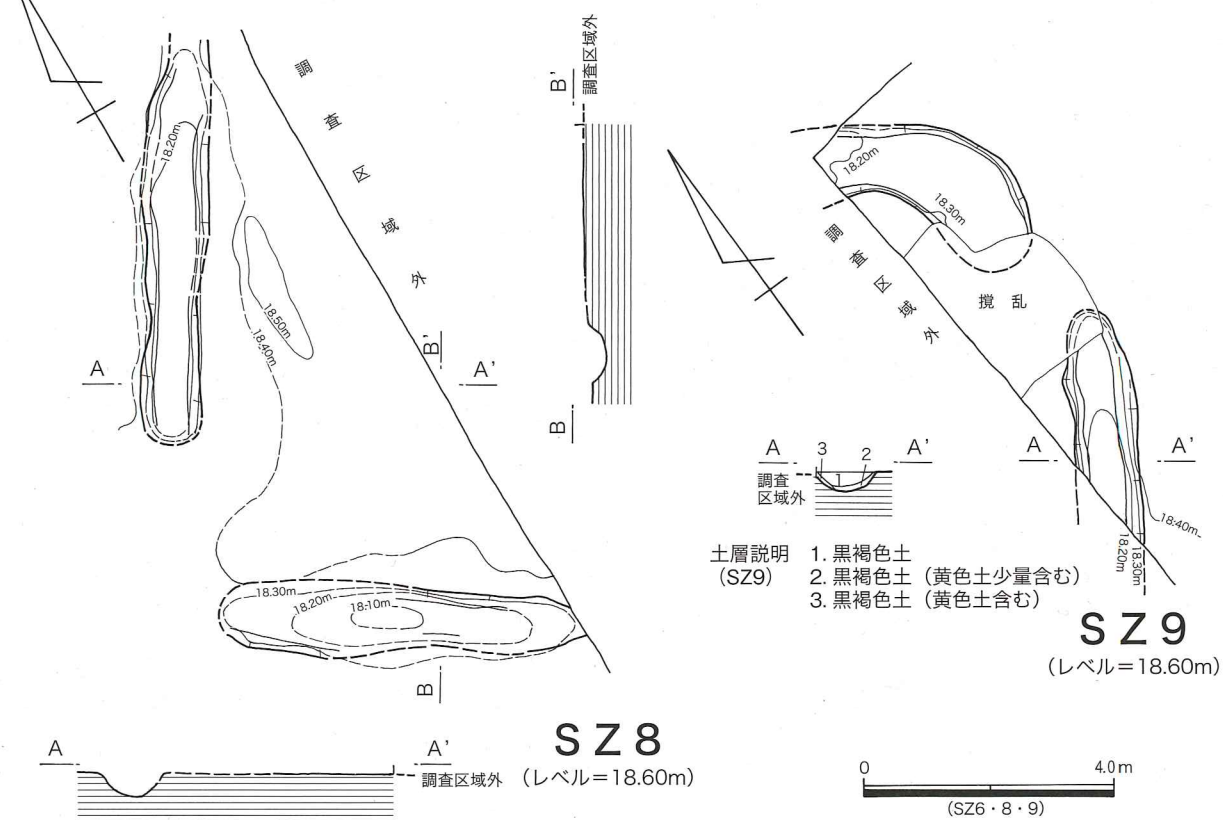
第196図 第54次 SZ6・8・9実測図
