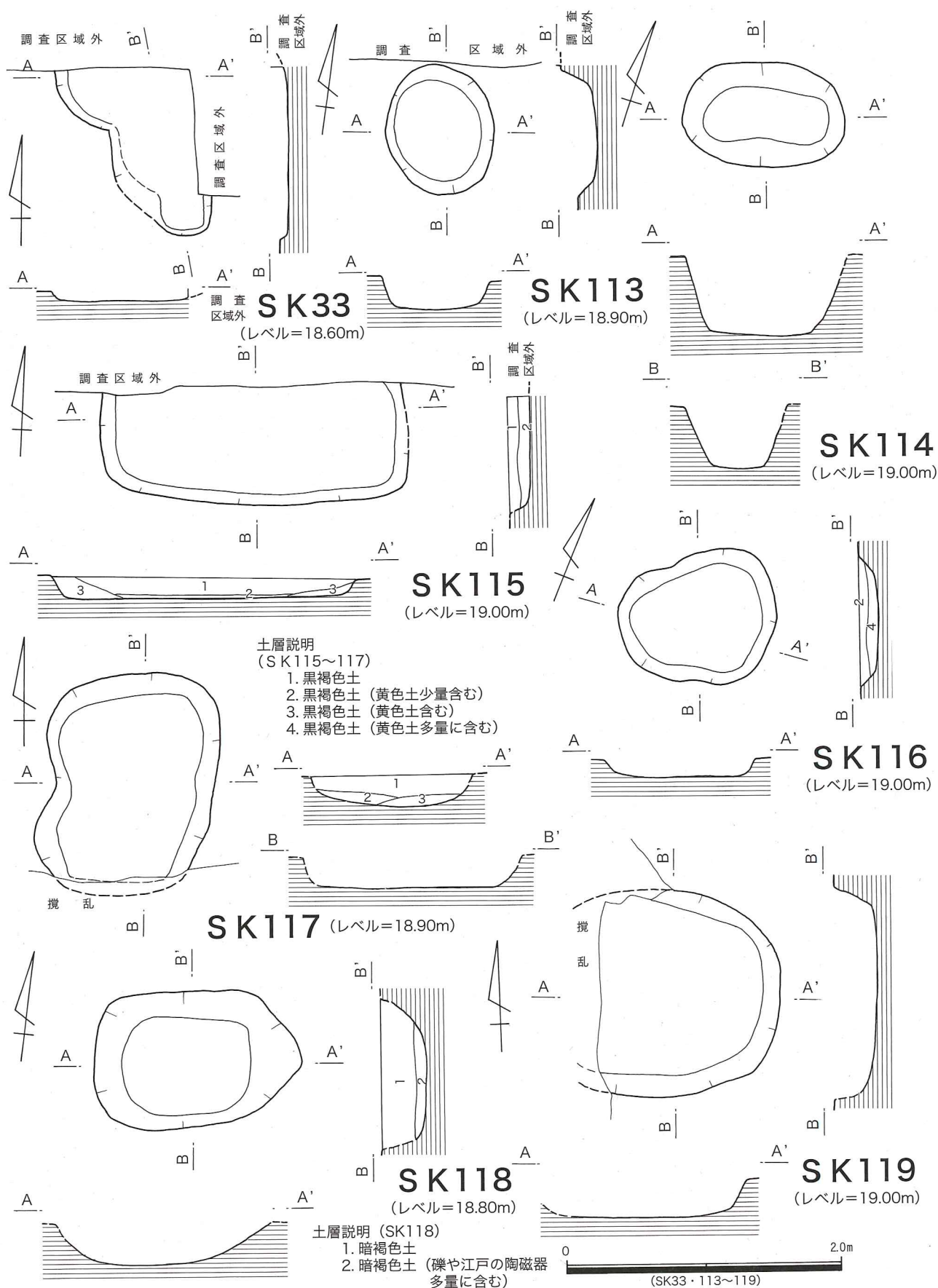
第127図 第47・51次 SK33・113～119実測図
