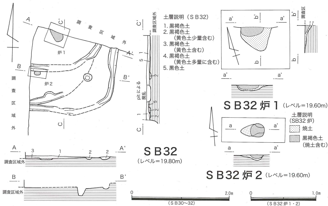
第142図 第49次 S B 30 ~ 32実測図
