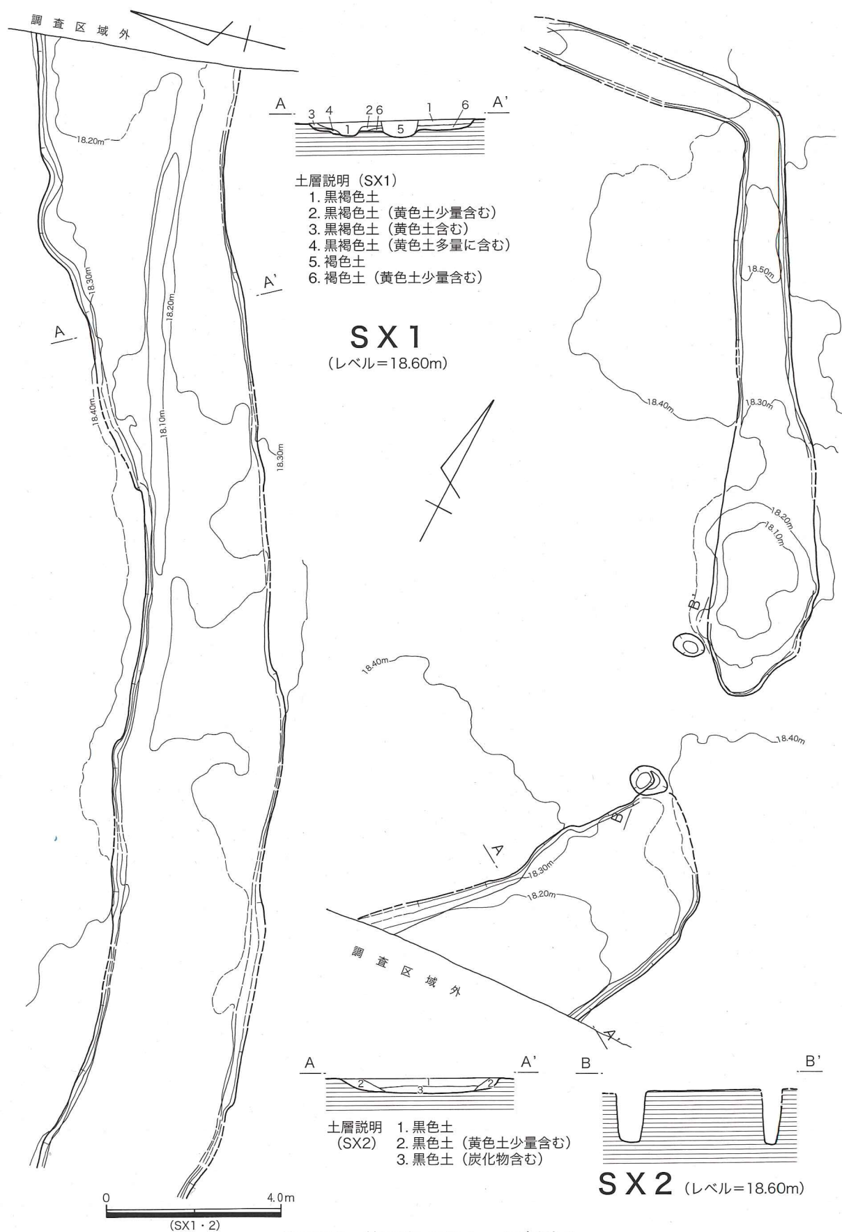
第210図 第55次 SX1・2実測図
