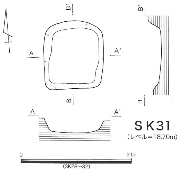
第126図 第47・51次 S K28 ~ 32実測図
