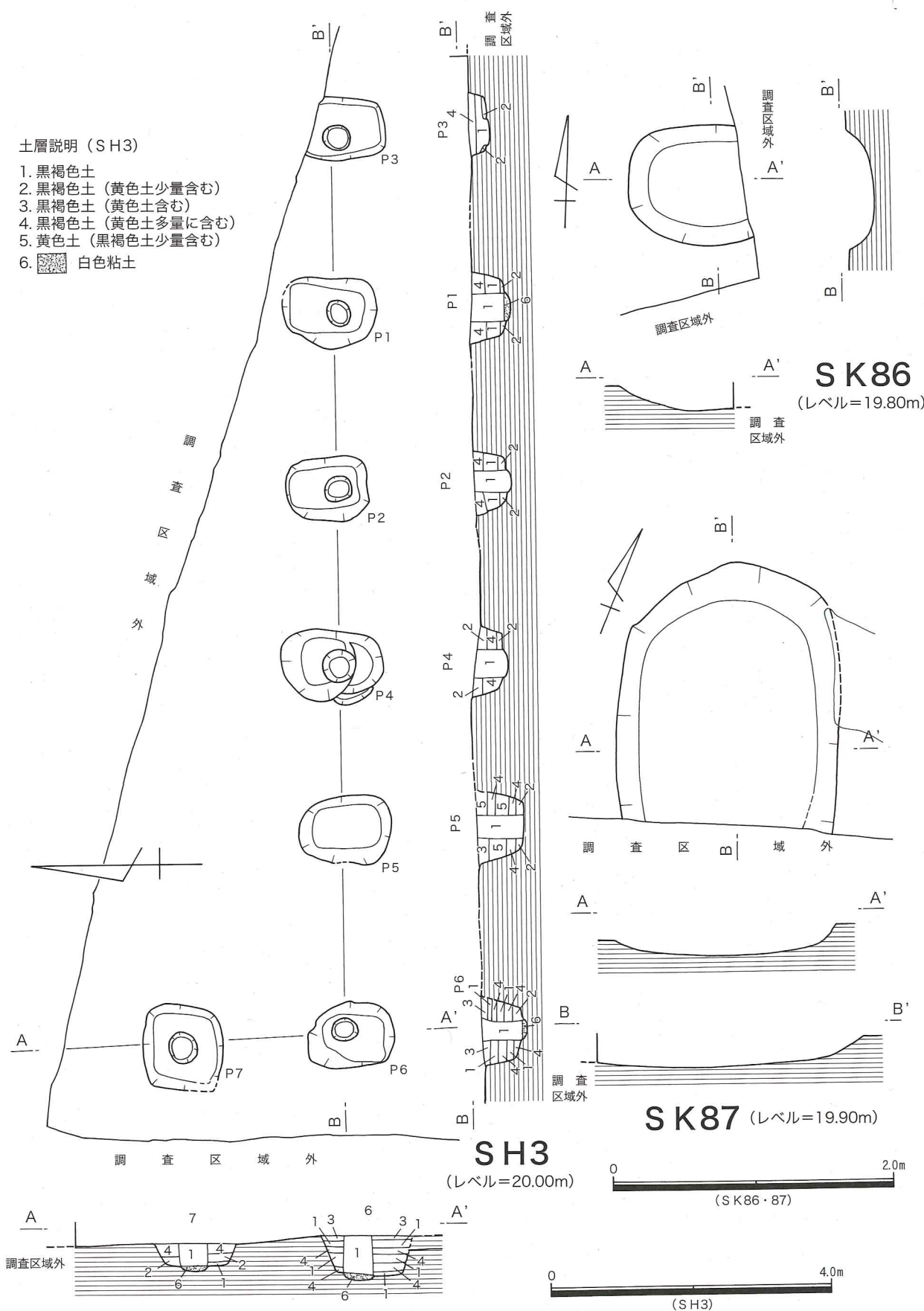
第143図 第49次 SH3、SK86・87実測図
