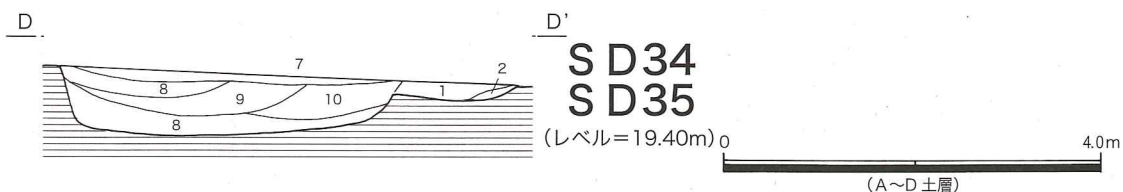
第175図 第52次 P55・127実測図、SD31～35土層図
