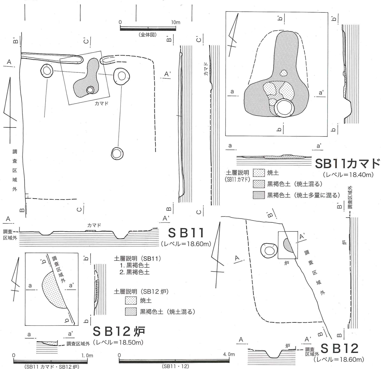
第195図 第54次 基本土層図、SB11・12実測図
