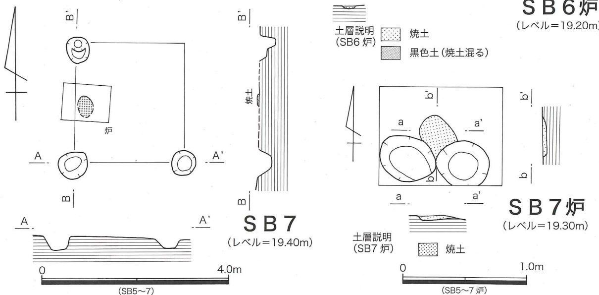
第171図 第52次 SB5~7実測図
