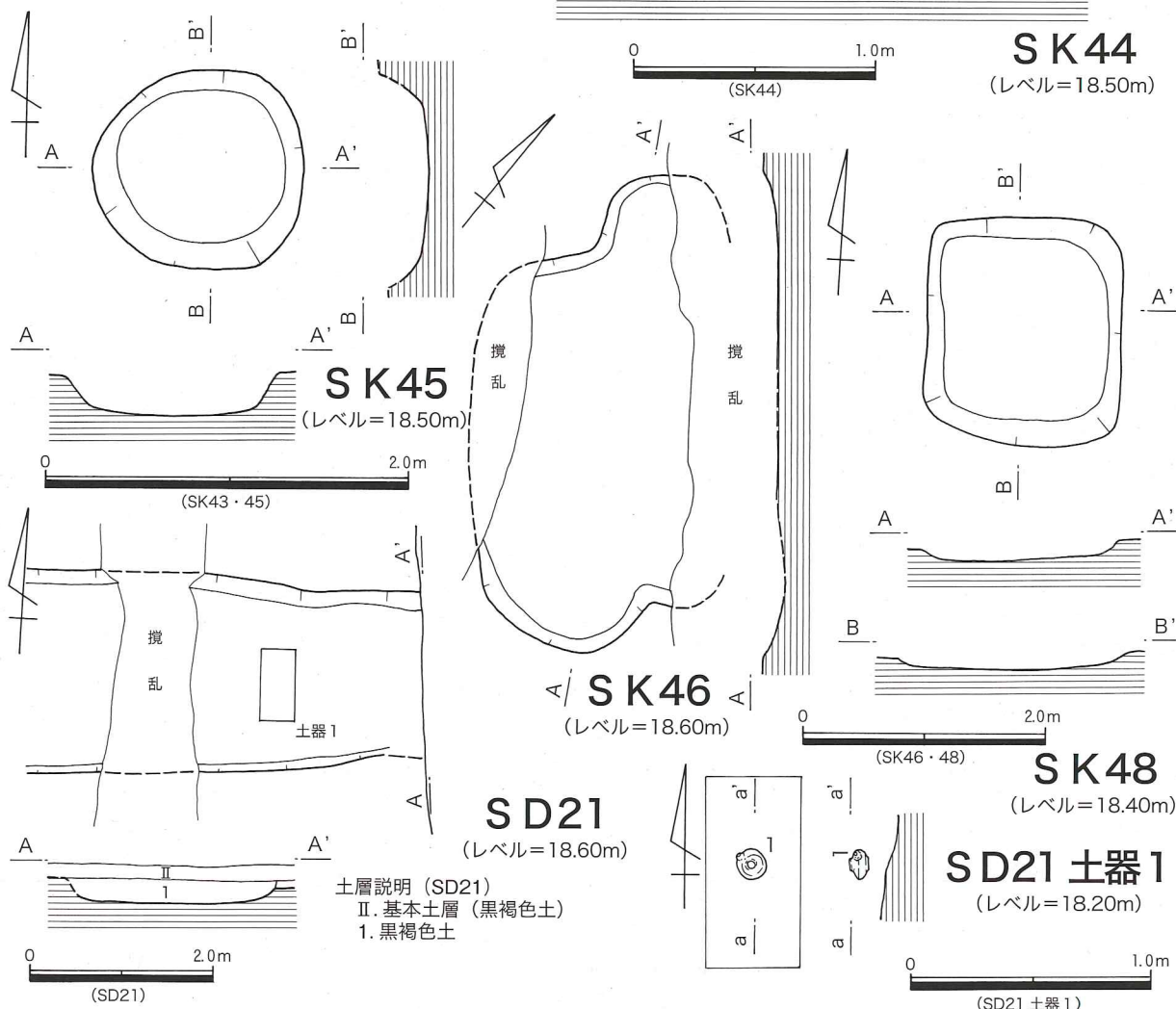
第197図 第54次 SK43～46・48、SD21実測図
