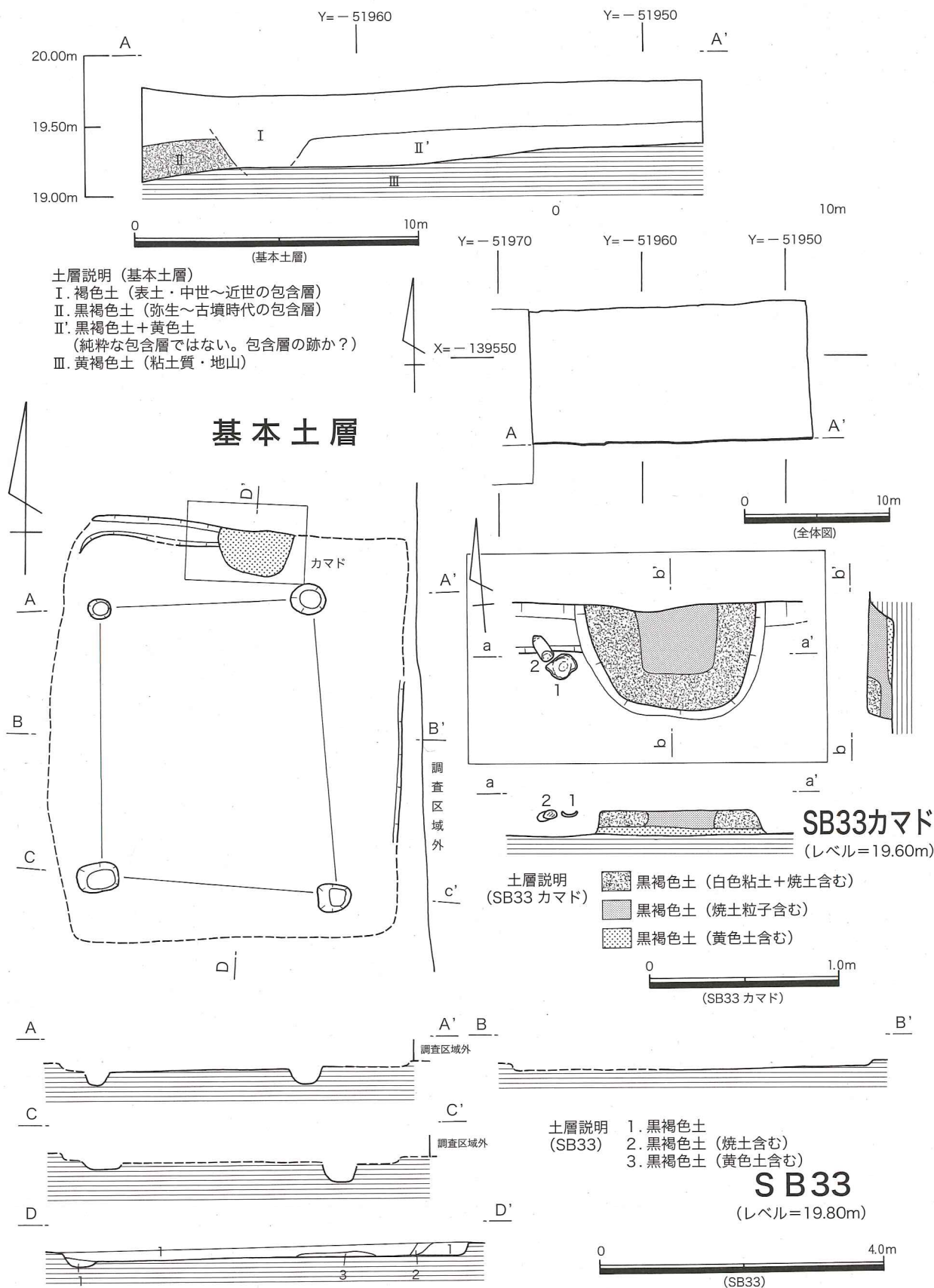
第159図 第50次 基本土層図、S B 33実測図
