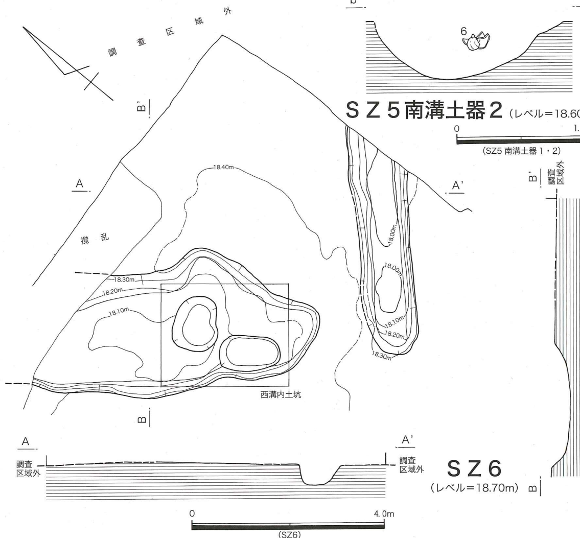
第207図 第55次 S Z 5土器出土状況図、S Z 6実測図
