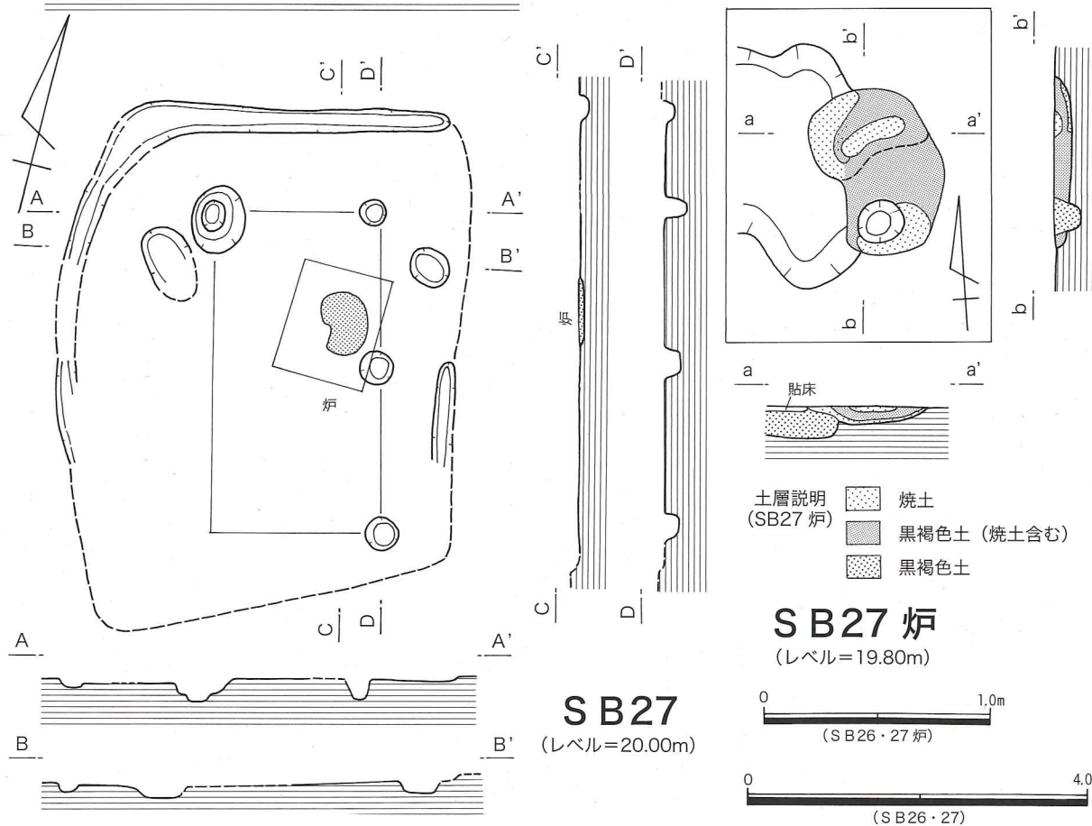
第140図 第49次 S B 26・27実測図
