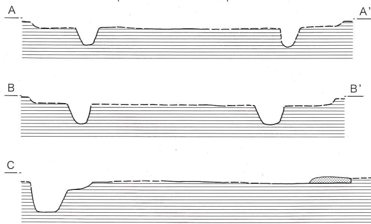
第204図 第55次 基本土層図、SB3実測図
