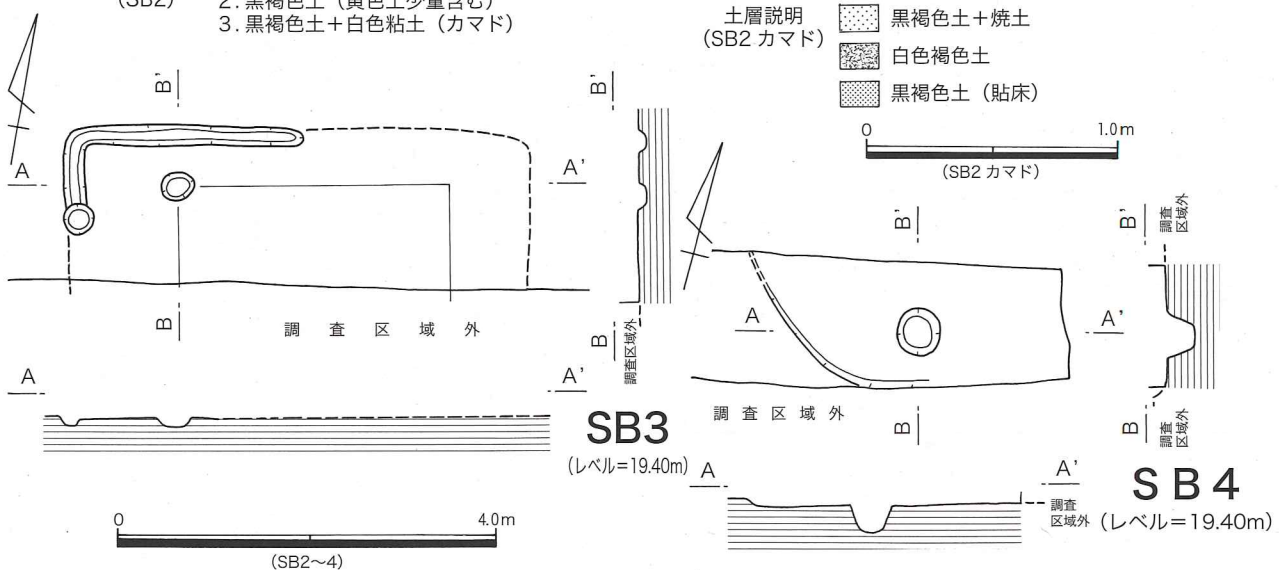
第170図 第52次 基本土層図、SB2～4実測図
