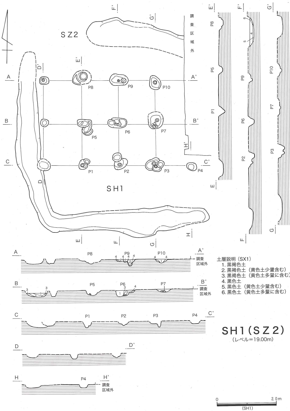
第186図 第53次 SH1 (SZ2) 実測図
