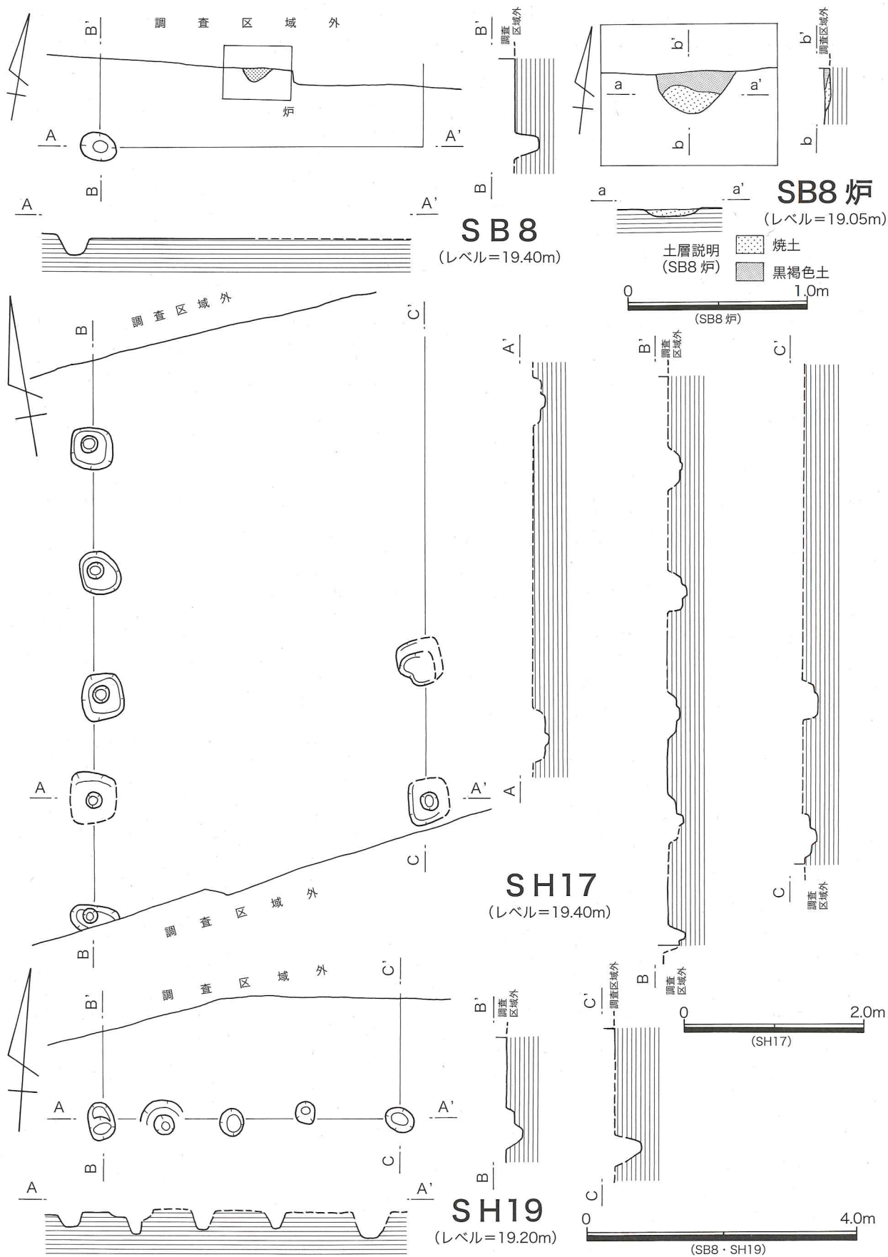
第172図 第52次 SB8、SH17・19実測図
