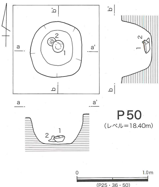
第188図 第53次 SK41・42、P25・36・50実測図、SD16土層図
