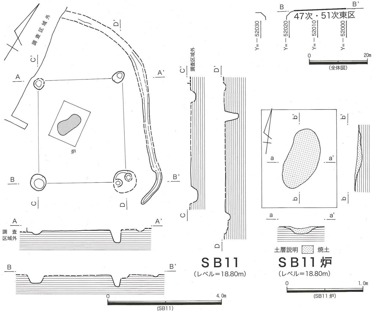
第121図 第47・51次 基本土層図、SB11実測図
