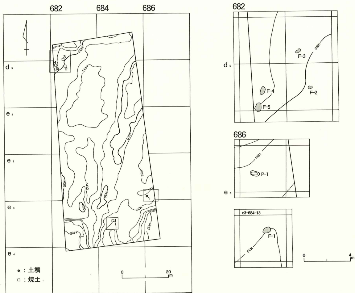
図Ⅻ-5 遺構位置図
