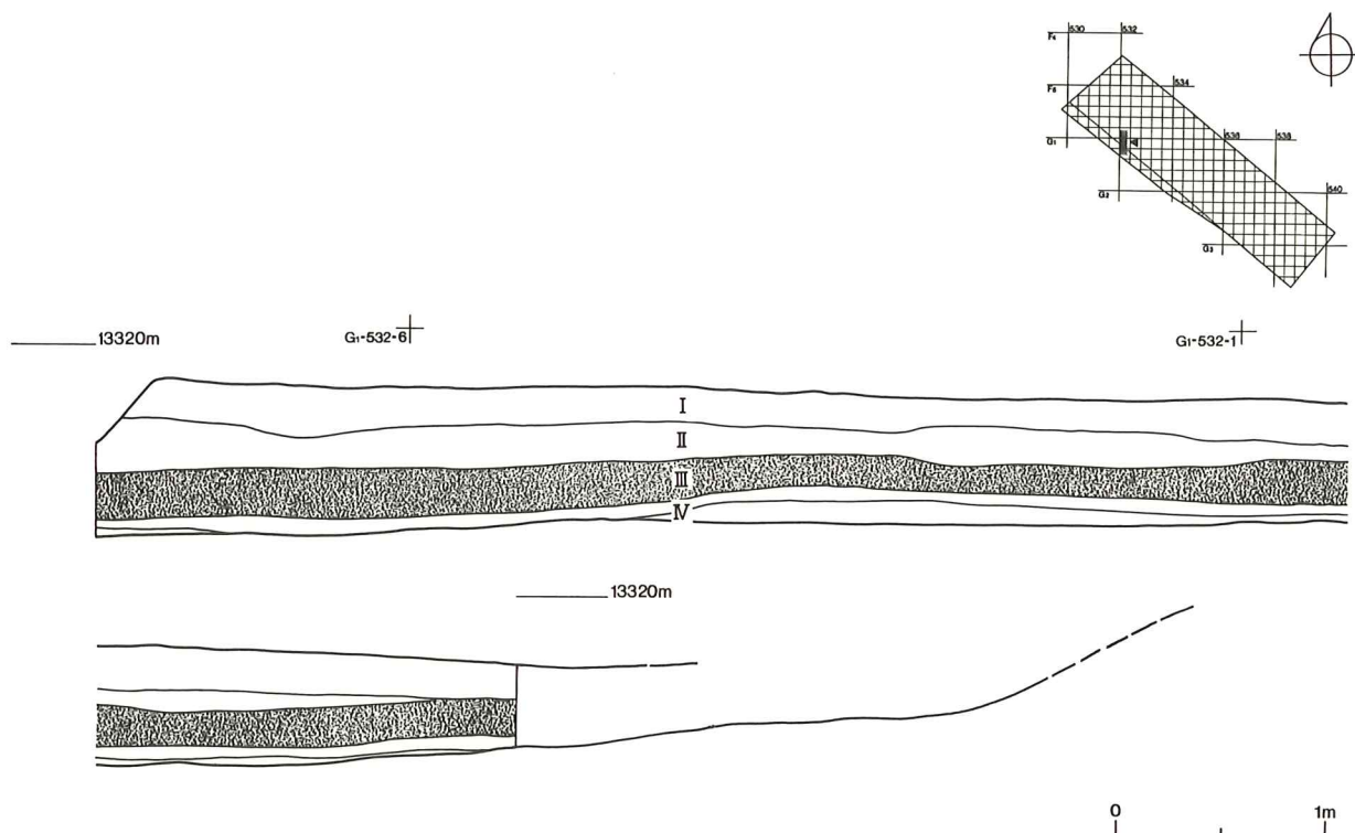
図Ⅶ-3 土層断面図
