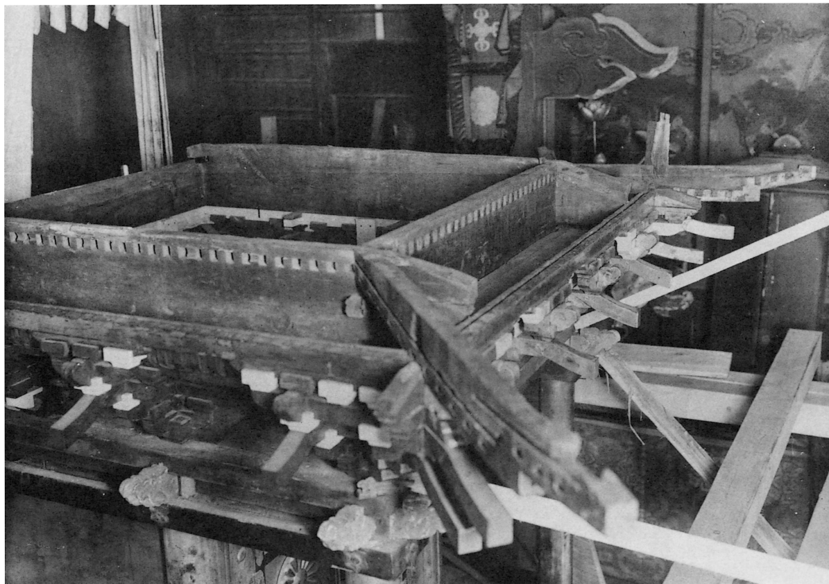
113 組立 桁廻
