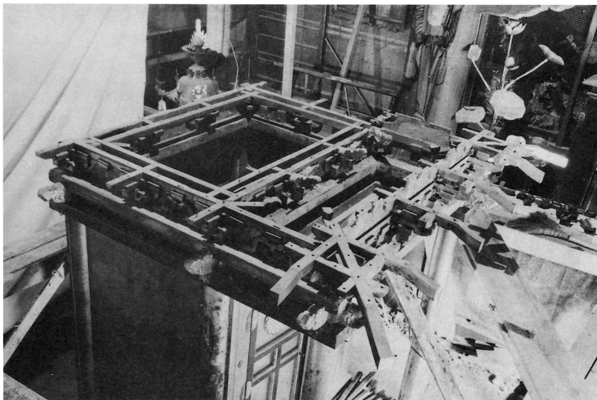
111 組立 斗拱
