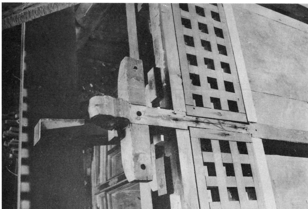
112 組立 軒天井、秤肘木、拳鼻の取合せ
