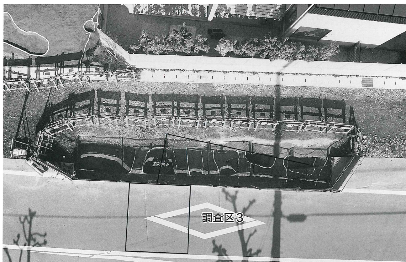
(2) 第56次調査区歩道区2空中写真全景 (奈良時代の大型掘立柱建物であるSH1の北側の柱列が検出された。上が北である。真上より。)
