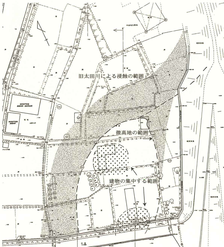
図12 西向遺跡 2次調査地の遺構状況 (S=1/1,000)
