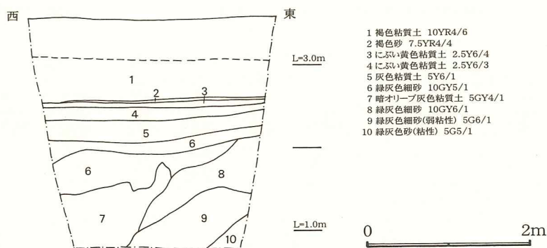
図13 1トレンチ土層断面図
