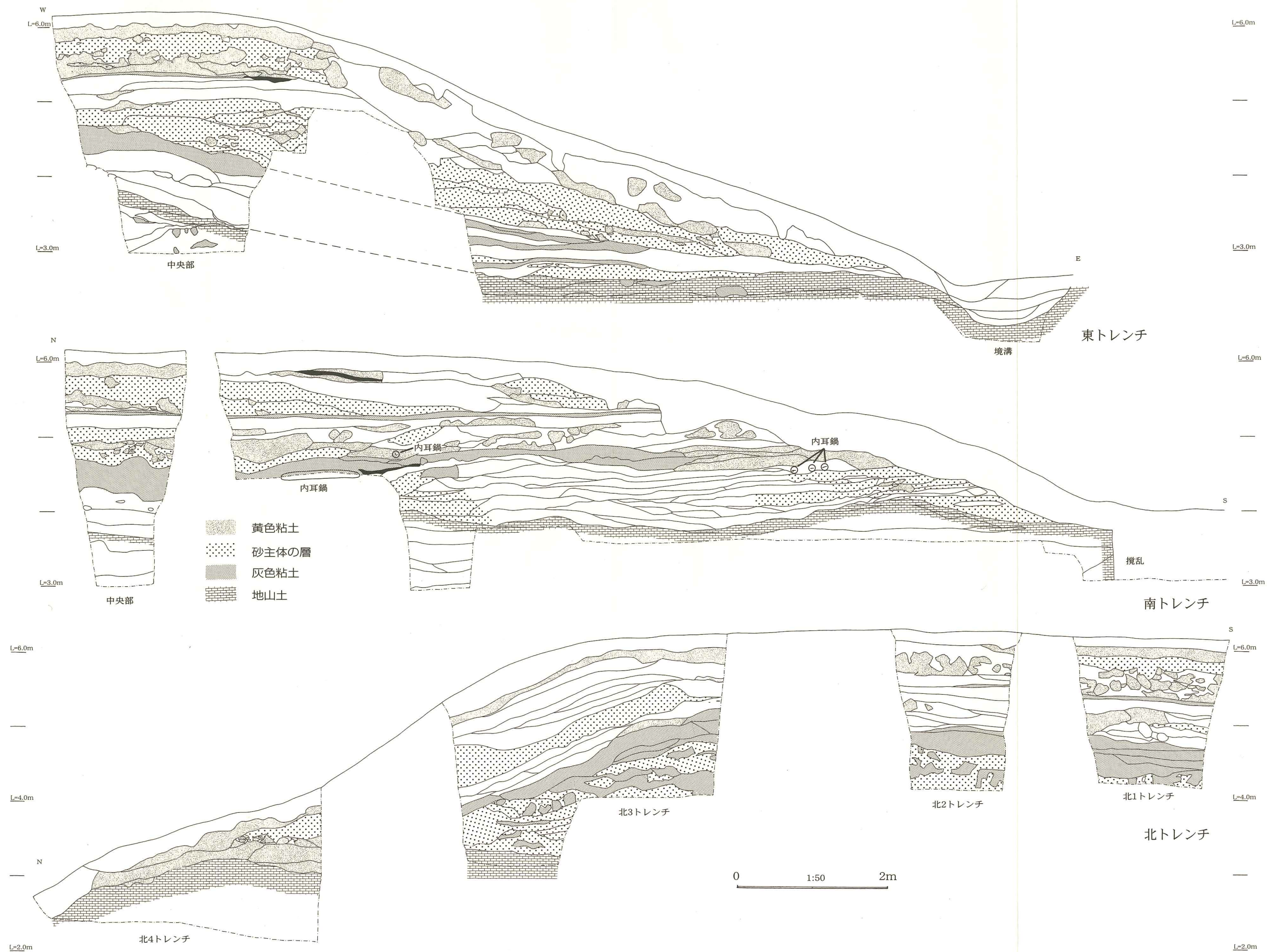
図28 大野命山土層断面図
