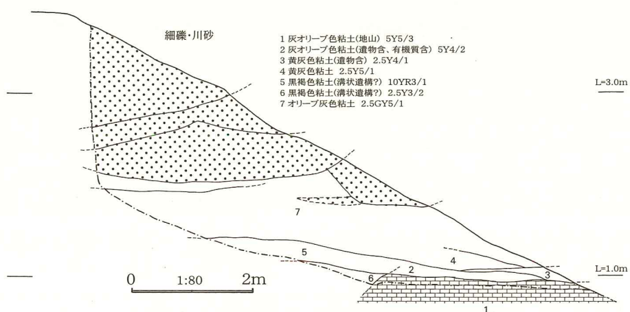
図5-2 西向遺跡試掘調査概要図・断面図
