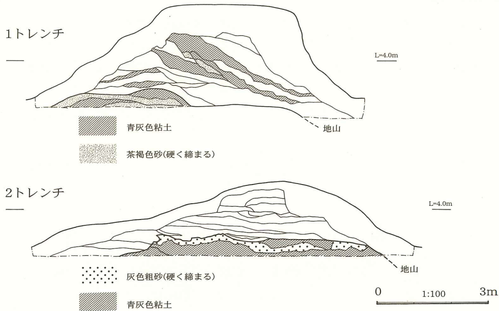
図22 富里旧堤防 2次調査土層断面図
