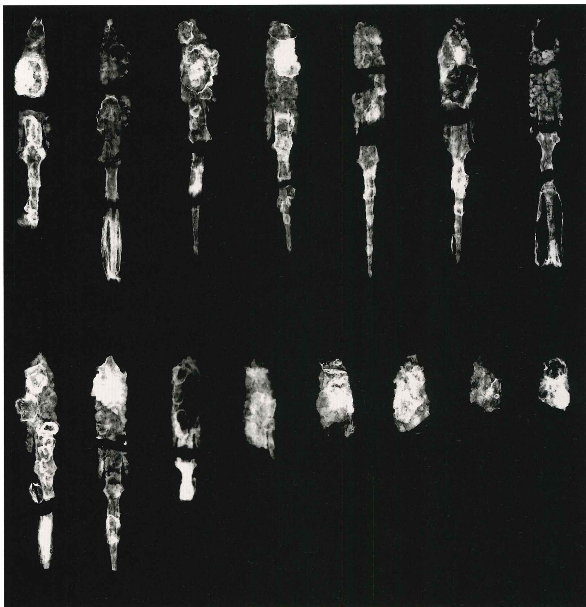
A類鉄鏃 (2) X線写真
