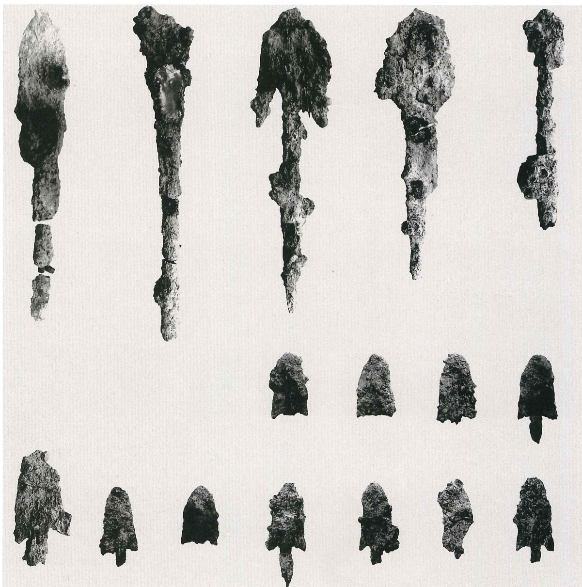
1 B・C類鉄鏃 保存処理前
