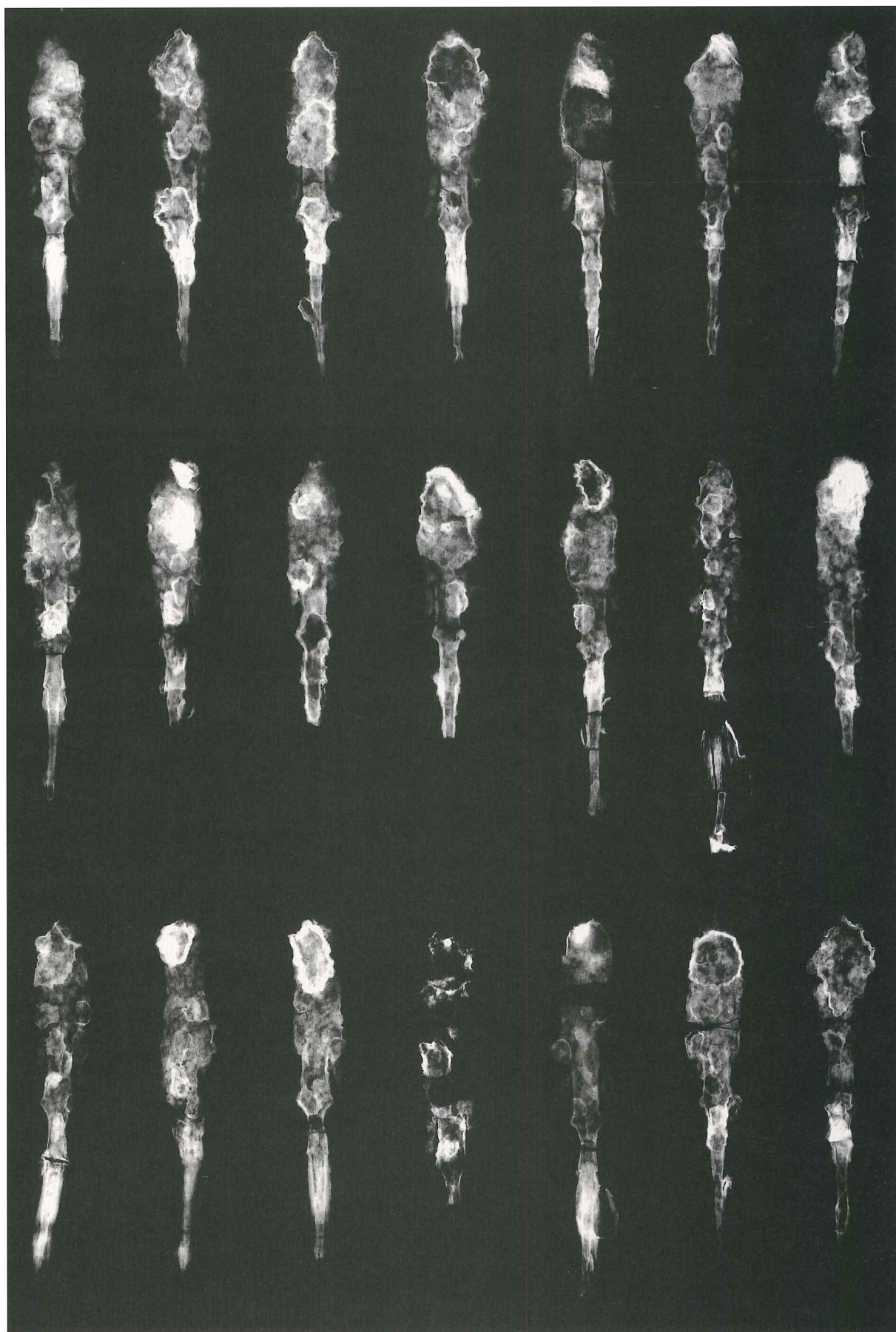
A類鉄鏃 (1) X線写真
