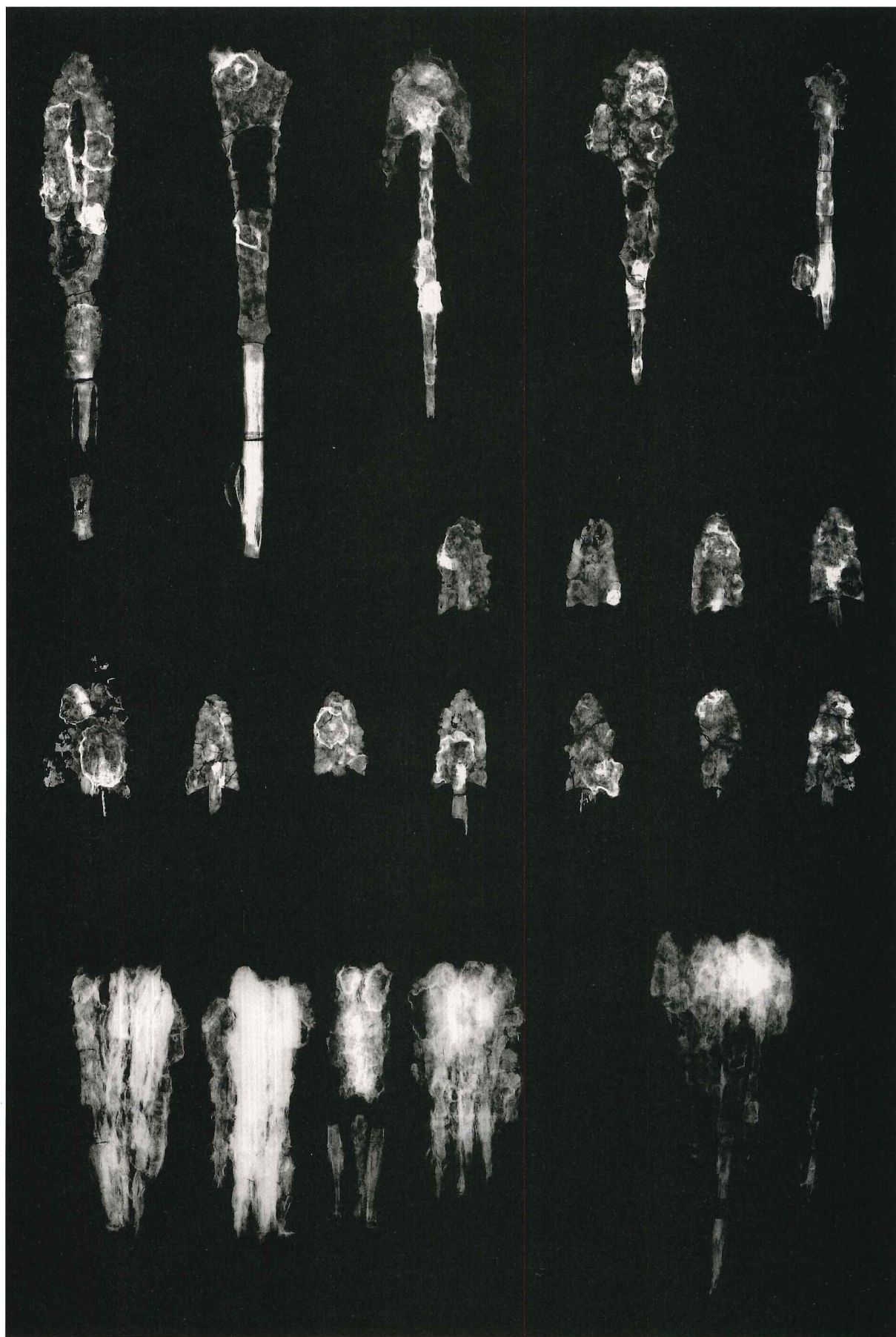
B・C類鉄鏃他 X線写真
