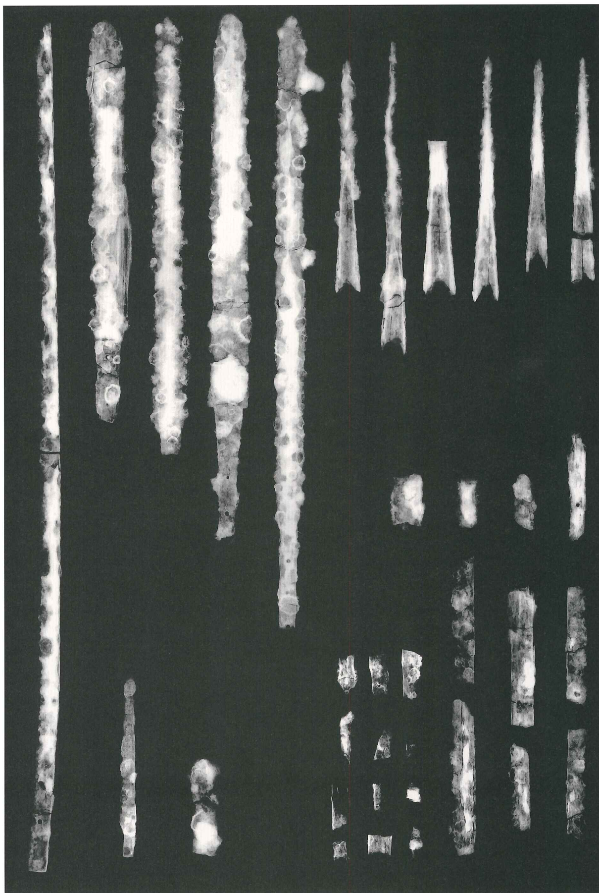
刀・剣・槍・鉾 X線写真
