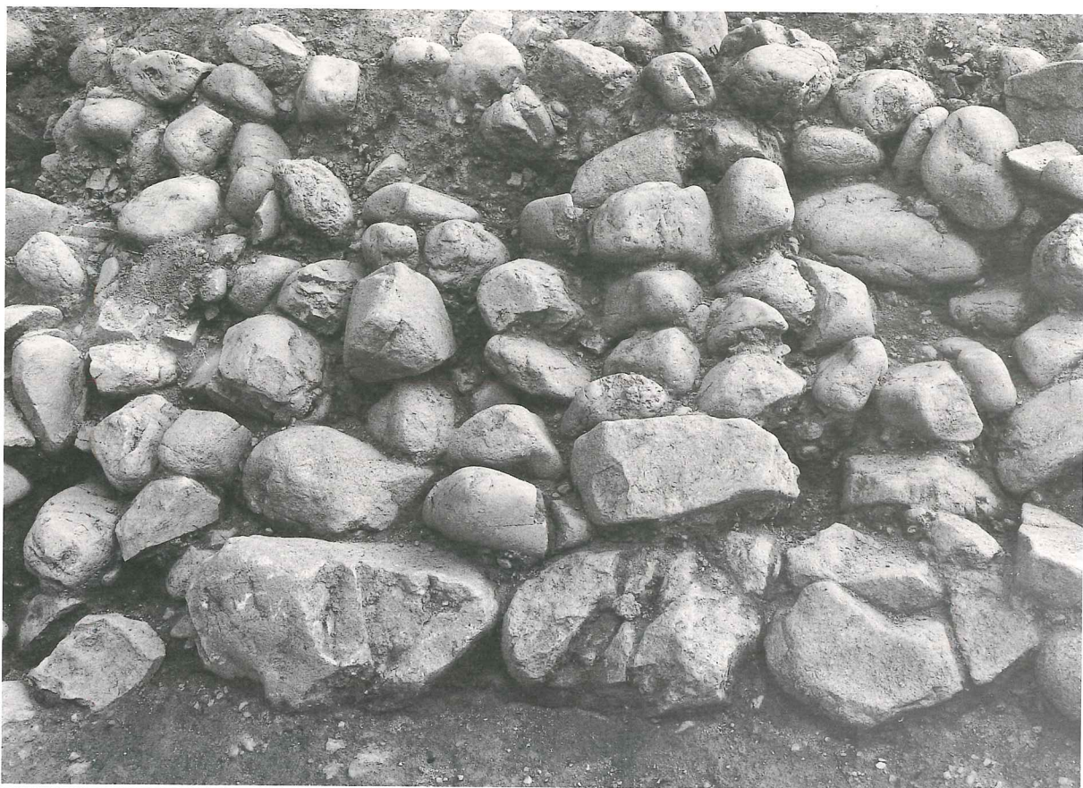
2 北側上段斜面 葺石基底石（北から）
