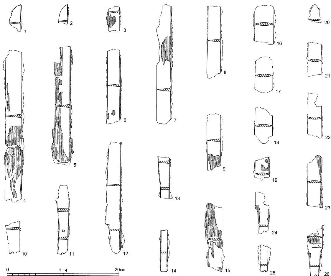
図55 攪乱出土刀剣類実測図
