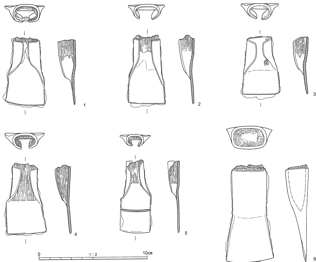
図32 斧実測図
