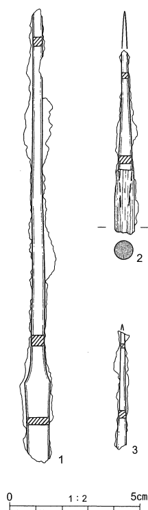
図35 錐実測図
