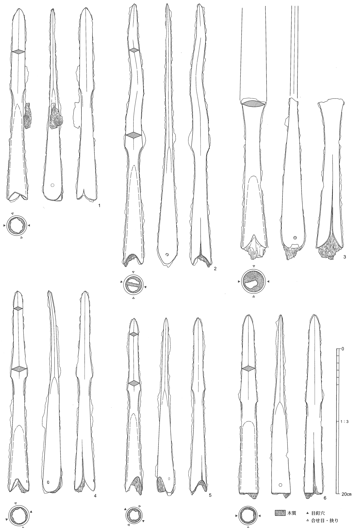
図47 鉾実測図
