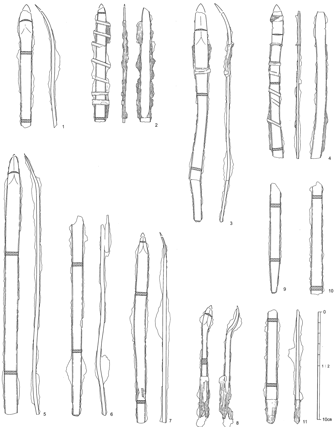
図33 鉋実測図
