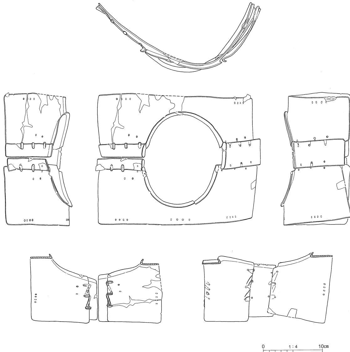
図44 頸甲実測図
