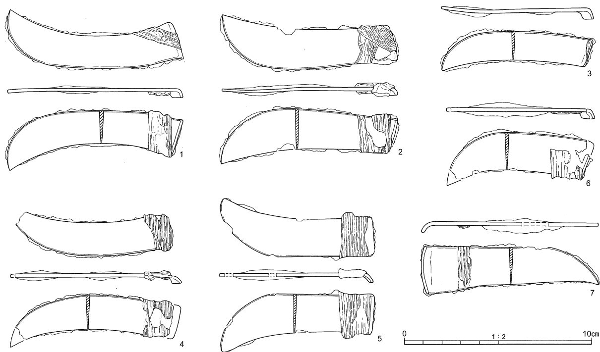
図29 鎌実測図
