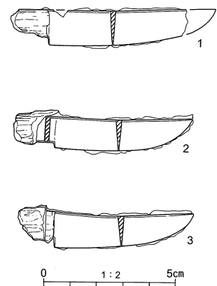
図31 刀子実測図
