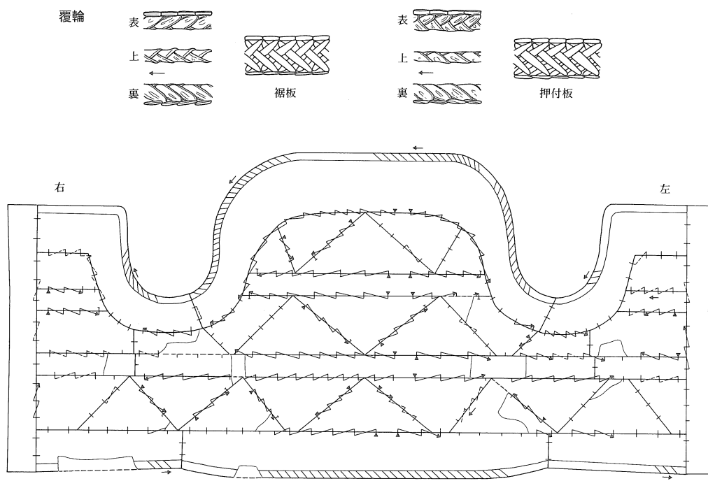
図37 短甲模式図
