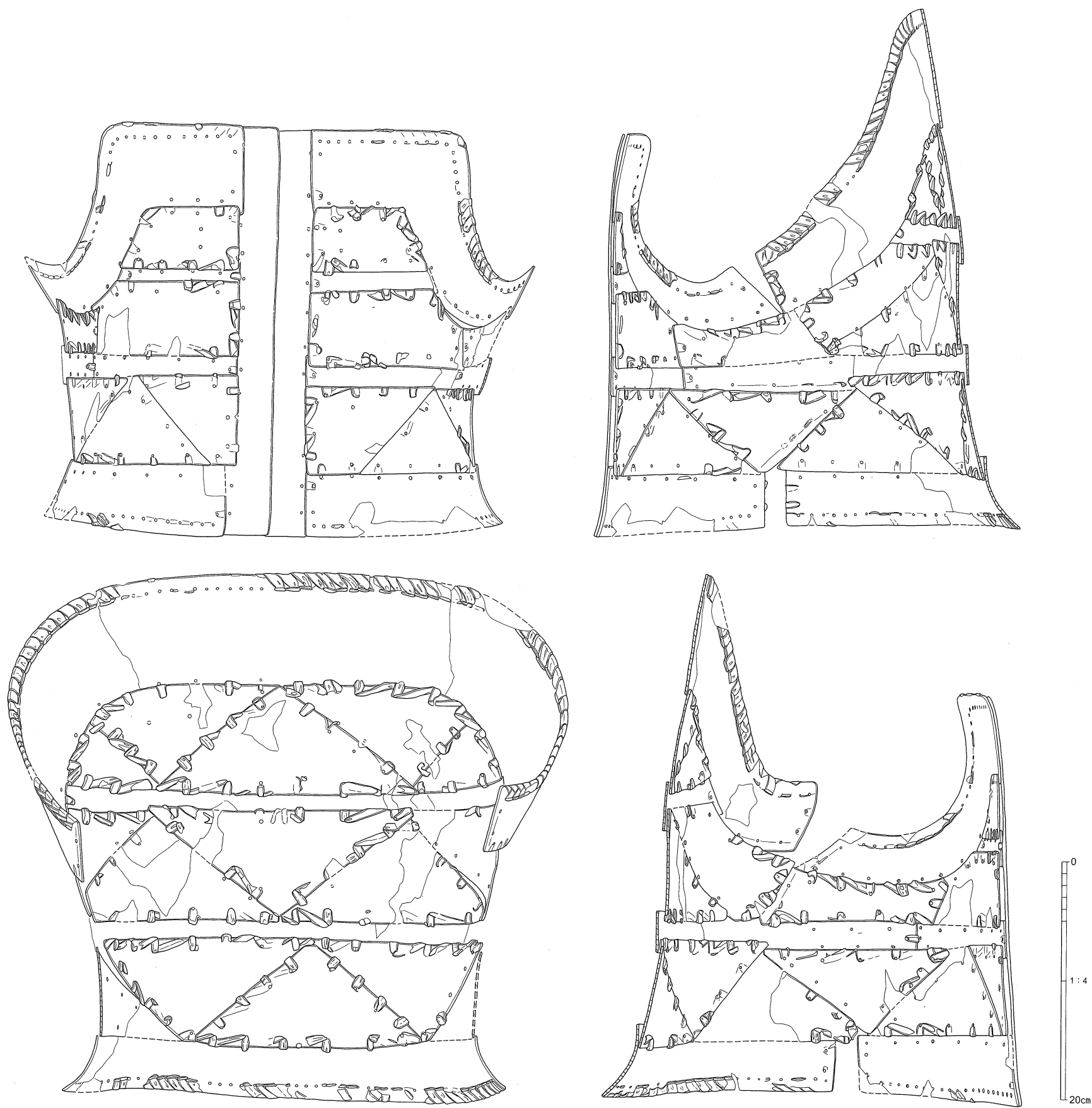
图39 短甲实测图 (内面)
