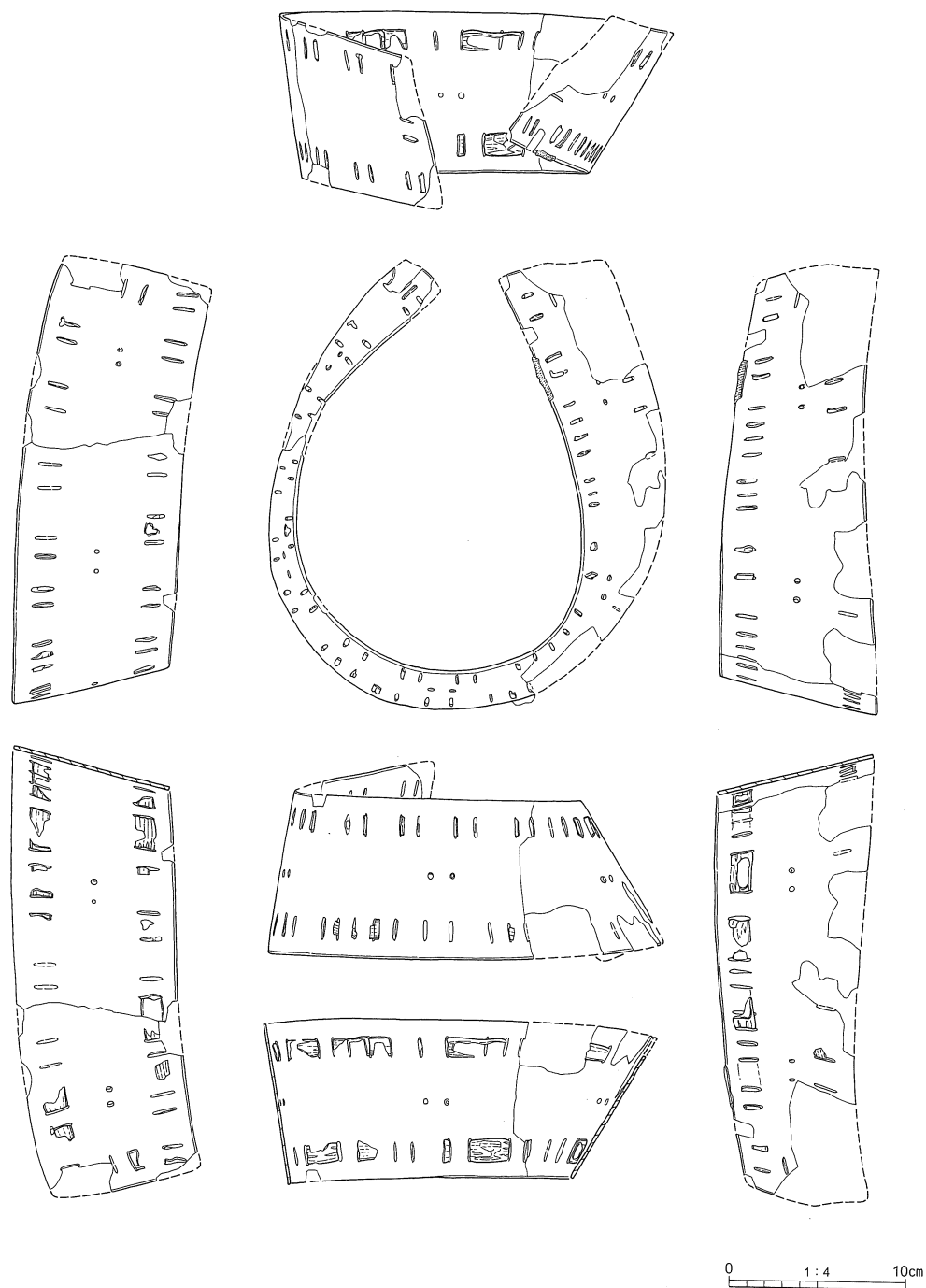
図43 板鋳実測図
