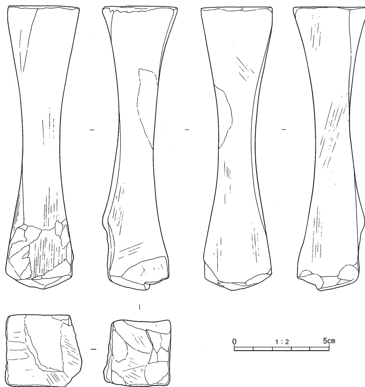
図28 砥石実測図
