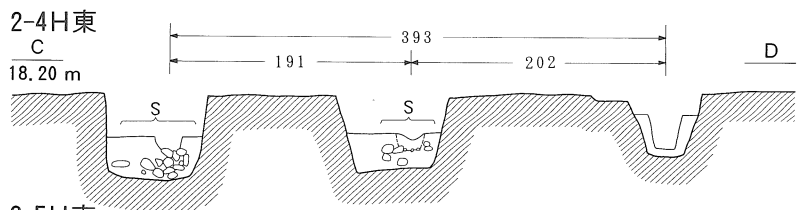
図版53 遺構断面図 2 (1:60)
