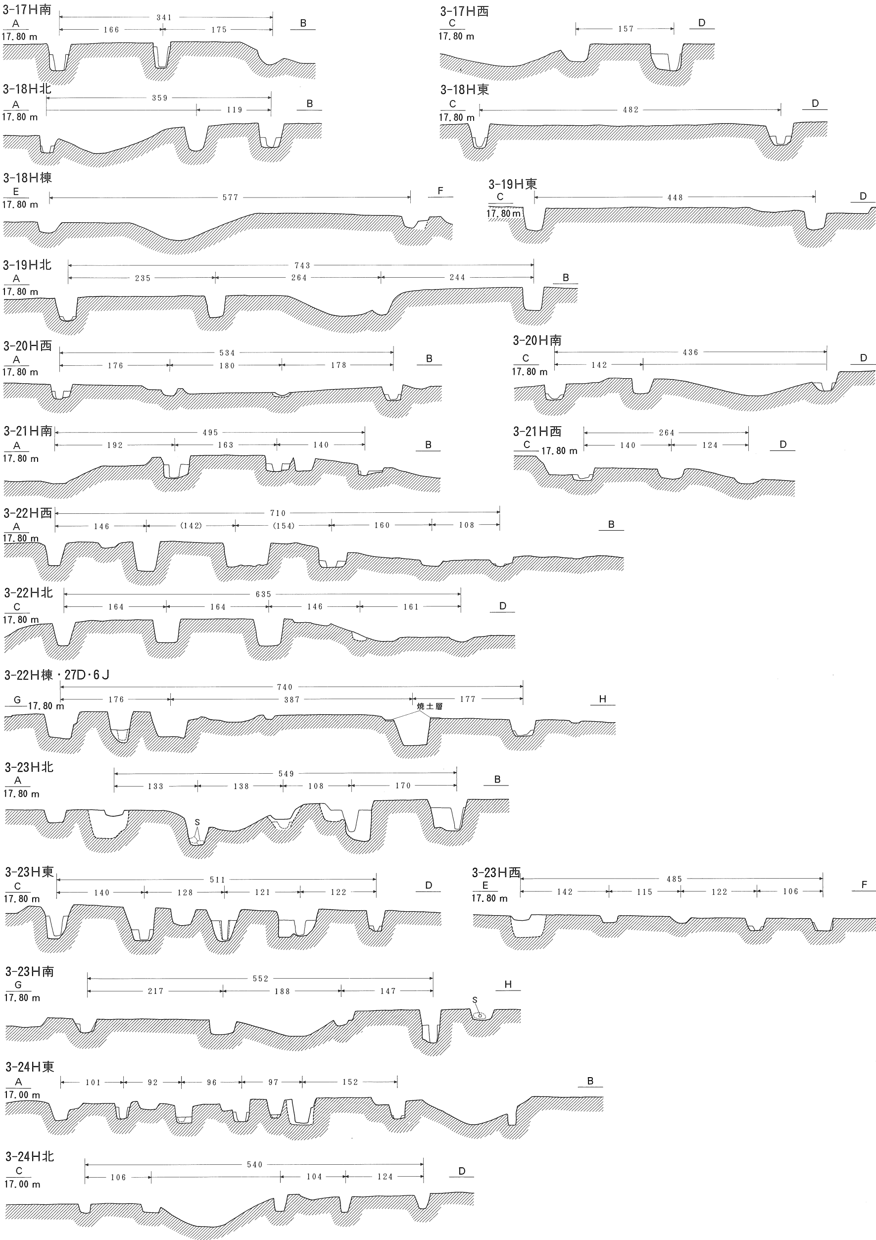
図版56 遺構断面図 5 (1:60)
