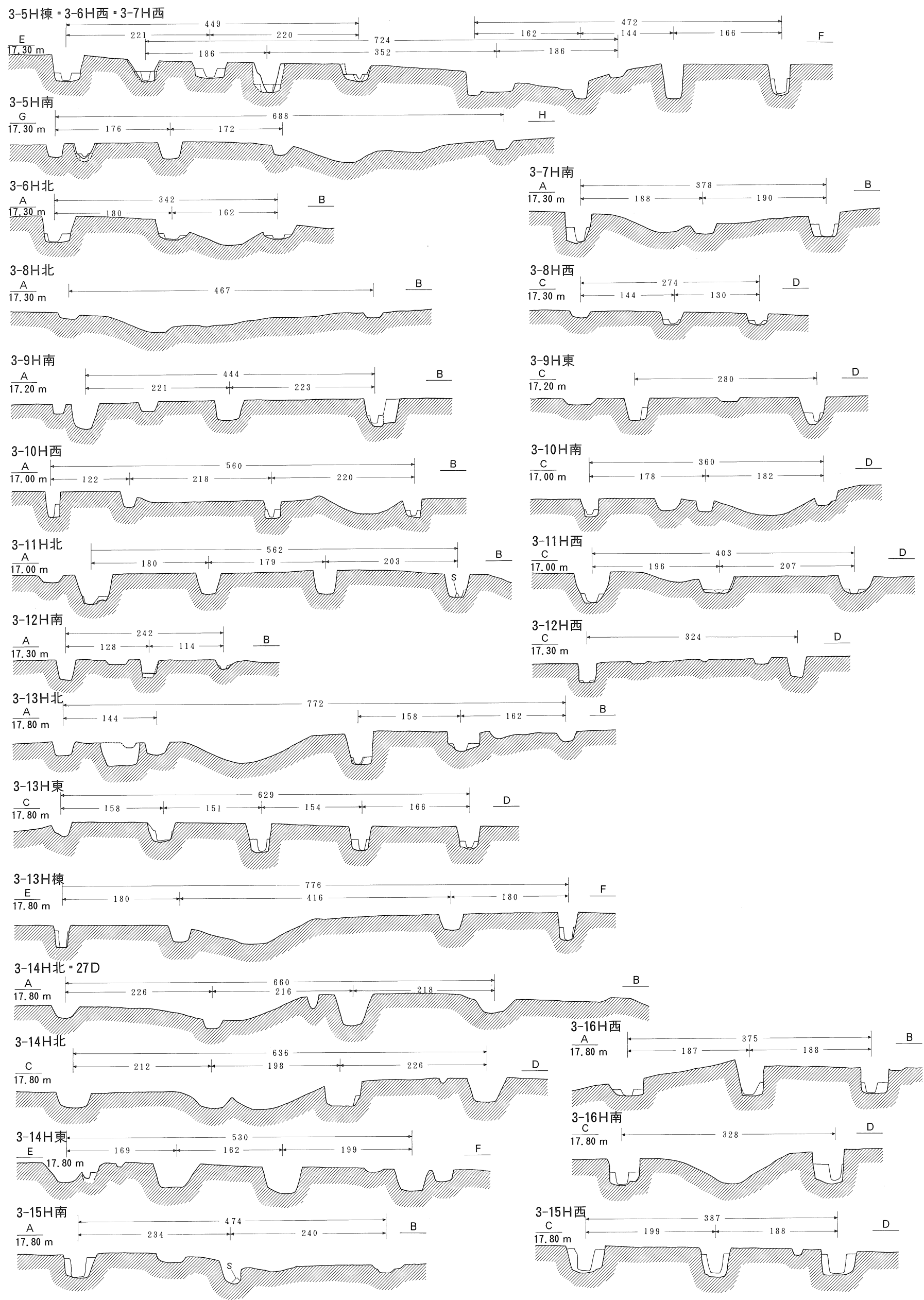
图版55 遺構断面図 4 (1:60)
