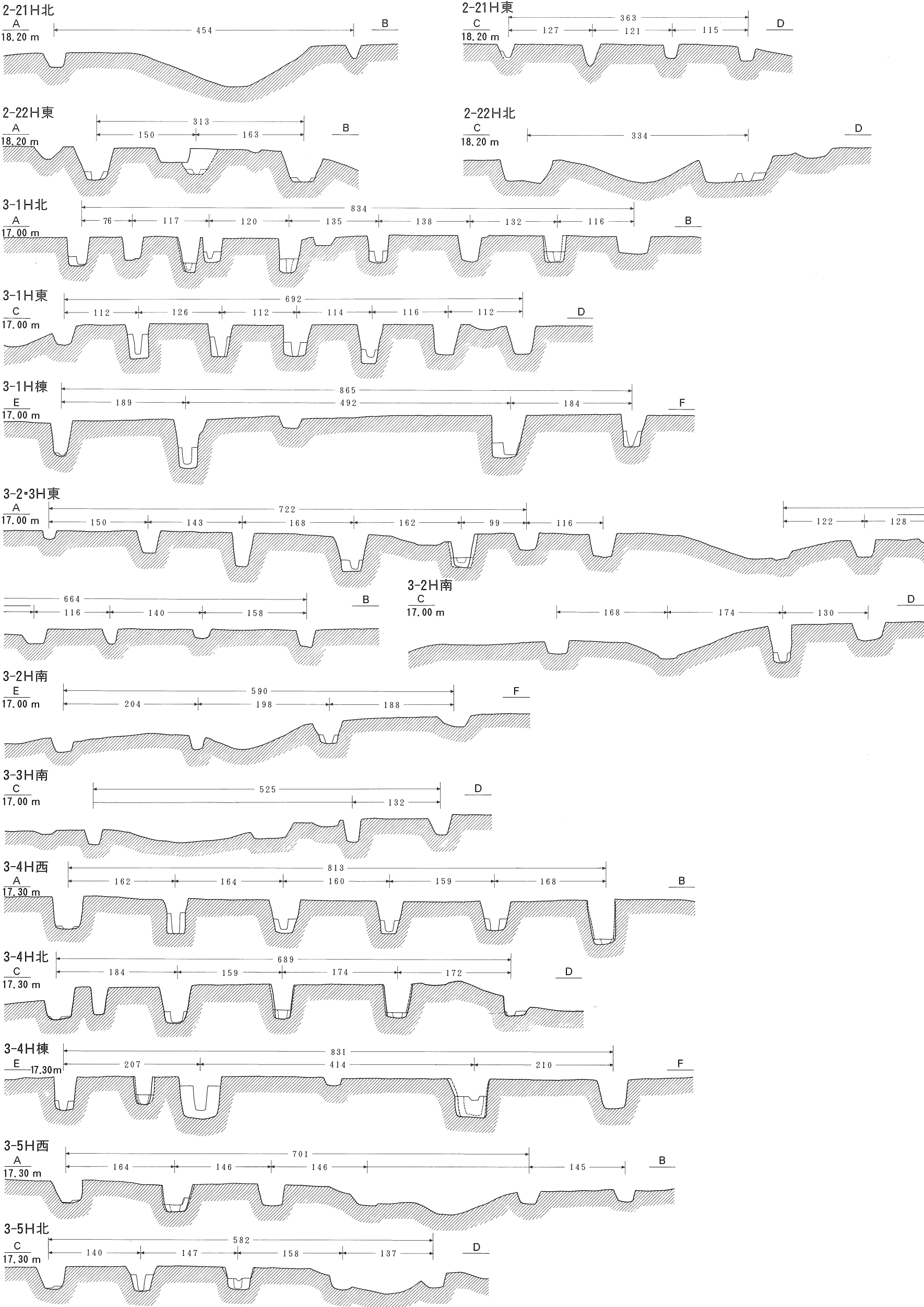
図版54 遺構断面図 3 (1:60)
