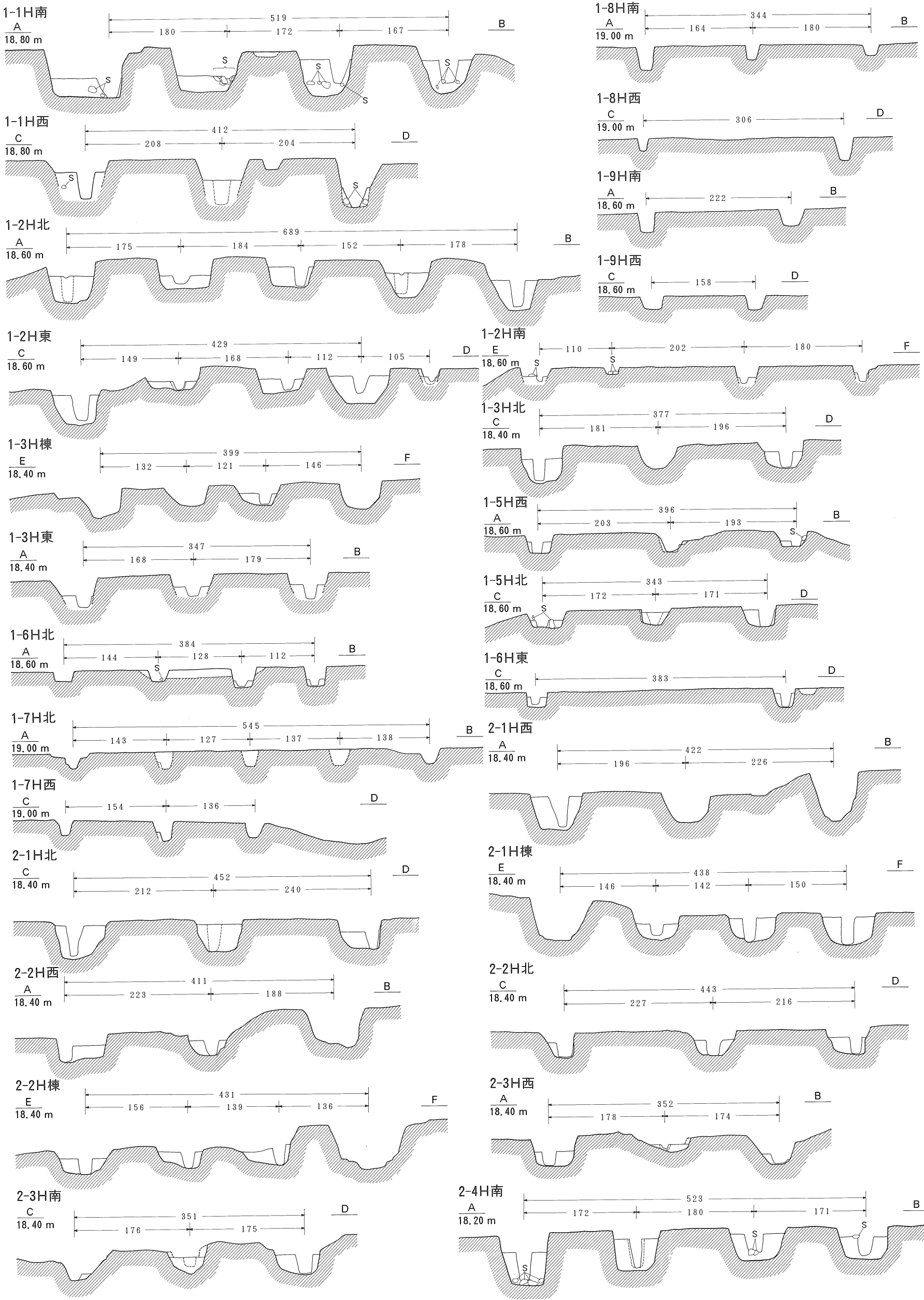
图版52 遺構断面図1 (1:60)
