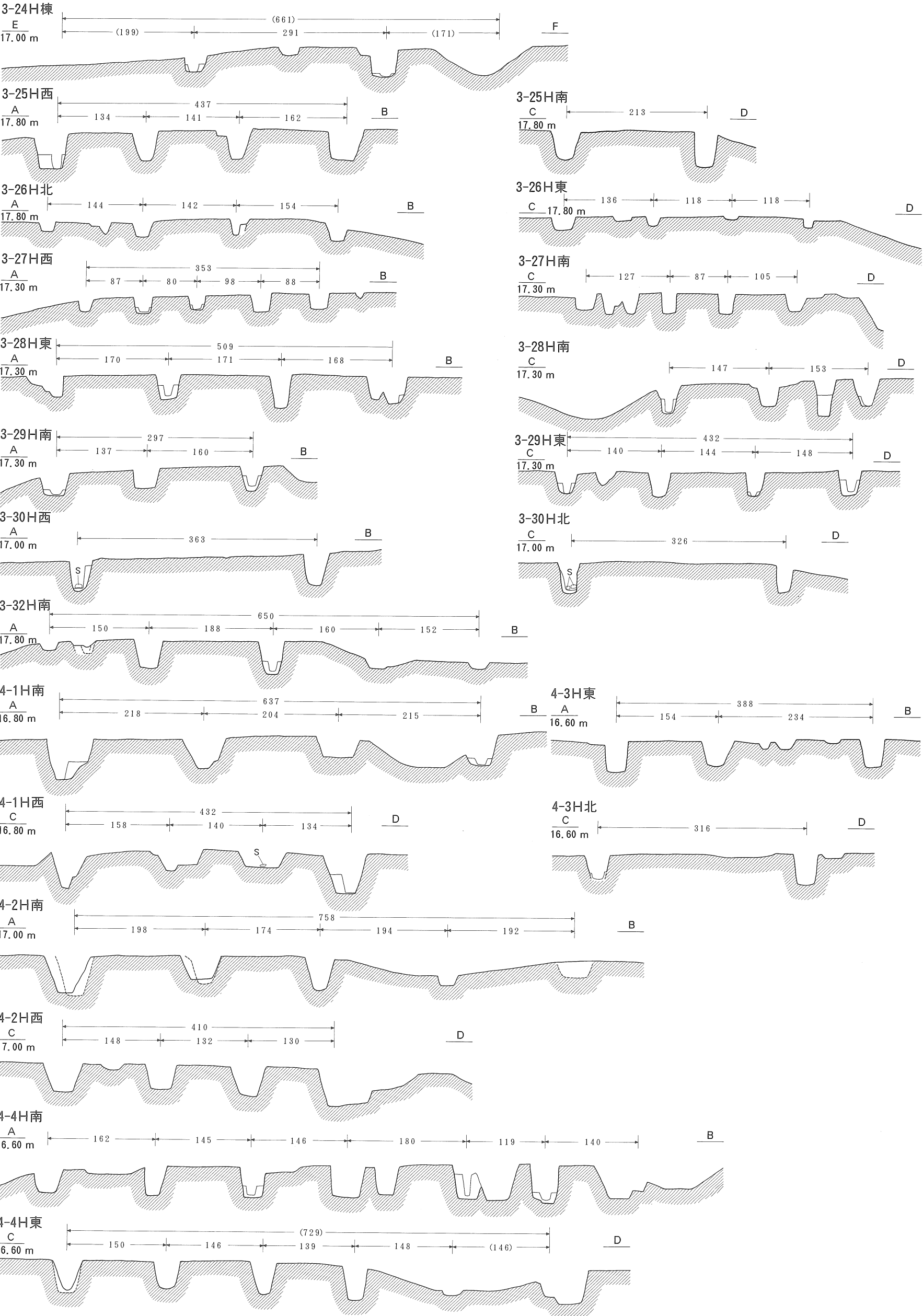
図版57 遺構断面図 6 (1:60)
