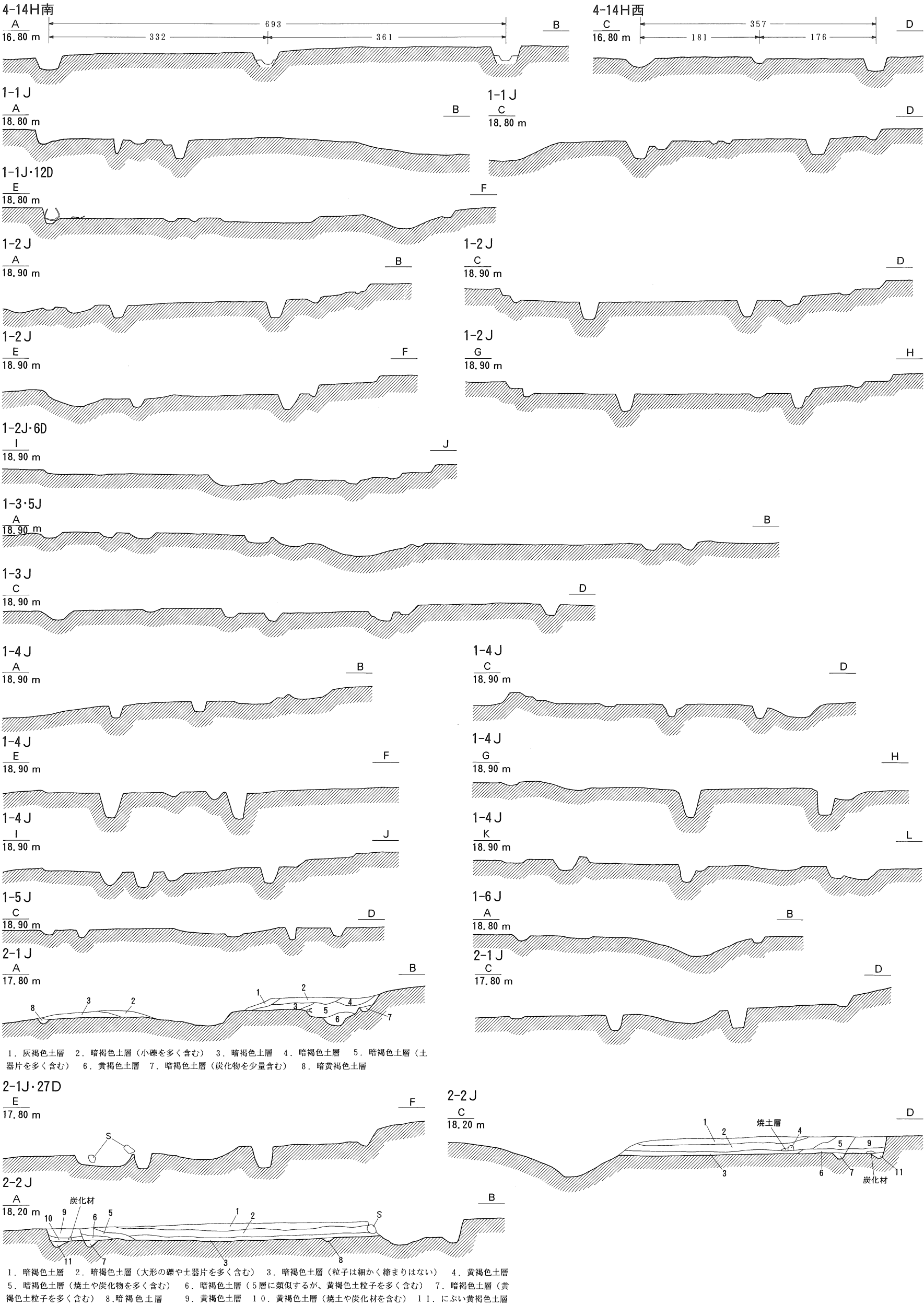
図版59 遺構断面図 8 (1:60)
