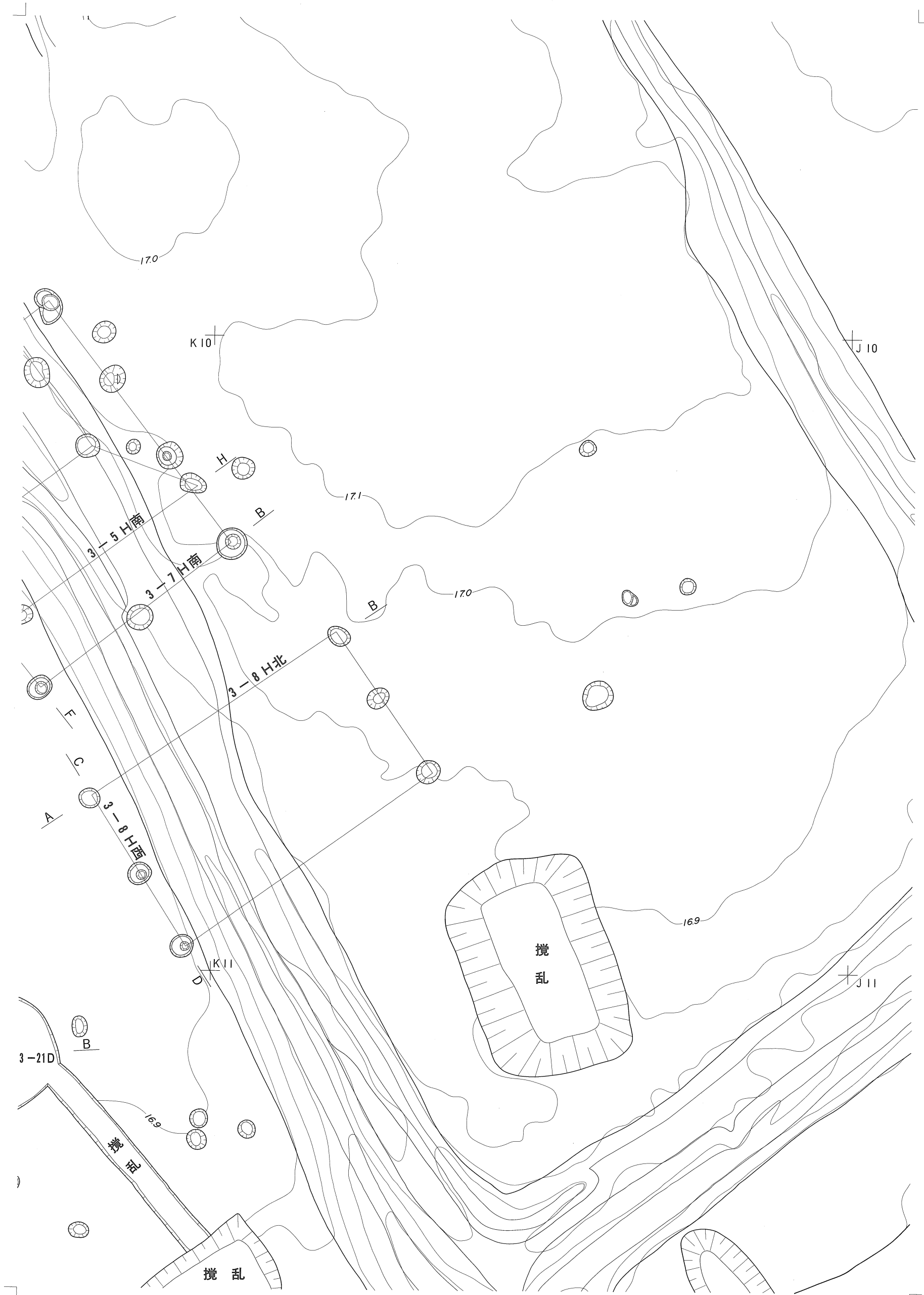
图版38 遺構平面図36 (1:60)
