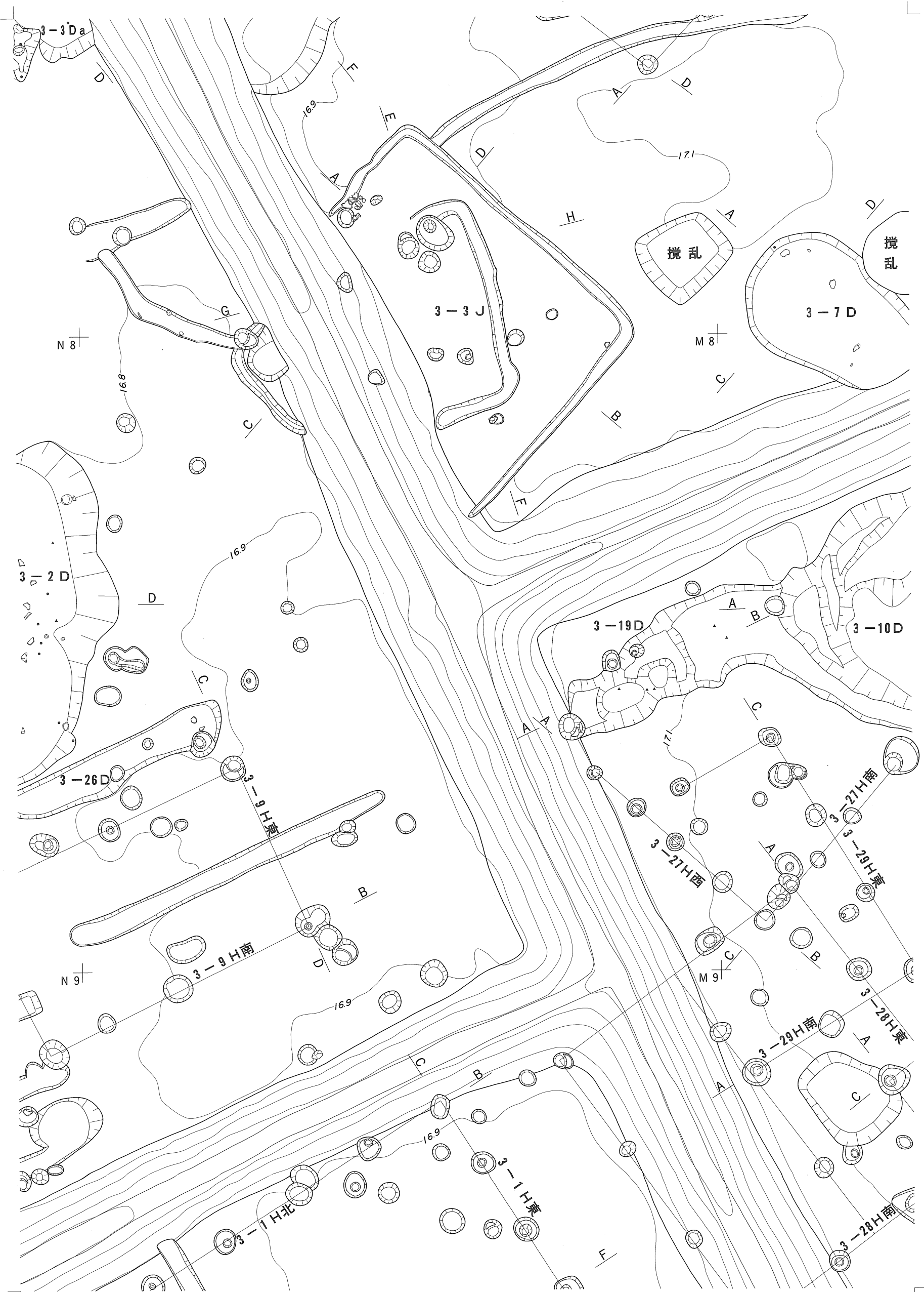
图版32 遺構平面図30 (1:60)
