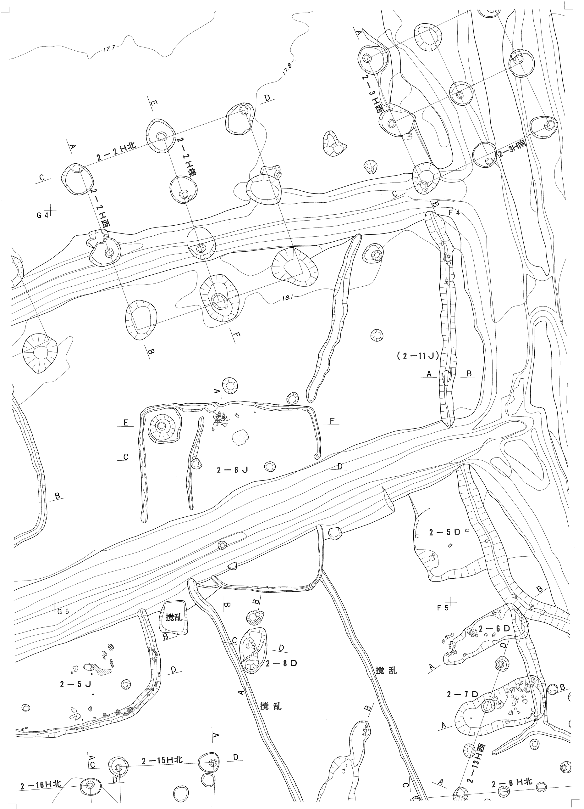
図版12 遺構平面図10 (1:60)
