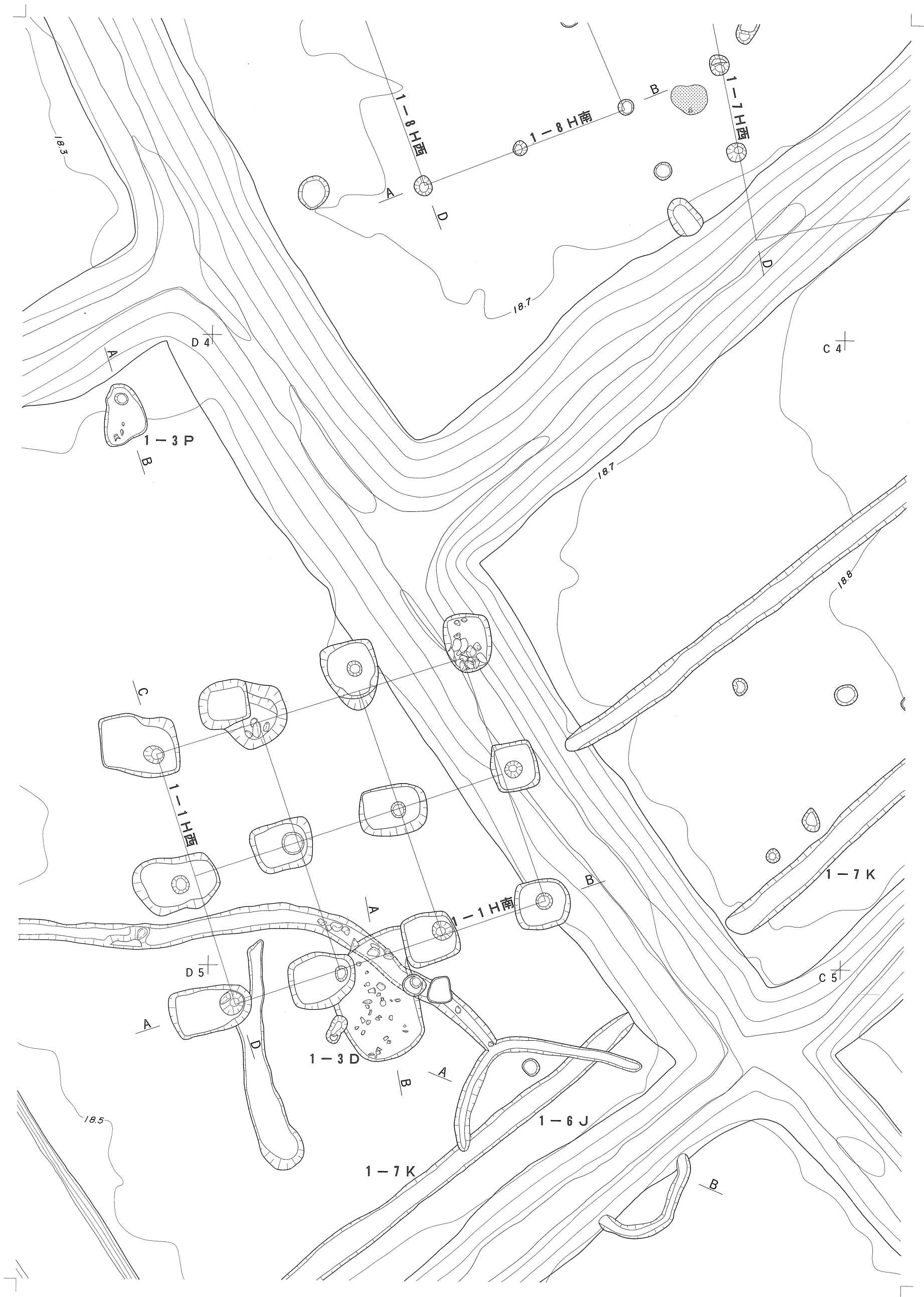
图版10 遺構平面図 8 (1:60)
