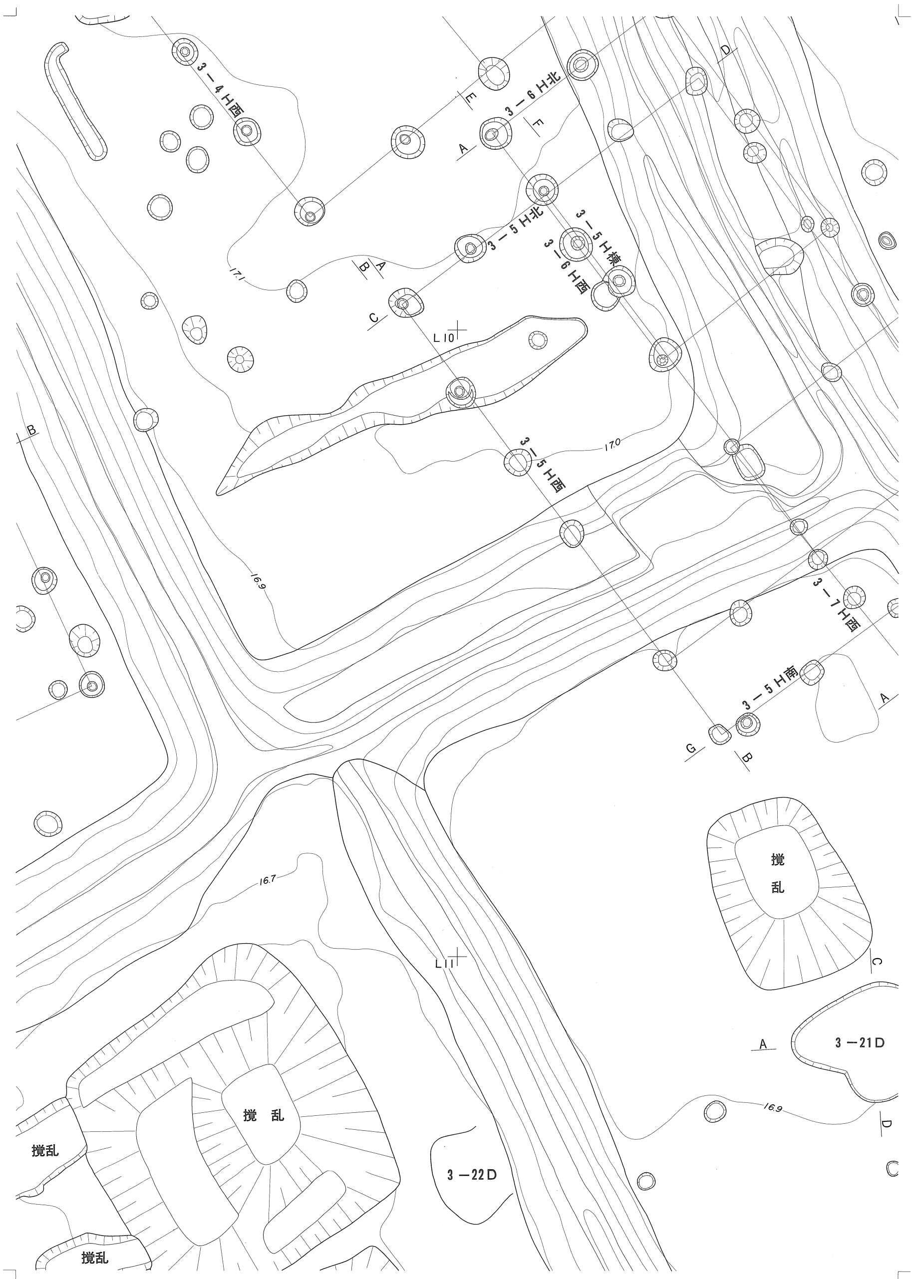
图版39 遺構平面図37 (1:60)
