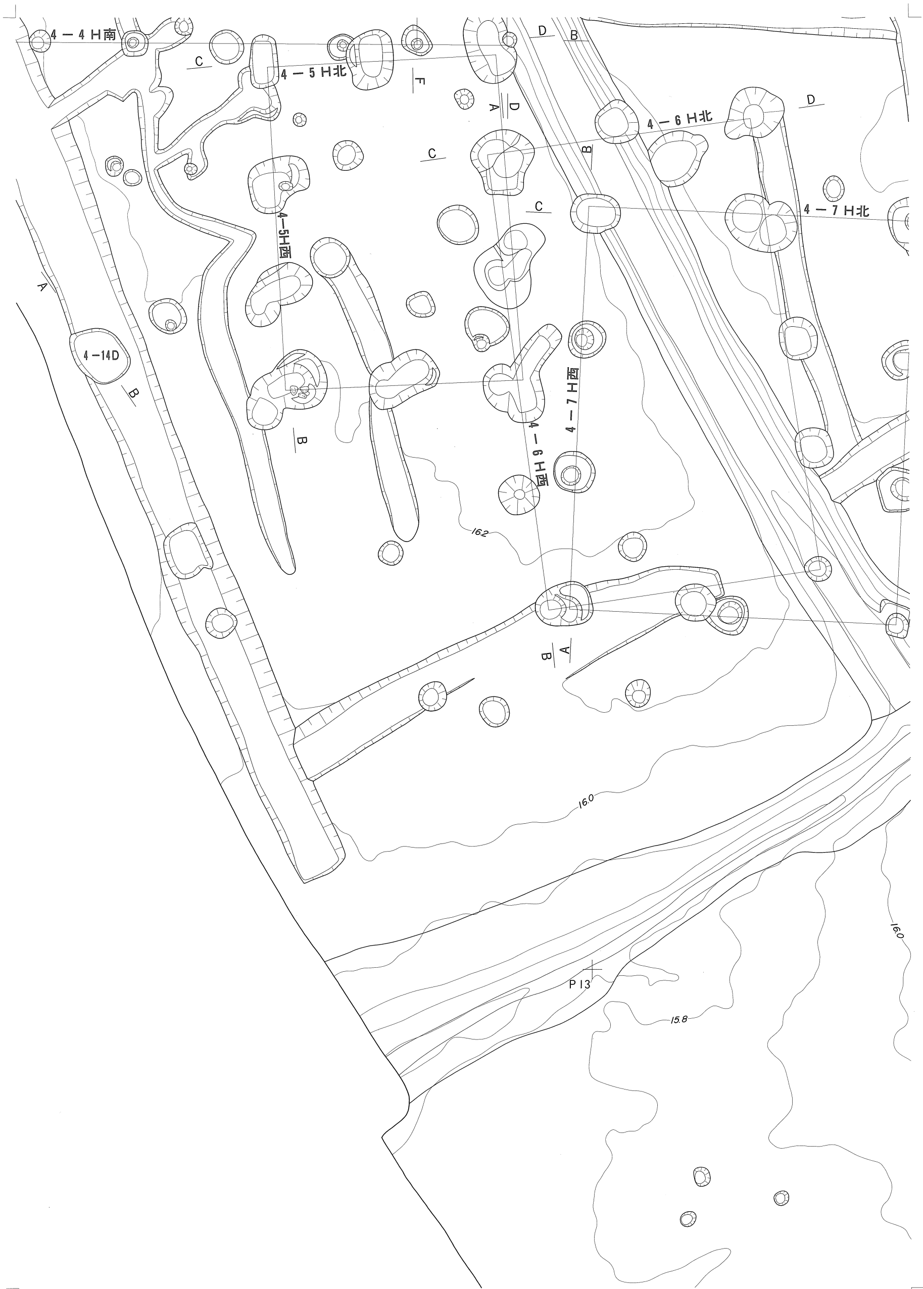
图版49 遺構平面図47 (1:60)
