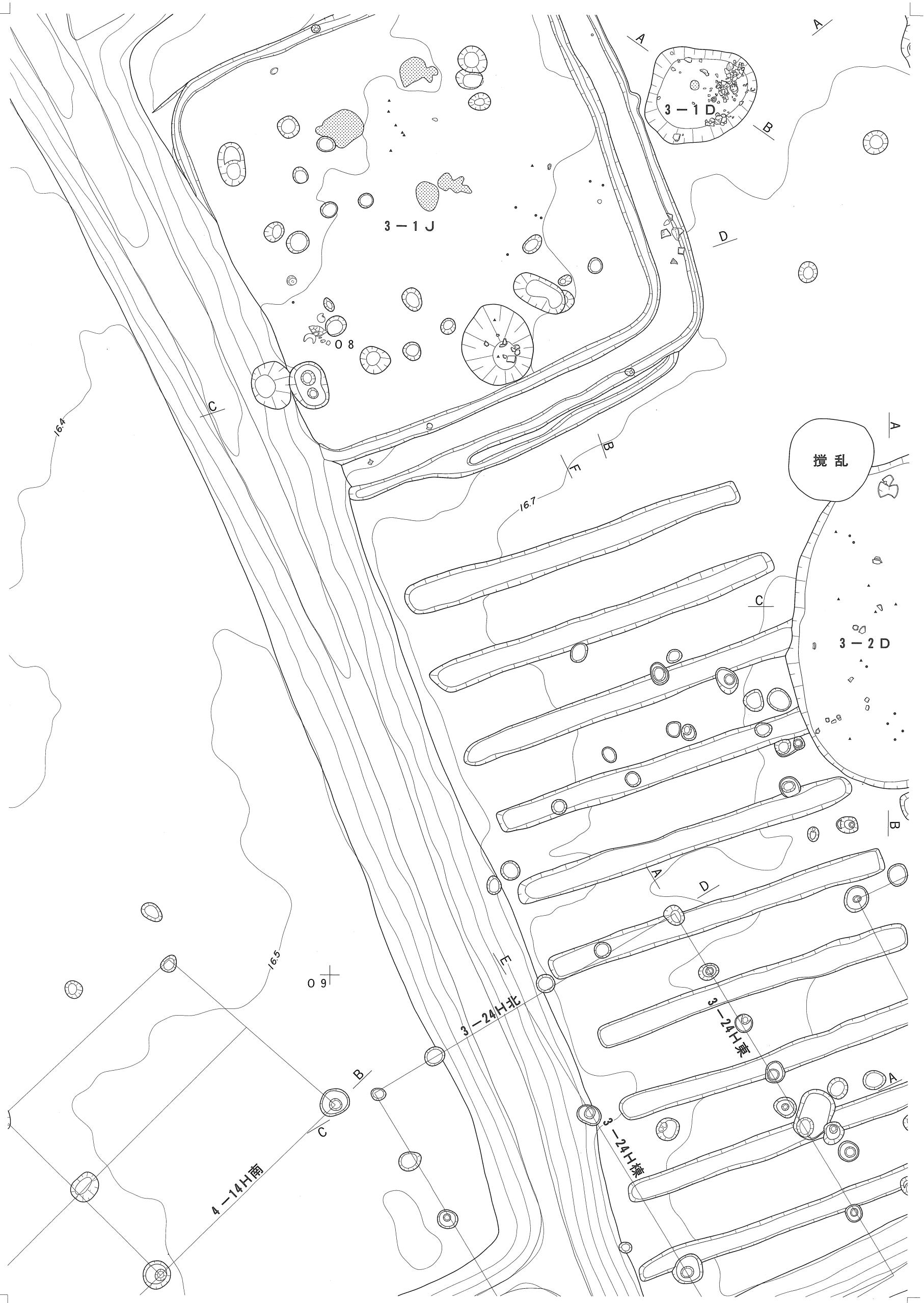
図版33 遺構平面図31 (1:60)
