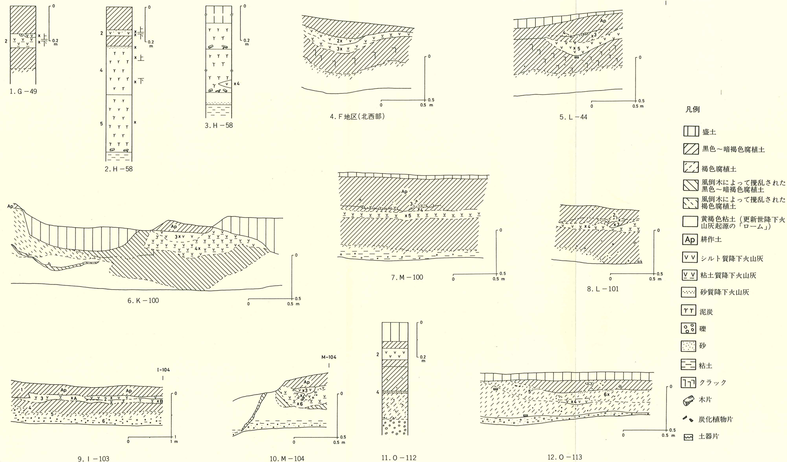
図IX-1 火山灰の産状を示す土層断面図と柱状図
