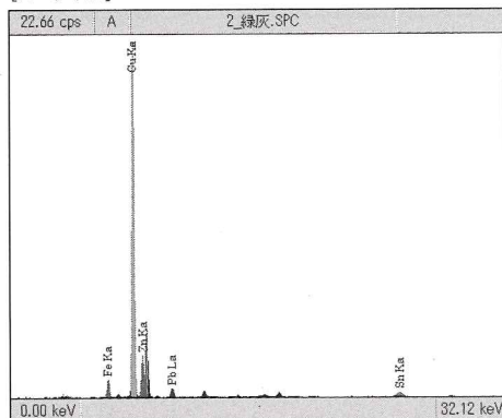
1 耳環A部分のXRFスペクトル
