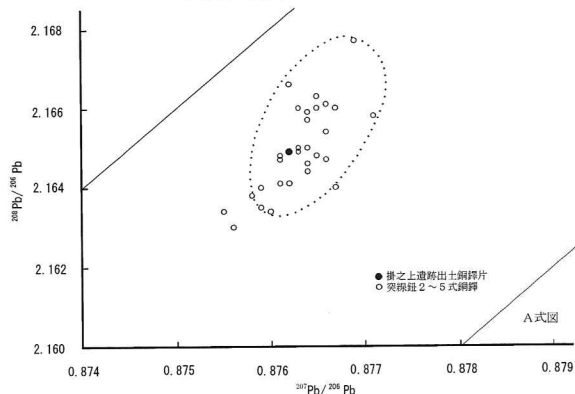
5 掛之上遺跡出土銅鐸片と突線鈕2~5式銅鐸の鉛同位体比
