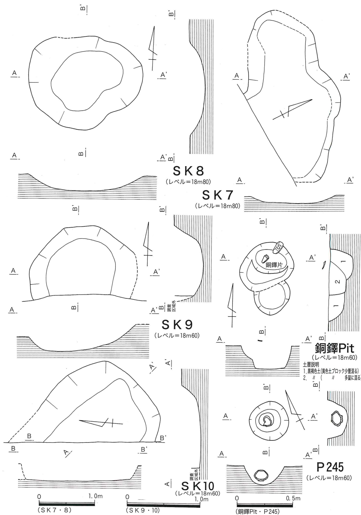
第12図 SK 7~10・銅鐸ピット・P 245 実測図
