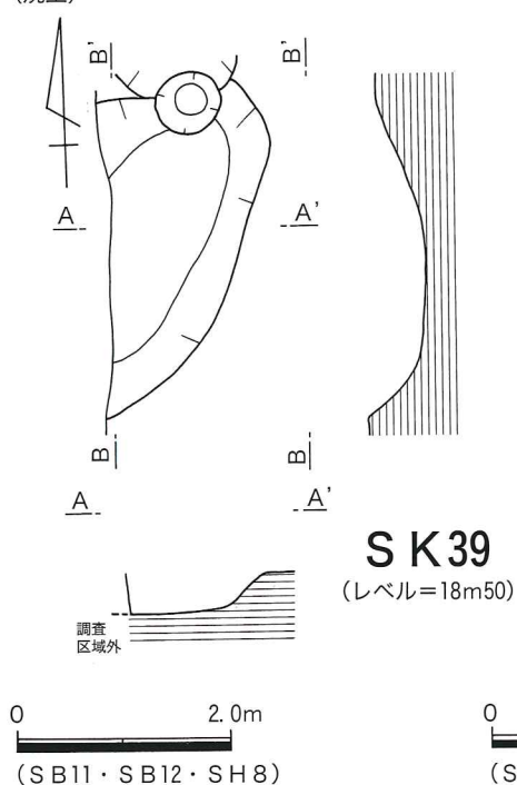
第26図 SB11・12・SH8・SK39・45 実測図
