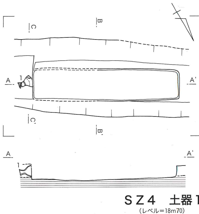
第10図 SZ4 実測図
