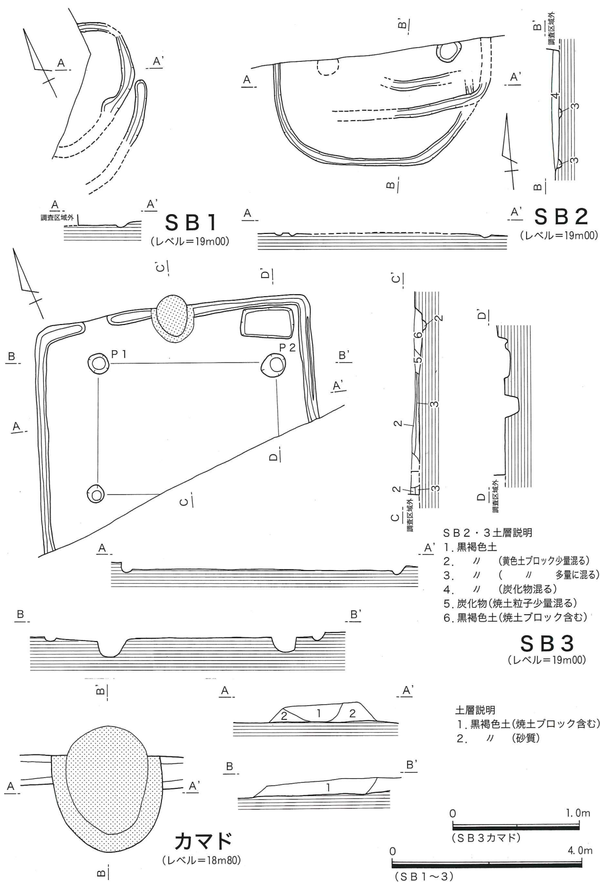
第4図 SB1~3 実測図
