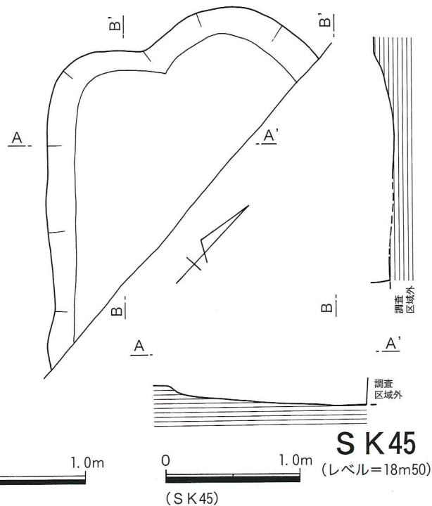
第26図 SB11・12・SH8・SK39・45 実測図
