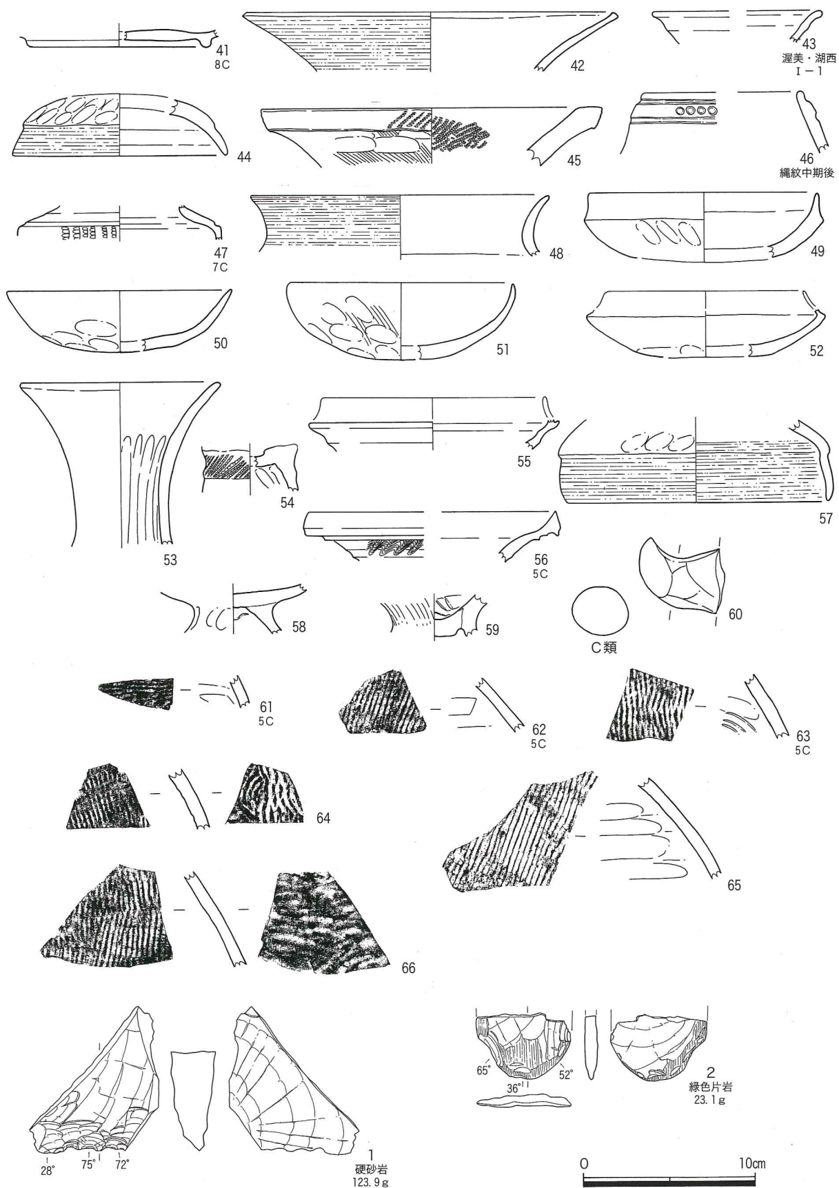
第31図 土器実測図4・石製品実測図1
