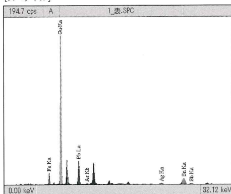
3 銅鐸片表面のXRFスペクトル
