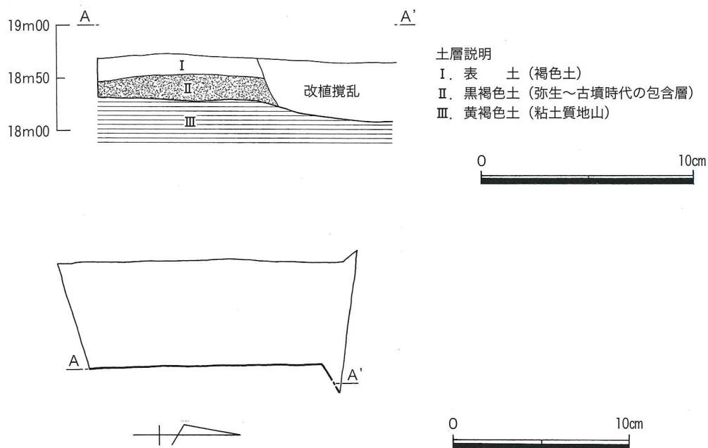
第24図 第10次発掘調査 土層図
