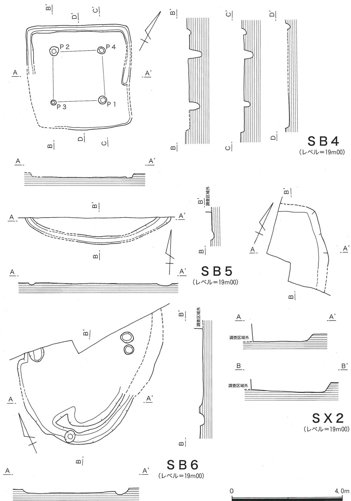
第5図 SB4～6 SX2 実測図
