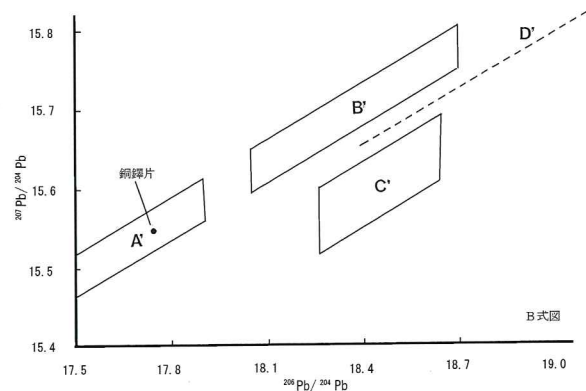
4 掛之上遺跡から出土した銅鐸片の鉛同位体比
