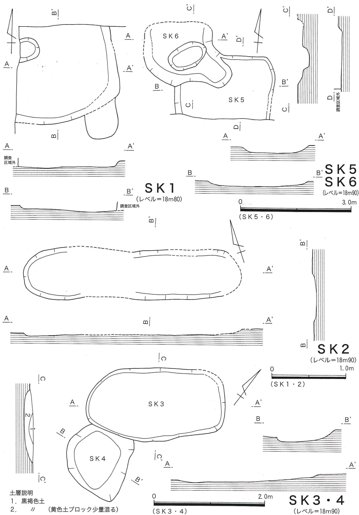
第11図 SK1～6 実測図
