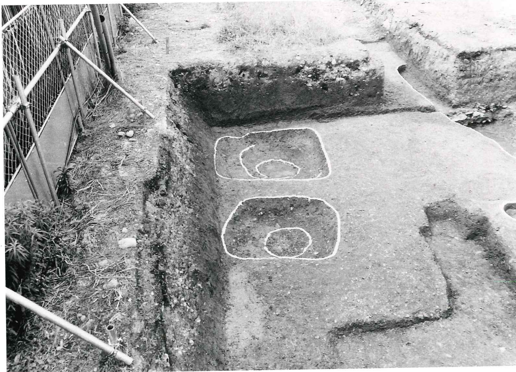
(2) SH6 (奈良時代大 型掘立柱建物か。南 より)
