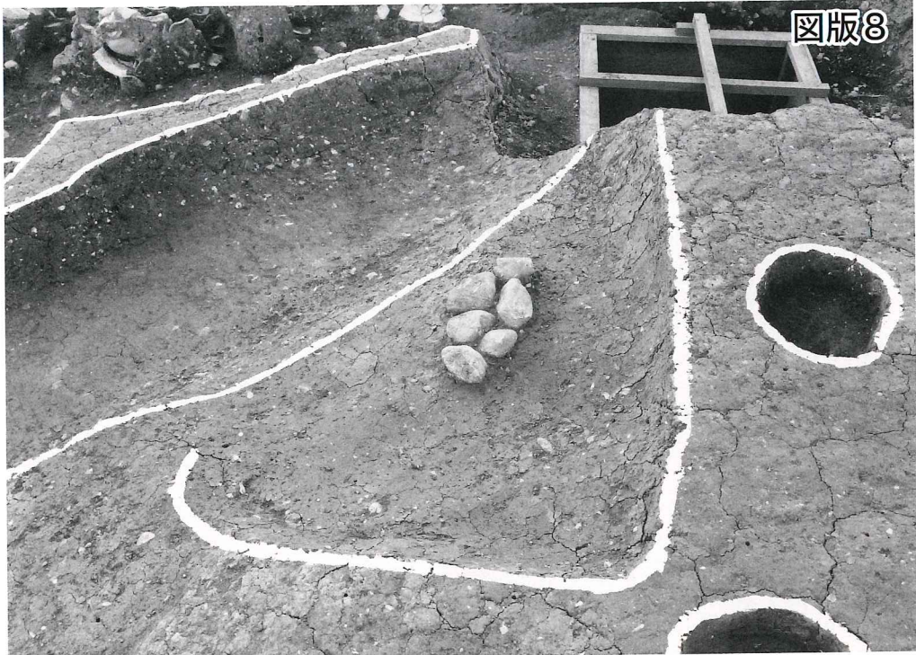
(1) SH1P12 (根固礫 か。東より)
