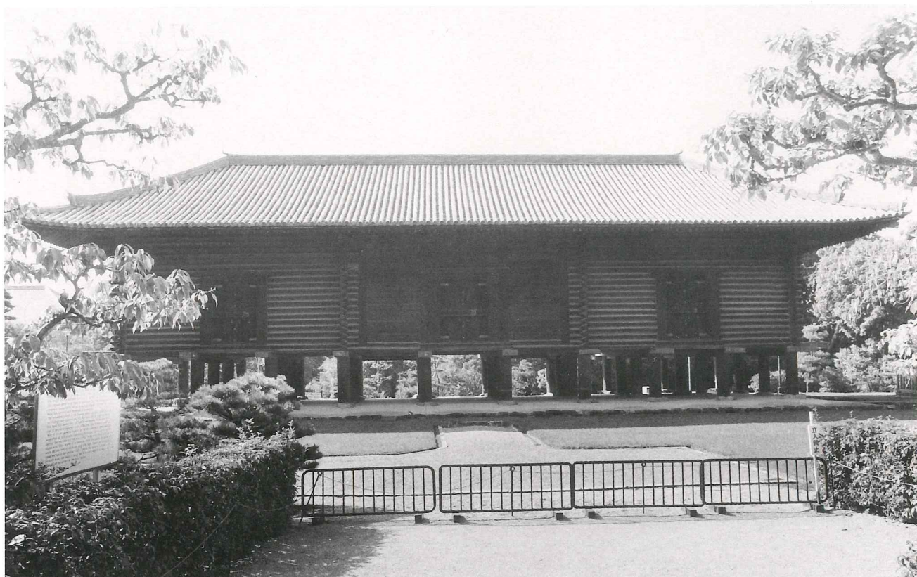
(1) 東大寺正倉院（中央板倉部分が旧形状は壁がない可能性がある。東より）
